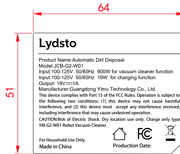
集尘宝铭牌
