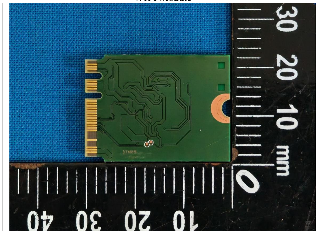
WIFI Module
