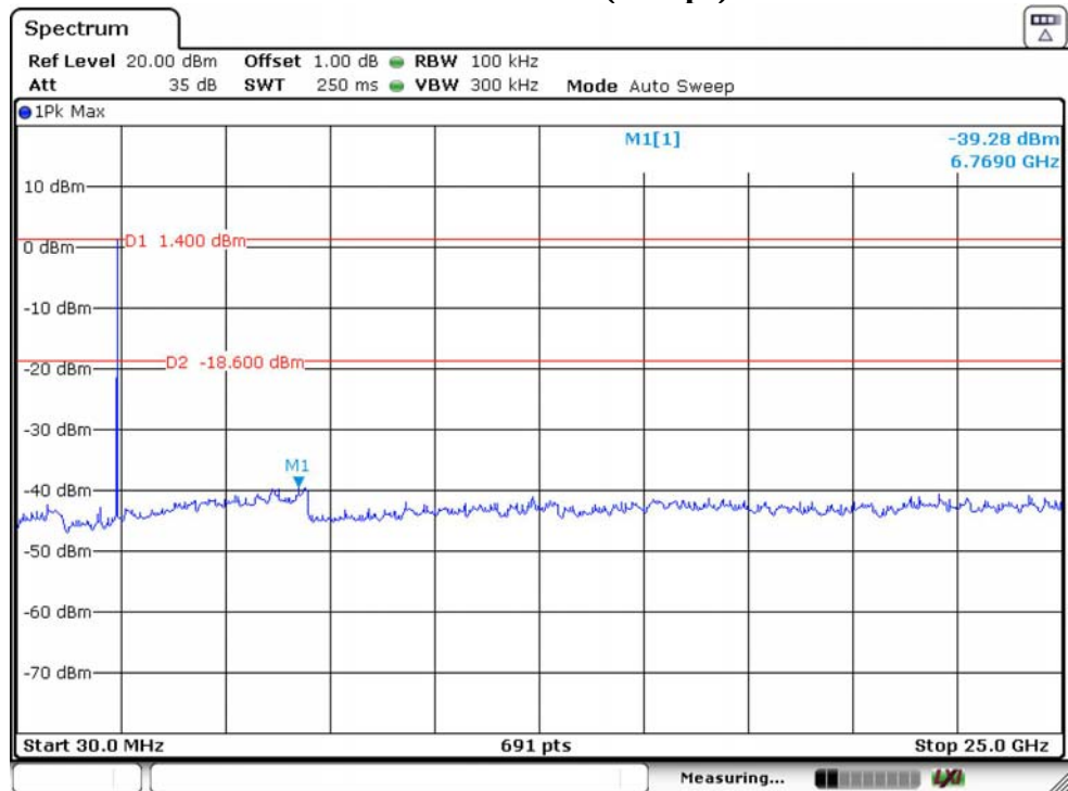
GFSK 2440MHz (2Mbps)
