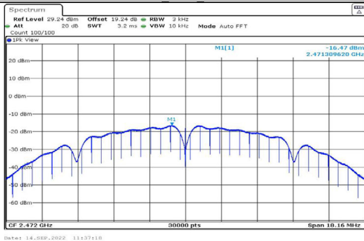
11B Ant1 2472
