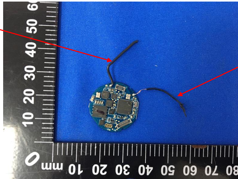
BR/EDR Antenna
