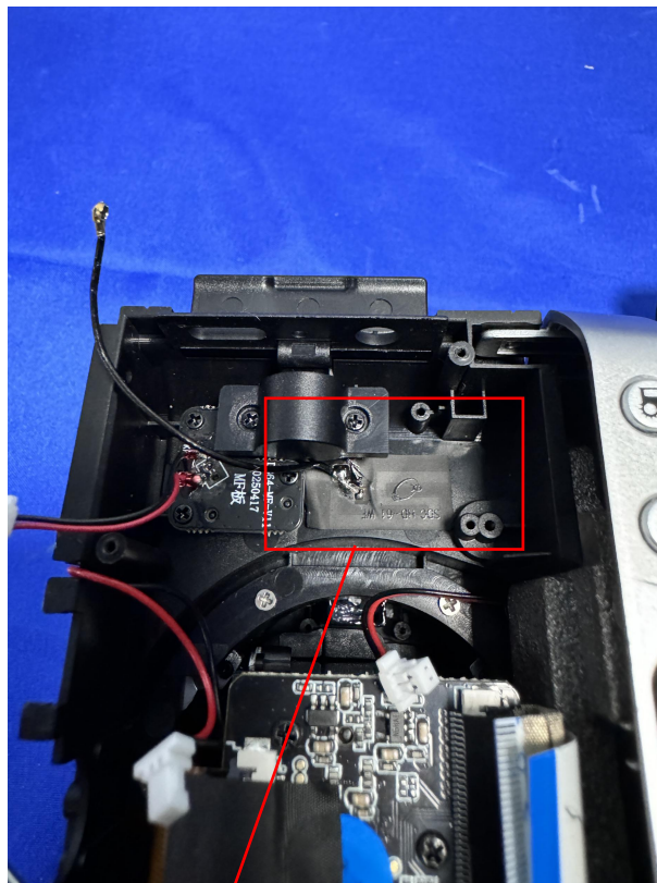
antenna
