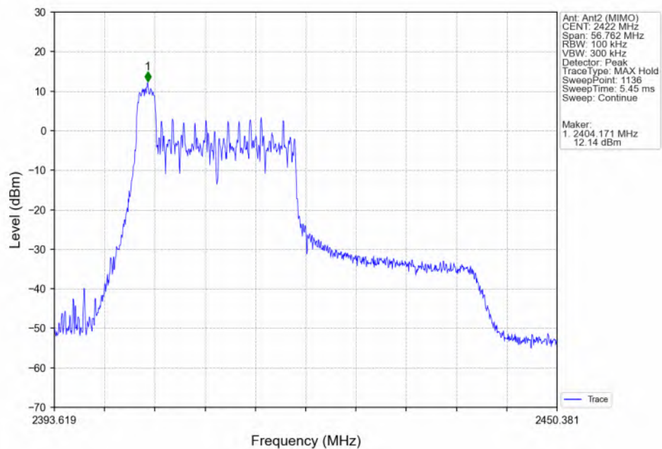
802.11be(EHT40)_LCH_2422MHz_RU26_Left(0)_Ant2 (MIMO)_NTNV
