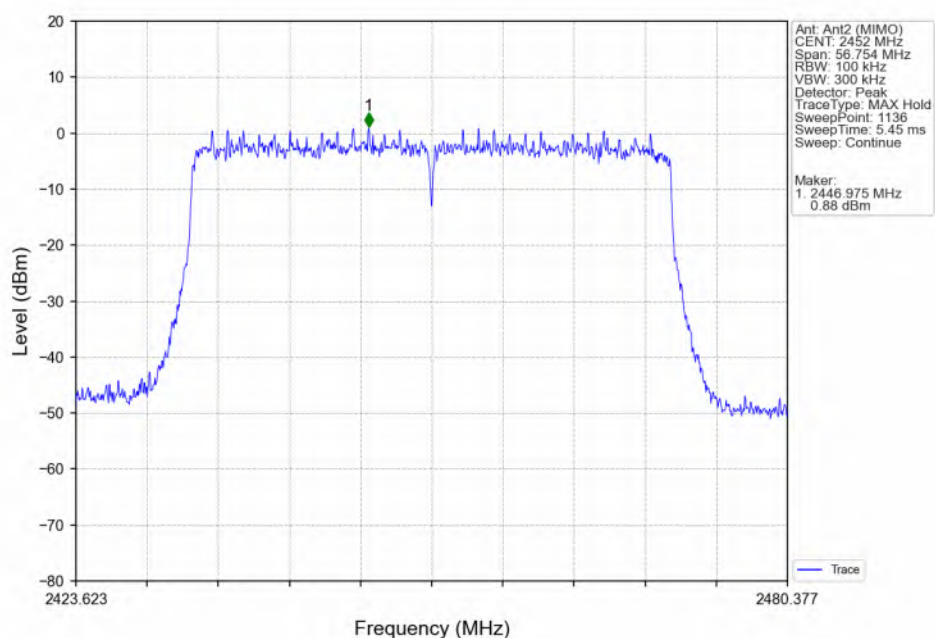
802.11be(EHT40)_HCH_2452MHz_RU484_Left(65)_Ant2 (MIMO)_NTNV
