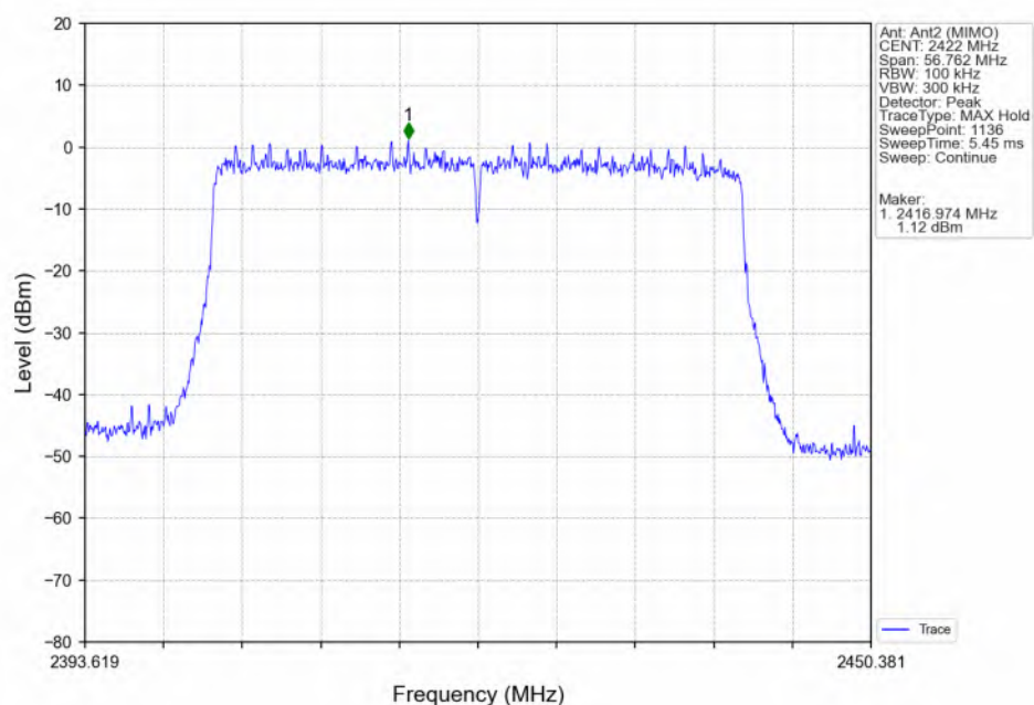
802.11be(EHT40)_LCH_2422MHz_RU484_Left(65)_Ant2 (MIMO)_NTNV
