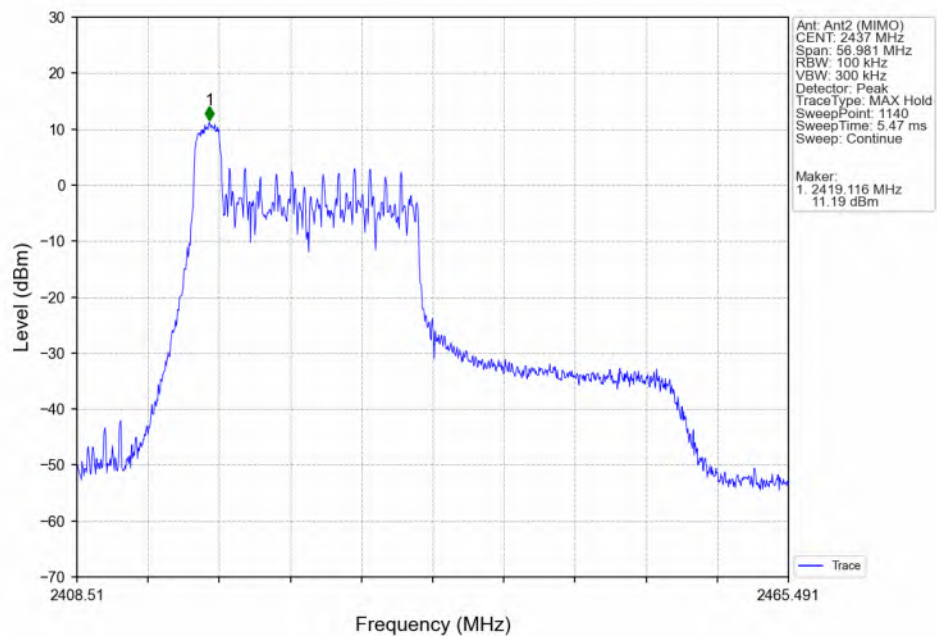
802.11be(EHT40)_MCH_2437MHz_RU26_Left(0)_Ant2 (MIMO)_NTNV
