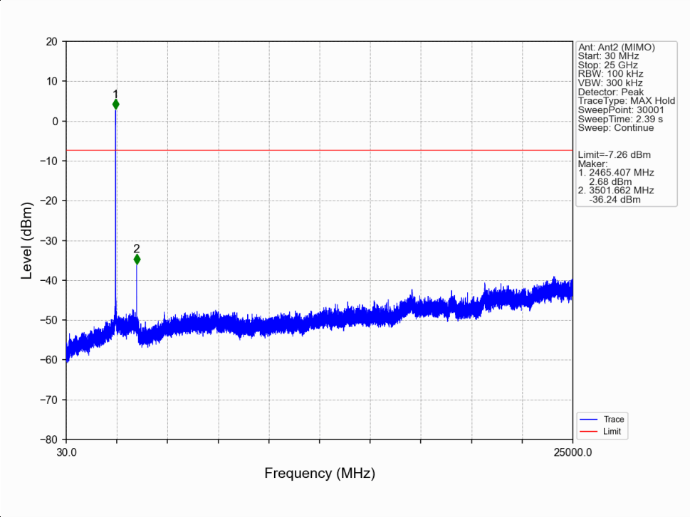
802.11be(EHT20)_HCH_2462MHz_RU242_Left(61)_Ant2 (MIMO)_NTNV
