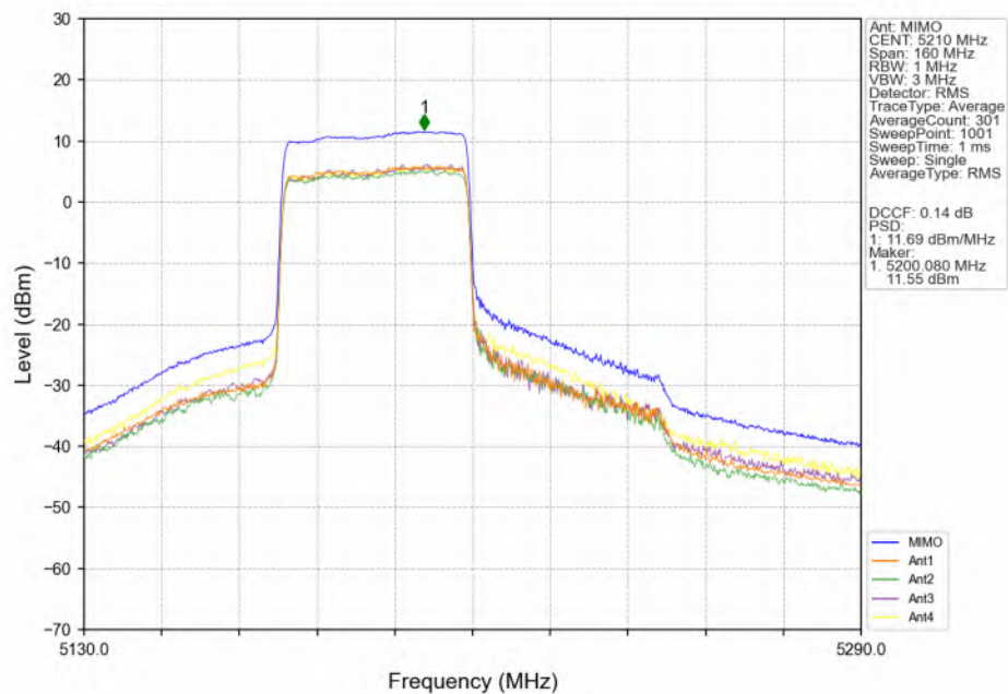
802.11ax(HEW80) MCH_5210MHz_RU484_Left(65)_MIMO_NTNV
