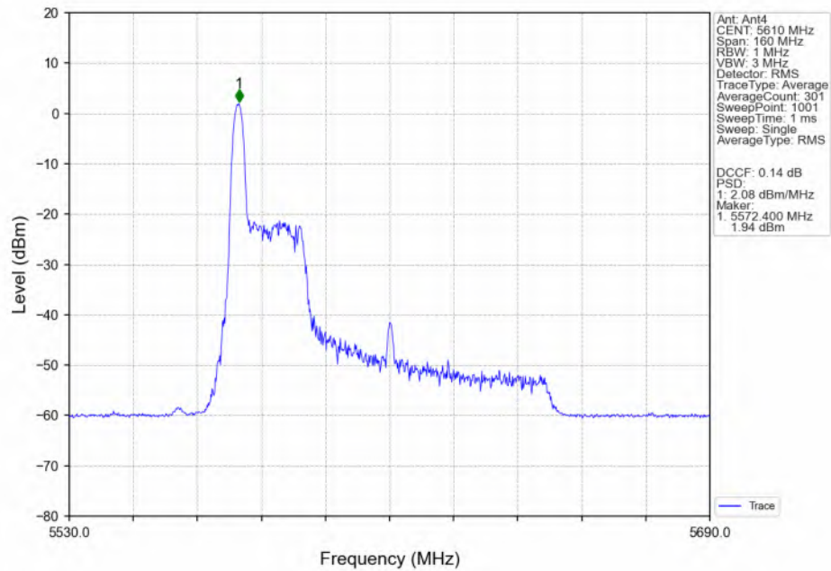
802.11ax(HEW80) HCH_5610MHz_RU26_Left(0)_MIMO_NTNV
