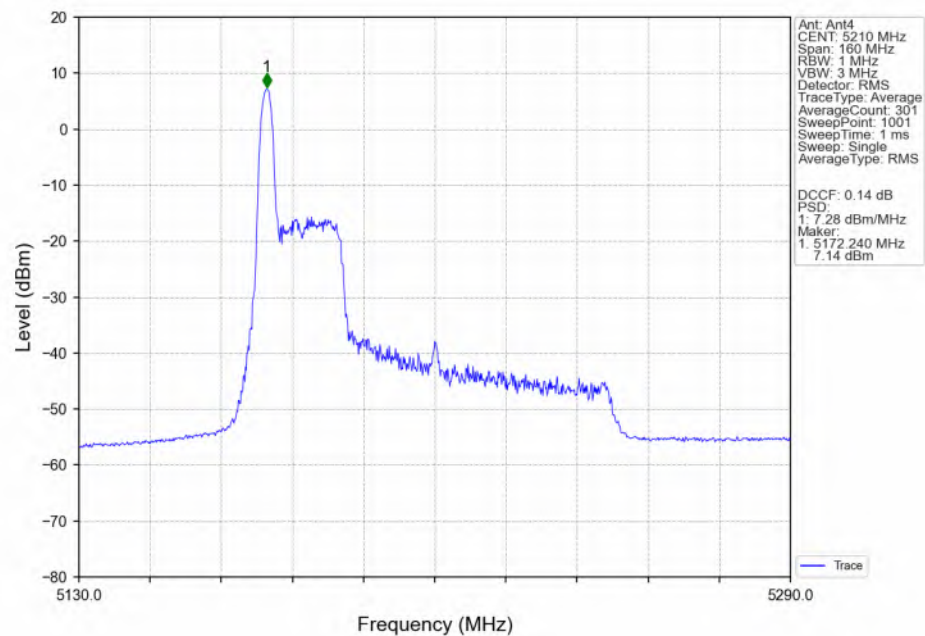
802.11ax(HEW80)_MCH_5210MHz_RU26_Left(0)_Ant4_NTNV
