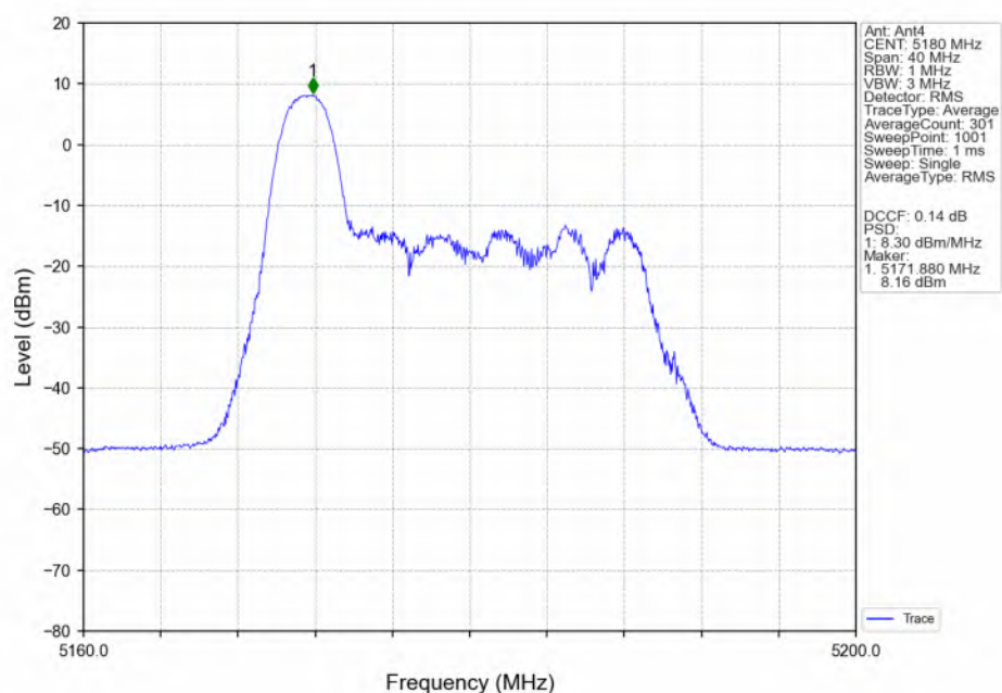
802.11be(EHT20) LCH_5180MHz_RU26_Left(0)_Ant4_NTNV
