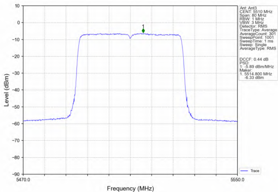
802.11ax(HEW40)_LCH_5510MHz_RU484_Left(65)_Ant3_NTNV
