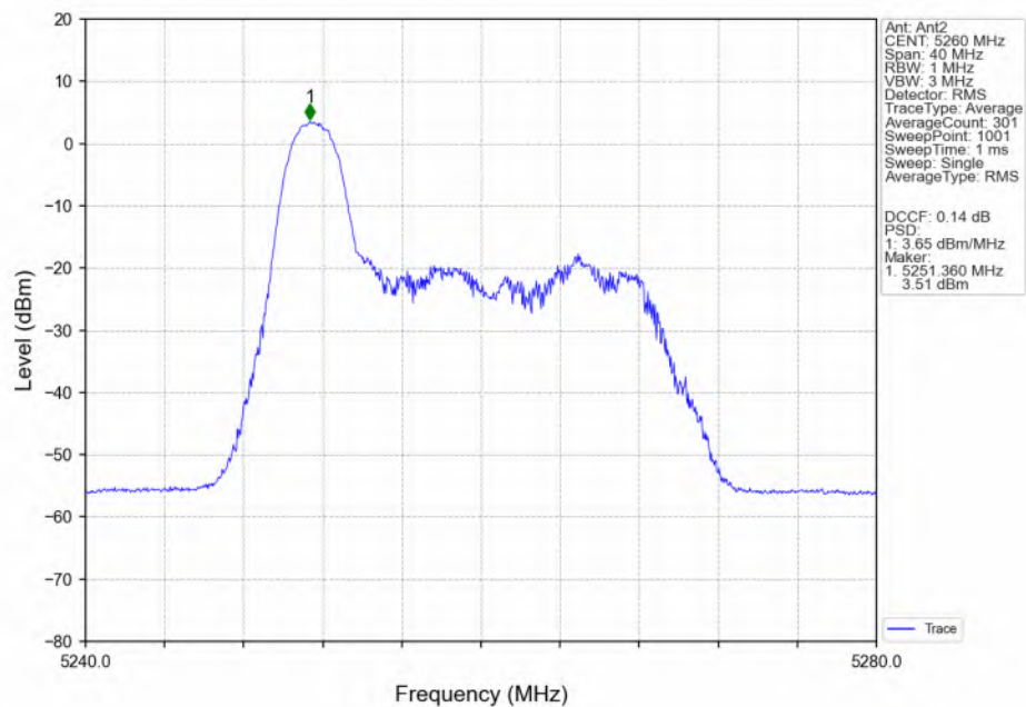
802.11be(EHT20) LCH_5260MHz_RU26_Left(0)_Ant2_NTNV
