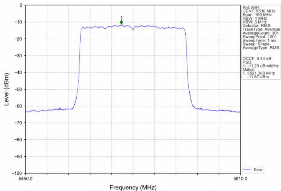
802.11ax(HEW80)_LCH_5530MHz_RU996_Left(67)_Ant4_NTNV
