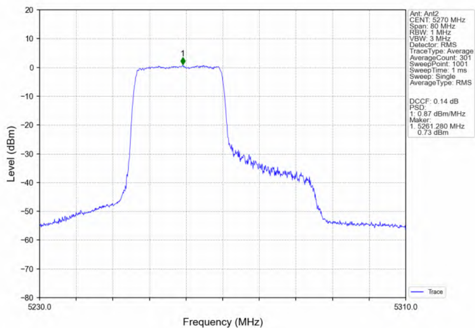
802.11ax(HEW40)_LCH_5270MHz_RU242_Left(61)_Ant2_NTNV
