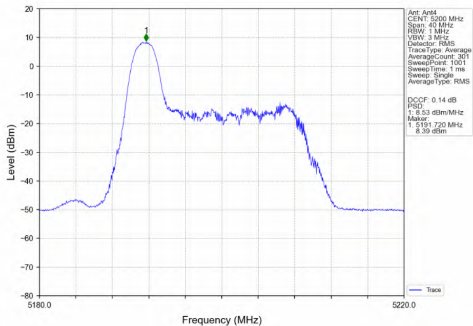
802.11be(EHT20)_MCH_5200MHz_RU26_Left(0)_Ant4_NTNV
