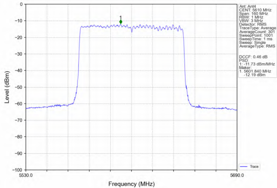
802.11ax(HEW80)_HCH_5610MHz_RU996_Left(67)_MIMO_NTNV
