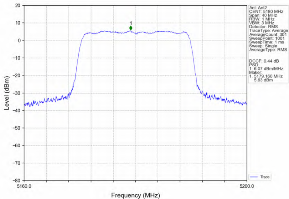
802.11be(EHT20) LCH_5180MHz_RU242_Left(61)_Ant2_NTNV
