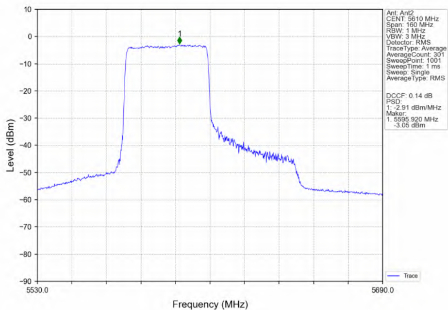
802.11ax(HEW80)_HCH_5610MHz_RU484_Left(65)_Ant2_NTNV
