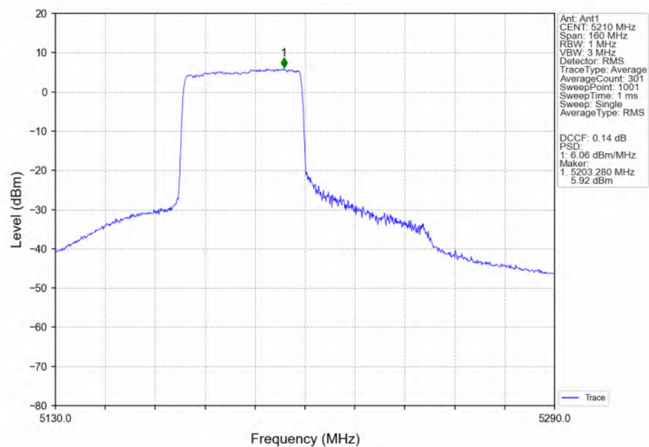
802.11ax(HEW80)_MCH_5210MHz_RU484_Left(65)_Ant1_NTNV
