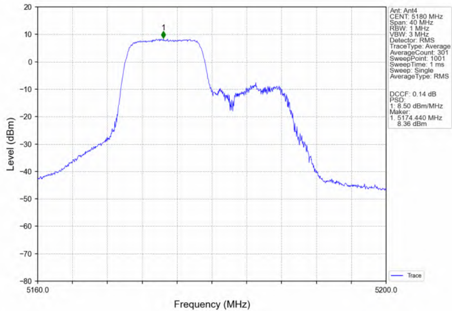
802.11be(EHT20) LCH 5180MHz RU106 Left(53) MIMO NTN
