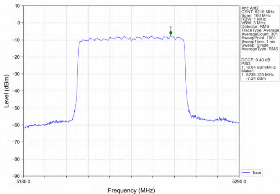
802.11ax(HEW80) MCH_5210MHz_RU996_Left(67)_Ant2_NTNV
