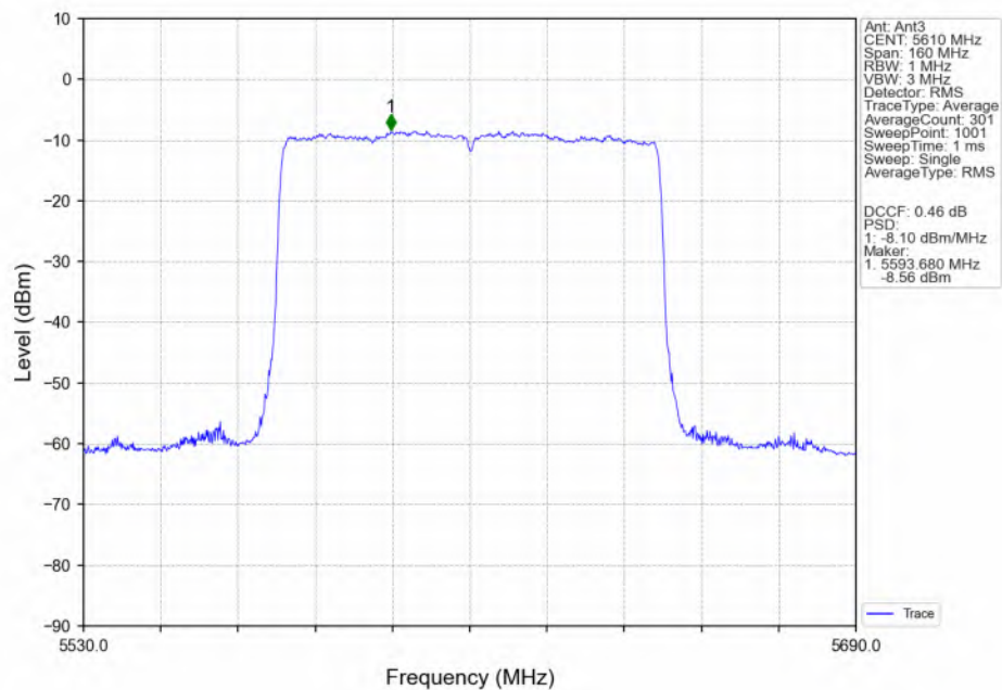
802.11ax(HEW80)_HCH_5610MHz_RU996_Left(67)_Ant3_NTNV
