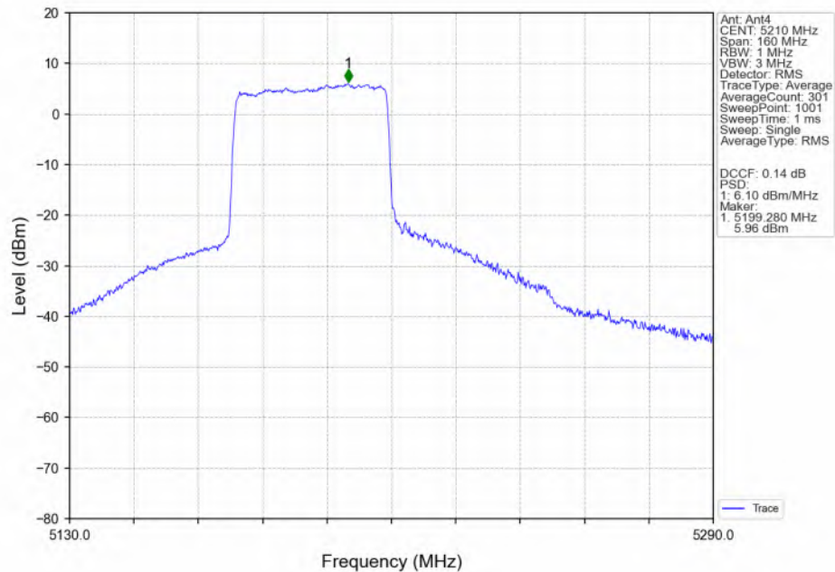
802.11ax(HEW80) MCH_5210MHz_RU484_Left(65)_MIMO_NTNV
