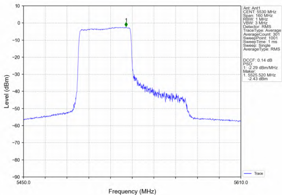
802.11ax(HEW80)_LCH_5530MHz_RU484_Left(65)_Ant1_NTNV
