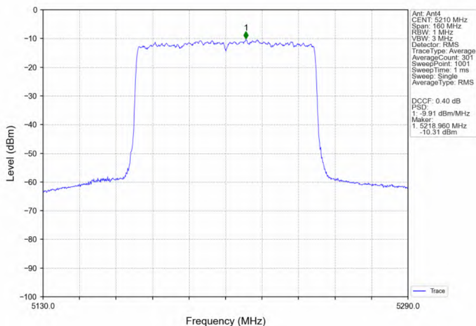
802.11ax(HEW80) MCH_5210MHz_RU996_Left(67)_Ant4_NTNV
