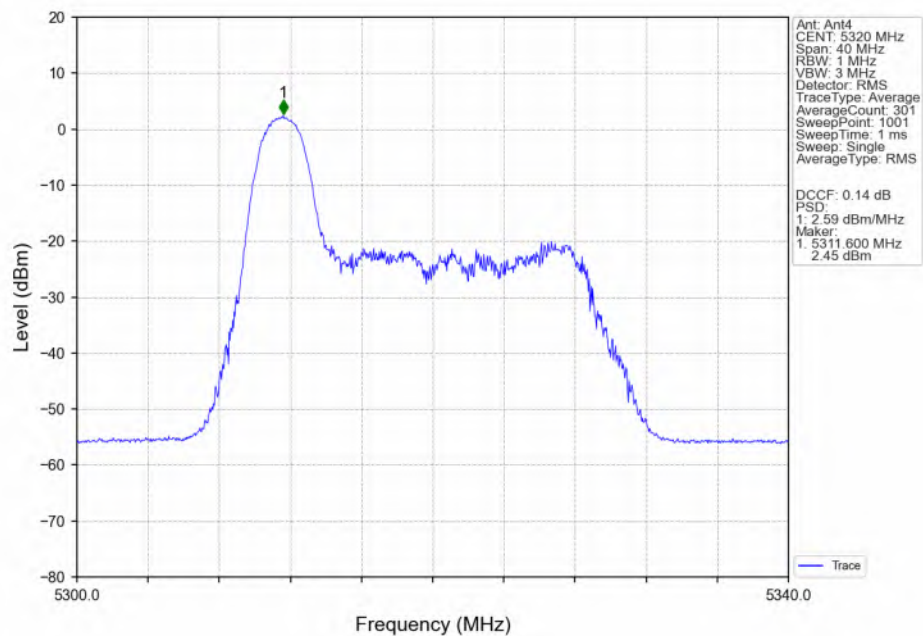
802.11be(EHT20)_HCH_5320MHz_RU26_Left(0)_Ant4_NTNV
