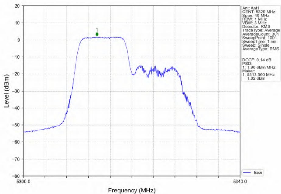
802.11be(EHT20)_HCH_5320MHz_RU106_Left(53)_Ant1_NTNV
