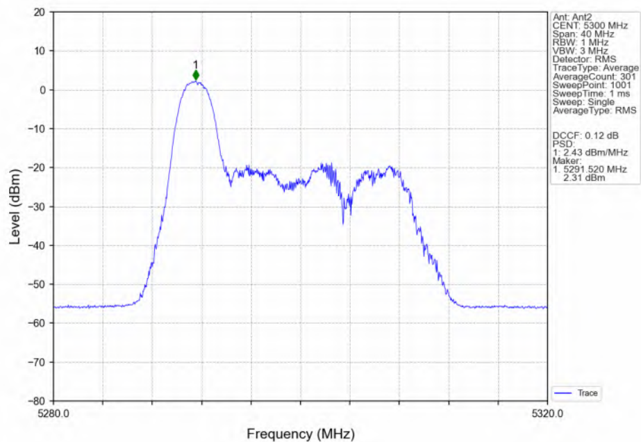
802.11be(EHT20)_MCH_5300MHz_RU26_Left(0)_Ant2_NTNV
