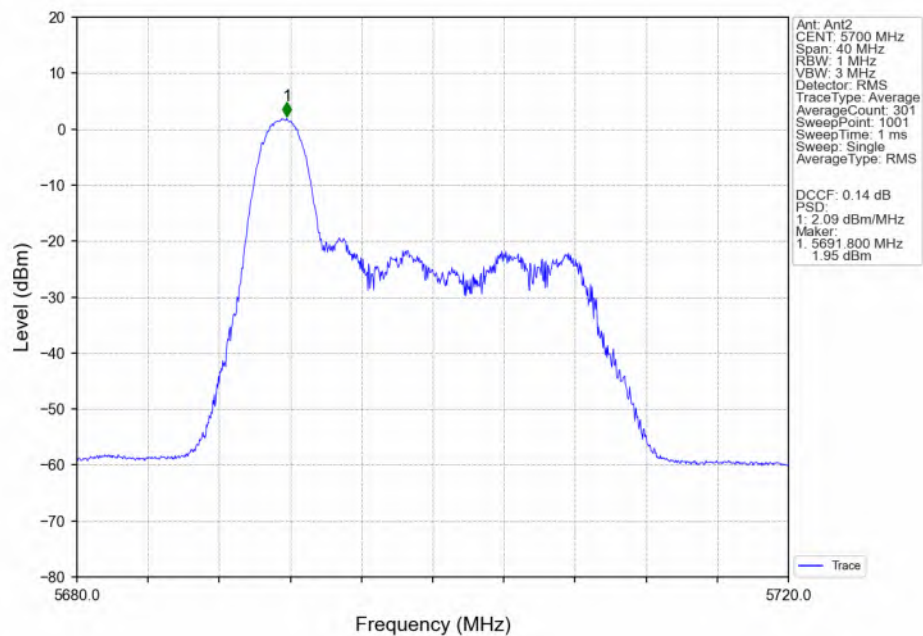
802.11be(EHT20)_HCH_5700MHz_RU26_Left(0)_Ant2_NTNV
