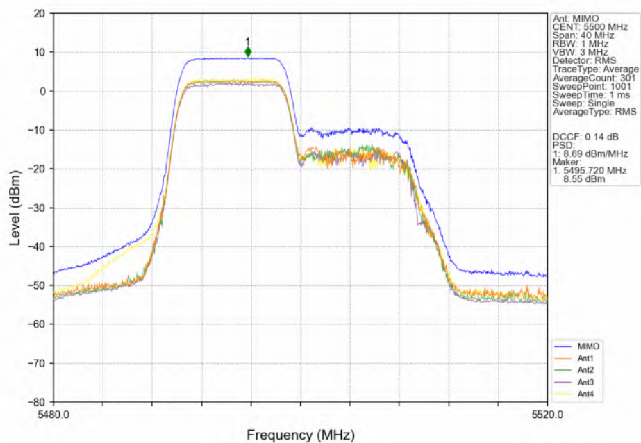
802.11be(EHT20)_LCH_5500MHz_RU106_Left(53)_MIMO_NTNV
