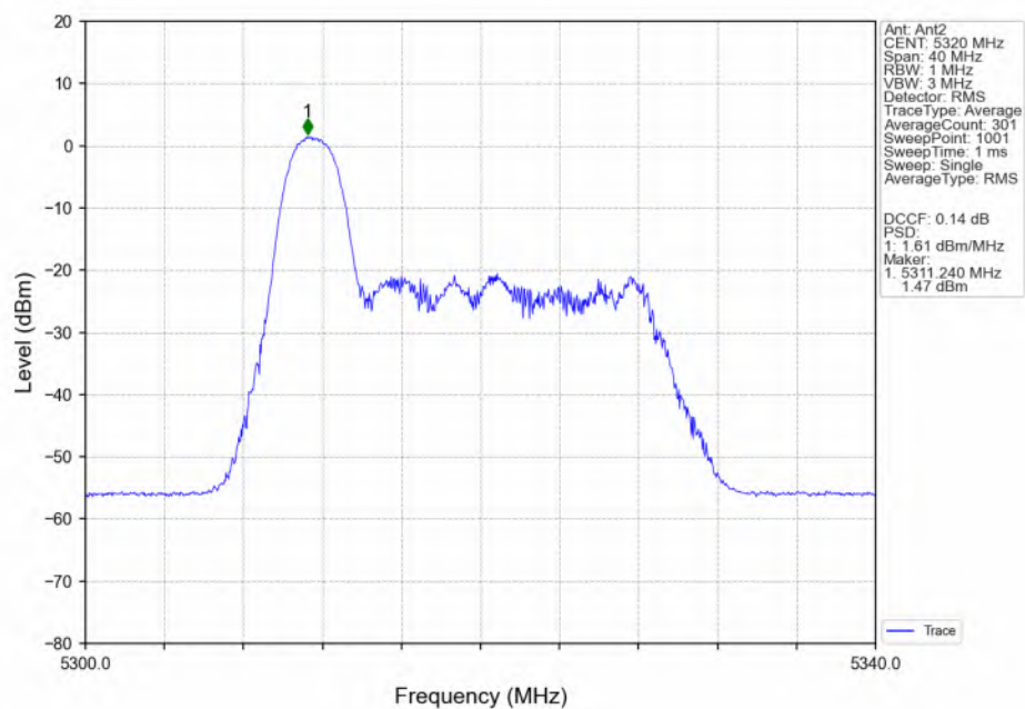
802.11be(EHT20)_HCH_5320MHz_RU26_Left(0)_Ant2_NTNV
