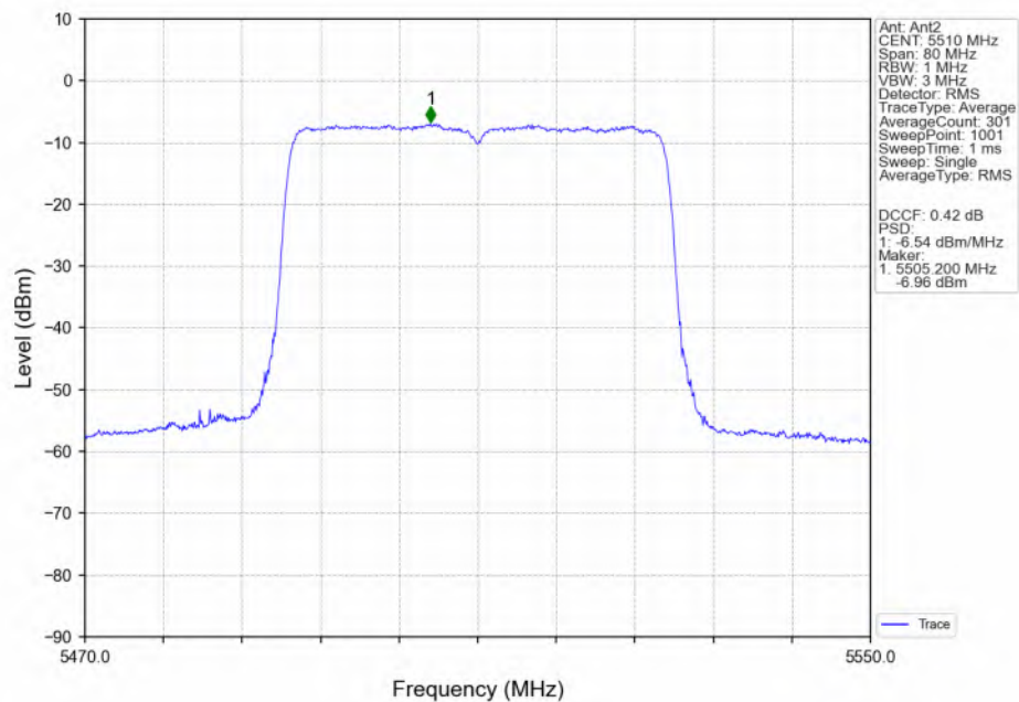
802.11be(EHT40) LCH_5510MHz_RU484_Left(65)_Ant2_NTNV
