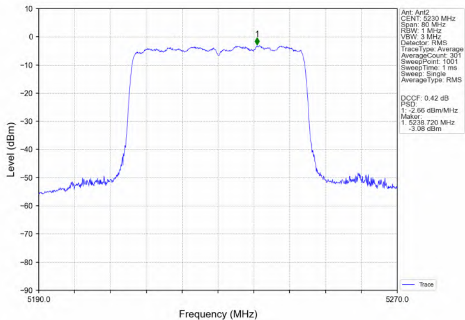
802.11be(EHT40)_HCH_5230MHz_RU484_Left(65)_Ant2_NTNV
