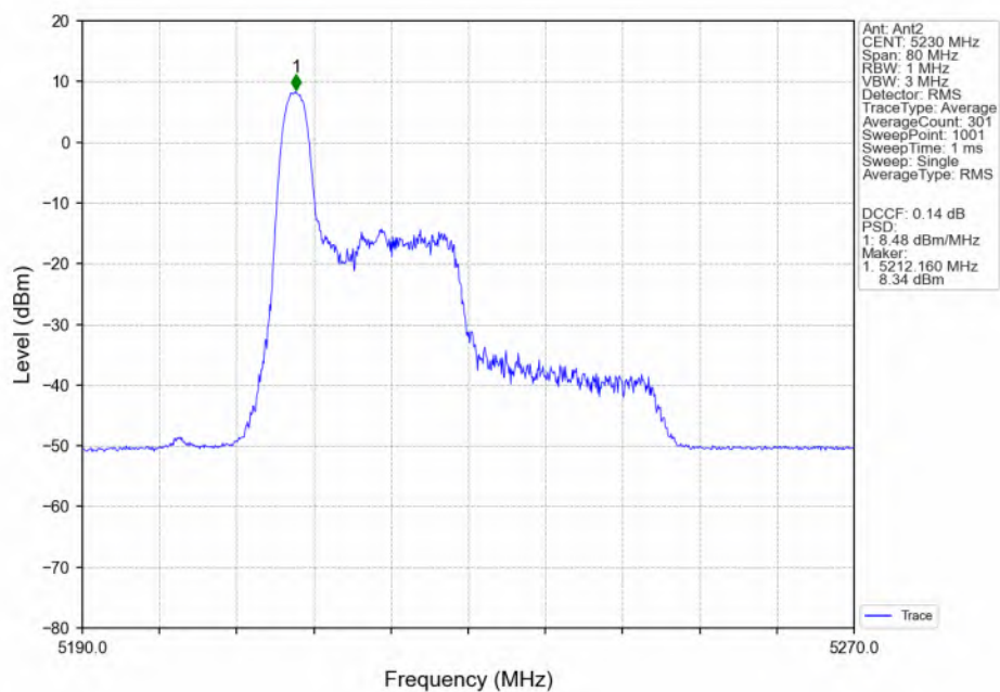
802.11be(EHT40)_HCH_5230MHz_RU26_Left(0)_Ant2_NTNV
