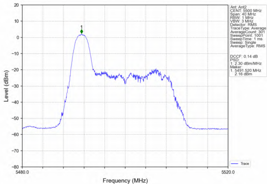
802.11be(EHT20) LCH_5500MHz_RU26_Left(0)_Ant2_NTNV
