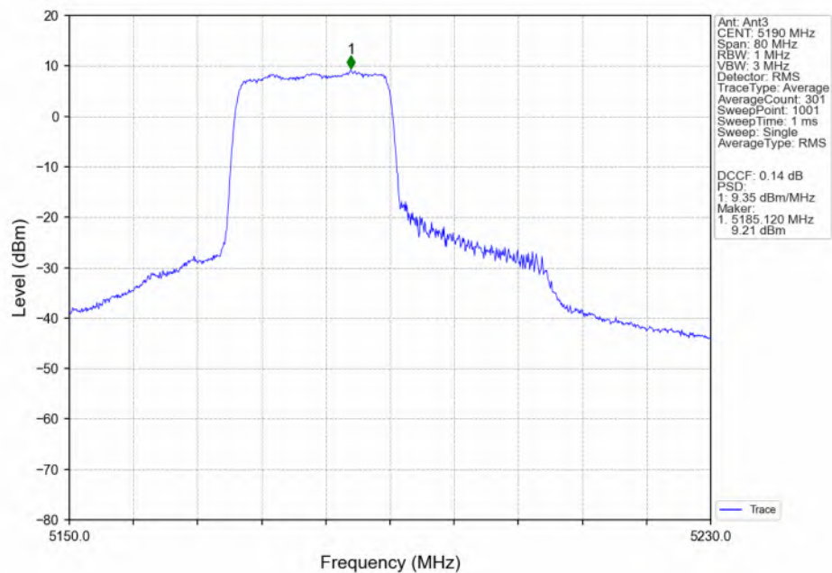
802.11be(EHT40) LCH_5190MHz_RU242_Left(61)_Ant3_NTNV
