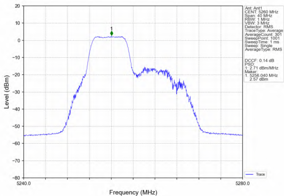
802.11be(EHT20)_LCH_5260MHz_26+52_ / _Ant1_NTNV
