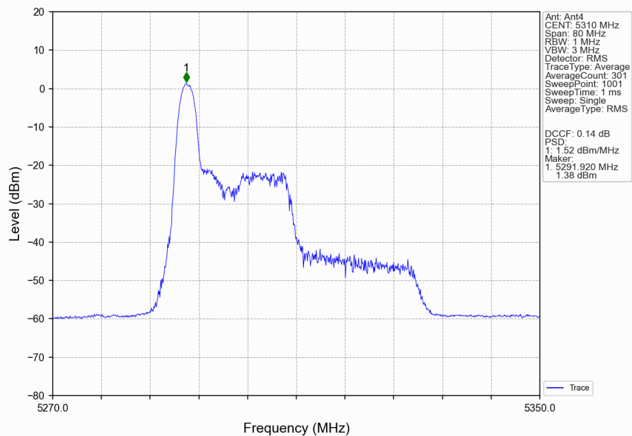
802.11be(EHT40)_HCH_5310MHz_RU26_Left(0)_Ant4_NTNV
