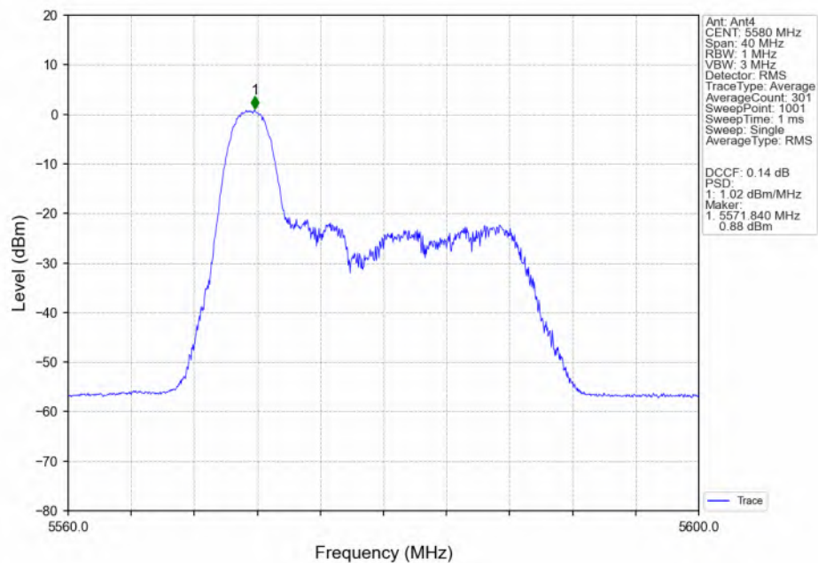
802.11be(EHT20)_MCH_5580MHz_RU26_Left(0)_Ant4_NTNV
