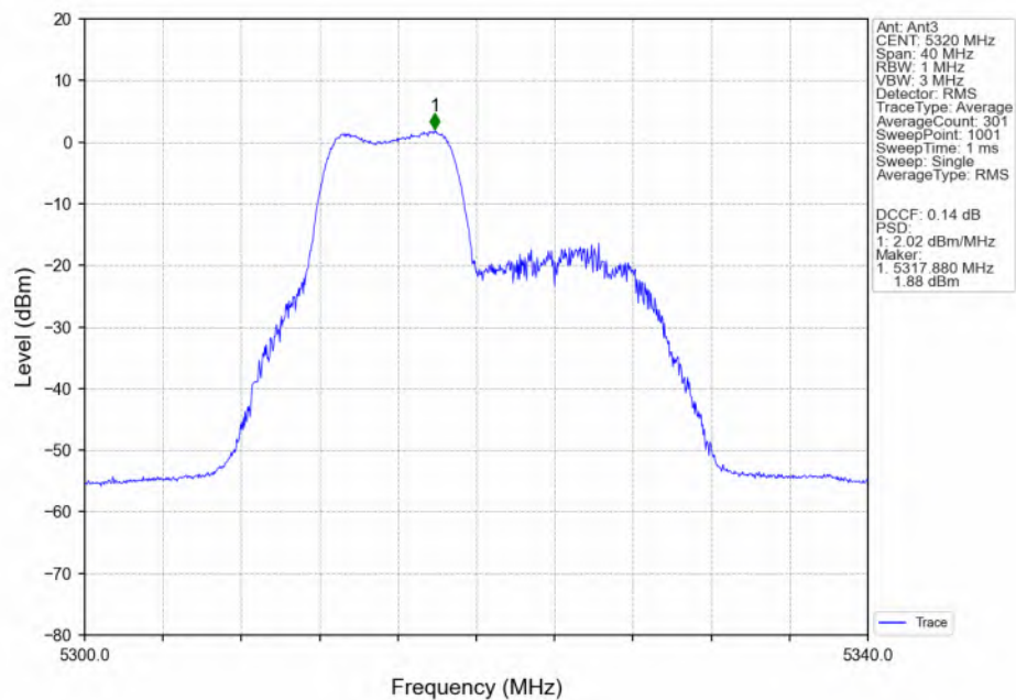
802.11be(EHT20)_HCH_5320MHz_26+52_ / Ant3_NTNV
