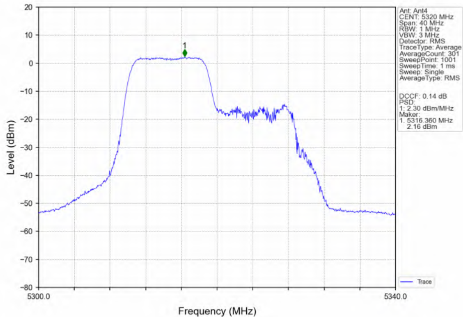
802.11be(EHT20)_HCH_5320MHz_RU106_Left(53)_MIMO_NTNV
