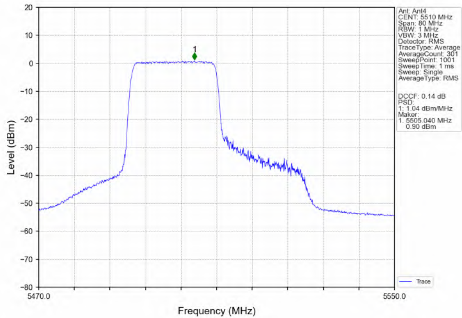
802.11be(EHT40) LCH 5510MHz RU242 Left(61) MIMO NTN
