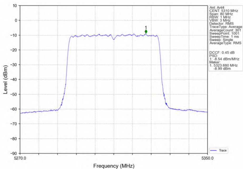
802.11be(EHT40)_HCH_5310MHz_RU484_Left(65)_Ant4_NTNV
