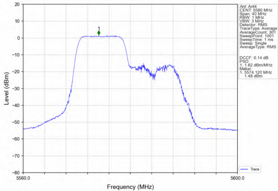
802.11be(EHT20)_MCH_5580MHz_RU106_Left(53)_MIMO_NTNV
