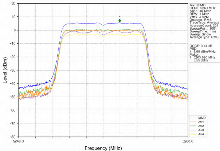
802.11be(EHT20)_LCH_5260MHz_26+52_ / _Ant1_NTNV
