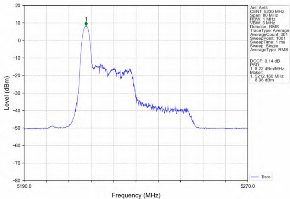
802.11be(EHT40)_HCH_5230MHz_RU26_Left(0)_Ant4_NTNV
