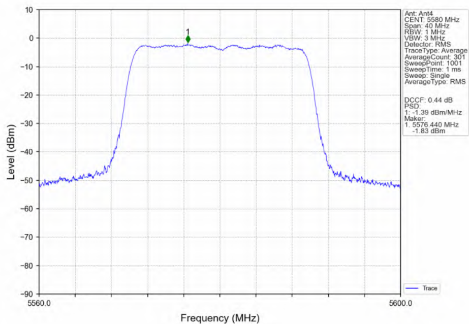
802.11be(EHT20)_MCH_5580MHz_RU242_Left(61)_Ant4_NTNV
