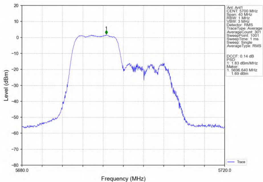
802.11be(EHT20)_HCH_5700MHz_RU106_Left(53)_Ant1_NTNV
