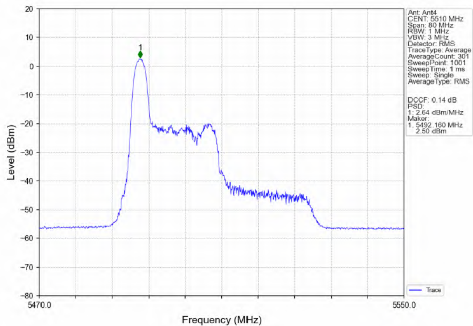
802.11be(EHT40) LCH_5510MHz_RU26_Left(0)_Ant4_NTNV
