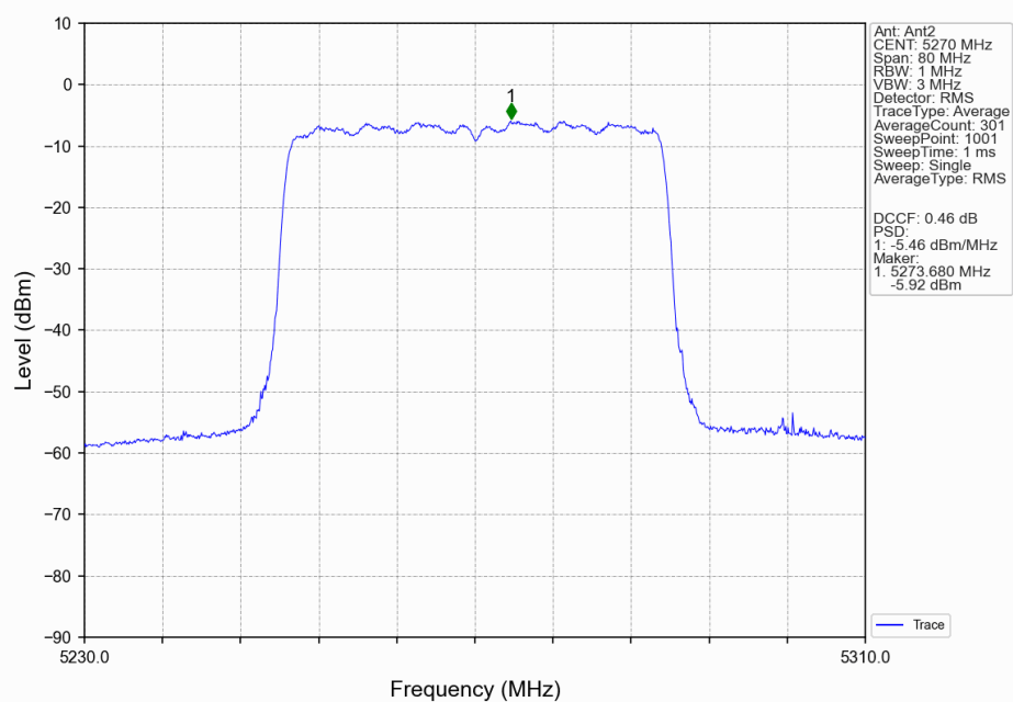
802.11be(EHT40) LCH_5270MHz_RU484_Left(65)_Ant2_NTNV
