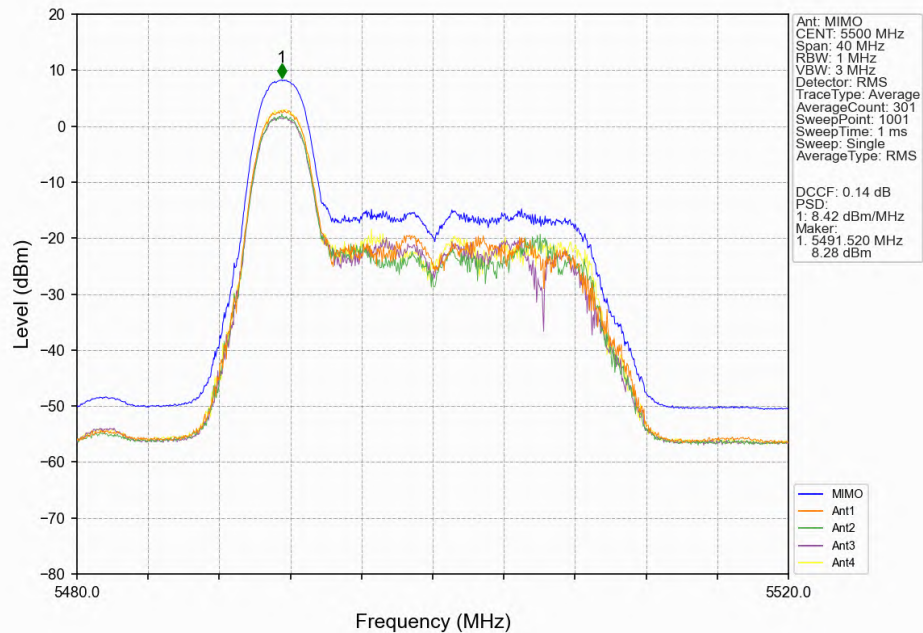
802.11be(EHT20) LCH_5500MHz_RU26 Left(0) MIMO_NTNV
