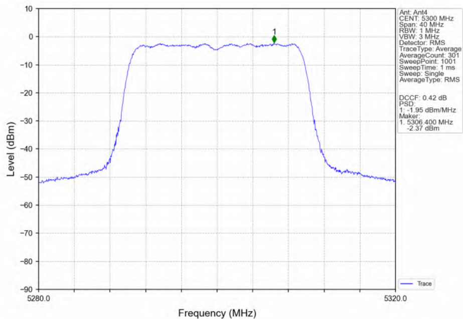
802.11be(EHT20)_MCH_5300MHz_RU242_Left(61)_Ant4_NTNV
