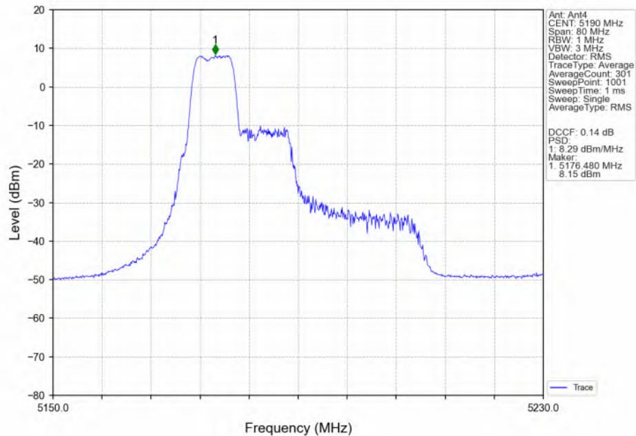
802.11be(EHT40) LCH_5190MHz_26+52 / MIMO_NTNV
