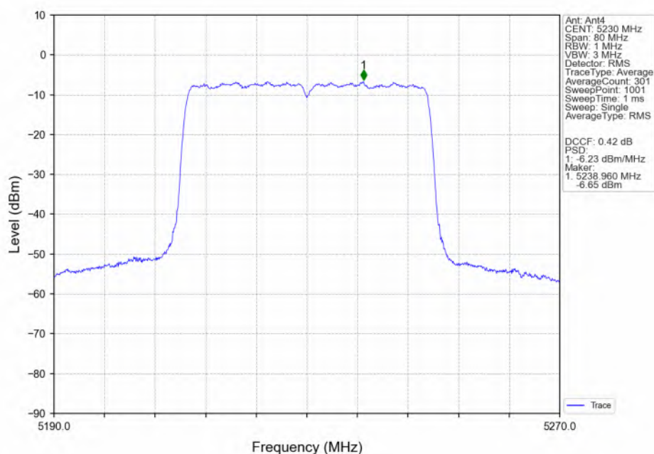
802.11be(EHT40)_HCH_5230MHz_RU484_Left(65)_Ant4_NTNV
