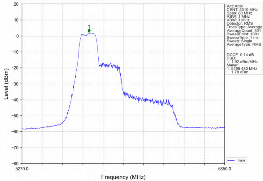
802.11be(EHT40)_HCH_5310MHz_26+52_ / MIMO_NTNV
