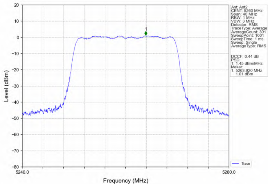
802.11be(EHT20) LCH_5260MHz_RU242_Left(61)_Ant2_NTNV
