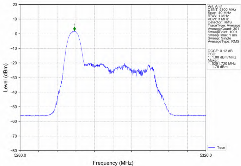
802.11be(EHT20)_MCH_5300MHz_RU26_Left(0)_Ant4_NTNV
