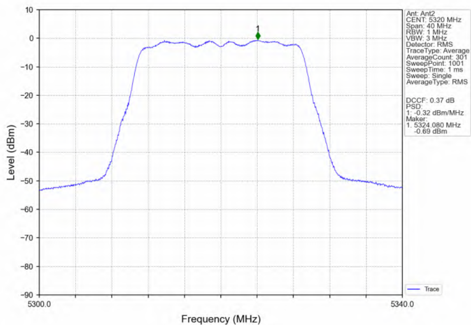
802.11be(EHT20)_HCH_5320MHz_RU242_Left(61)_Ant2_NTNV
