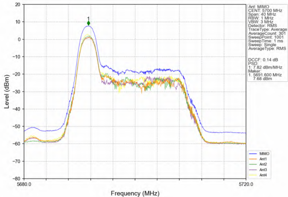
802.11be(EHT20)_HCH_5700MHz_RU106_Left(53)_Ant1_NTNV
