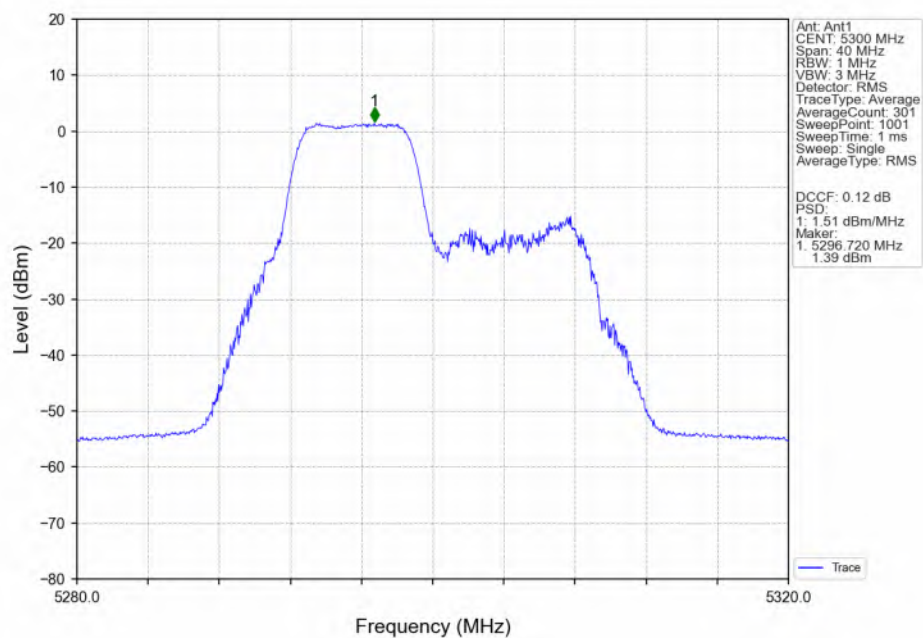
802.11be(EHT20)_MCH_5300MHz_26+52_/_Ant1_NTNV
