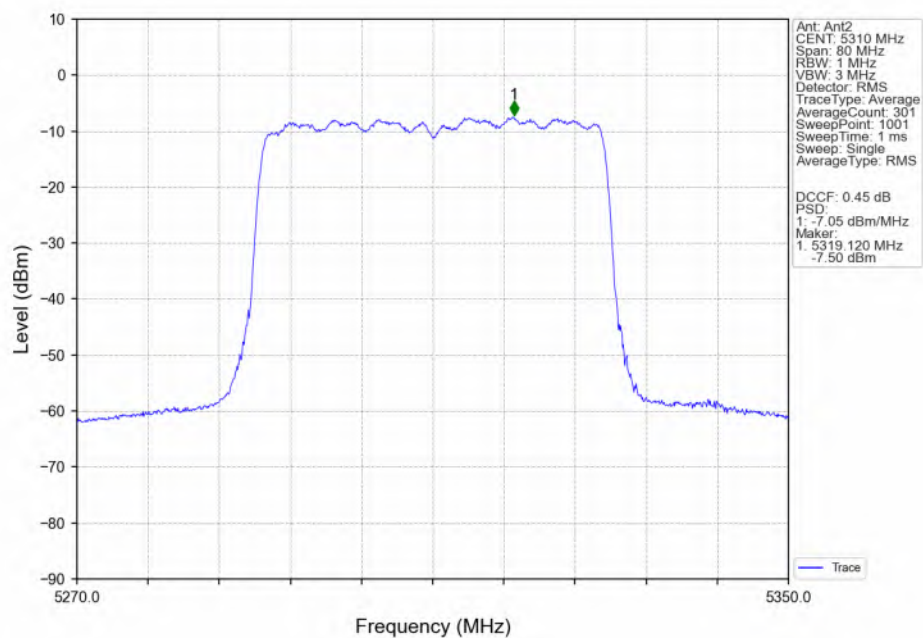
802.11be(EHT40)_HCH_5310MHz_RU484_Left(65)_Ant2_NTNV
