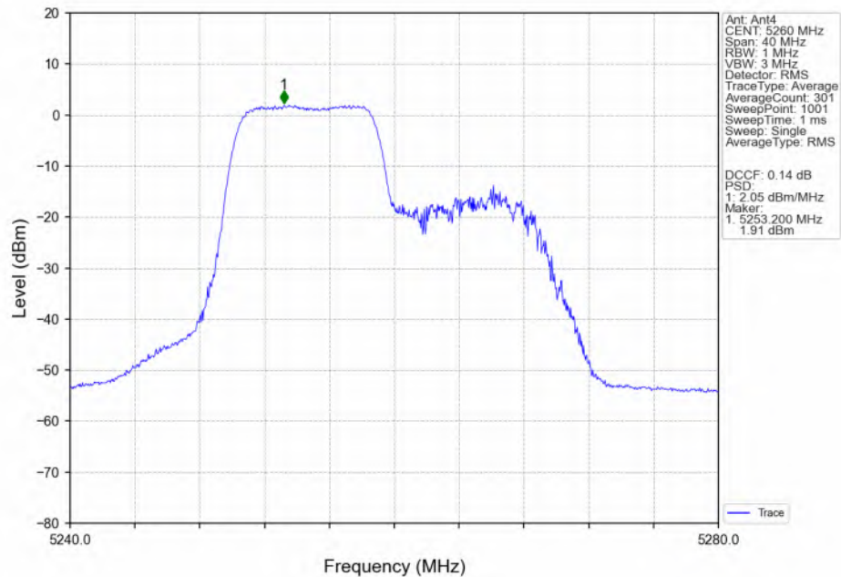
802.11be(EHT20) LCH 5260MHz RU106 Left(53) MIMO NTN
