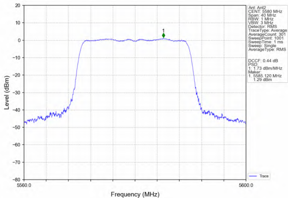
802.11be(EHT20)_MCH_5580MHz_RU242_Left(61)_Ant2_NTNV
