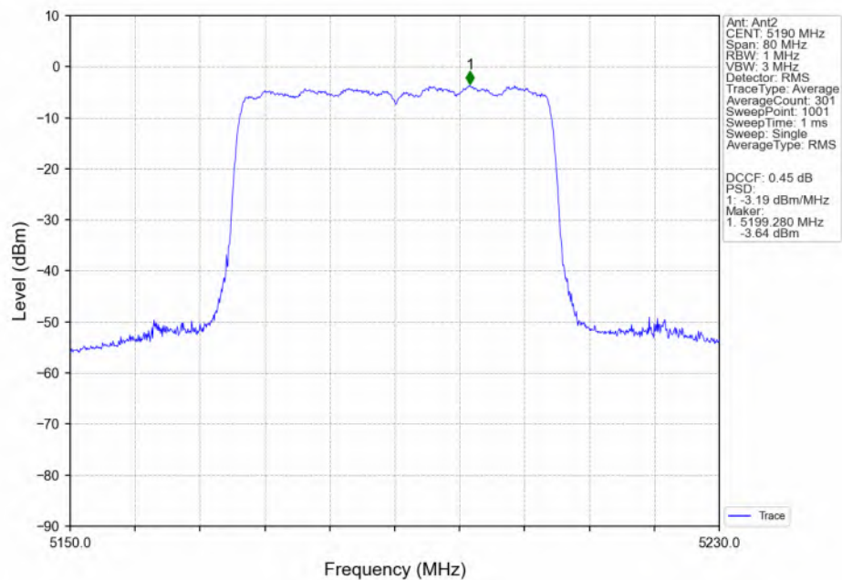
802.11be(EHT40) LCH_5190MHz_RU484_Left(65)_Ant2_NTNV
