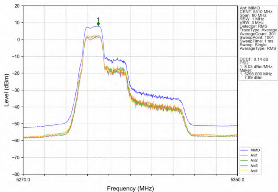
802.11be(EHT40)_HCH_5310MHz_26+52_ / MIMO_NTNV
