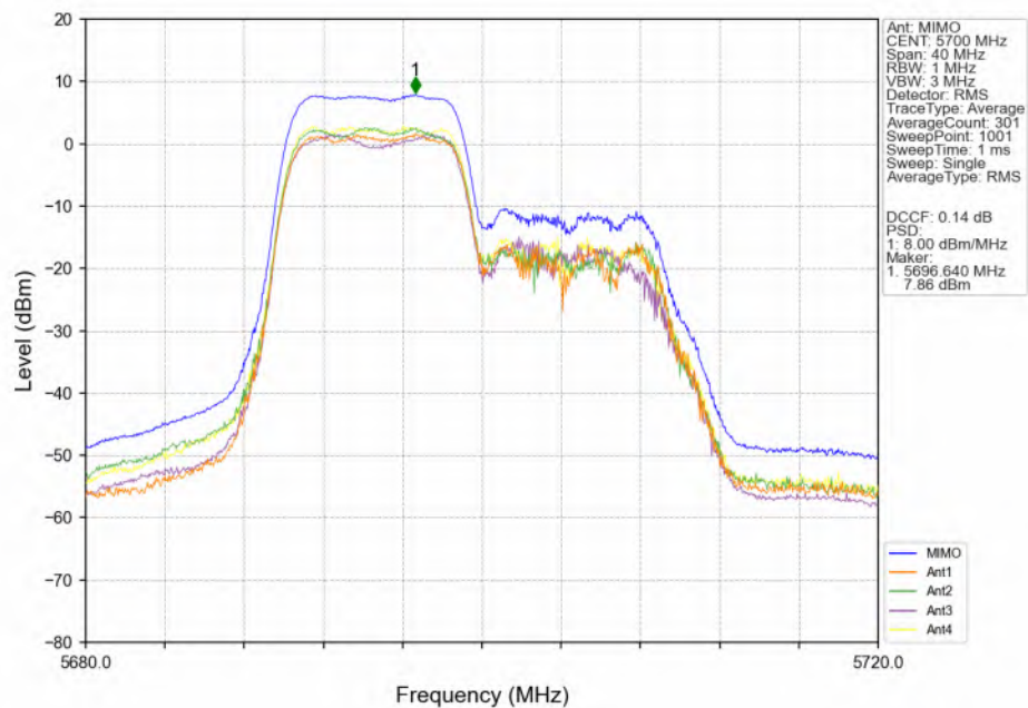
802.11be(EHT20)_HCH_5700MHz_RU106_Left(53)_MIMO_NTNV
