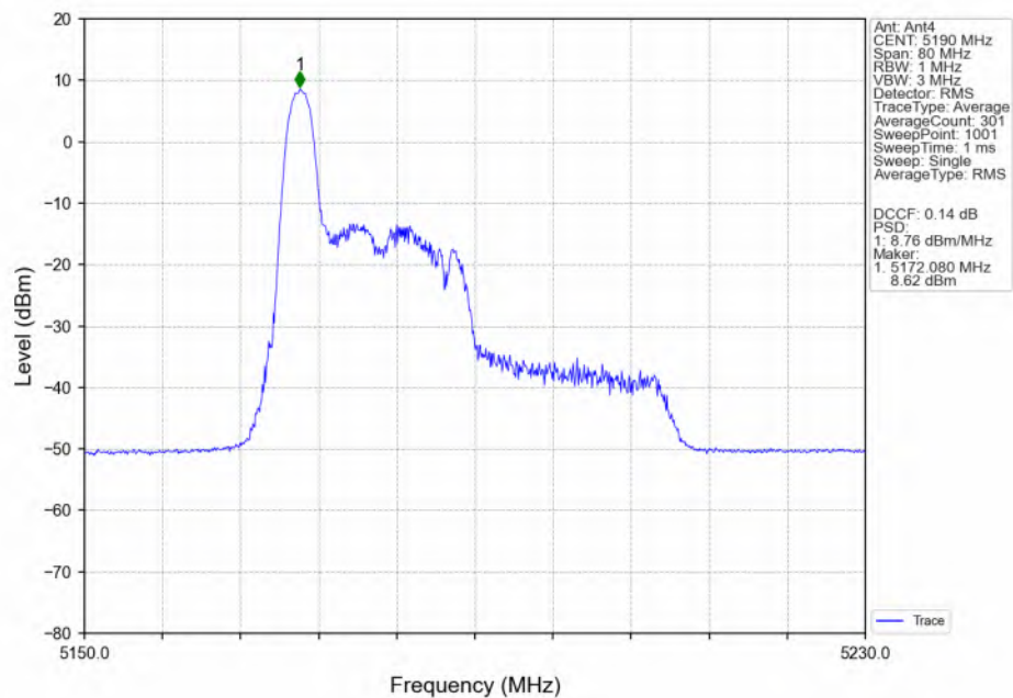
802.11be(EHT40) LCH_5190MHz_RU26_Left(0)_Ant4_NTNV
