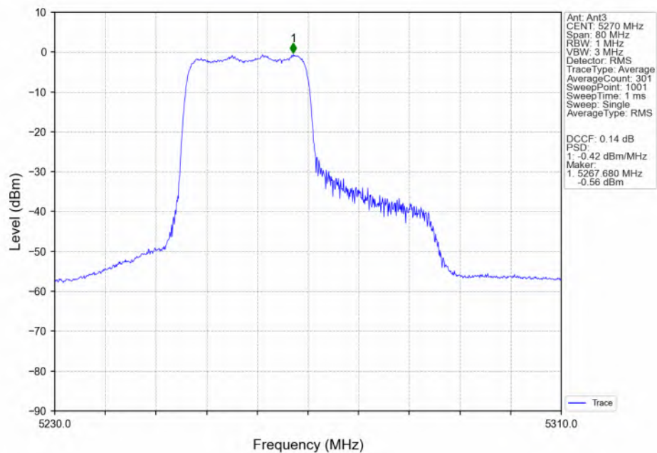
802.11be(EHT40) LCH_5270MHz_RU242_Left(61)_Ant3_NTNV
