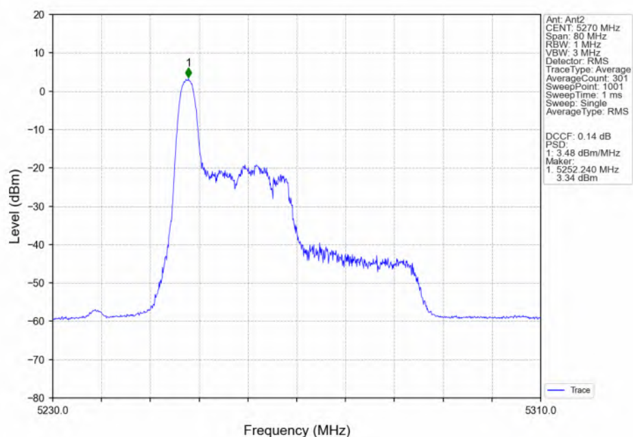
802.11be(EHT40) LCH_5270MHz_RU26_Left(0)_Ant2_NTNV
