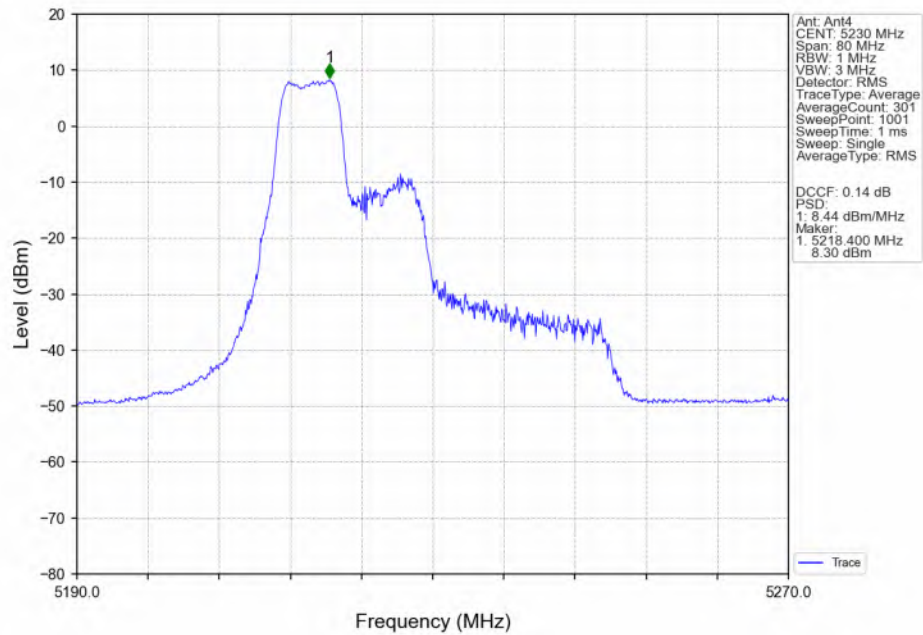
802.11be(EHT40)_HCH_5230MHz_26+52_ / MIMO_NTNV
