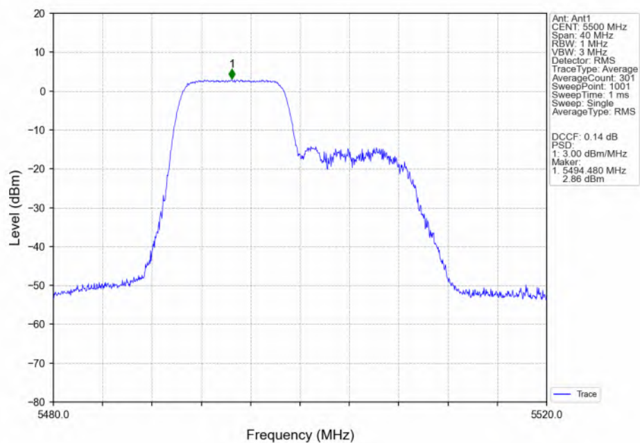
802.11be(EHT20) LCH_5500MHz_RU106 Left(53) Ant1_NTNV
