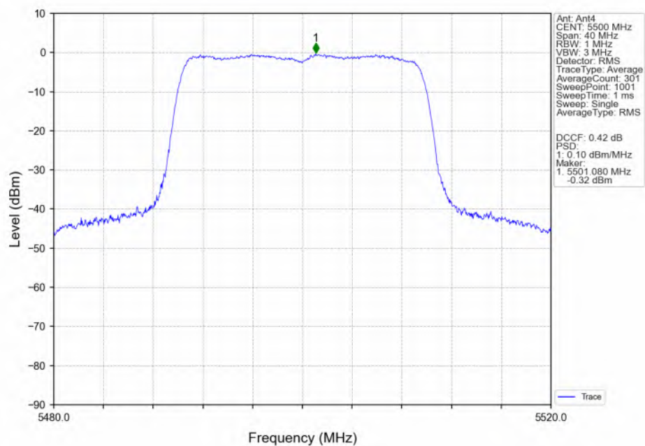
802.11be(EHT20) LCH_5500MHz_RU242_Left(61)_Ant4_NTNV
