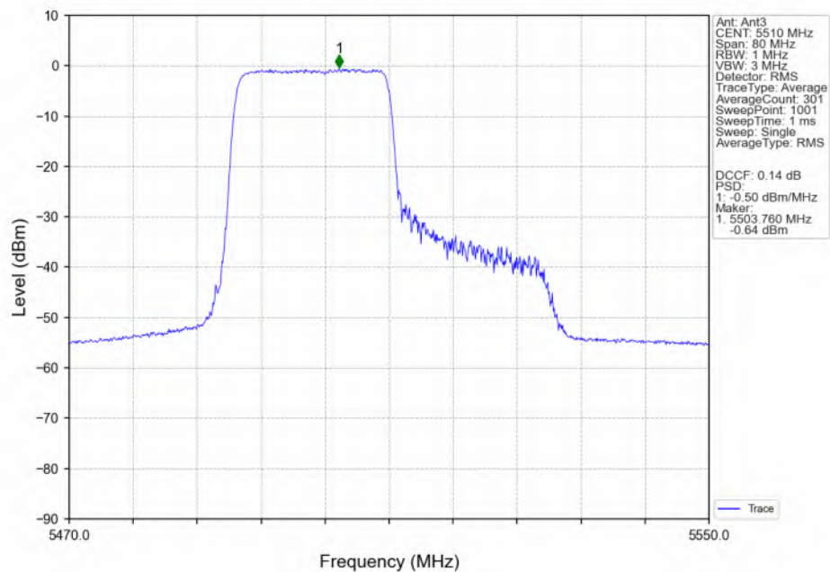
802.11be(EHT40) LCH_5510MHz_RU242_Left(61)_Ant3_NTNV
