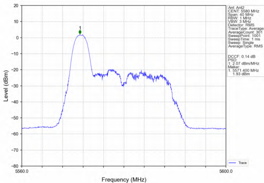
802.11be(EHT20)_MCH_5580MHz_RU26_Left(0)_Ant2_NTNV
