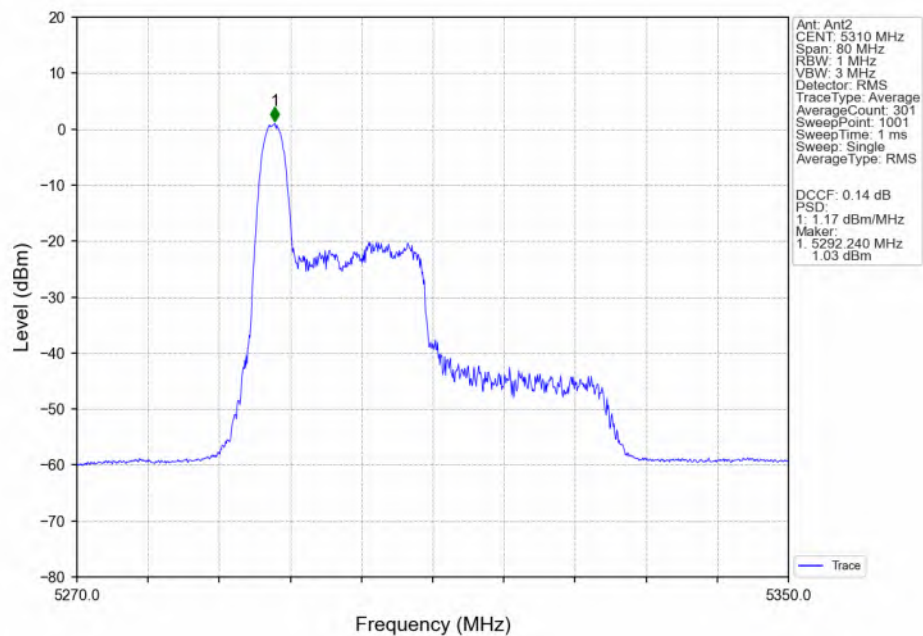
802.11be(EHT40)_HCH_5310MHz_RU26_Left(0)_Ant2_NTNV
