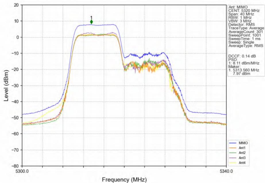
802.11be(EHT20)_HCH_5320MHz_RU106_Left(53)_MIMO_NTNV
