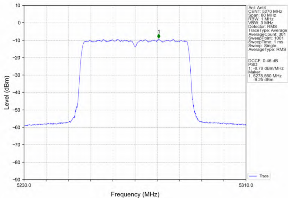
802.11be(EHT40) LCH_5270MHz_RU484_Left(65)_Ant4_NTNV
