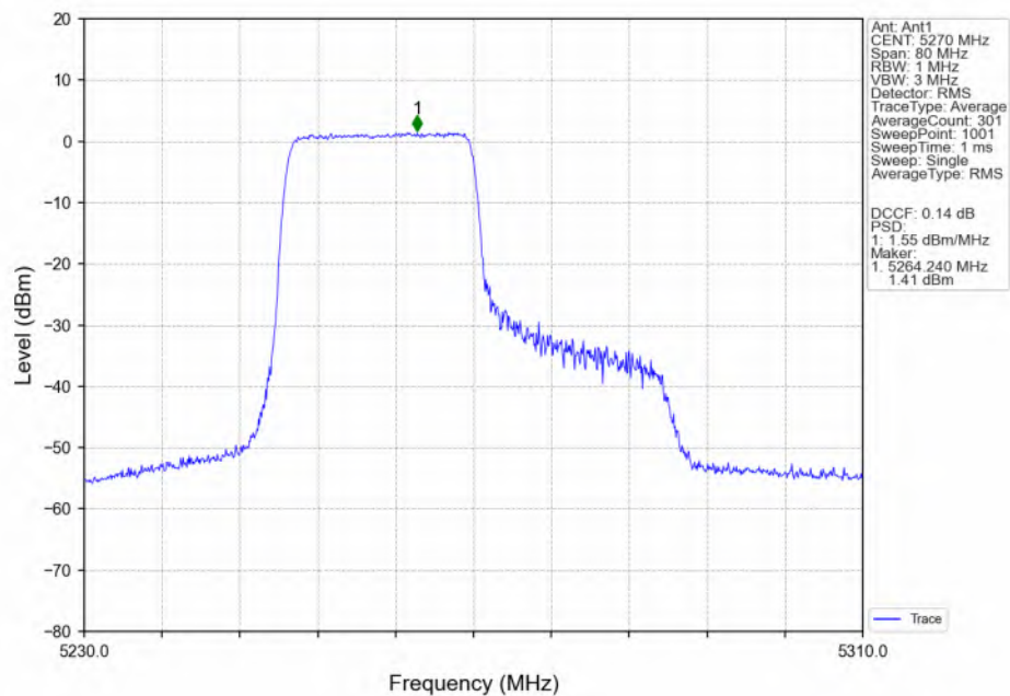
802.11be(EHT40) LCH_5270MHz_RU242_Left(61)_Ant1_NTNV
