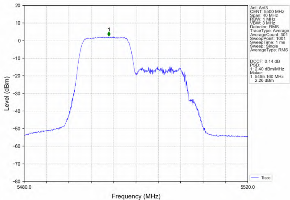
802.11be(EHT20) LCH_5500MHz_RU106_Left(53)_Ant3_NTNV
