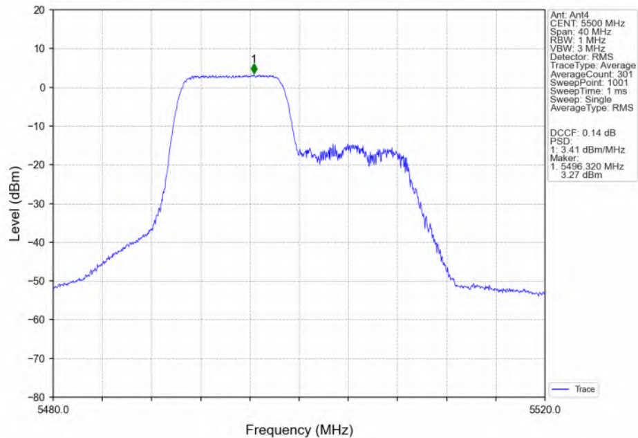
802.11be(EHT20)_LCH_5500MHz_RU106_Left(53)_MIMO_NTNV
