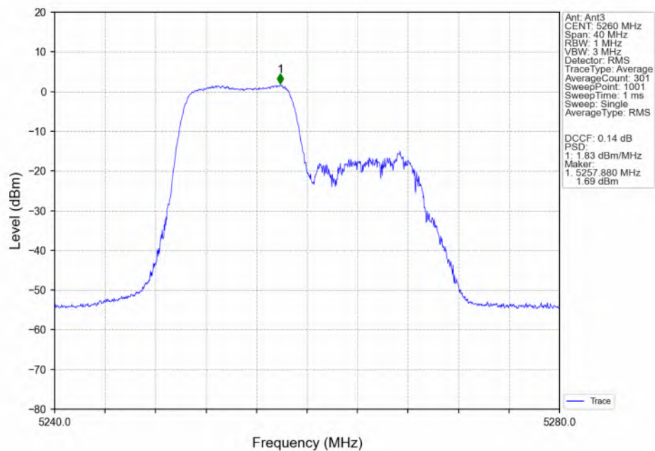
802.11be(EHT20) LCH_5260MHz_RU106_Left(53)_Ant3_NTNV
