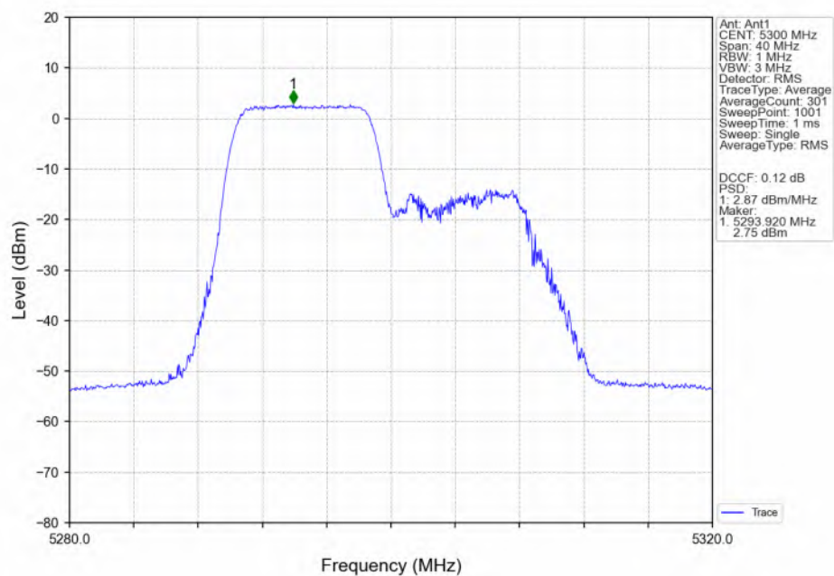
802.11be(EHT20)_MCH_5300MHz_RU106_Left(53)_Ant1_NTNV
