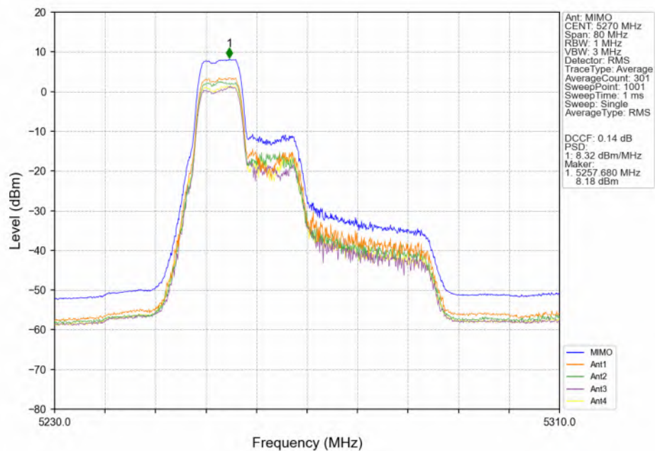
802.11be(EHT40) LCH_5270MHz_26+52 / MIMO_NTNV
