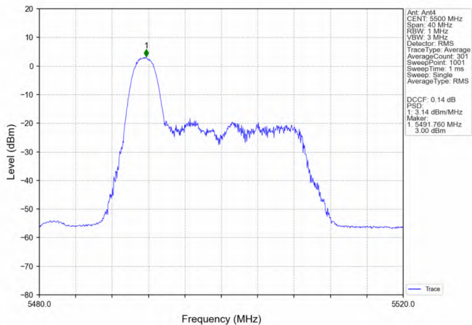
802.11be(EHT20) LCH_5500MHz_RU26_Left(0)_Ant4_NTNV
