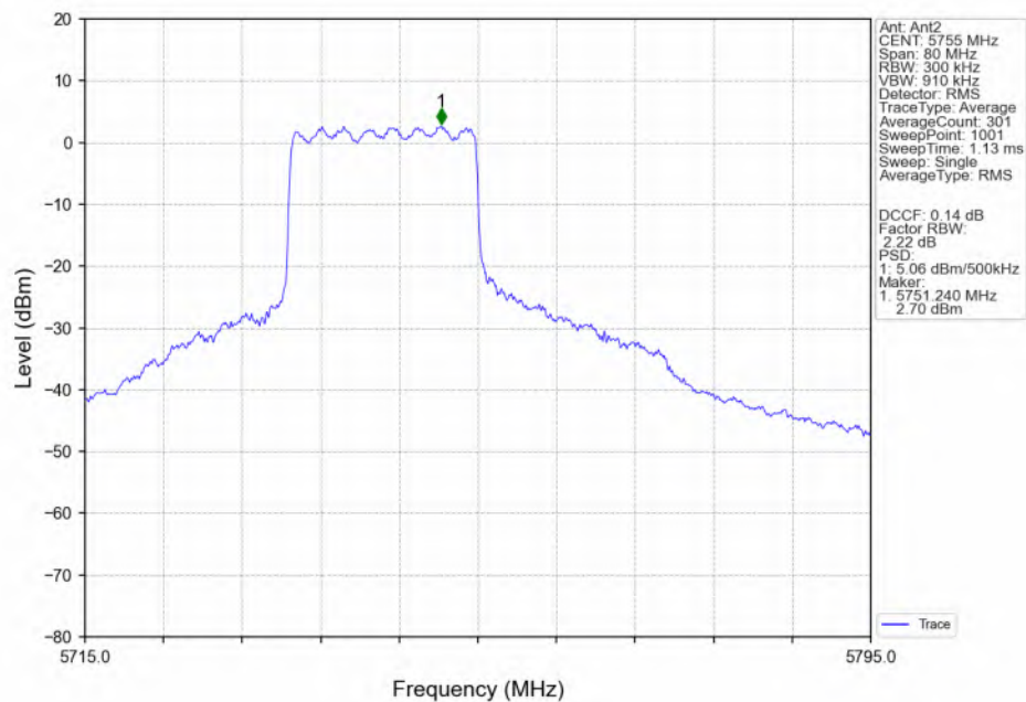
802.11be(EHT40) LCH_5755MHz_RU242_Left(61)_Ant2_NTNV
