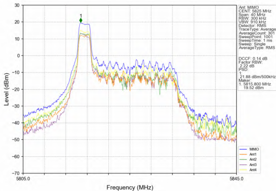
802.11be(EHT20)_HCH_5825MHz_RU26_Left(0)_MIMO_NTNV
