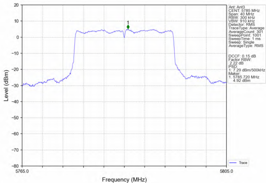
802.11be(EHT20)_MCH_5785MHz_RU242_Left(61)_Ant3_NTNV
