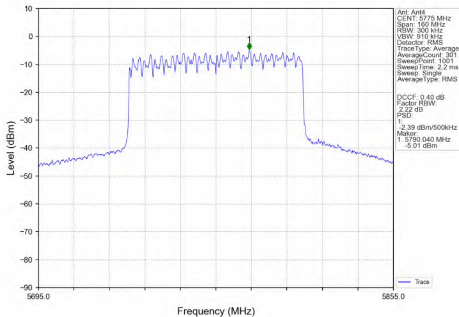
802.11ax(HEW80) MCH_5775MHz_RU996_Left(67)_Ant4_NTNV
