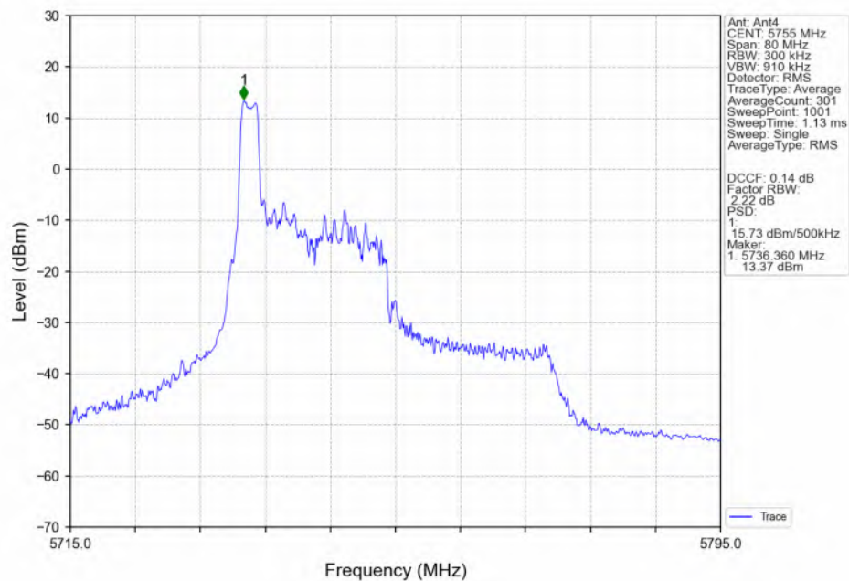
802.11ax(HEW40)_LCH_5755MHz_RU26_Left(0)_Ant4_NTNV
