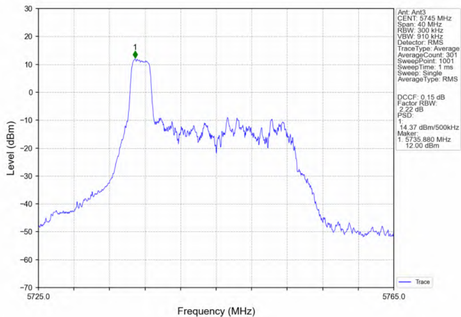
802.11be(EHT20) LCH_5745MHz_RU26_Left(0)_Ant3_NTNV
