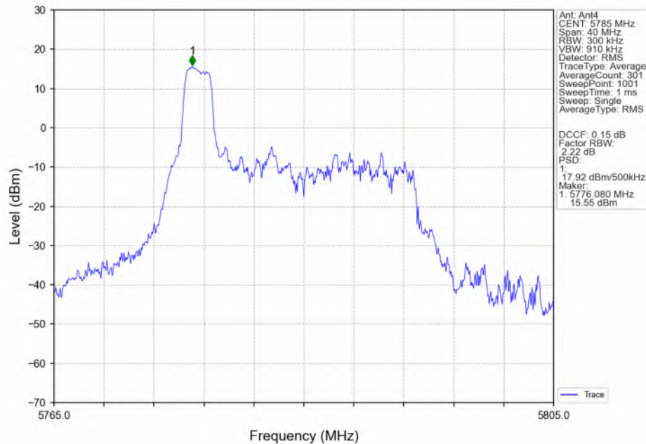
802.11be(EHT20)_MCH_5785MHz_RU26_Left(0)_MIMO_NTNV
