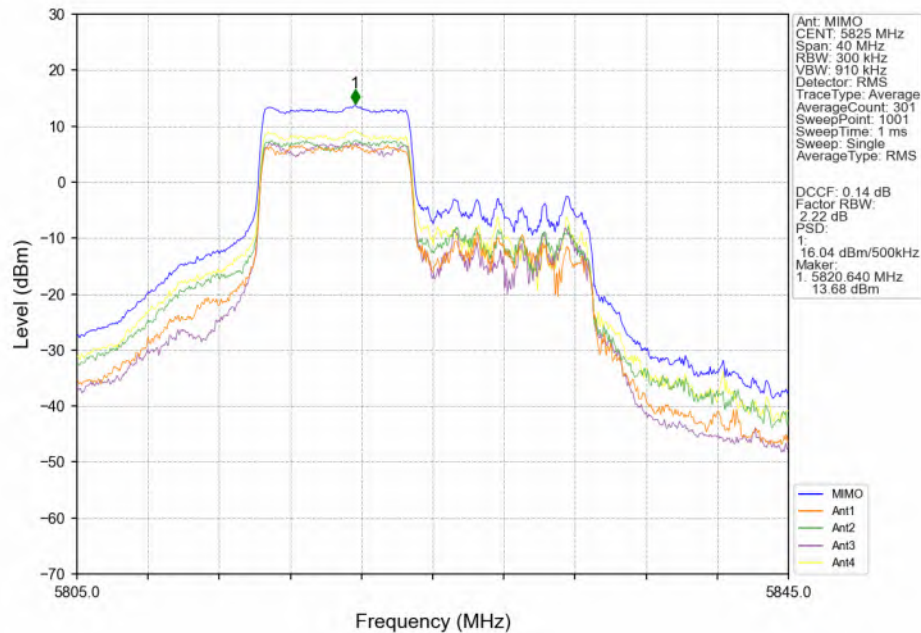
802.11be(EHT20)_HCH_5825MHz_RU242_Left(61)_Ant1_NTNV
