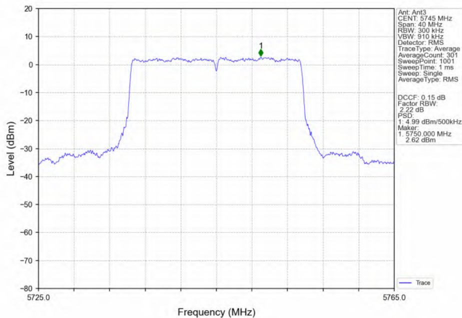
802.11be(EHT20) LCH_5745MHz_RU242_Left(61)_Ant3_NTNV
