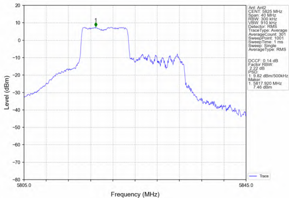
802.11be(EHT20)_HCH_5825MHz_RU106_Left(53)_Ant2_NTNV
