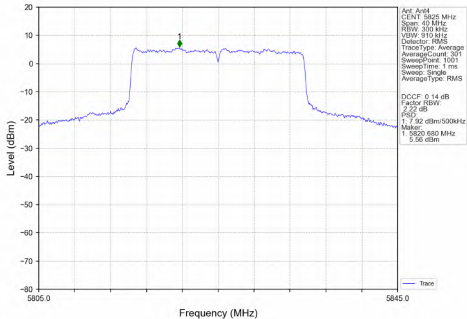
802.11be(EHT20)_HCH_5825MHz_RU242_Left(61)_MIMO_NTNV
