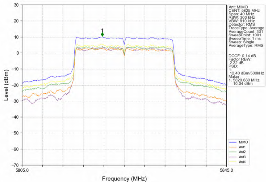
802.11be(EHT20)_HCH_5825MHz_RU242_Left(61)_MIMO_NTNV
