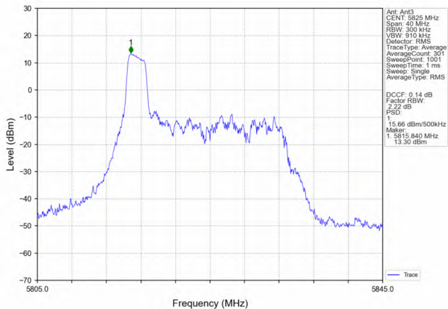
802.11be(EHT20)_HCH_5825MHz_RU26_Left(0)_Ant3_NTNV
