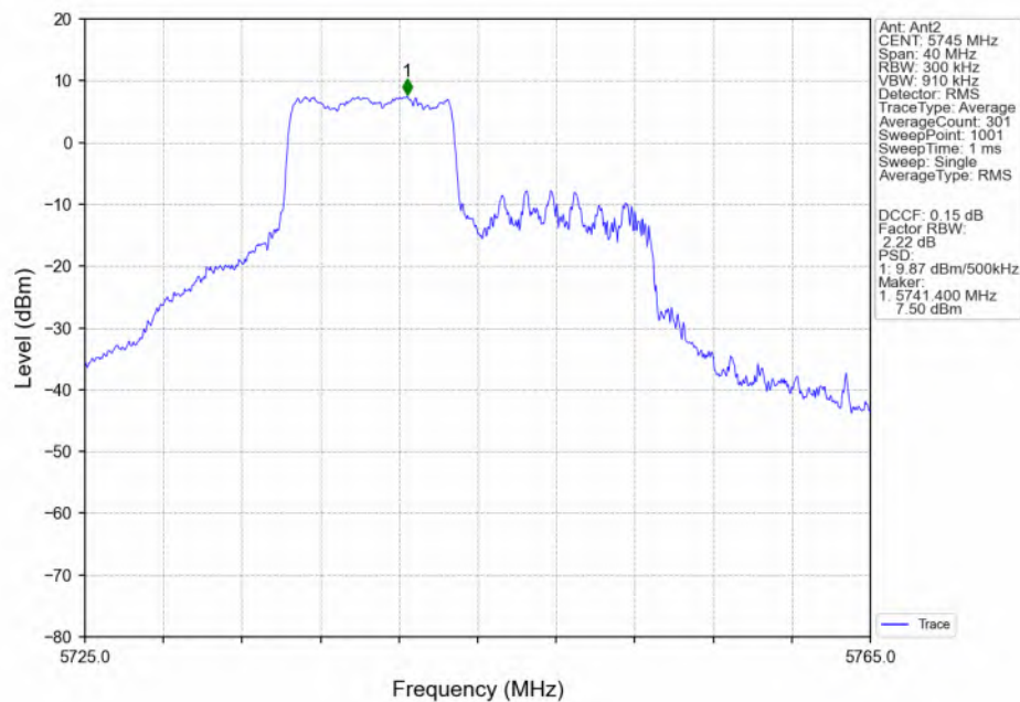
802.11be(EHT20) LCH_5745MHz_RU106_Left(53)_Ant2_NTNV
