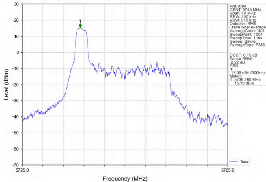
802.11be(EHT20) LCH 5745MHz RU26 Left(0) MIMO NTN
