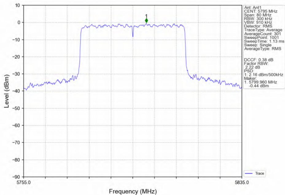
802.11ax(HEW40)_HCH_5795MHz_RU484_Left(65)_Ant1_NTNV
