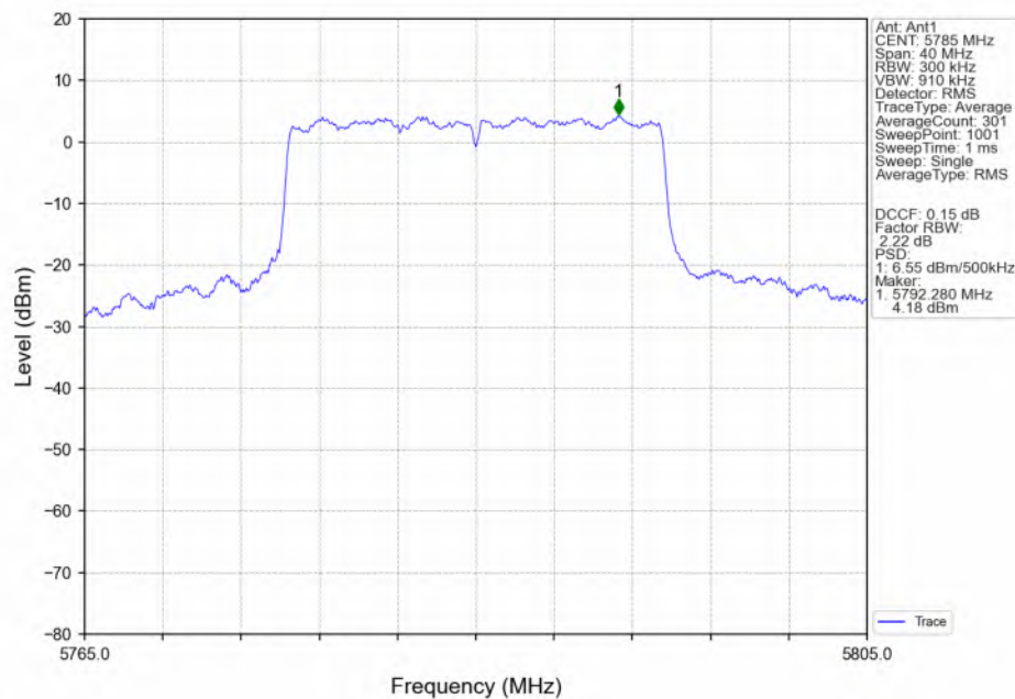
802.11be(EHT20)_MCH_5785MHz_RU242_Left(61)_Ant1_NTNV
