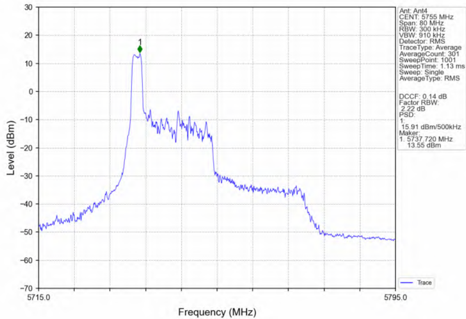
802.11be(EHT40) LCH 5755MHz RU26 Left(0) MIMO NTN
