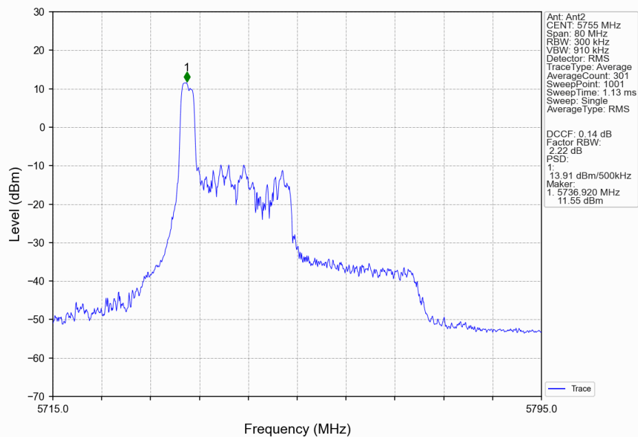
802.11ax(HEW40)_LCH_5755MHz_RU26_Left(0)_Ant2_NTNV
