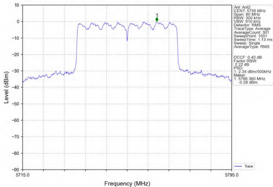
802.11ax(HEW40)_LCH_5755MHz_RU484_Left(65)_Ant2_NTNV
