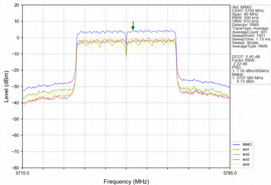
802.11be(EHT40) LCH 5755MHz RU484 Left(65) MIMO NTN
