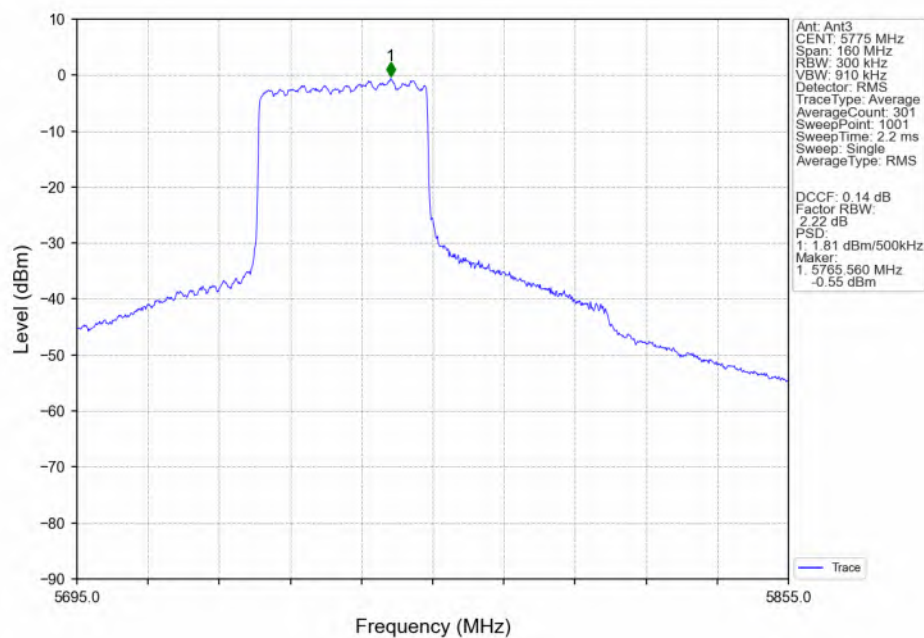
802.11ax(HEW80) MCH_5775MHz_RU484_Left(65)_Ant3_NTNV
