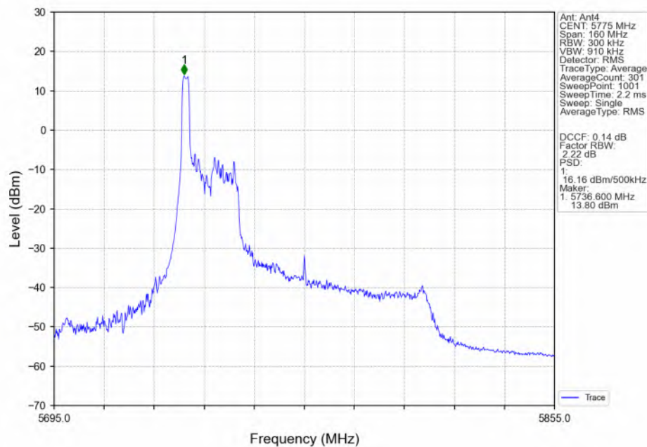
802.11ax(HEW80) MCH_5775MHz_RU26_Left(0)_Ant4_NTNV
