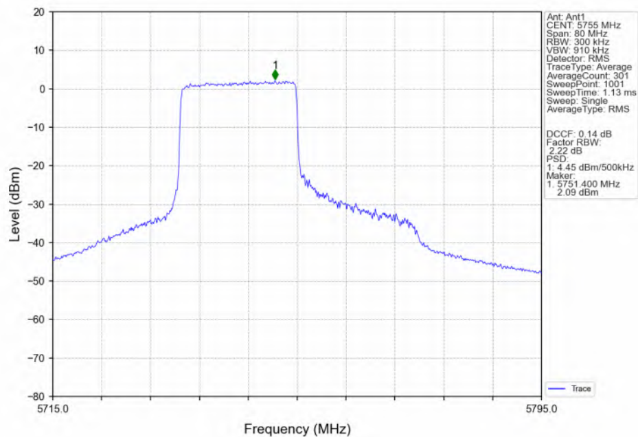
802.11ax(HEW40)_LCH_5755MHz_RU242_Left(61)_Ant1_NTNV
