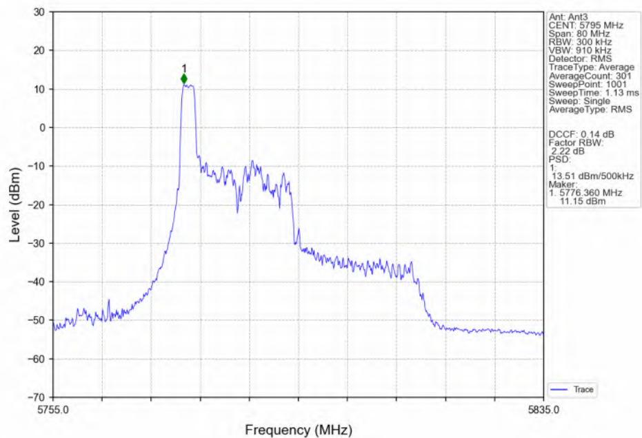
802.11be(EHT40)_HCH_5795MHz_RU26_Left(0)_Ant3_NTNV
