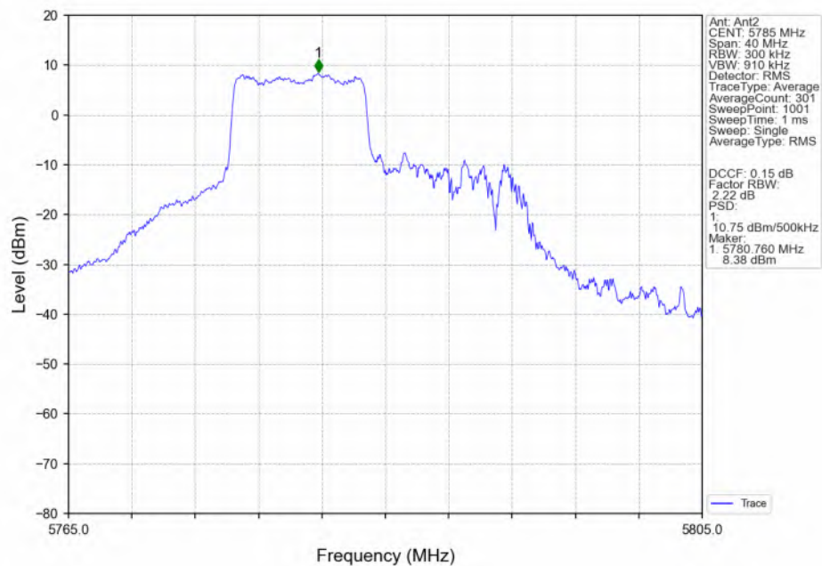
802.11be(EHT20)_MCH_5785MHz_RU106_Left(53)_Ant2_NTNV
