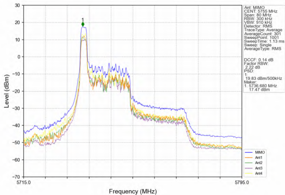
802.11be(EHT40) LCH 5755MHz RU26 Left(0) MIMO NTN
