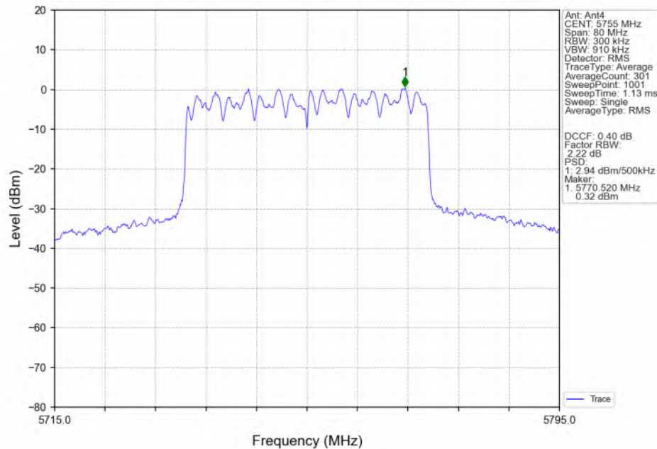
802.11be(EHT40) LCH 5755MHz RU484 Left(65) MIMO NTN
