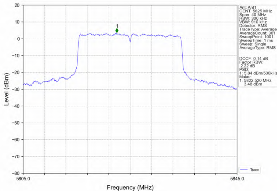
802.11be(EHT20)_HCH_5825MHz_RU242_Left(61)_Ant1_NTNV
