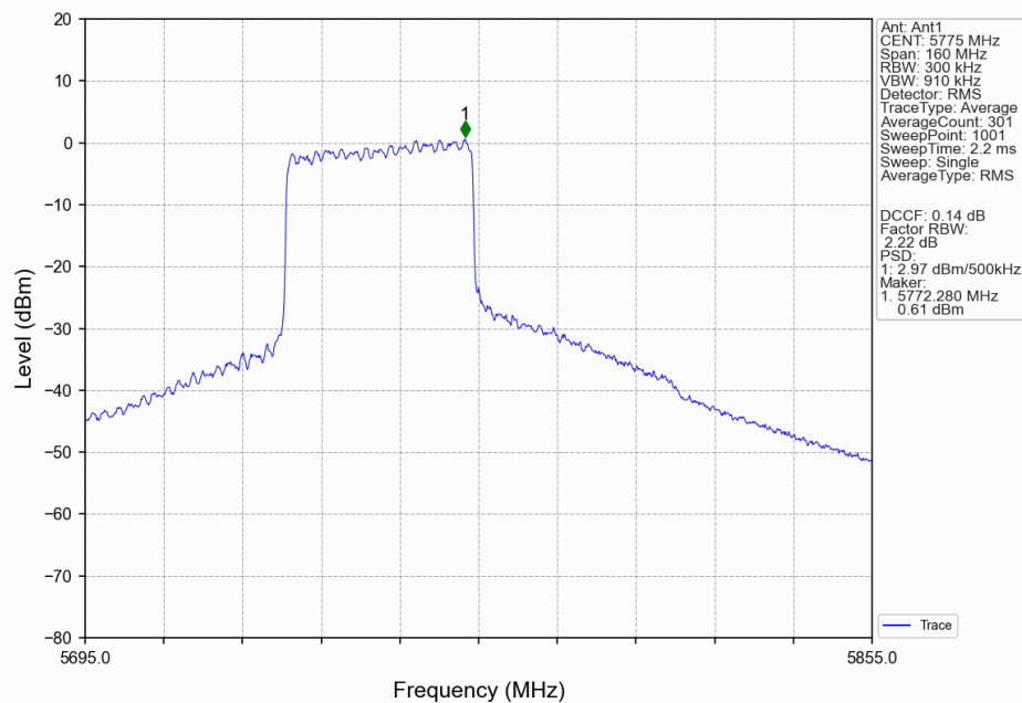
802.11ax(HEW80)_MCH_5775MHz_RU484_Left(65)_Ant1_NTNV
