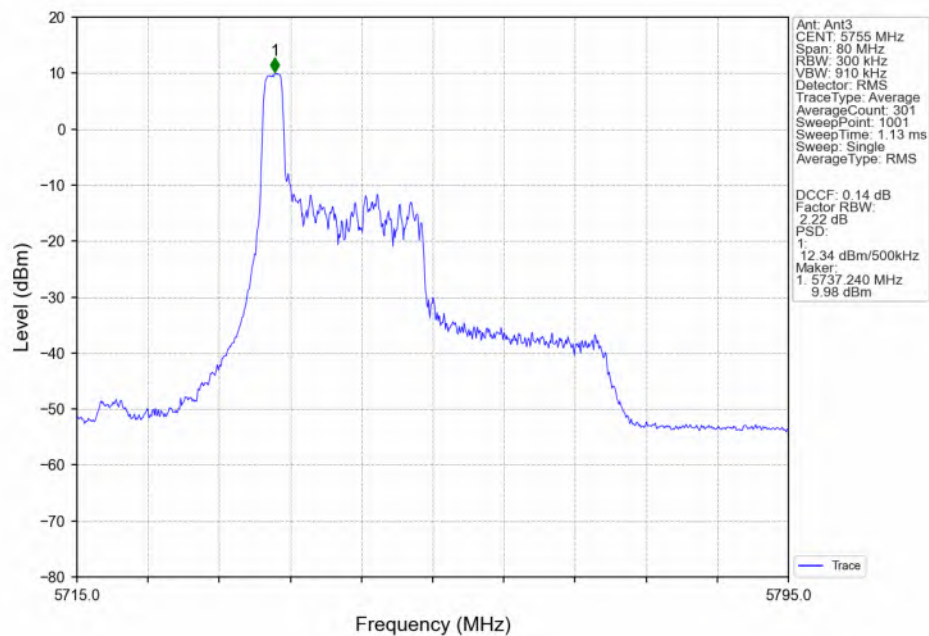
802.11be(EHT40) LCH_5755MHz_RU26_Left(0)_Ant3_NTNV
