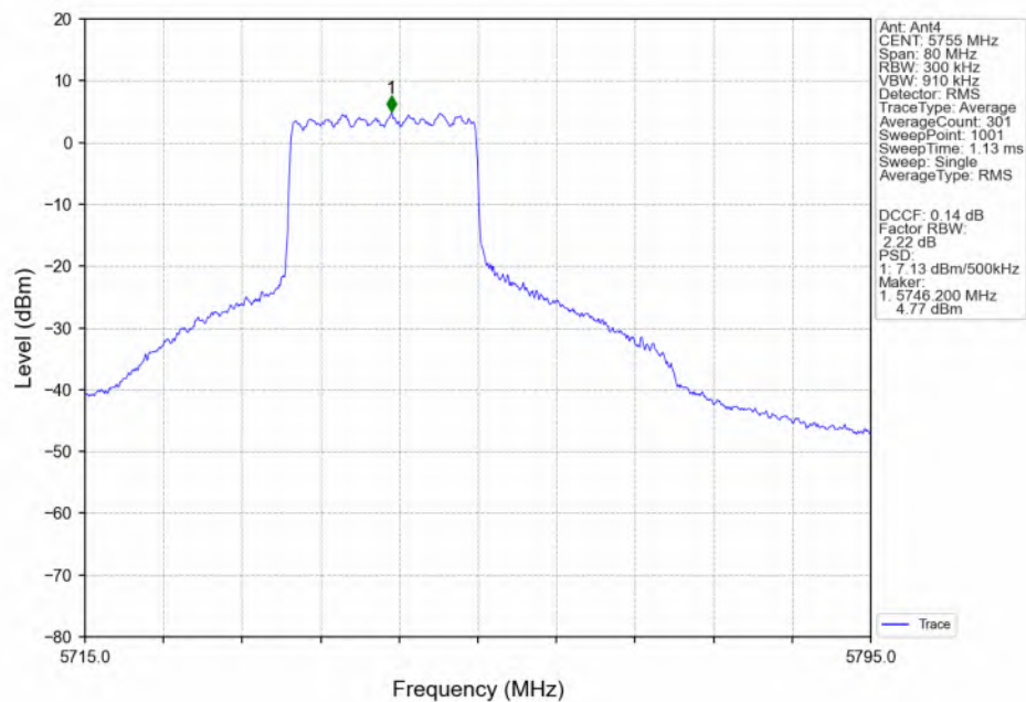
802.11be(EHT40) LCH_5755MHz_RU242_Left(61)_Ant4_NTNV
