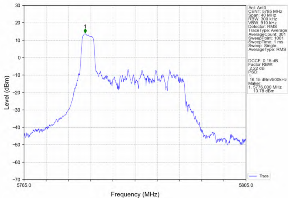
802.11be(EHT20)_MCH_5785MHz_RU26_Left(0)_Ant3_NTNV
