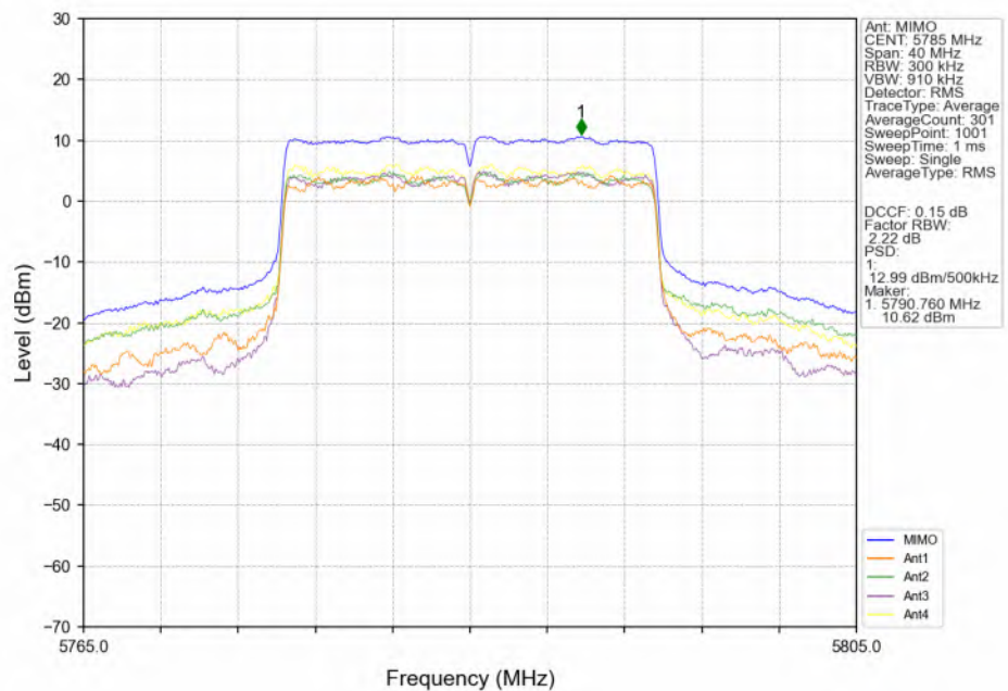
802.11be(EHT20)_MCH_5785MHz_RU242_Left(61)_MIMO_NTNV
