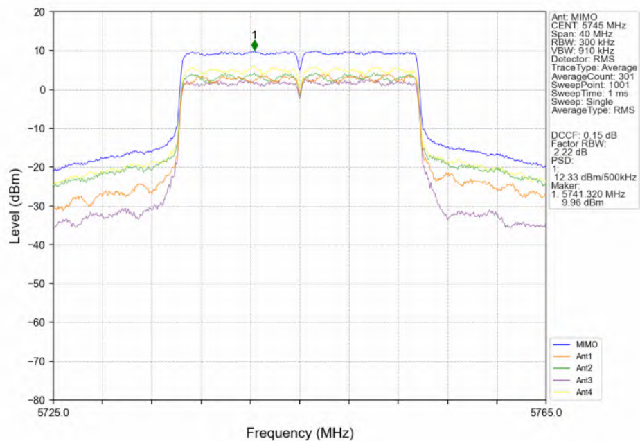
802.11be(EHT20)_LCH_5745MHz_RU242_Left(61)_MIMO_NTNV
