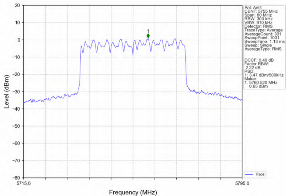
802.11ax(HEW40)_LCH_5755MHz_RU484_Left(65)_Ant4_NTNV
