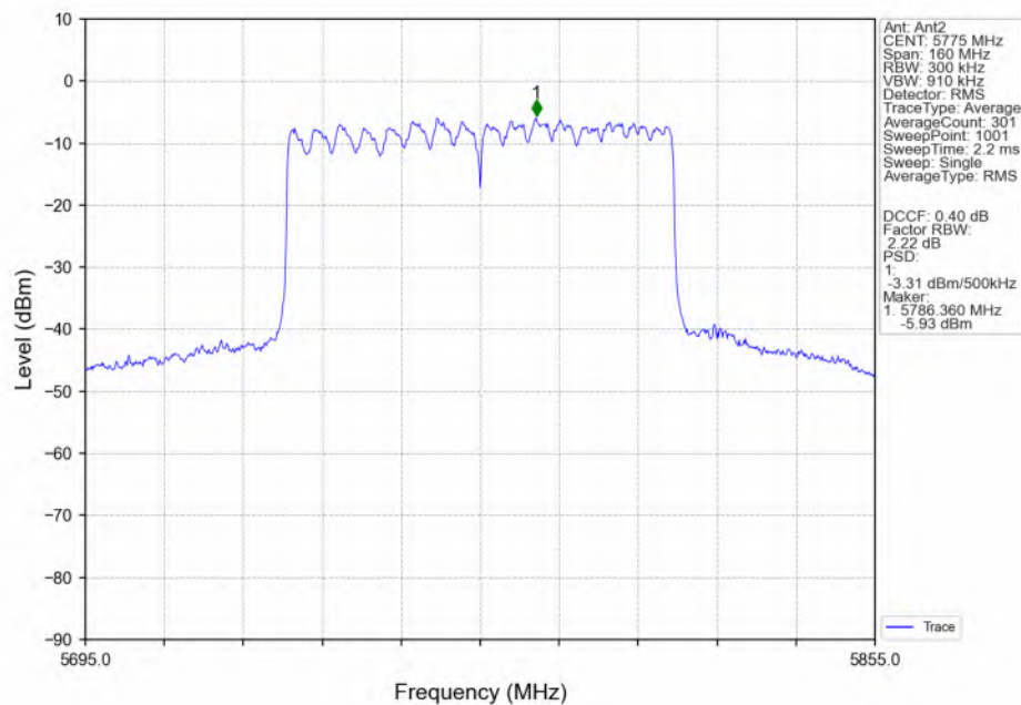
802.11ax(HEW80) MCH_5775MHz_RU996_Left(67)_Ant2_NTNV
