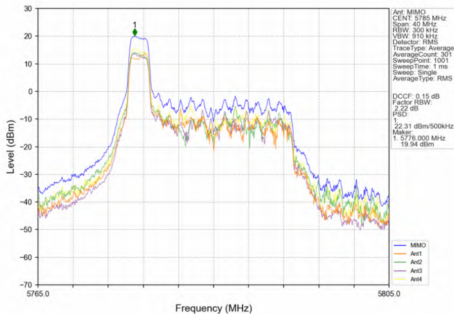
802.11be(EHT20)_MCH_5785MHz_RU26_Left(0)_MIMO_NTNV
