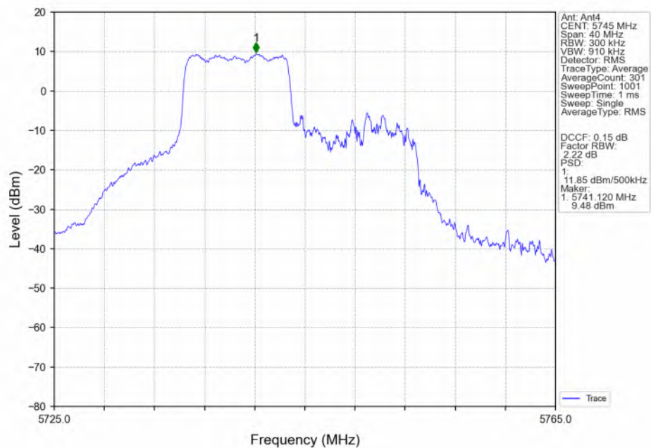
802.11be(EHT20) LCH_5745MHz_RU106_Left(53)_Ant4_NTNV
