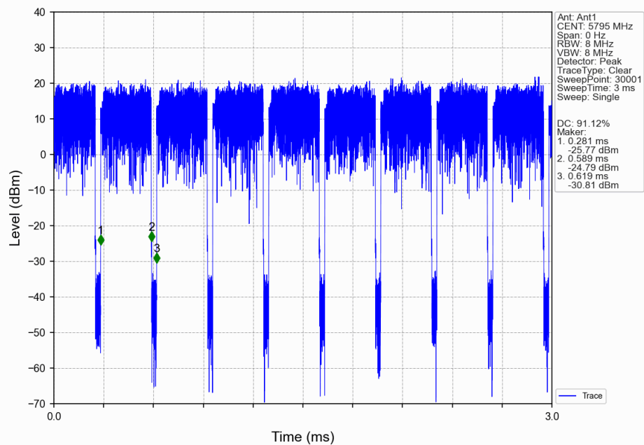
802.11be(EHT40) HCH 5795MHz RU484 Left(65) Ant1 NTN
