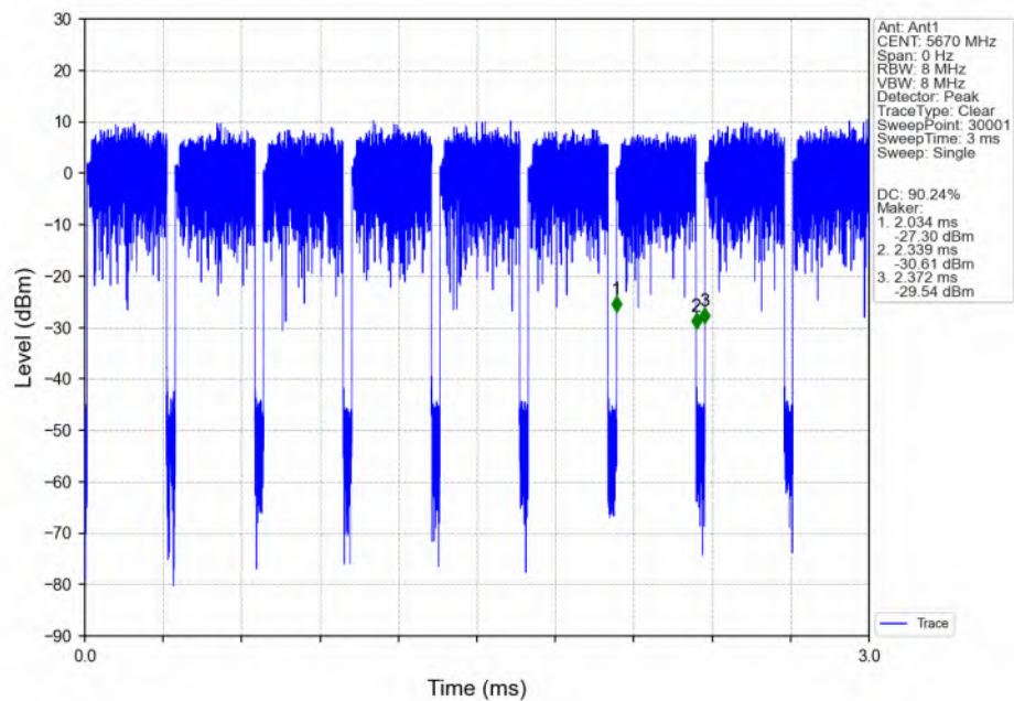
802.11be(EHT40)_HCH_5670MHz_RU484_Left(65)_Ant1_NTNV
