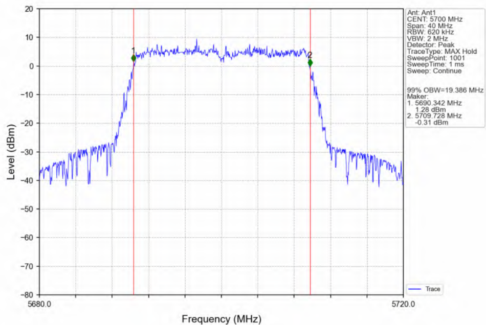
802.11be(EHT20)_HCH_5700MHz_RU242_Left(61)_Ant1_NTNV
