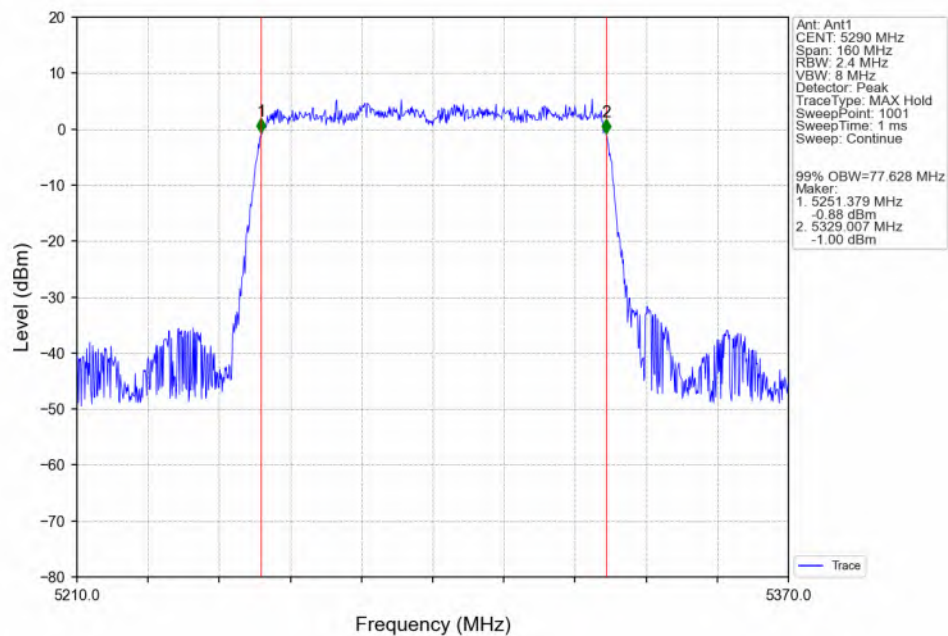
802.11ax(HEW80) MCH_5290MHz_RU996_Left(67)_Ant1_NTNV
