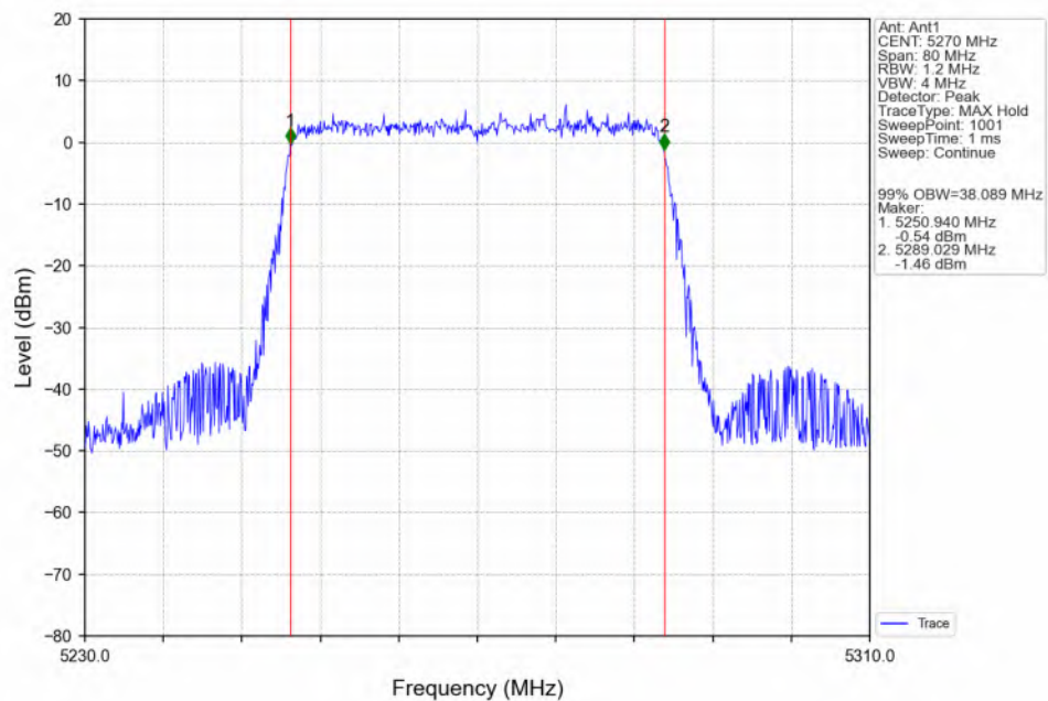
802.11be(EHT40)_LCH_5270MHz_RU484_Left(65)_Ant1_NTNV
