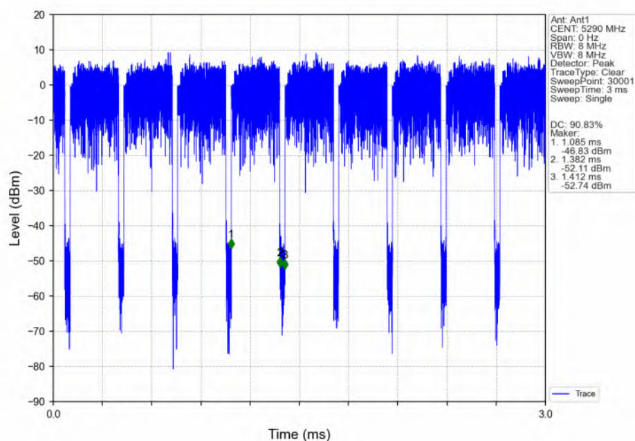
802.11be(EHT80)_MCH_5290MHz_RU996_Left(67)_Ant1_NTNV
