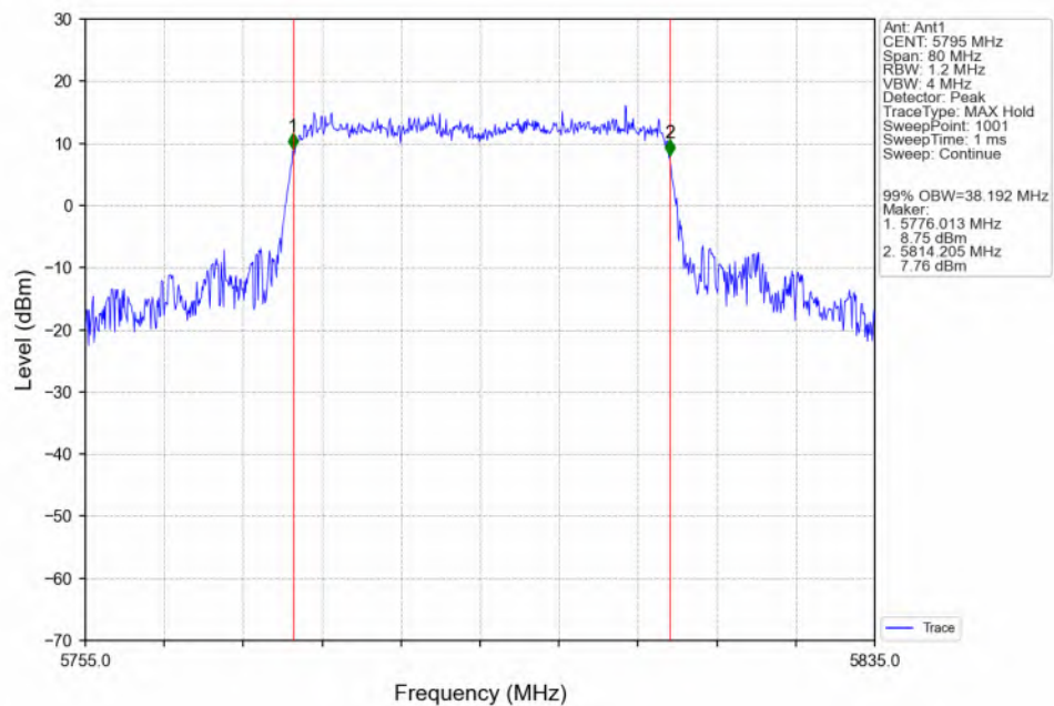
802.11ax(HEW40)_HCH_5795MHz_RU484_Left(65)_Ant1_NTNV
