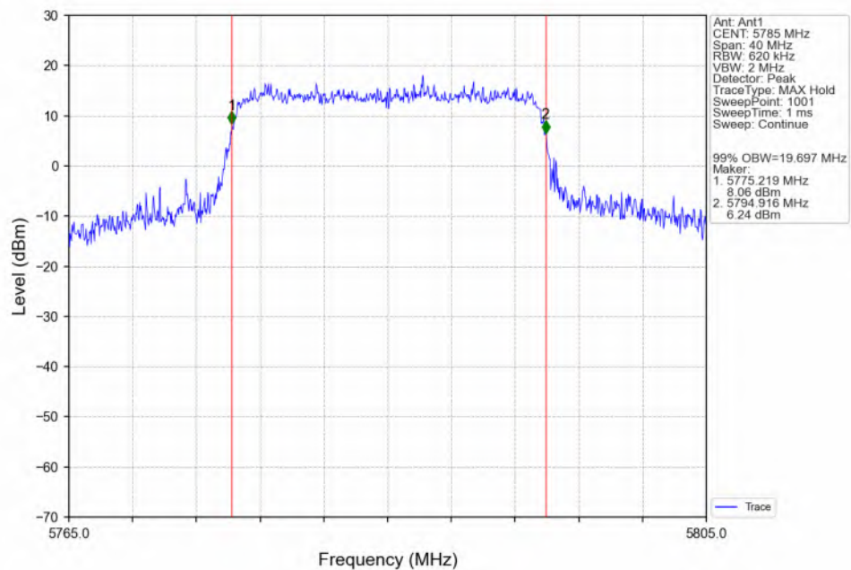
802.11be(EHT20) MCH_5785MHz_RU242_Left(61)_Ant1_NTNV
