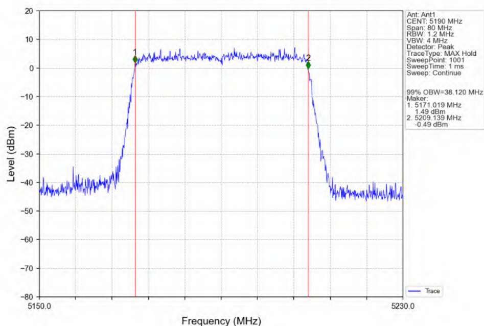
802.11ax(HEW40) LCH_5190MHz_RU484_Left(65)_Ant1_NTNV
