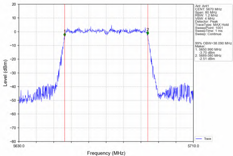
802.11be(EHT40)_HCH_5670MHz_RU484_Left(65)_Ant1_NTNV
