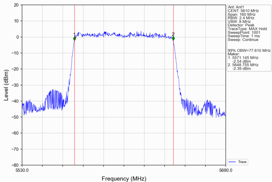
802.11ax(HEW80)_HCH_5610MHz_RU996_Left(67)_Ant1_NTNV
