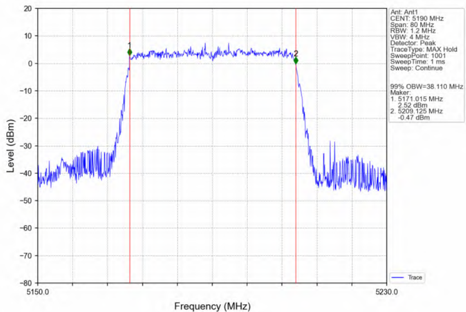
802.11be(EHT40)_LCH_5190MHz_RU484_Left(65)_Ant1_NTNV
