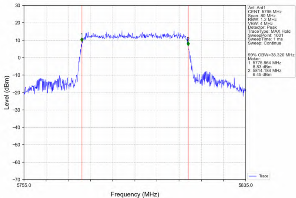
802.11be(EHT40) HCH_5795MHz_RU484_Left(65)_Ant1_NTNV
