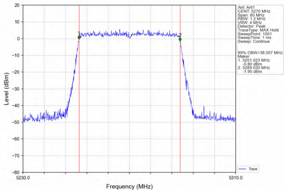
802.11ax(HEW40) LCH_5270MHz_RU484_Left(65)_Ant1_NTNV
