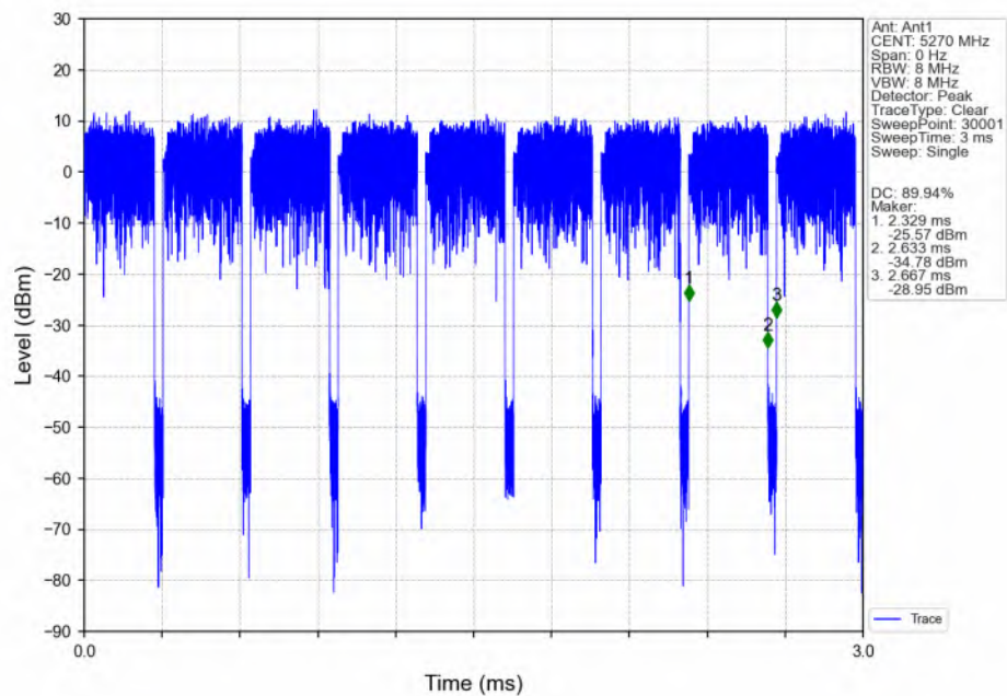
802.11be(EHT40)_LCH_5270MHz_RU484_Left(65)_Ant1_NTNV
