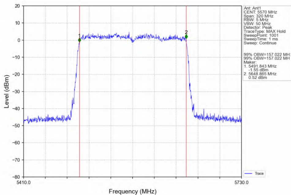
802.11ax(HEW160) MCH_5570MHz_2xRU996_Left(68)_Ant1_NTNV
