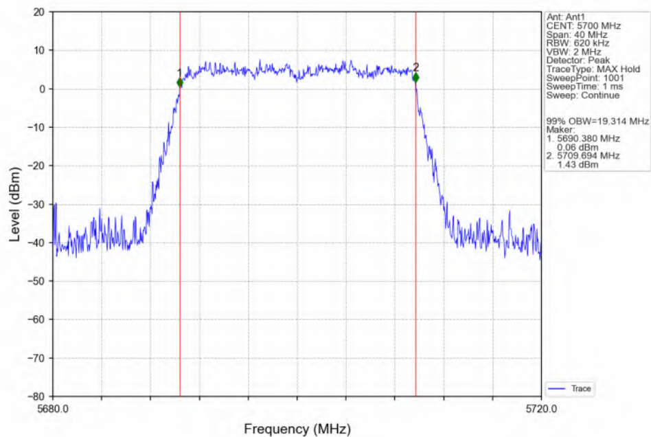
802.11ax(HEW20) HCH_5700MHz_RU242_Left(61)_Ant1_NTNV
