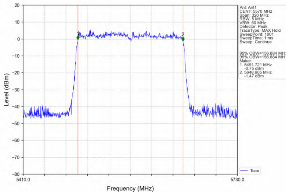
802.11be(EHT160)_MCH_5570MHz_2xRU996_Left(68)_Ant1_NTNV
