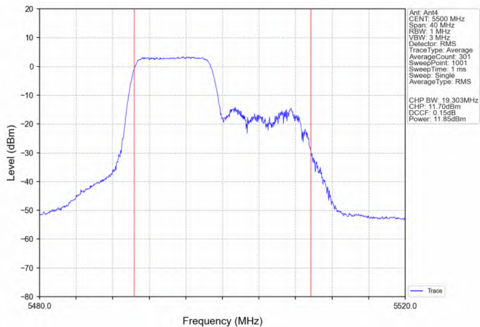
802.11ax(HEW20)_LCH_5500MHz_RU106_Left(53)_Ant4_NTNV
