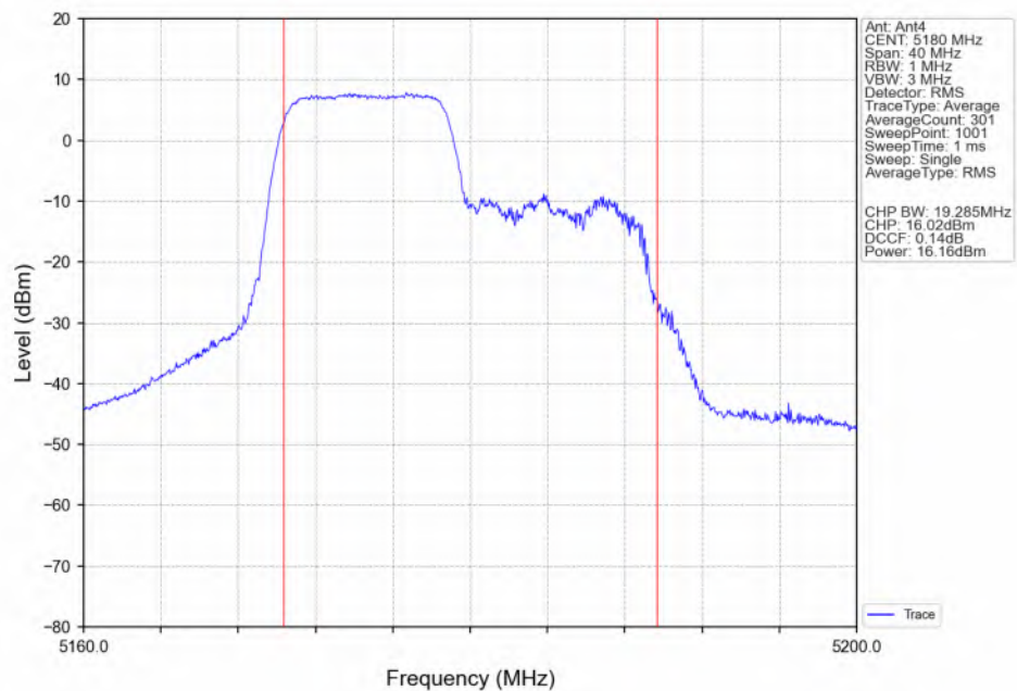
802.11ax(HEW20)_LCH_5180MHz_RU106_Left(53)_Ant4_NTNV
