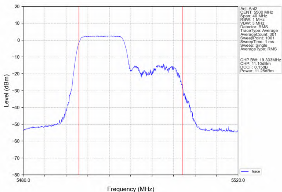
802.11ax(HEW20)_LCH_5500MHz_RU106_Left(53)_Ant2_NTNV
