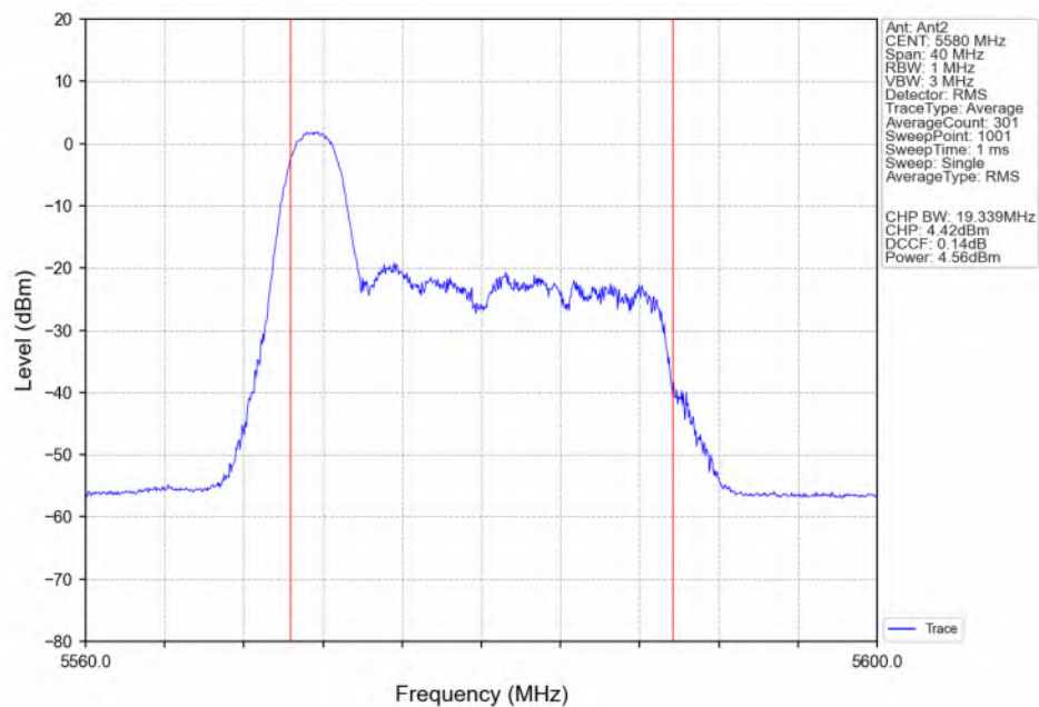
802.11ax(HEW20)_MCH_5580MHz_RU26_Left(0)_Ant2_NTNV
