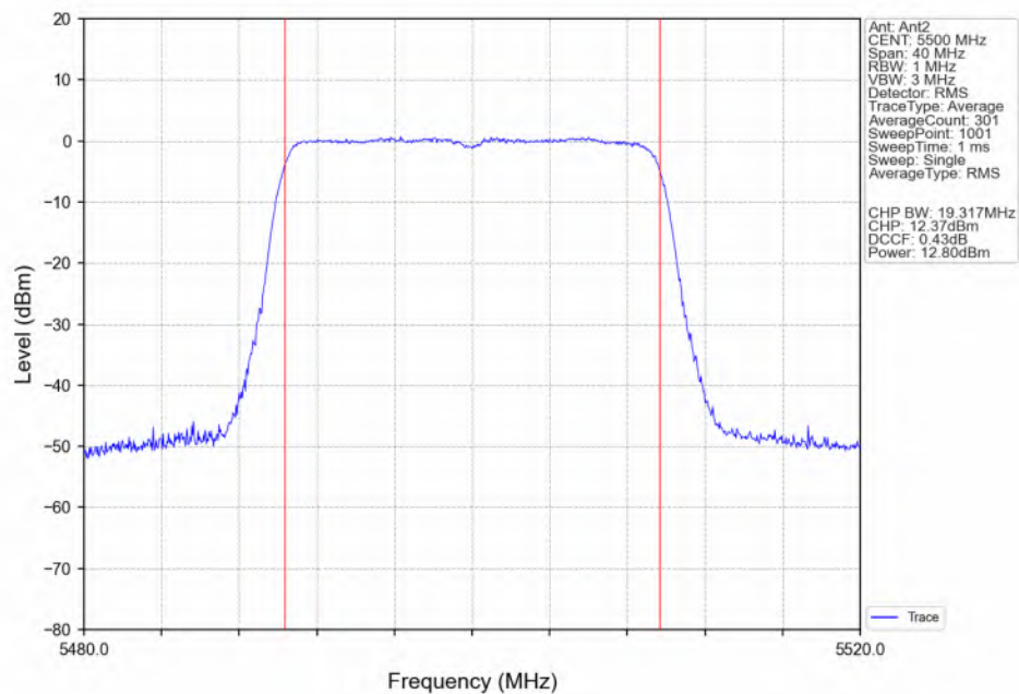
802.11ax(HEW20)_LCH_5500MHz_RU242_Left(61)_Ant2_NTNV
