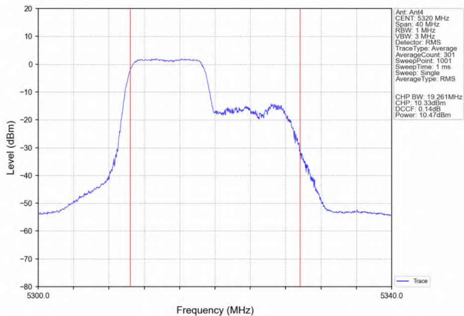
802.11ax(HEW20)_HCH_5320MHz_RU106_Left(53)_Ant4_NTNV
