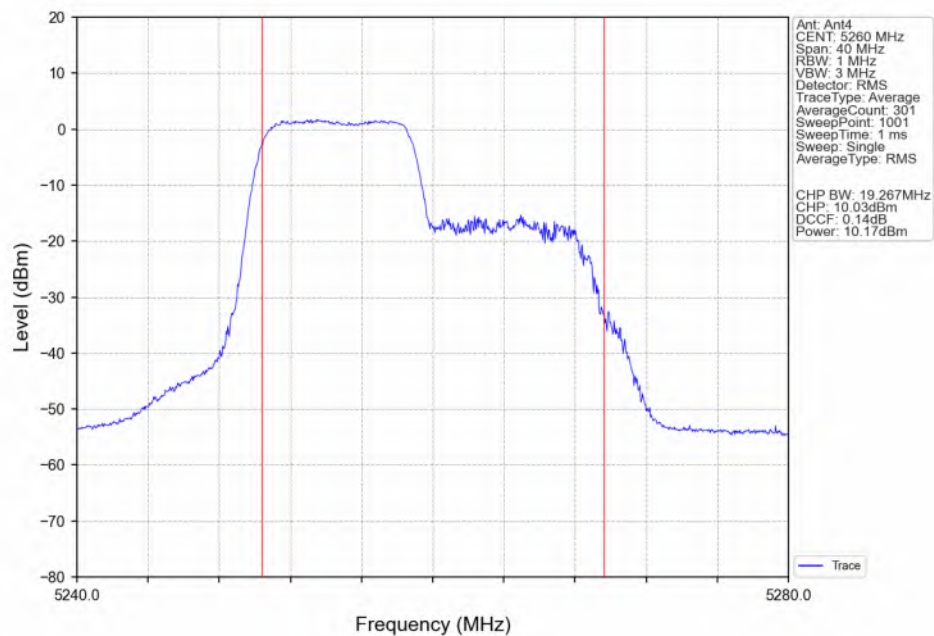
802.11ax(HEW20)_LCH_5260MHz_RU106_Left(53)_Ant4_NTNV
