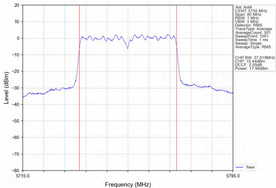
802.11n(HT40)_LCH_5755MHz_Ant4_NTNV
