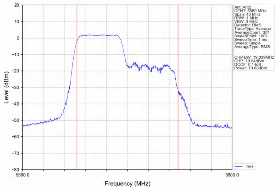
802.11ax(HEW20) MCH_5580MHz_RU106_Left(53)_Ant2_NTNV
