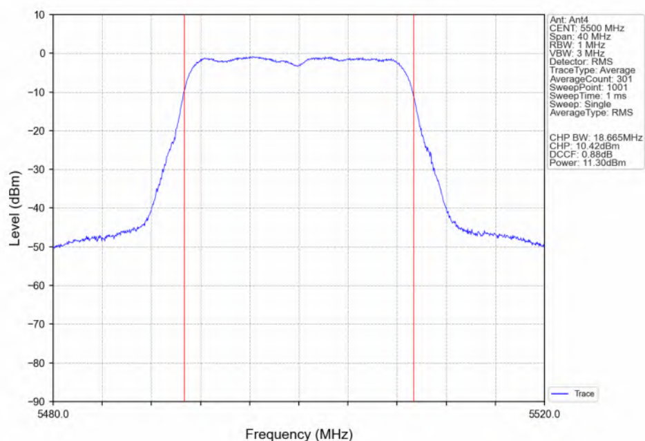
802.11ac(VHT20)_LCH_5500MHz_Ant4_NTNV
