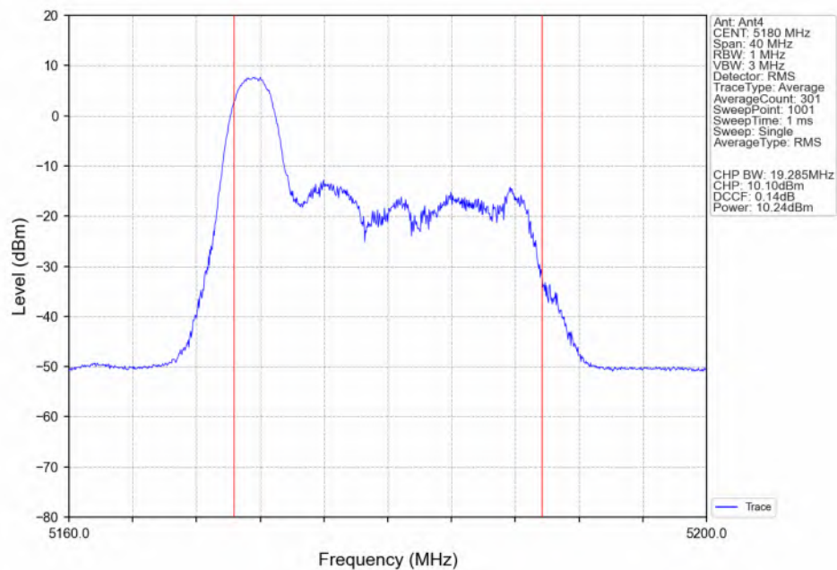
802.11ax(HEW20)_LCH_5180MHz_RU26_Left(0)_Ant4_NTNV
