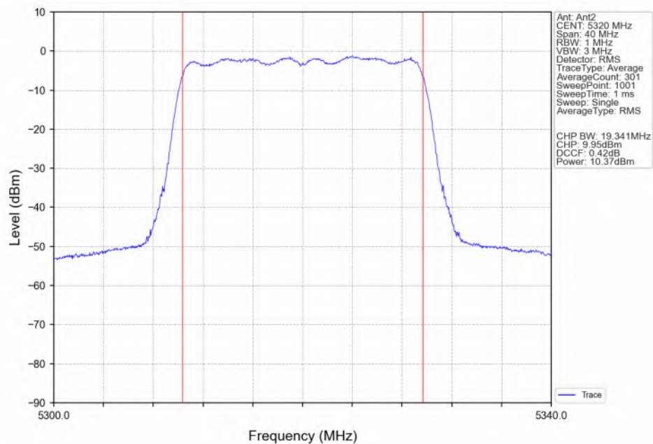
802.11ax(HEW20) HCH_5320MHz_RU242_Left(61)_Ant2_NTNV
