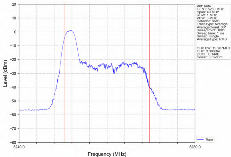
802.11ax(HEW20)_LCH_5260MHz_RU26_Left(0)_Ant4_NTNV
