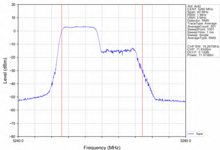
802.11ax(HEW20)_LCH_5260MHz_RU106_Left(53)_Ant2_NTNV
