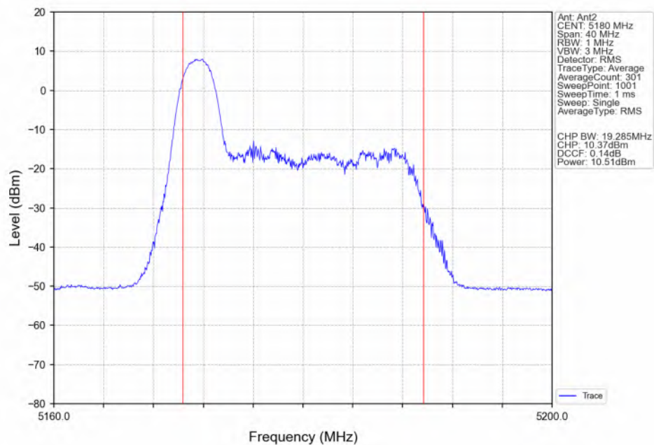
802.11ax(HEW20)_LCH_5180MHz_RU26_Left(0)_Ant2_NTNV
