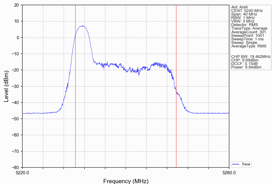
802.11ax(HEW20) HCH_5240MHz_RU26_Left(0)_Ant4_NTNV
