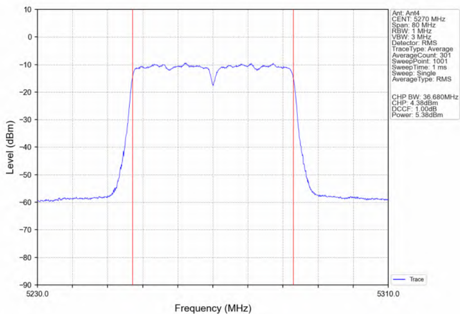
802.11ac(VHT40)_LCH_5270MHz_Ant4_NTNV
