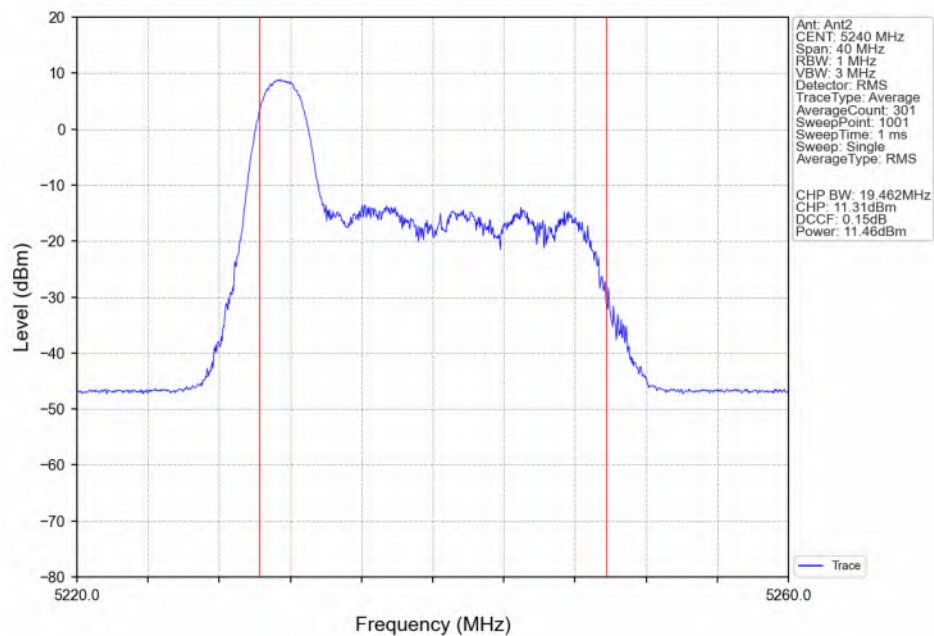
802.11ax(HEW20) HCH_5240MHz_RU26_Left(0)_Ant2_NTNV
