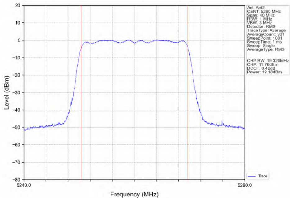
802.11ax(HEW20)_LCH_5260MHz_RU242_Left(61)_Ant2_NTNV
