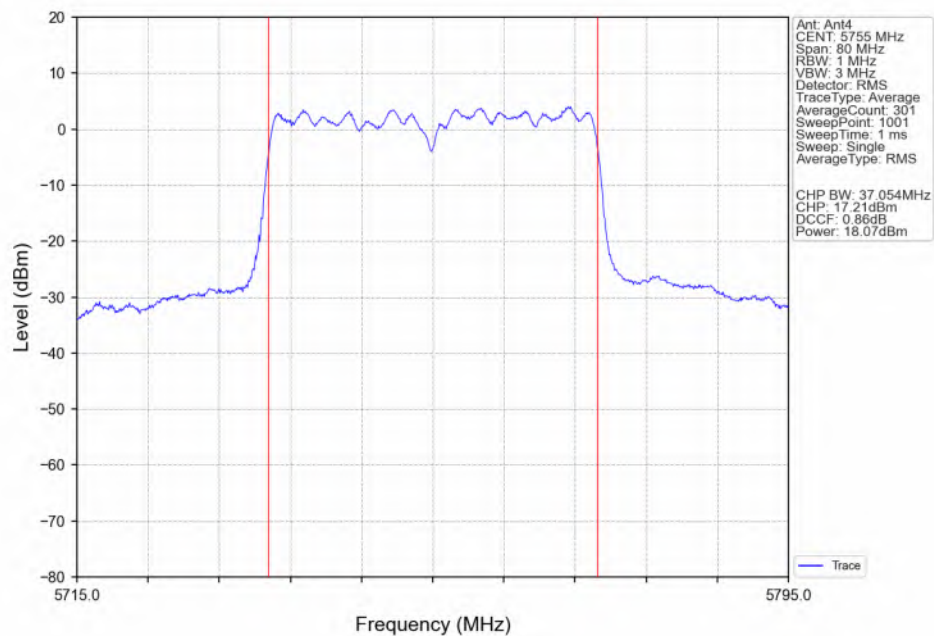
802.11ac(VHT40)_LCH_5755MHz_Ant4_NTNV
