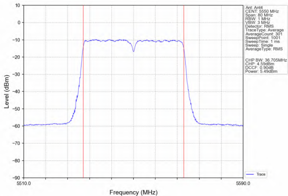
802.11ac(VHT40) MCH_5550MHz_Ant4_NTNV
