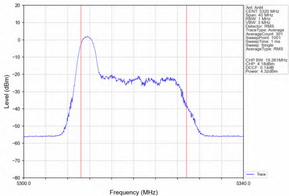
802.11ax(HEW20) HCH_5320MHz_RU26_Left(0)_Ant4_NTNV
