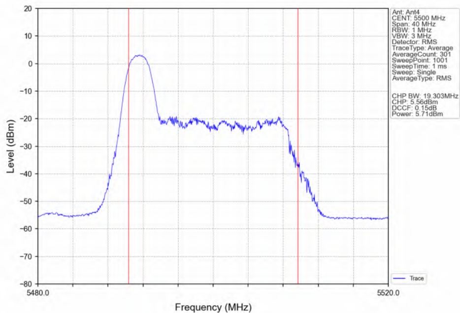
802.11ax(HEW20)_LCH_5500MHz_RU26_Left(0)_Ant4_NTNV
