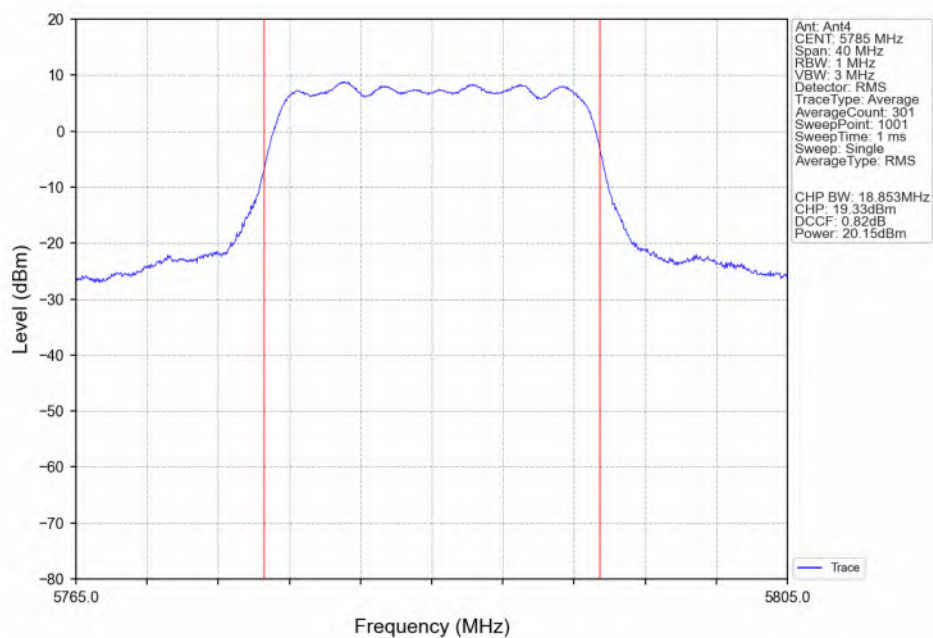
802.11ac(VHT20) MCH_5785MHz_Ant4_NTNV
