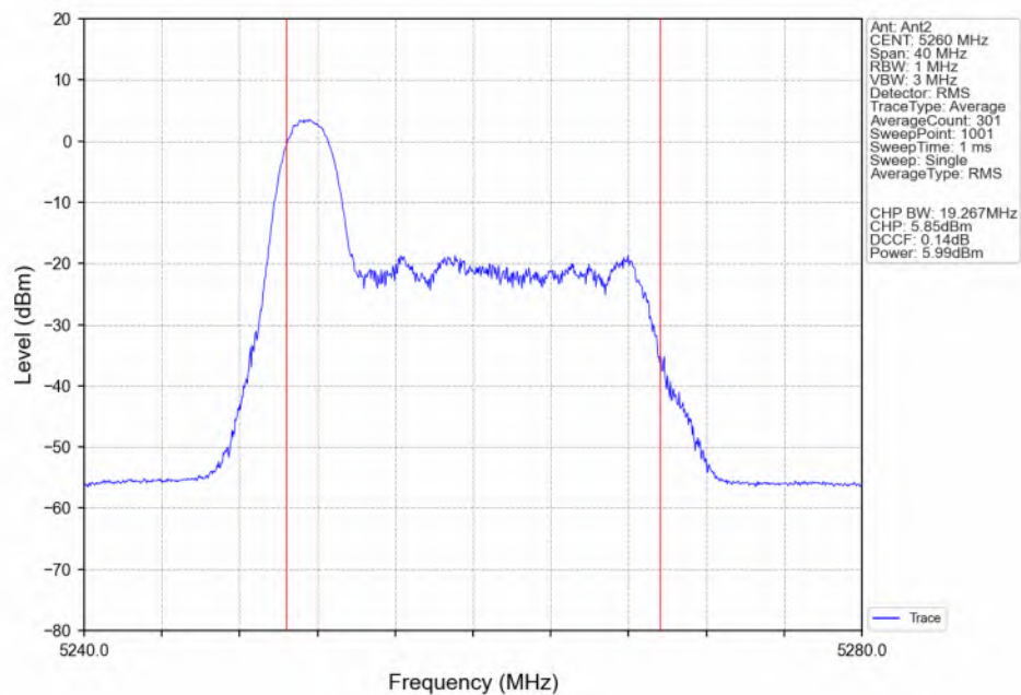
802.11ax(HEW20)_LCH_5260MHz_RU26_Left(0)_Ant2_NTNV
