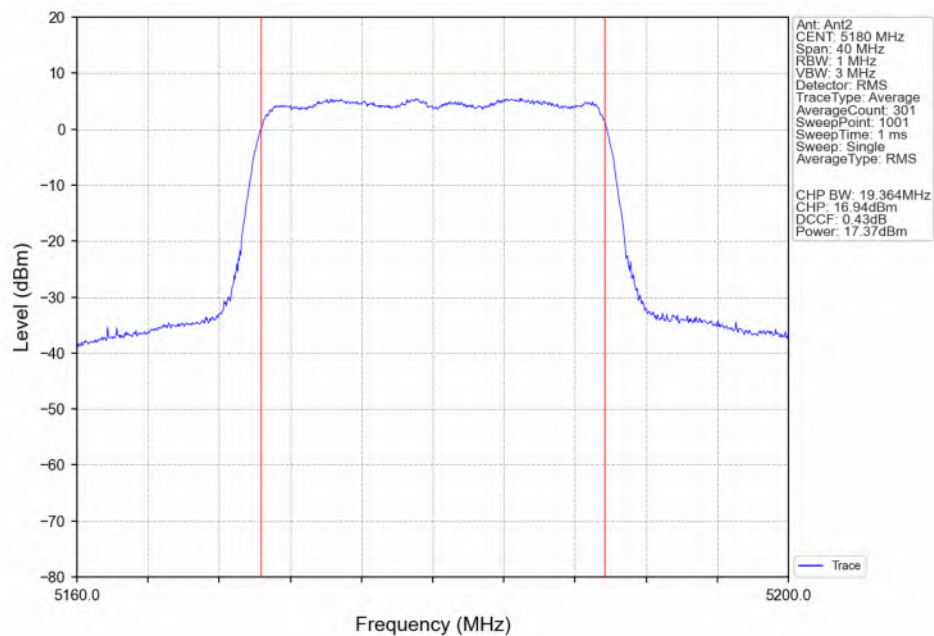
802.11ax(HEW20)_LCH_5180MHz_RU242_Left(61)_Ant2_NTNV
