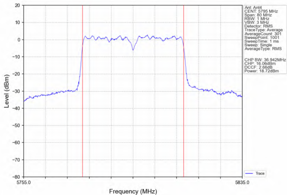
802.11n(HT40)_HCH_5795MHz_Ant4_NTNV
