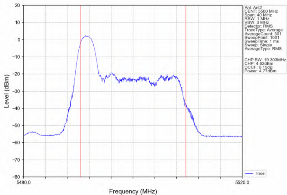
802.11ax(HEW20)_LCH_5500MHz_RU26_Left(0)_Ant2_NTNV
