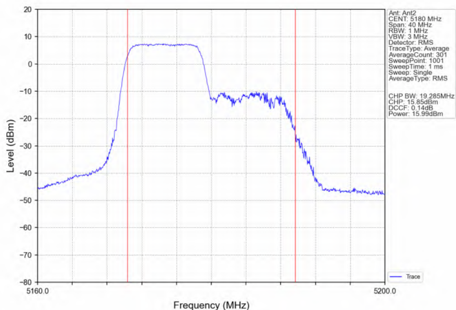
802.11ax(HEW20)_LCH_5180MHz_RU106_Left(53)_Ant2_NTNV
