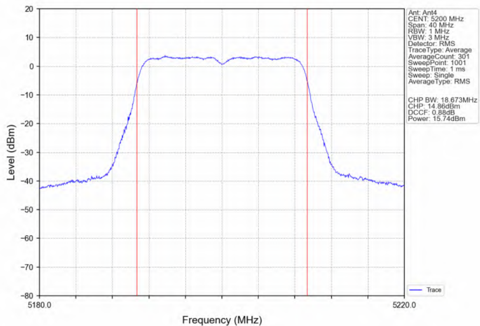
802.11ac(VHT20) MCH_5200MHz_Ant4_NTNV
