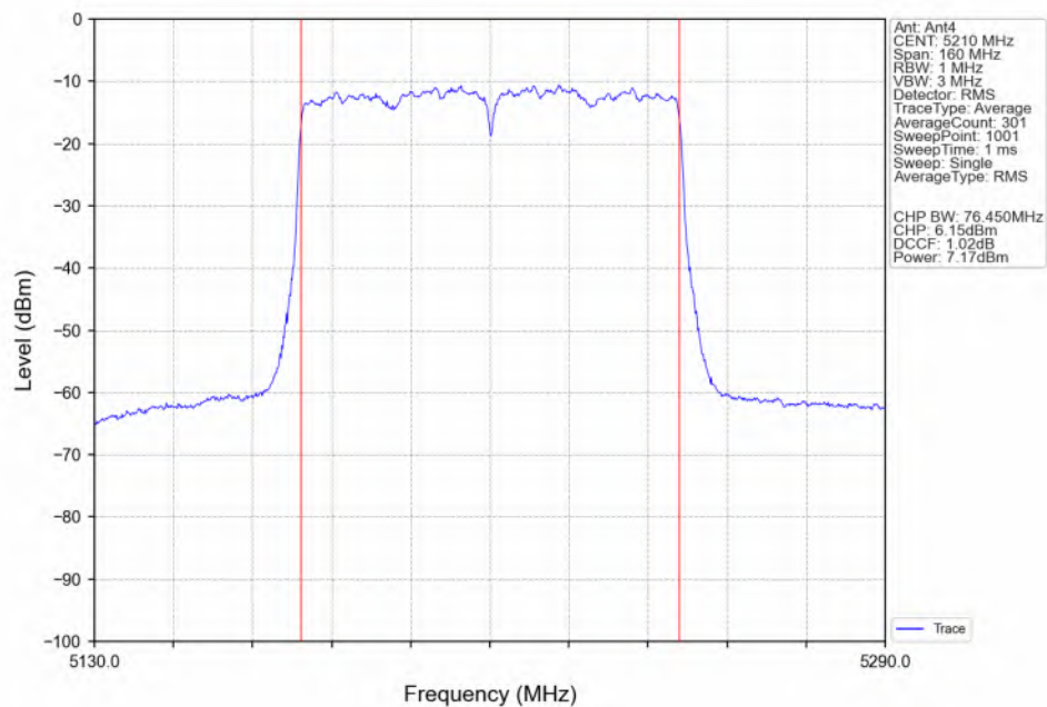
802.11ac(VHT80)_MCH_5210MHz_Ant4_NTNV
