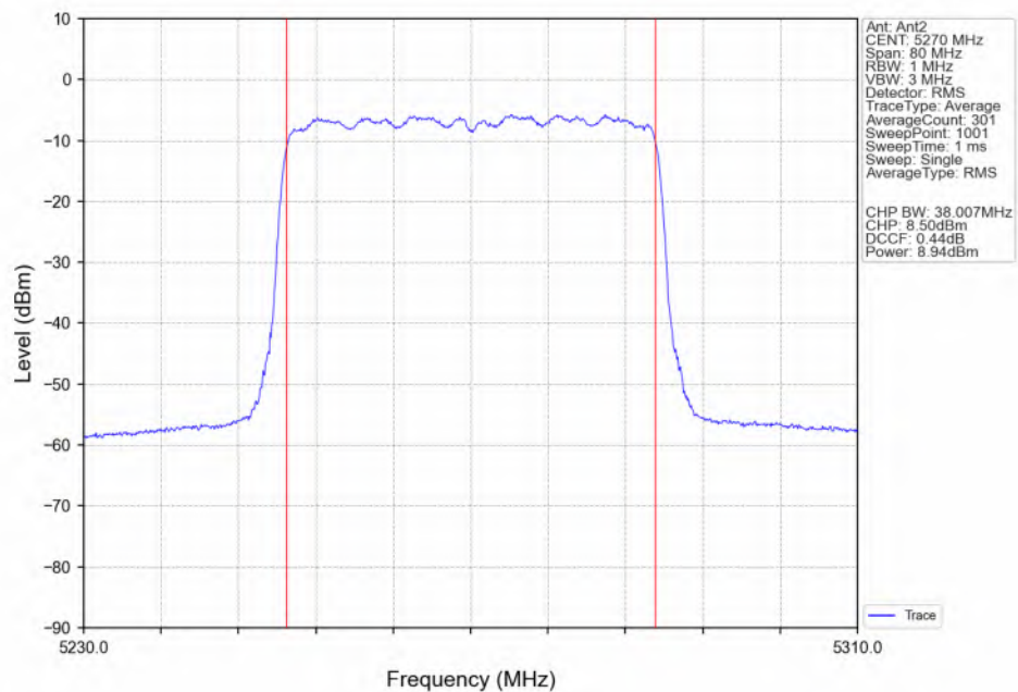
802.11ax(HEW40)_LCH_5270MHz_RU484_Left(65)_Ant2_NTNV
