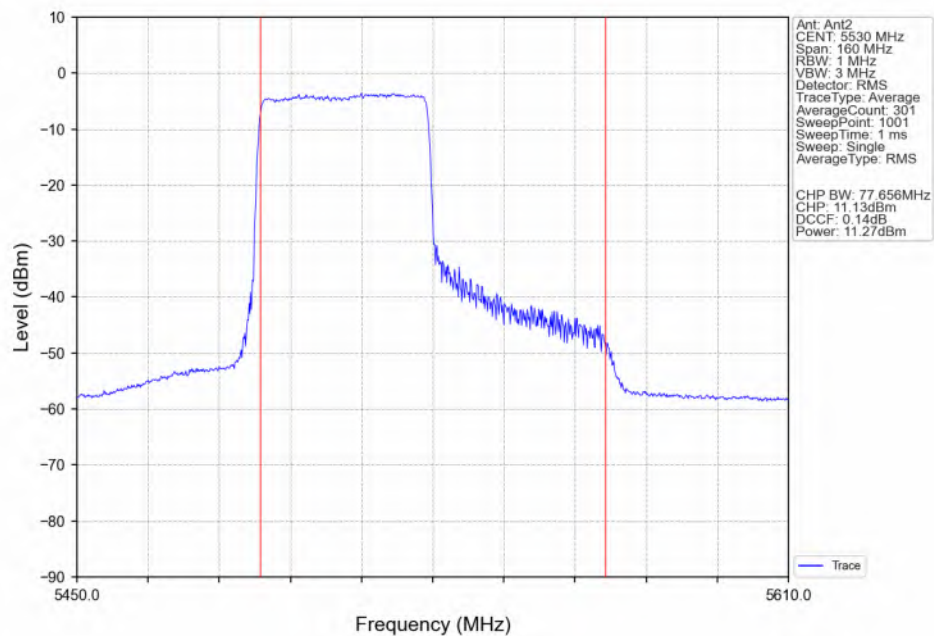
802.11ax(HEW80)_LCH_5530MHz_RU484_Left(65)_Ant2_NTNV
