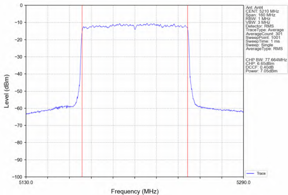
802.11ax(HEW80) MCH_5210MHz_RU996 Left(67)_Ant4_NTNV
