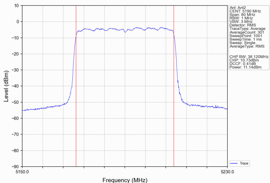
802.11ax(HEW40)_LCH_5190MHz_RU484_Left(65)_Ant2_NTNV
