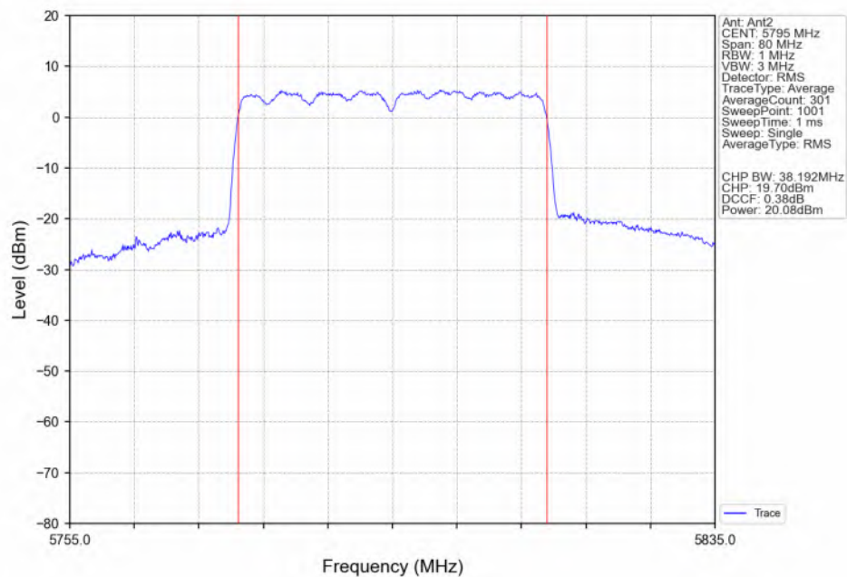
802.11ax(HEW40) HCH_5795MHz_RU484_Left(65)_Ant2_NTNV
