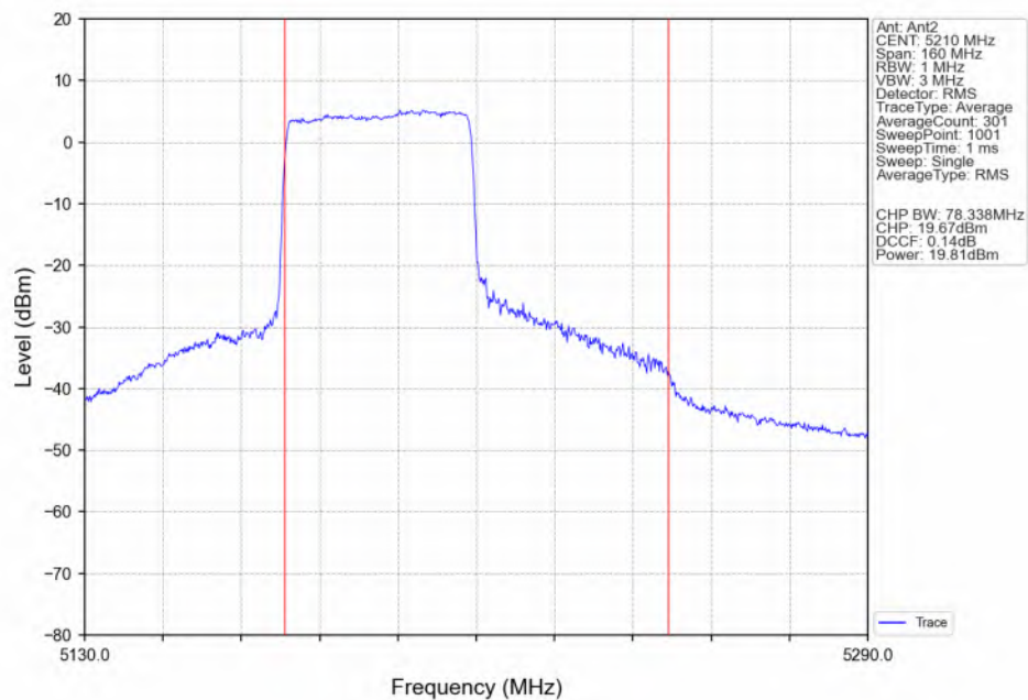
802.11ax(HEW80) MCH_5210MHz_RU484_Left(65)_Ant2_NTNV
