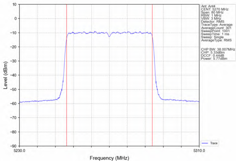
802.11ax(HEW40)_LCH_5270MHz_RU484_Left(65)_Ant4_NTNV
