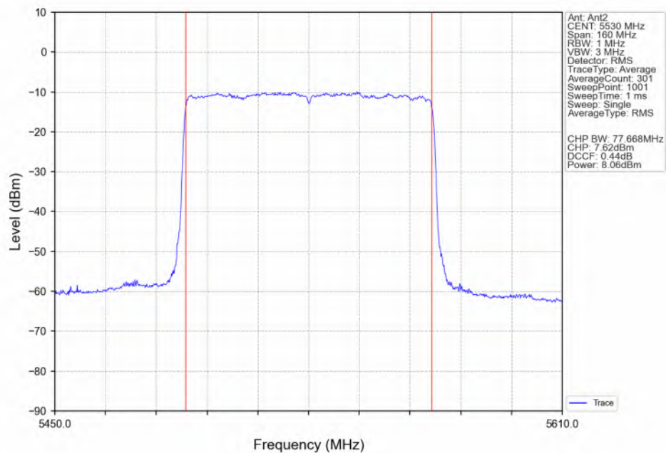
802.11ax(HEW80)_LCH_5530MHz_RU996_Left(67)_Ant2_NTNV
