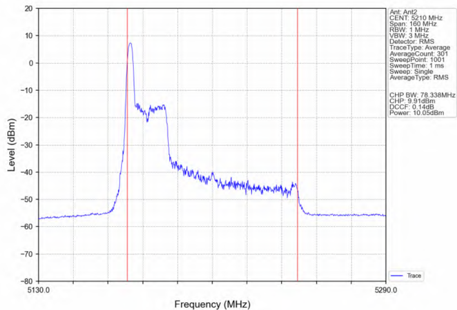
802.11ax(HEW80)_MCH_5210MHz_RU26_Left(0)_Ant2_NTNV
