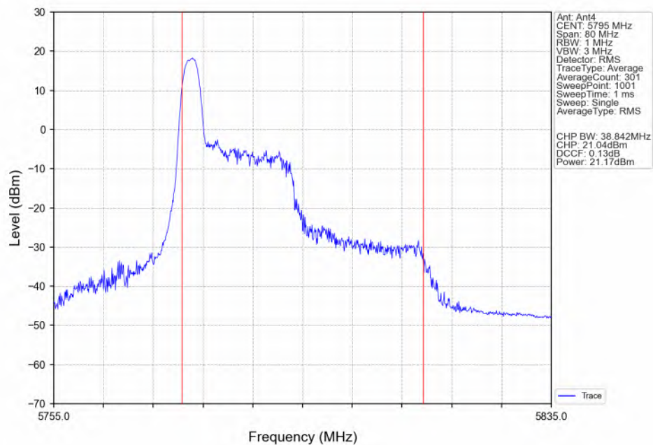
802.11ax(HEW40) HCH_5795MHz_RU26_Left(0)_Ant4_NTNV
