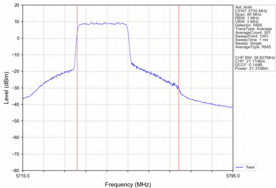
802.11ax(HEW40)_LCH_5755MHz_RU242_Left(61)_Ant4_NTNV
