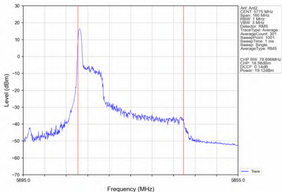
802.11ax(HEW80)_MCH_5775MHz_RU26_Left(0)_Ant2_NTNV
