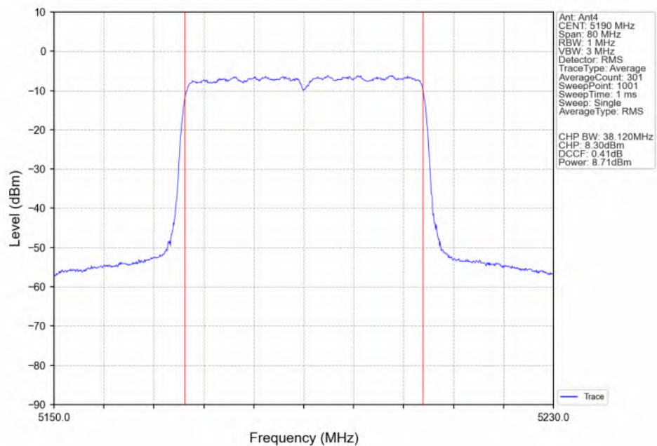
802.11ax(HEW40)_LCH_5190MHz_RU484_Left(65)_Ant4_NTNV
