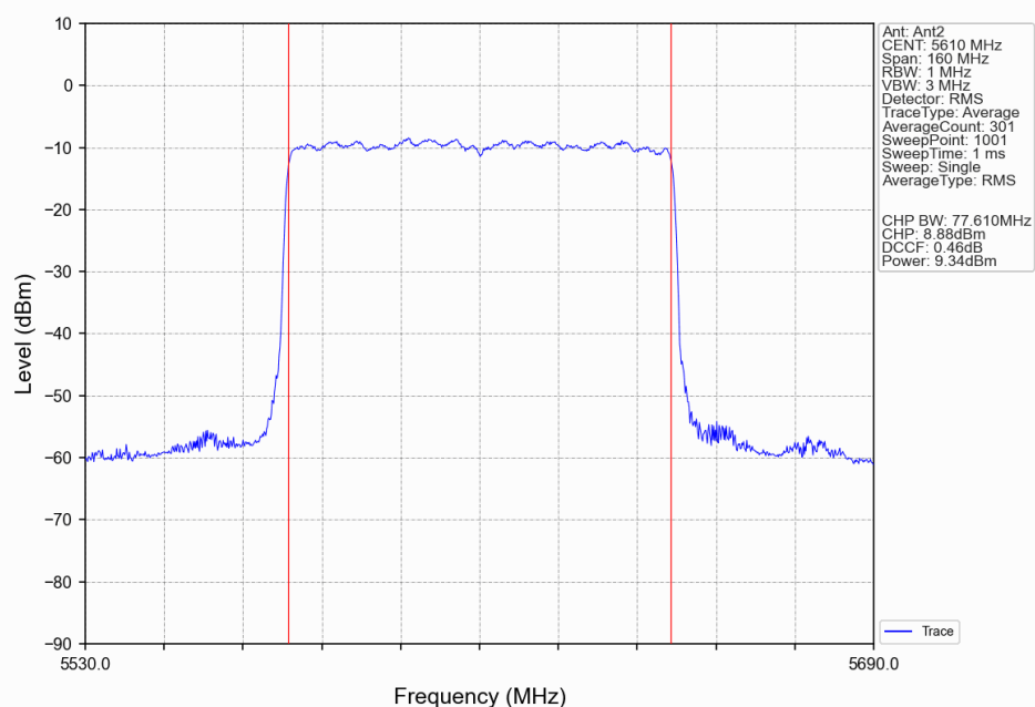
802.11ax(HEW80)_HCH_5610MHz_RU996_Left(67)_Ant2_NTNV
