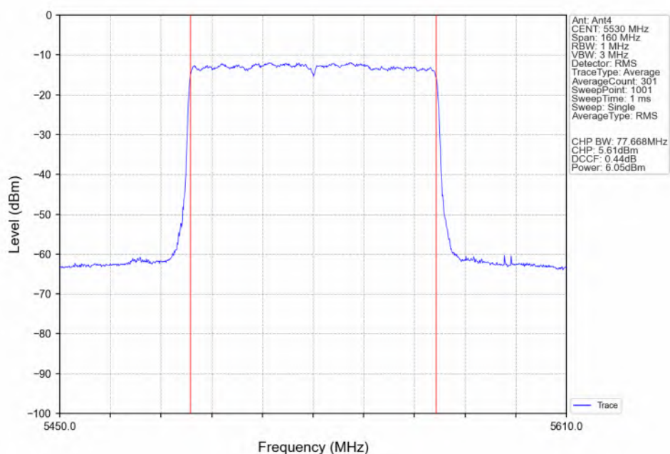
802.11ax(HEW80)_LCH_5530MHz_RU996_Left(67)_Ant4_NTNV
