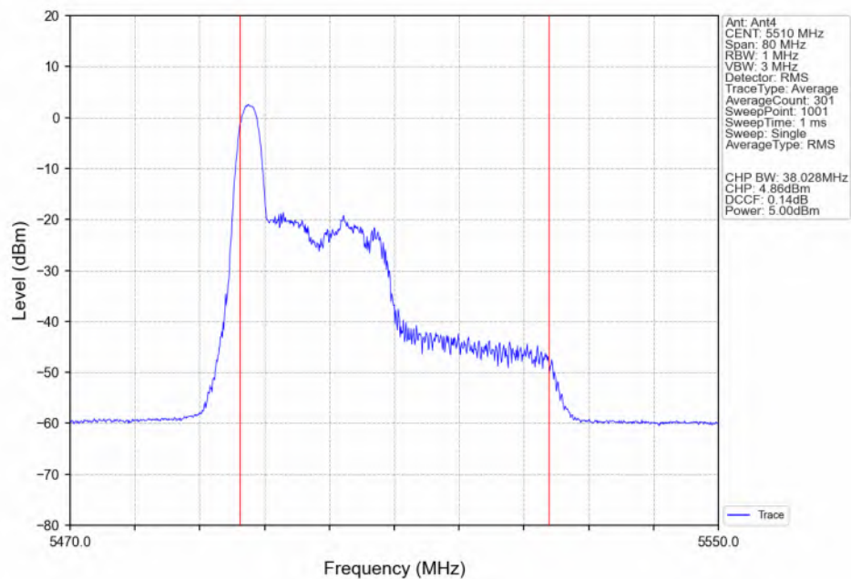
802.11ax(HEW40)_LCH_5510MHz_RU26_Left(0)_Ant4_NTNV
