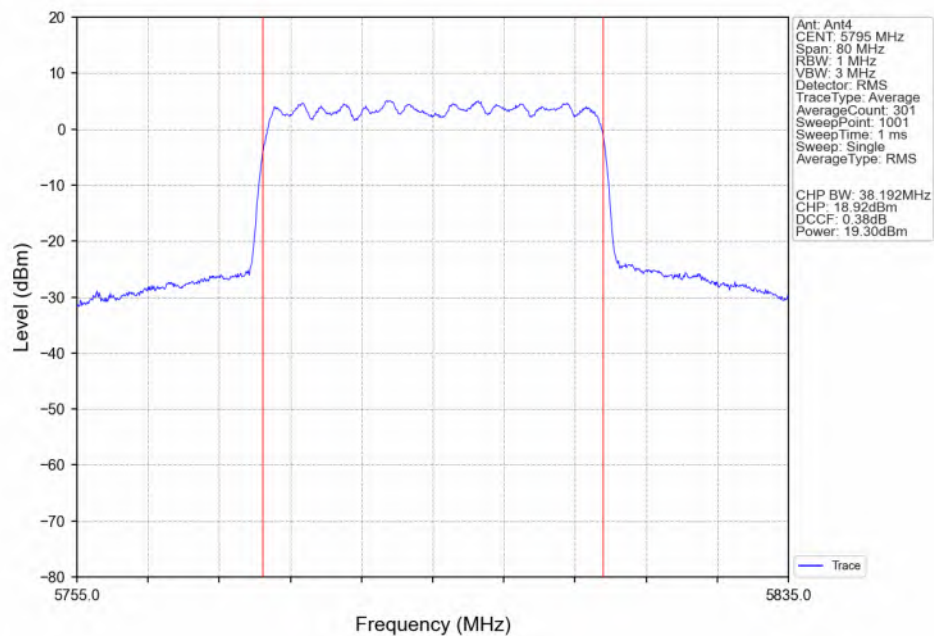
802.11ax(HEW40) HCH_5795MHz_RU484_Left(65)_Ant4_NTNV
