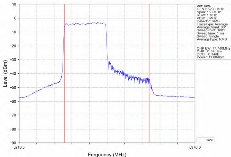
802.11ax(HEW80) MCH_5290MHz_RU484_Left(65)_Ant4_NTNV
