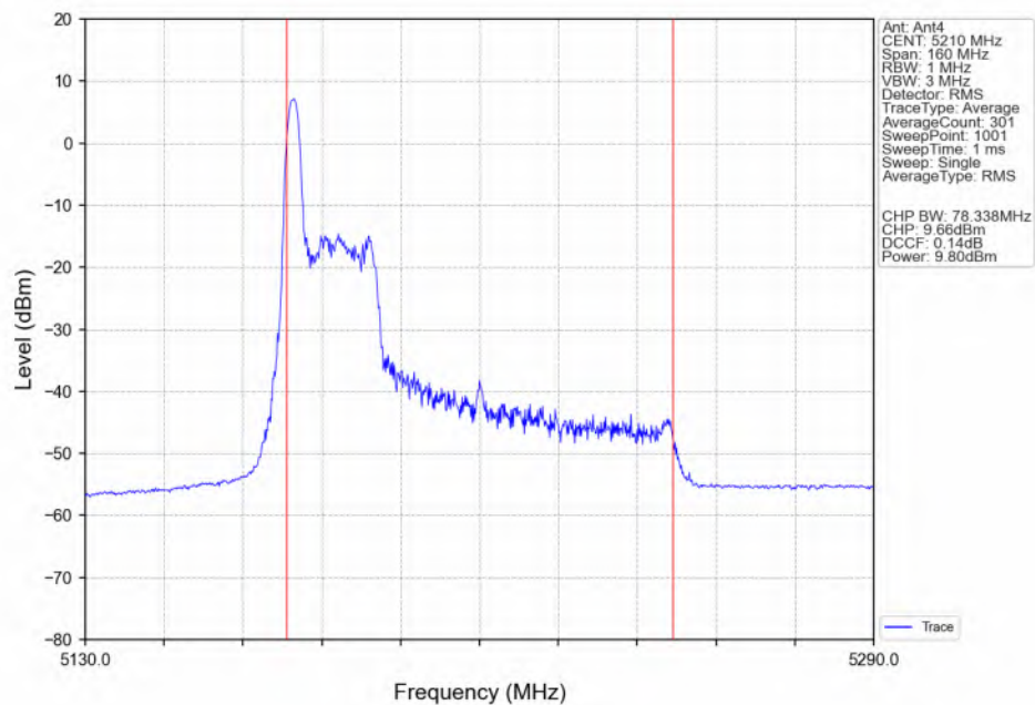
802.11ax(HEW80)_MCH_5210MHz_RU26_Left(0)_Ant4_NTNV
