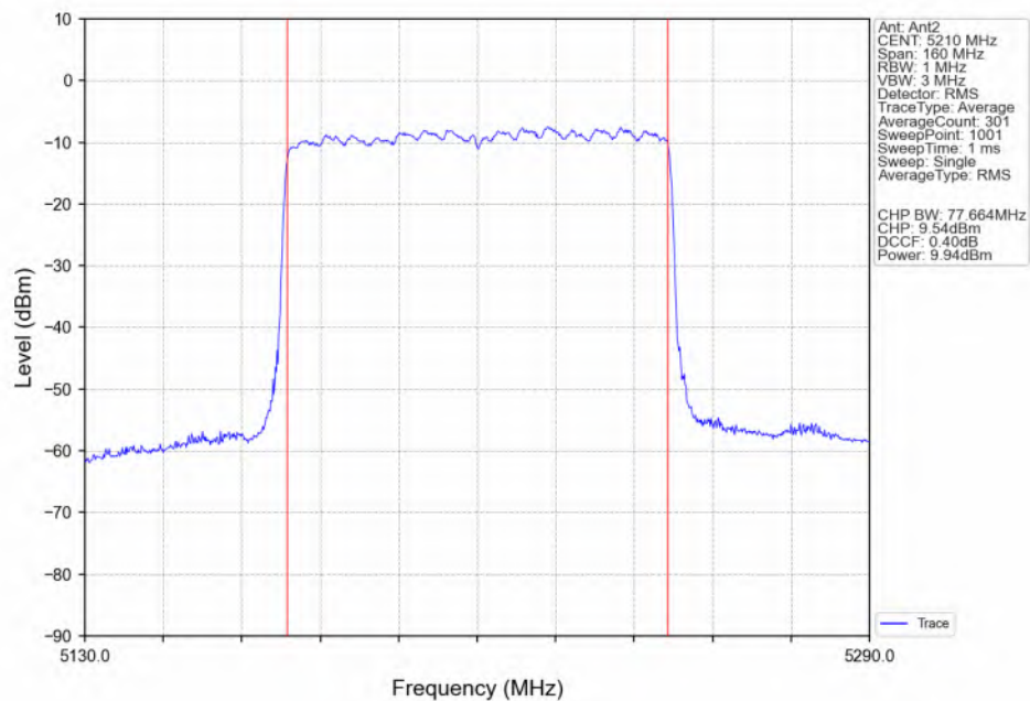
802.11ax(HEW80) MCH_5210MHz_RU996_Left(67)_Ant2_NTNV
