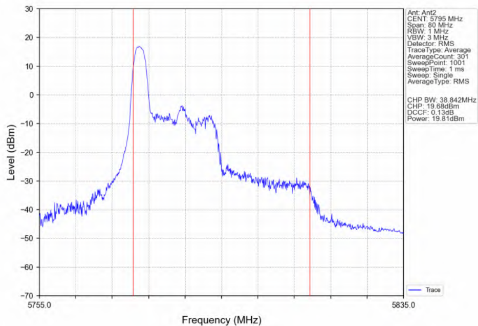
802.11ax(HEW40) HCH_5795MHz_RU26 Left(0)_Ant2_NTNV
