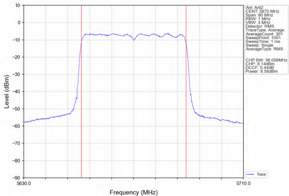
802.11ax(HEW40) HCH_5670MHz_RU484_Left(65)_Ant2_NTNV
