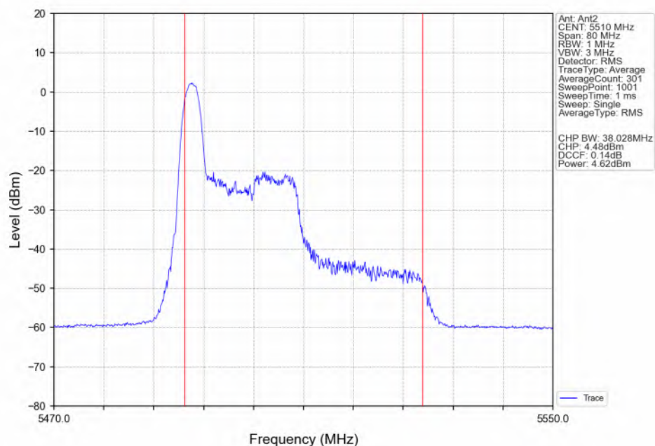
802.11ax(HEW40)_LCH_5510MHz_RU26_Left(0)_Ant2_NTNV
