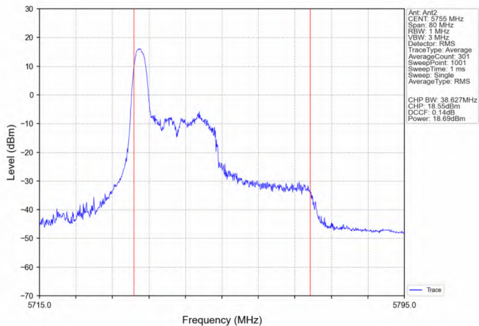
802.11ax(HEW40)_LCH_5755MHz_RU26_Left(0)_Ant2_NTNV
