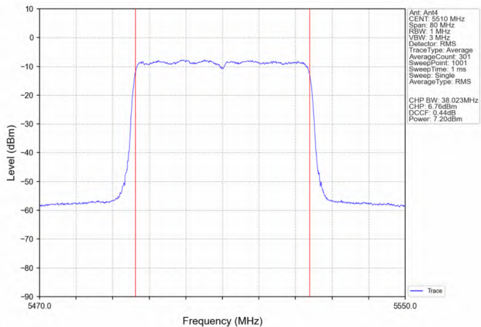
802.11ax(HEW40)_LCH_5510MHz_RU484_Left(65)_Ant4_NTNV
