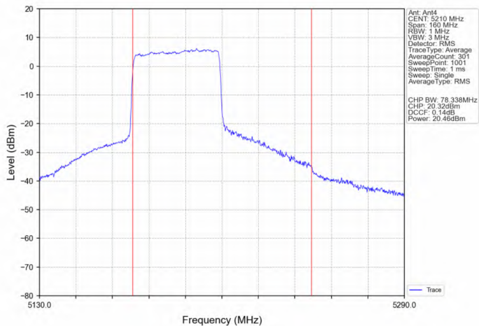
802.11ax(HEW80) MCH_5210MHz RU484 Left(65) Ant4 NTN
