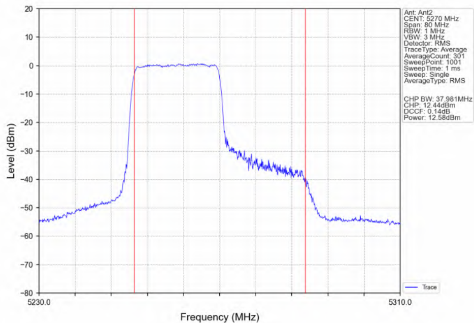
802.11ax(HEW40)_LCH_5270MHz_RU242_Left(61)_Ant2_NTNV
