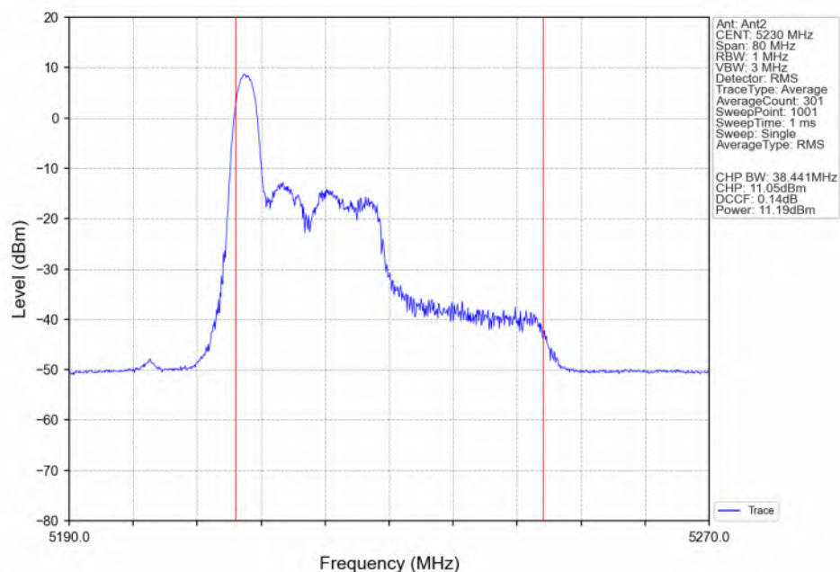
802.11ax(HEW40) HCH_5230MHz_RU26_Left(0)_Ant2_NTNV
