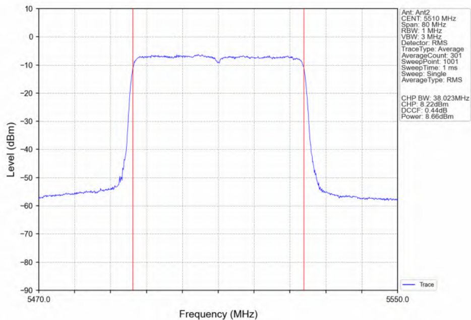
802.11ax(HEW40)_LCH_5510MHz_RU484_Left(65)_Ant2_NTNV
