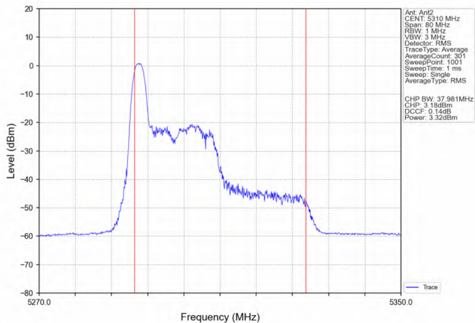
802.11ax(HEW40) HCH_5310MHz_RU26_Left(0)_Ant2_NTNV
