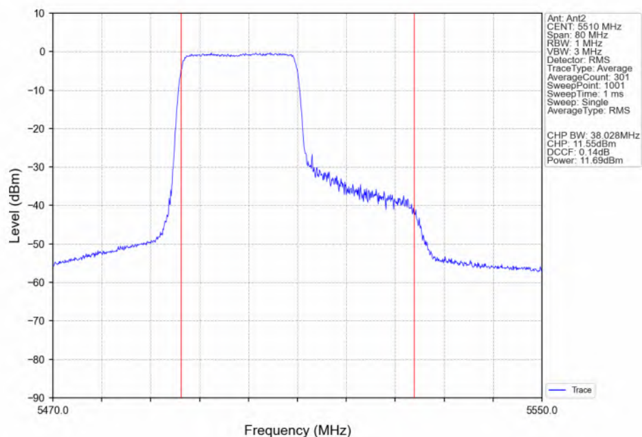
802.11ax(HEW40)_LCH_5510MHz_RU242_Left(61)_Ant2_NTNV
