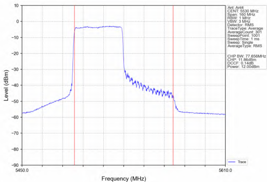
802.11ax(HEW80)_LCH_5530MHz_RU484_Left(65)_Ant4_NTNV
