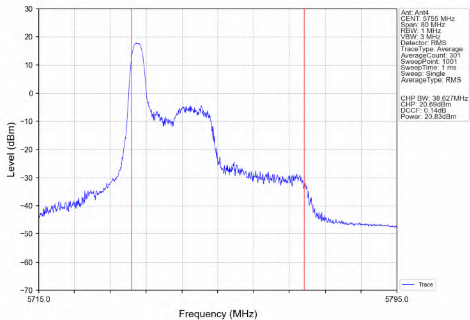
802.11ax(HEW40)_LCH_5755MHz_RU26_Left(0)_Ant4_NTNV
