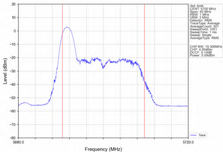
802.11ax(HEW20) HCH_5700MHz_RU26_Left(0)_Ant4_NTNV
