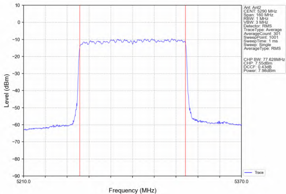
802.11ax(HEW80) MCH_5290MHz_RU996_Left(67)_Ant2_NTNV
