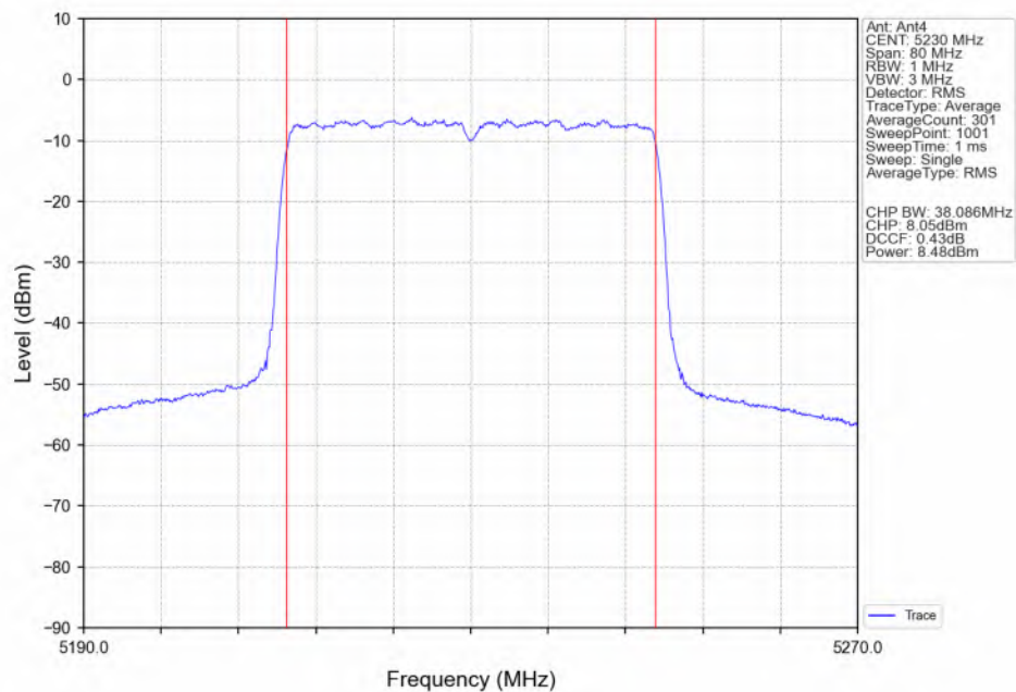
802.11ax(HEW40) HCH 5230MHz RU484 Left(65) Ant4 NTNv
