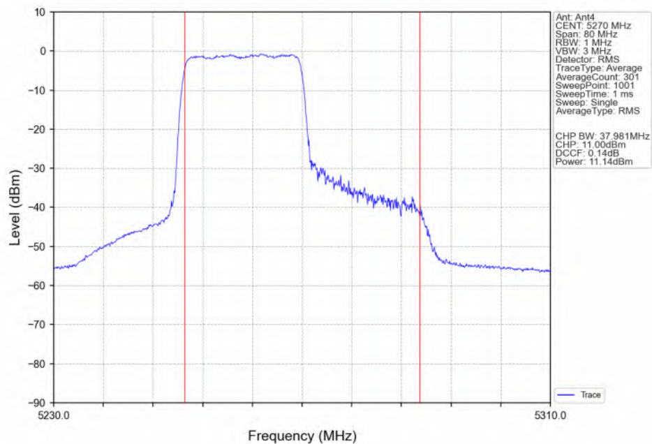
802.11ax(HEW40)_LCH_5270MHz_RU242_Left(61)_Ant4_NTNV
