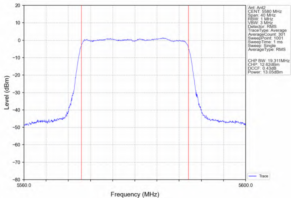
802.11ax(HEW20) MCH_5580MHz_RU242_Left(61)_Ant2_NTNV
