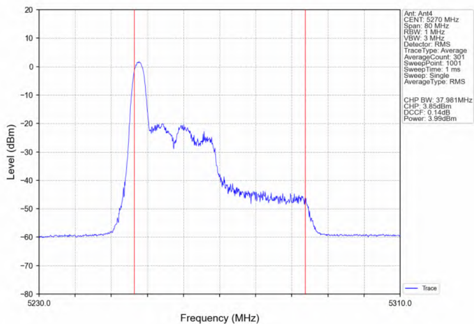
802.11ax(HEW40)_LCH_5270MHz_RU26_Left(0)_Ant4_NTNV
