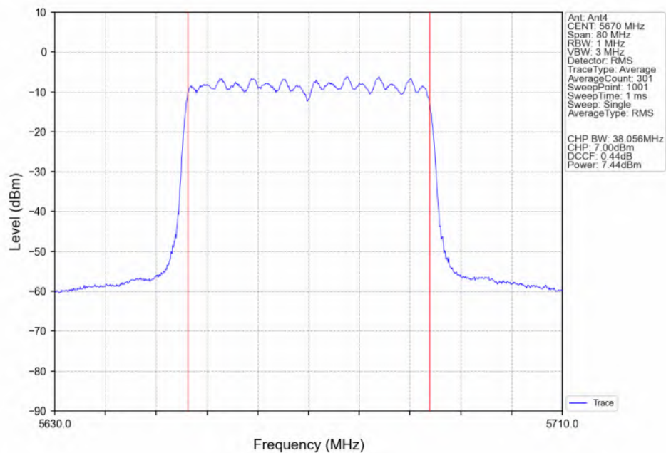
802.11ax(HEW40) HCH_5670MHz_RU484_Left(65)_Ant4_NTNV
