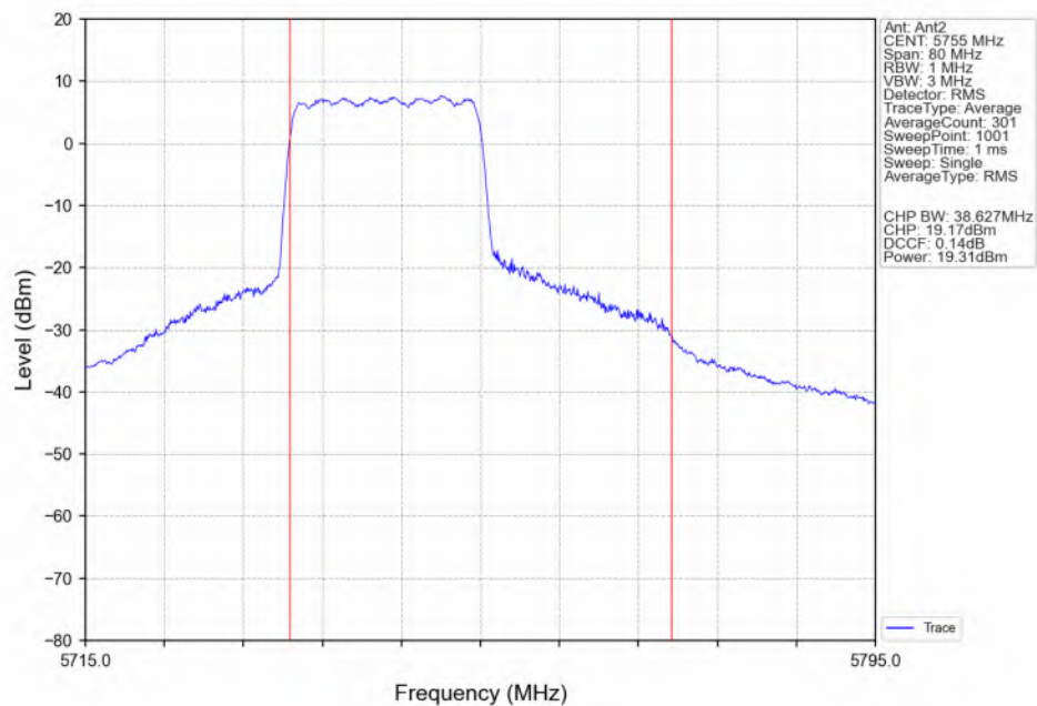
802.11ax(HEW40)_LCH_5755MHz_RU242_Left(61)_Ant2_NTNV
