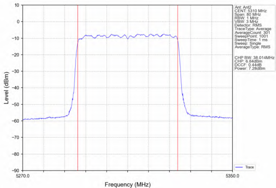
802.11ax(HEW40) HCH_5310MHz_RU484_Left(65)_Ant2_NTNV
