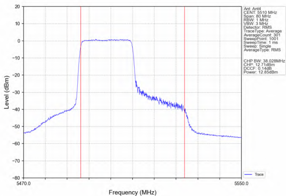
802.11ax(HEW40)_LCH_5510MHz_RU242_Left(61)_Ant4_NTNV
