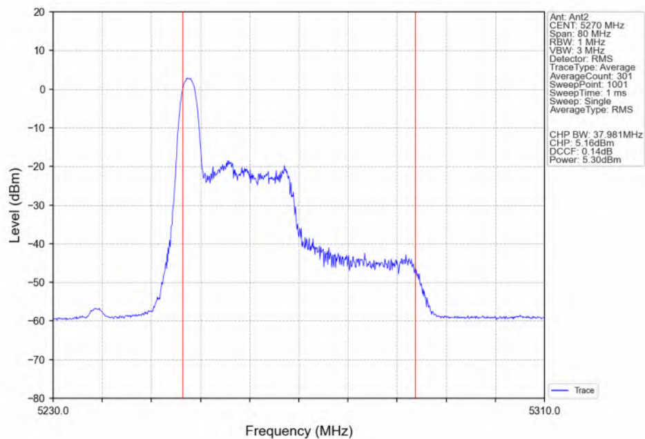
802.11ax(HEW40)_LCH_5270MHz_RU26_Left(0)_Ant2_NTNV
