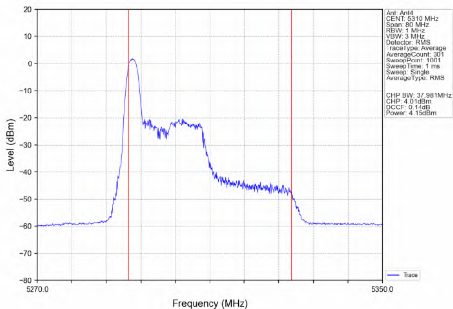
802.11ax(HEW40) HCH_5310MHz_RU26_Left(0)_Ant4_NTNV
