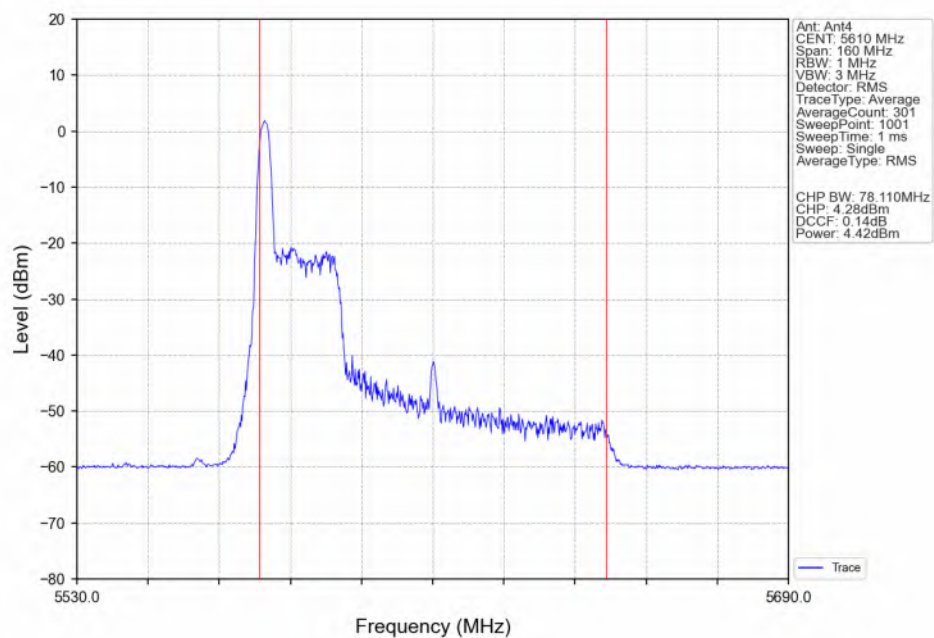
802.11ax(HEW80) HCH_5610MHz_RU26_Left(0)_Ant4_NTNV
