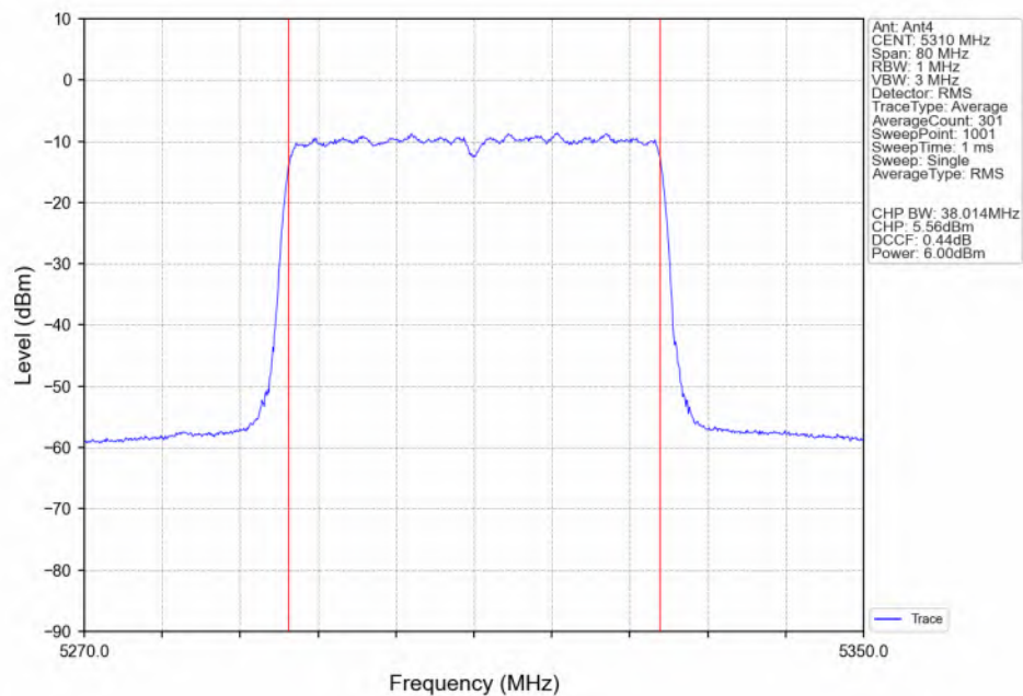
802.11ax(HEW40) HCH_5310MHz_RU484_Left(65)_Ant4_NTNV
