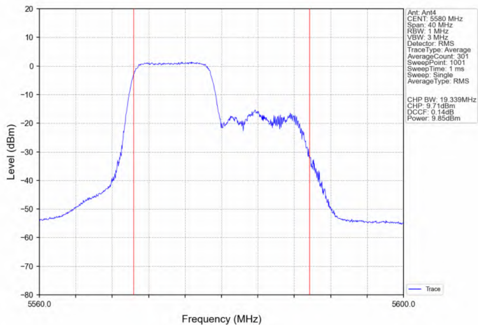
802.11ax(HEW20) MCH_5580MHz_RU106_Left(53)_Ant4_NTNV
