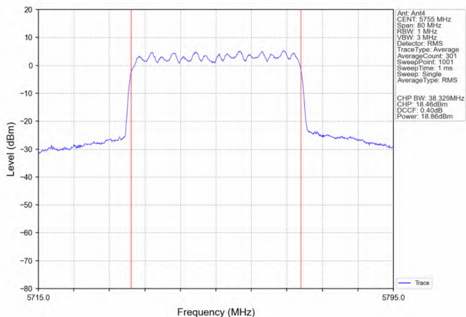
802.11ax(HEW40)_LCH_5755MHz_RU484_Left(65)_Ant4_NTNV
