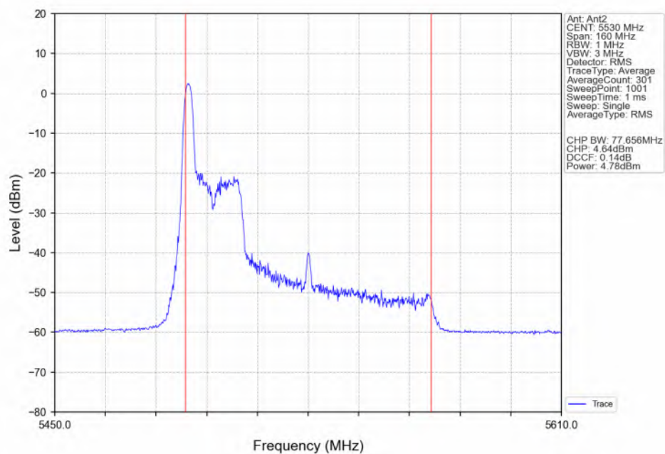
802.11ax(HEW80)_LCH_5530MHz_RU26_Left(0)_Ant2_NTNV
