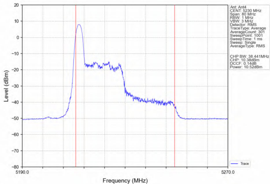
802.11ax(HEW40) HCH_5230MHz_RU26_Left(0)_Ant4_NTNV
