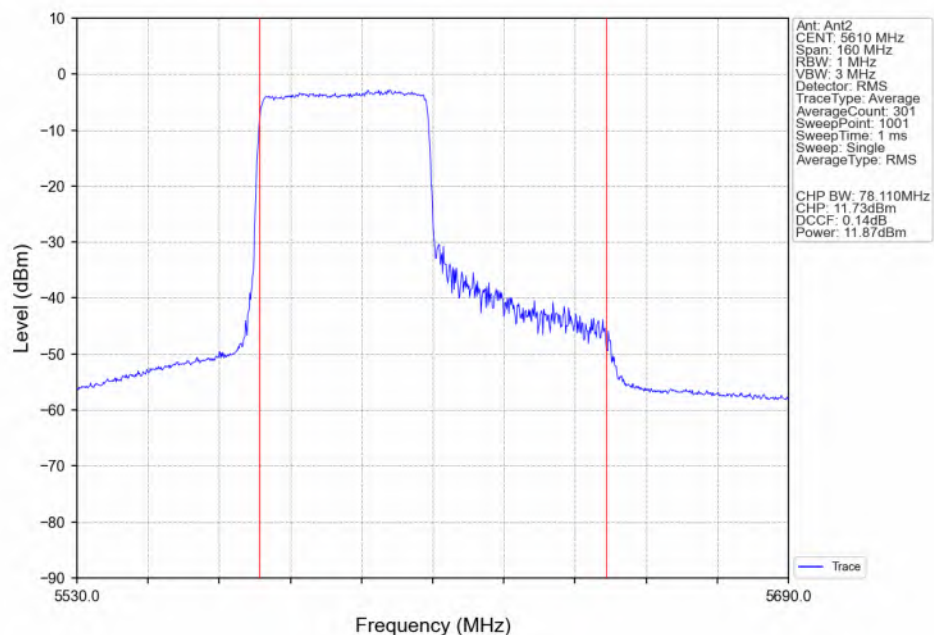
802.11ax(HEW80)_HCH_5610MHz_RU484_Left(65)_Ant2_NTNV
