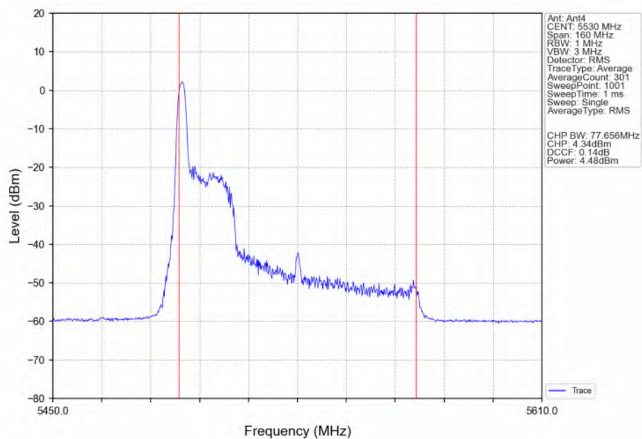
802.11ax(HEW80)_LCH_5530MHz_RU26_Left(0)_Ant4_NTNV
