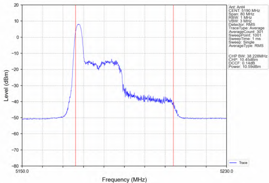
802.11ax(HEW40)_LCH_5190MHz_RU26_Left(0)_Ant4_NTNV
