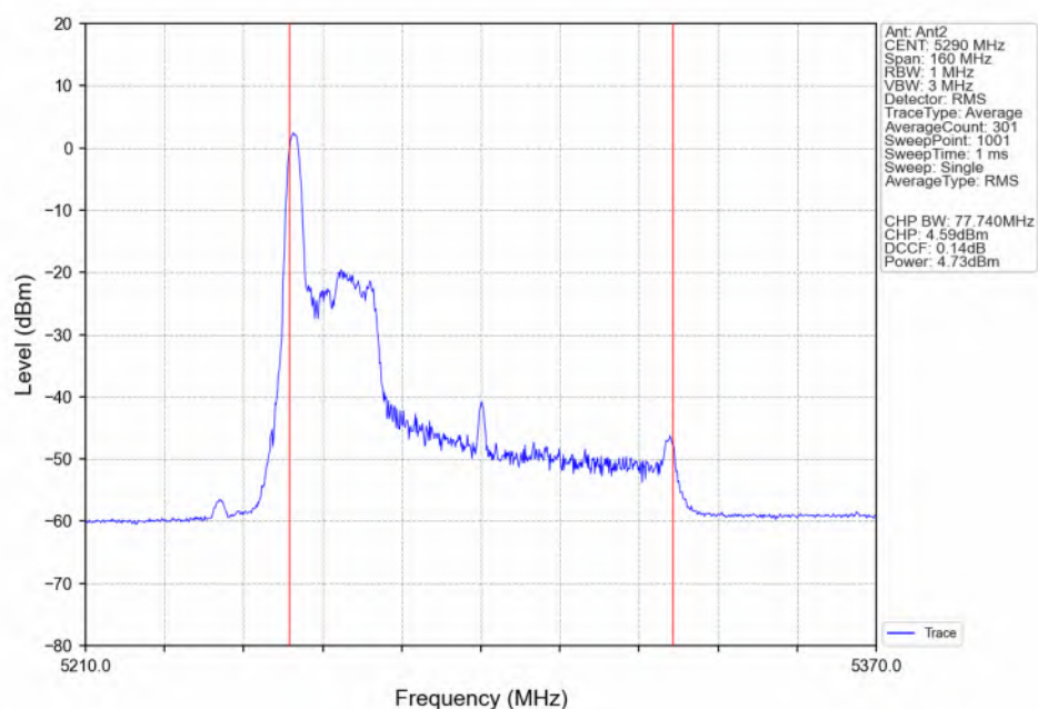
802.11ax(HEW80)_MCH_5290MHz_RU26_Left(0)_Ant2_NTNV
