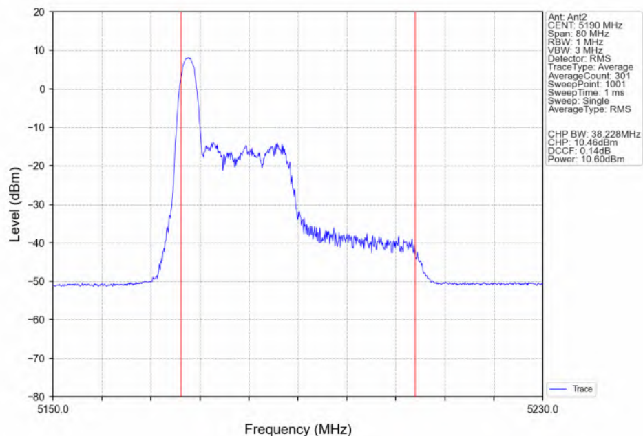
802.11ax(HEW40)_LCH_5190MHz_RU26_Left(0)_Ant2_NTNV
