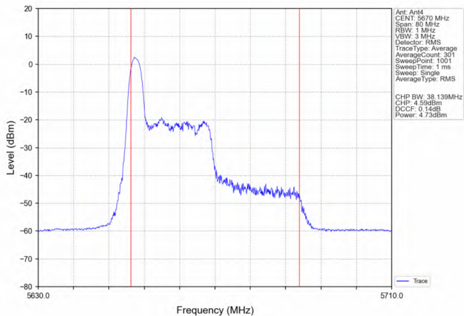
802.11ax(HEW40) HCH_5670MHz_RU26_Left(0)_Ant4_NTNV
