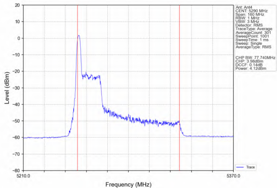
802.11ax(HEW80)_MCH_5290MHz_RU26_Left(0)_Ant4_NTNV
