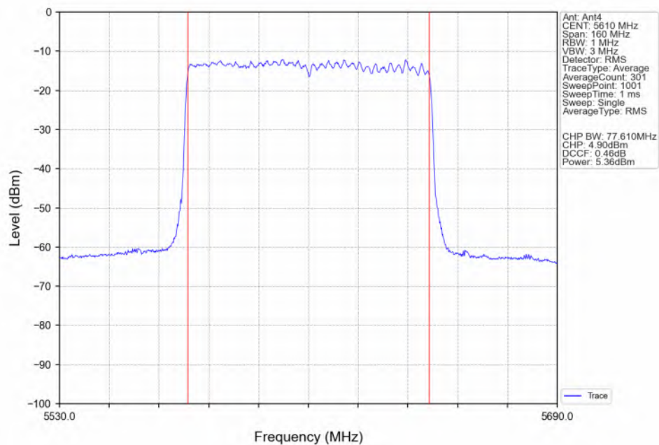
802.11ax(HEW80)_HCH_5610MHz_RU996_Left(67)_Ant4_NTNV
