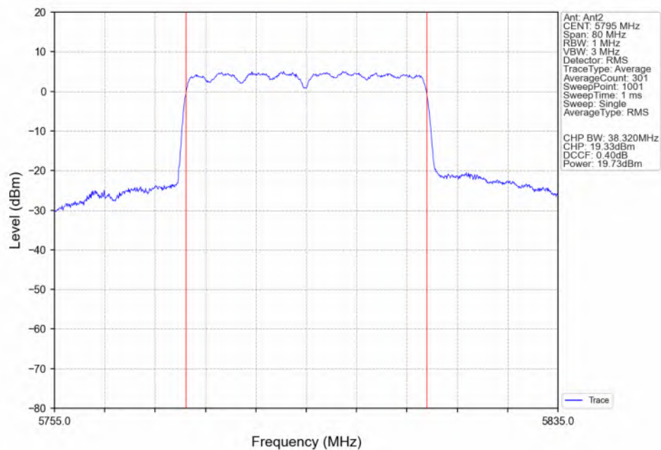
802.11be(EHT40)_HCH_5795MHz_RU484_Left(65)_Ant2_NTNV
