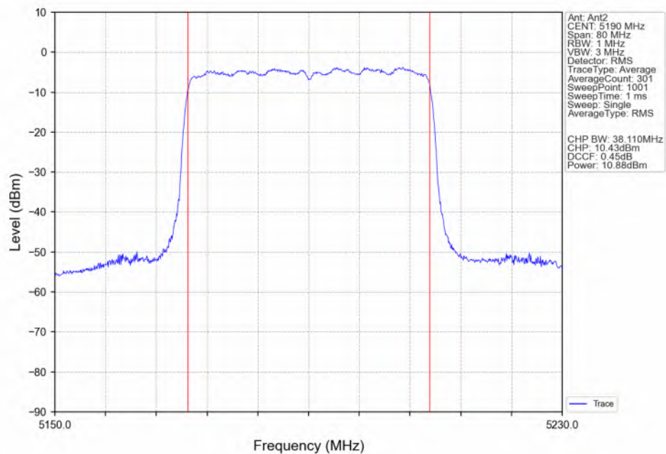
802.11be(EHT40) LCH_5190MHz_RU484_Left(65)_Ant2_NTNV
