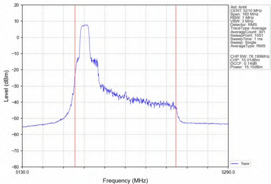
802.11be(EHT80)_MCH_5210MHz_26+52_/_Ant4_NTNV
