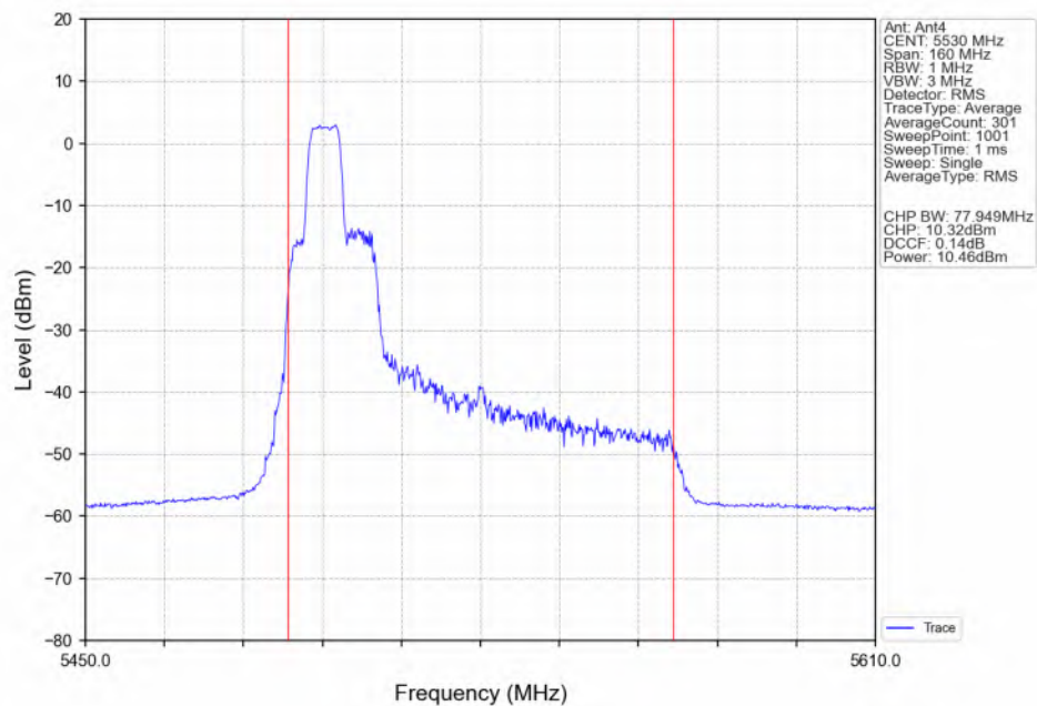
802.11be(EHT80)_LCH_5530MHz_26+52_ / Ant4_NTNV
