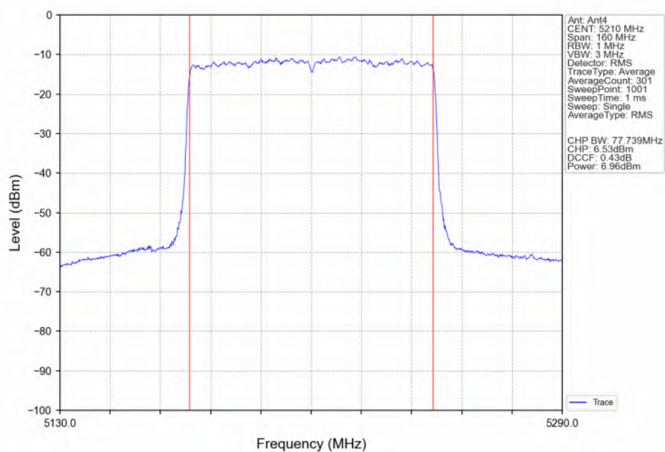
802.11be(EHT80)_MCH_5210MHz_RU996_Left(67)_Ant4_NTNV
