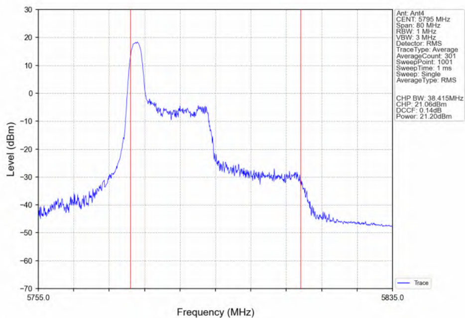
802.11be(EHT40)_HCH_5795MHz_RU26_Left(0)_Ant4_NTNV
