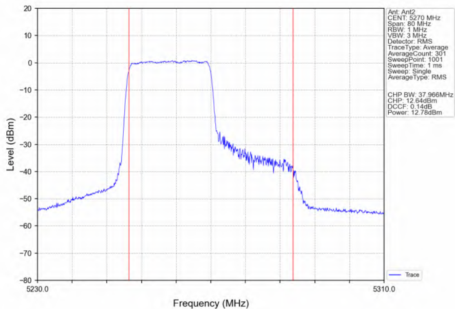
802.11be(EHT40) LCH_5270MHz_RU242_Left(61)_Ant2_NTNV
