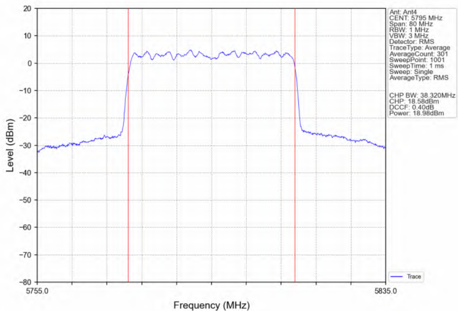
802.11be(EHT40)_HCH_5795MHz_RU484_Left(65)_Ant4_NTNV
