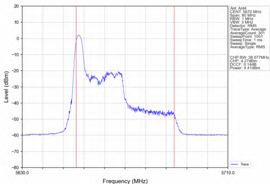
802.11be(EHT40)_HCH_5670MHz_RU26_Left(0)_Ant4_NTNV
