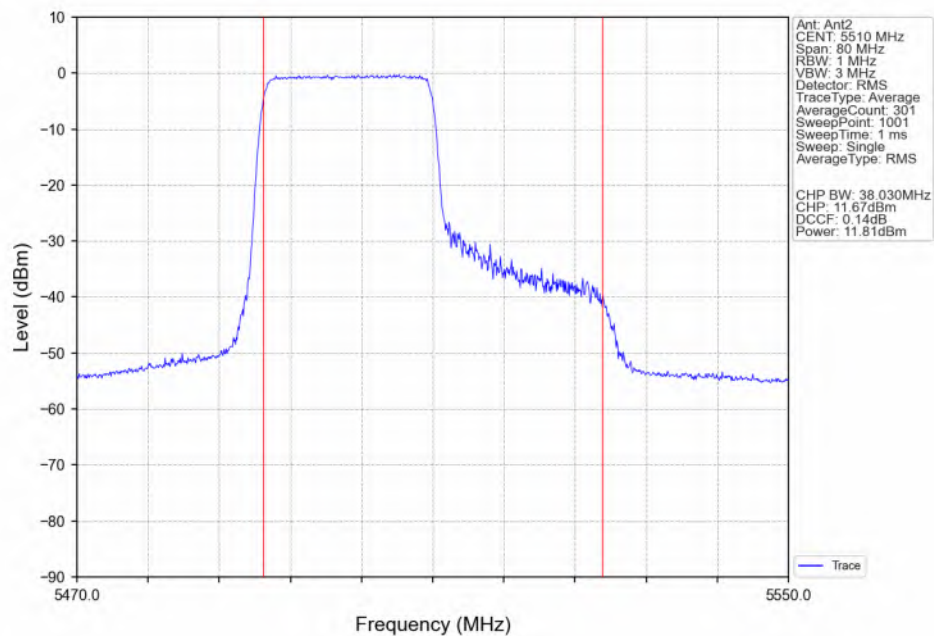
802.11be(EHT40) LCH_5510MHz_RU242_Left(61)_Ant2_NTNV
