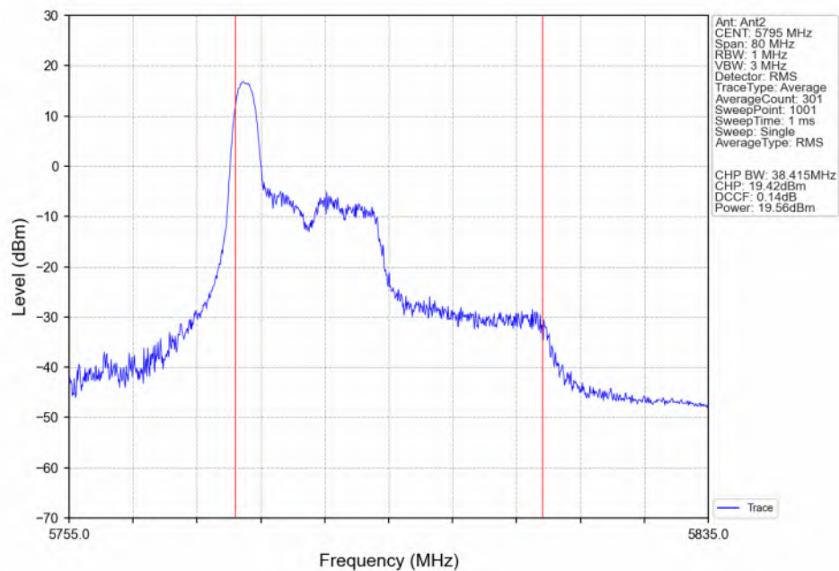
802.11be(EHT40)_HCH_5795MHz_RU26_Left(0)_Ant2_NTNV
