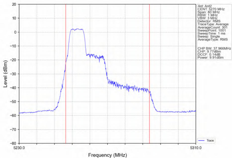
802.11be(EHT40)_LCH_5270MHz_26+52_ / Ant2_NTNV
