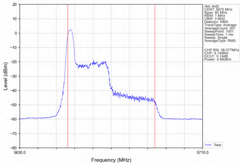
802.11be(EHT40)_HCH_5670MHz_RU26_Left(0)_Ant2_NTNV
