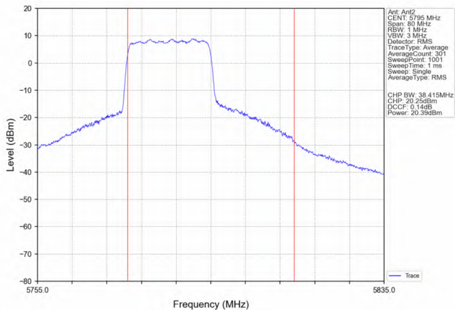
802.11be(EHT40)_HCH_5795MHz_RU242_Left(61)_Ant2_NTNV
