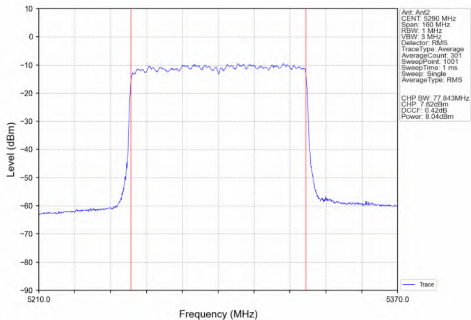
802.11be(EHT80)_MCH_5290MHz_RU996_Left(67)_Ant2_NTNV
