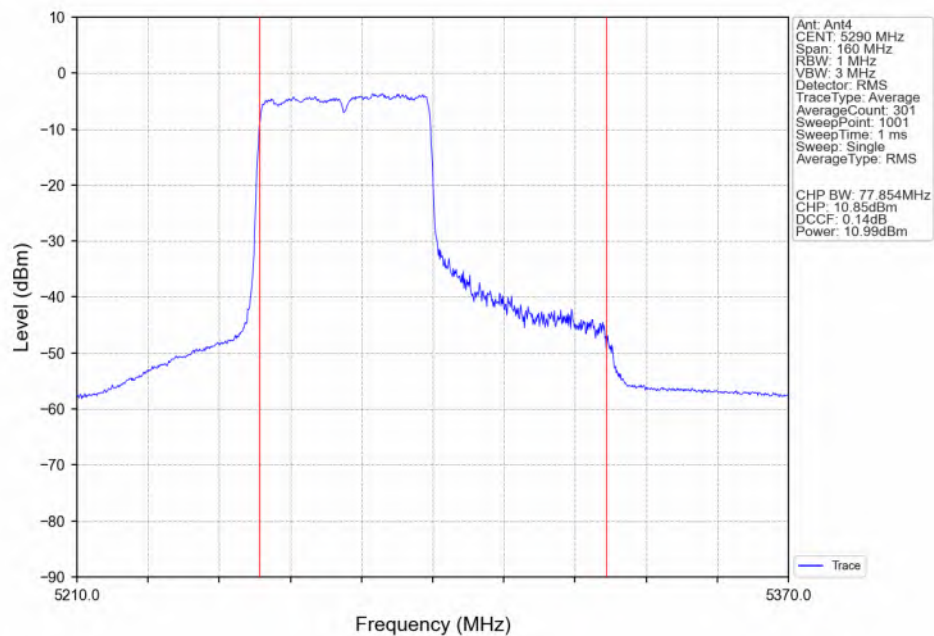
802.11be(EHT80)_MCH_5290MHz_RU484_Left(65)_Ant4_NTNV
