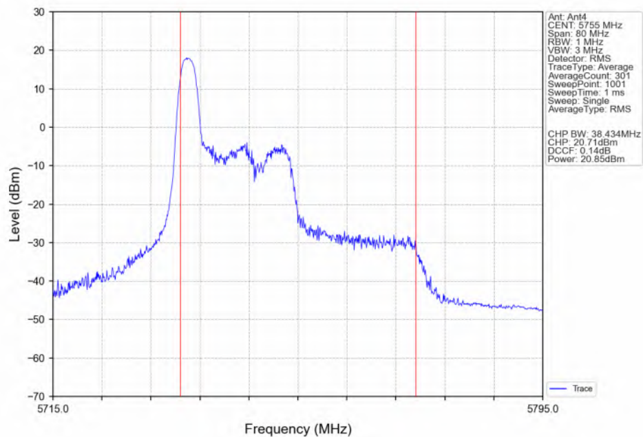
802.11be(EHT40) LCH_5755MHz_RU26_Left(0)_Ant4_NTNV
