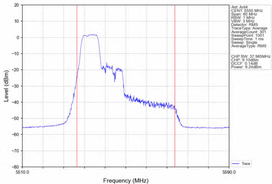
802.11be(EHT40) MCH 5550MHz 26+52 / Ant4_NTNV
