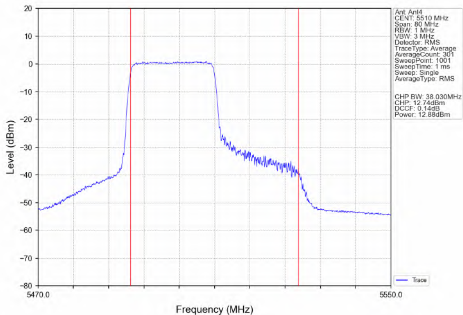
802.11be(EHT40) LCH_5510MHz_RU242_Left(61)_Ant4_NTNV
