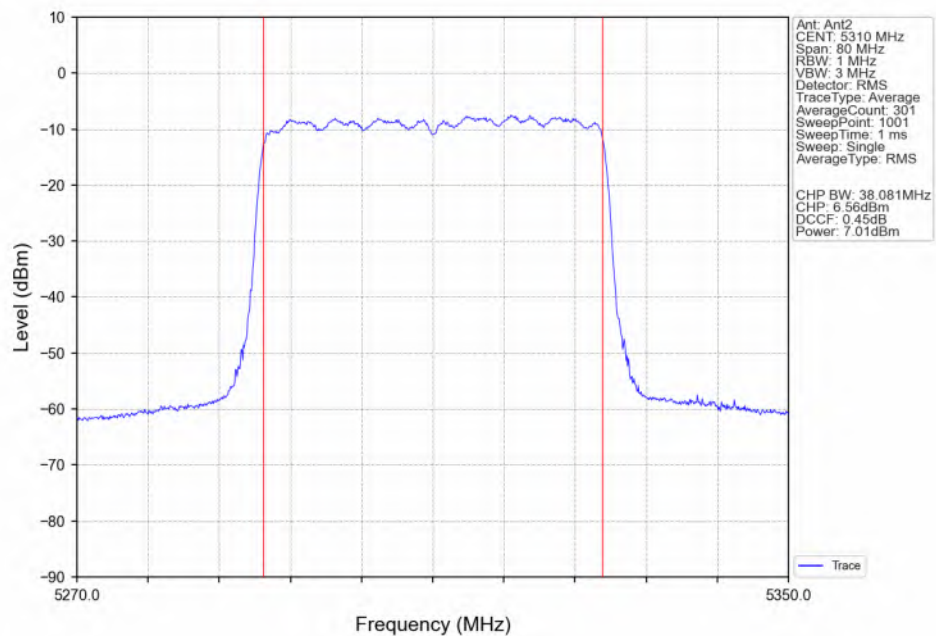
802.11be(EHT40)_HCH_5310MHz_RU484_Left(65)_Ant2_NTNV
