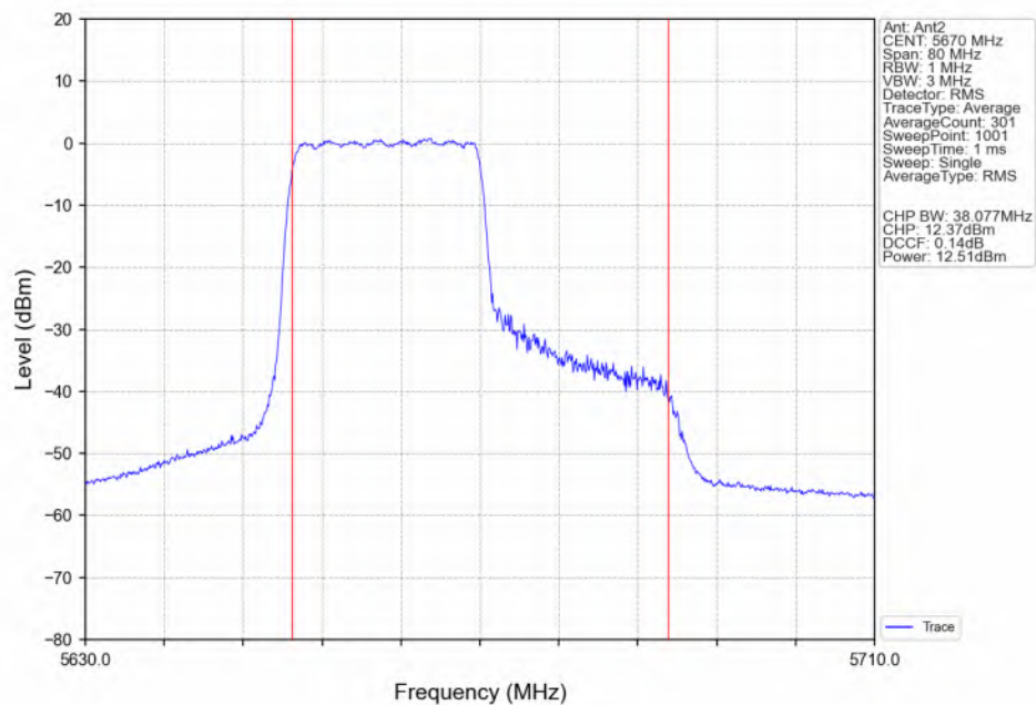
802.11be(EHT40)_HCH_5670MHz_RU242_Left(61)_Ant2_NTNV
