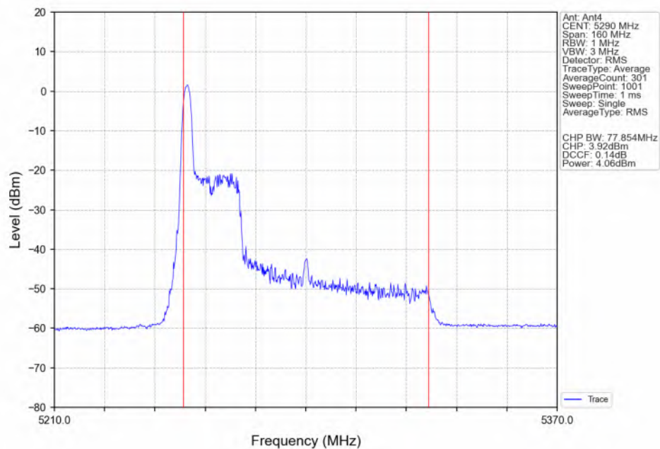
802.11be(EHT80)_MCH_5290MHz_RU26_Left(0)_Ant4_NTNV
