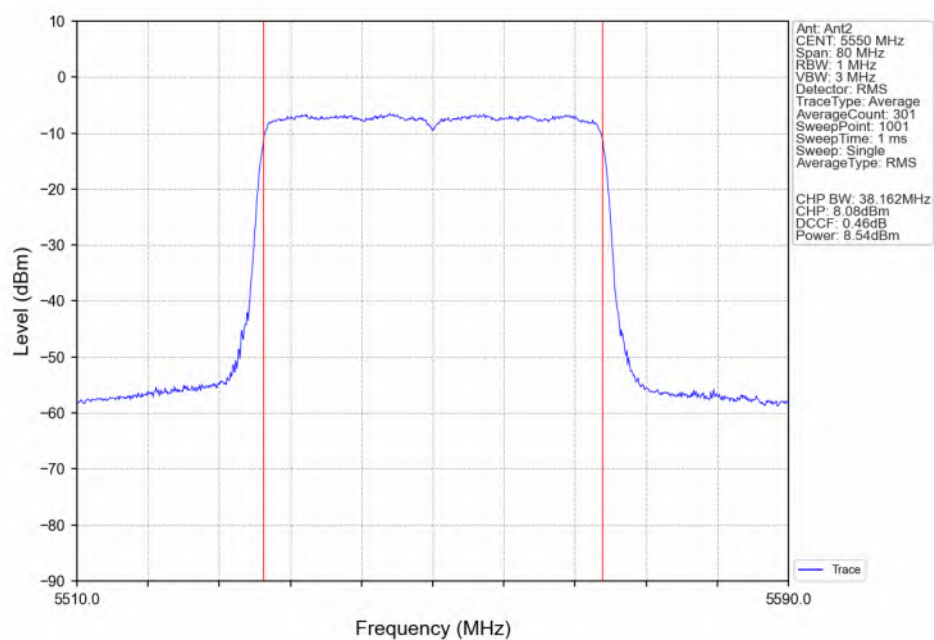
802.11be(EHT40)_MCH_5550MHz_RU484_Left(65)_Ant2_NTNV
