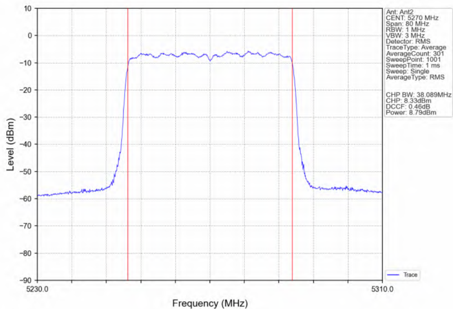
802.11be(EHT40) LCH_5270MHz_RU484_Left(65)_Ant2_NTNV
