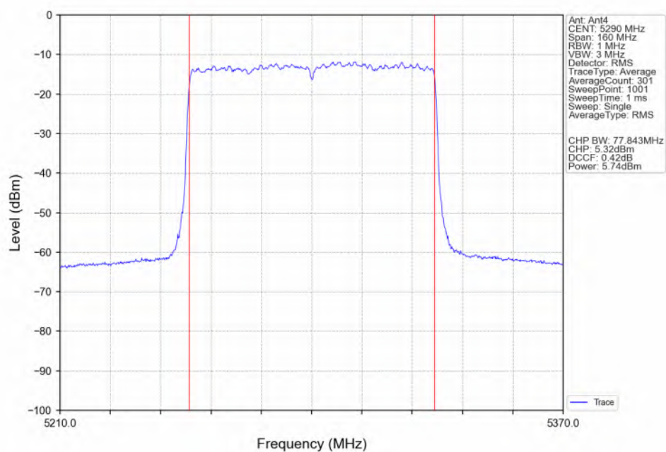
802.11be(EHT80)_MCH_5290MHz_RU996_Left(67)_Ant4_NTNV
