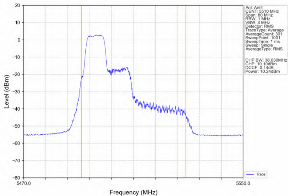
802.11be(EHT40)_LCH_5510MHz_26+52_ / Ant4_NTNV
