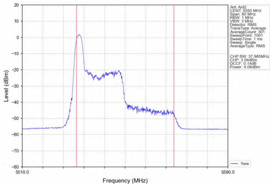
802.11be(EHT40)_MCH_5550MHz_RU26_Left(0)_Ant2_NTNV
