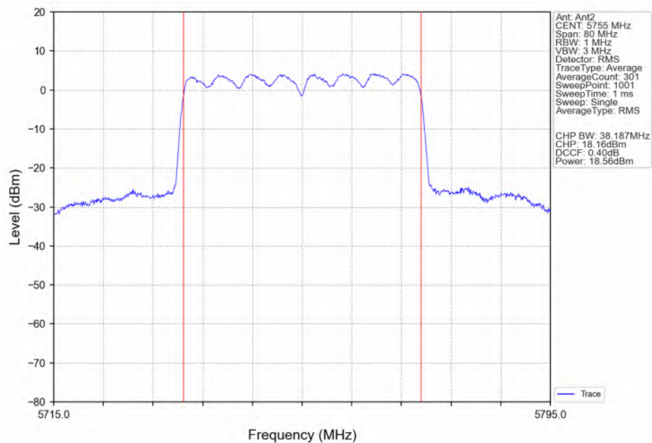
802.11be(EHT40) LCH_5755MHz_RU484_Left(65)_Ant2_NTNV
