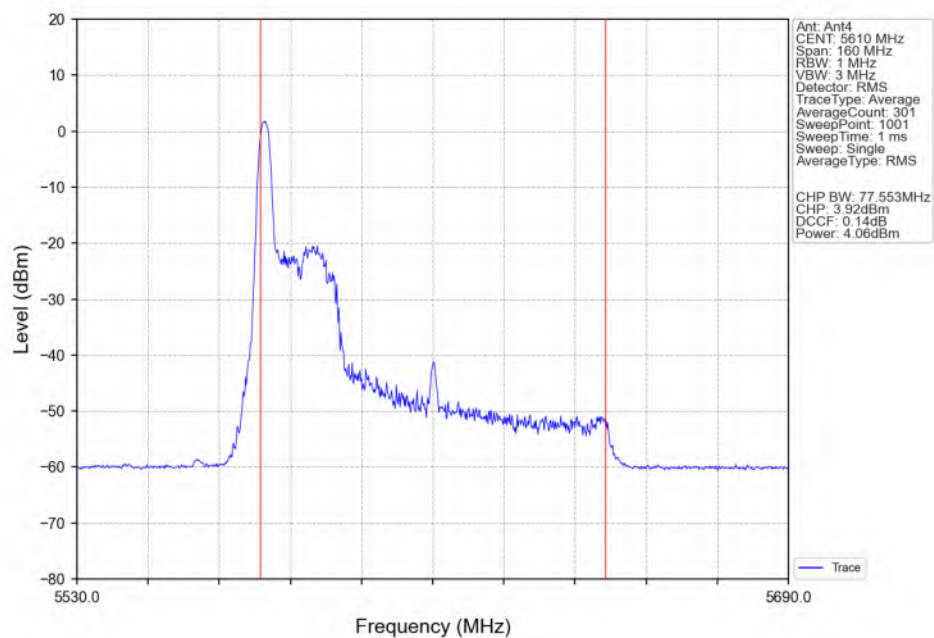
802.11be(EHT80)_HCH_5610MHz_RU26_Left(0)_Ant4_NTNV
