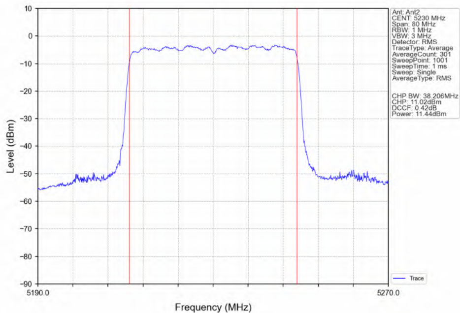
802.11be(EHT40)_HCH_5230MHz_RU484_Left(65)_Ant2_NTNV
