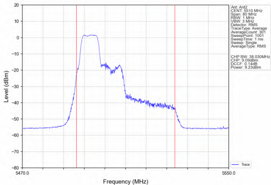
802.11be(EHT40)_LCH_5510MHz_26+52_ / Ant2_NTNV
