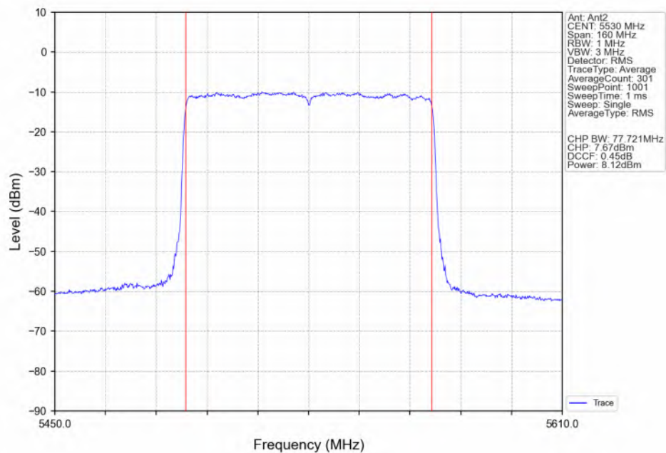
802.11be(EHT80) LCH_5530MHz_RU996_Left(67)_Ant2_NTNV
