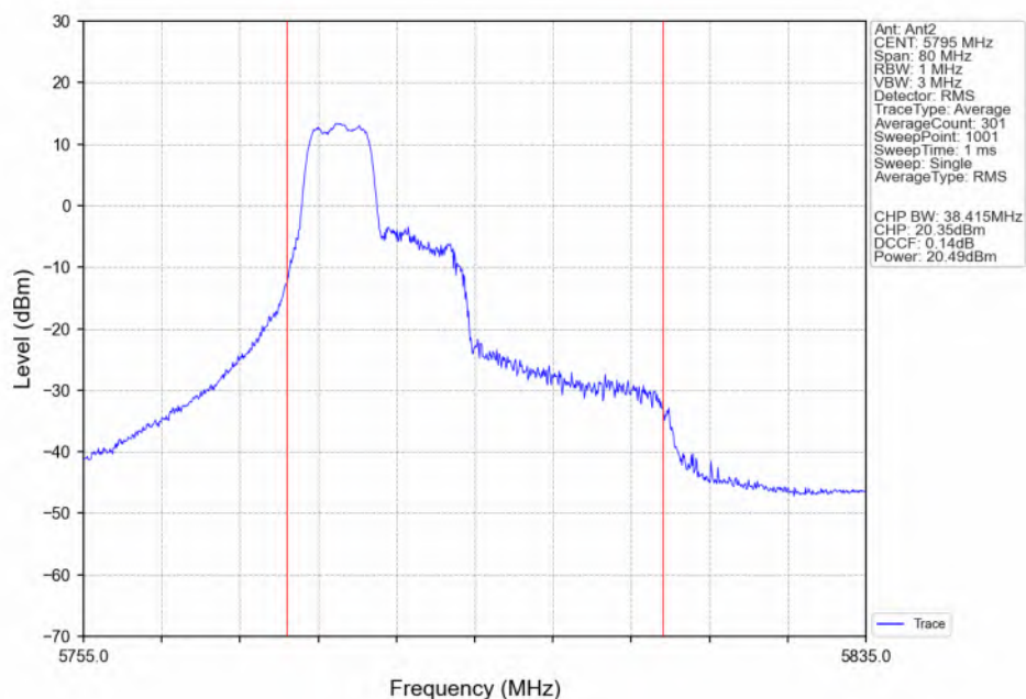
802.11be(EHT40) HCH 5795MHz 26+52 / Ant2_NTNV
