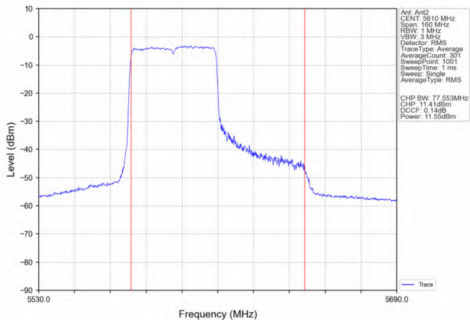
802.11be(EHT80)_HCH_5610MHz_RU484_Left(65)_Ant2_NTNV
