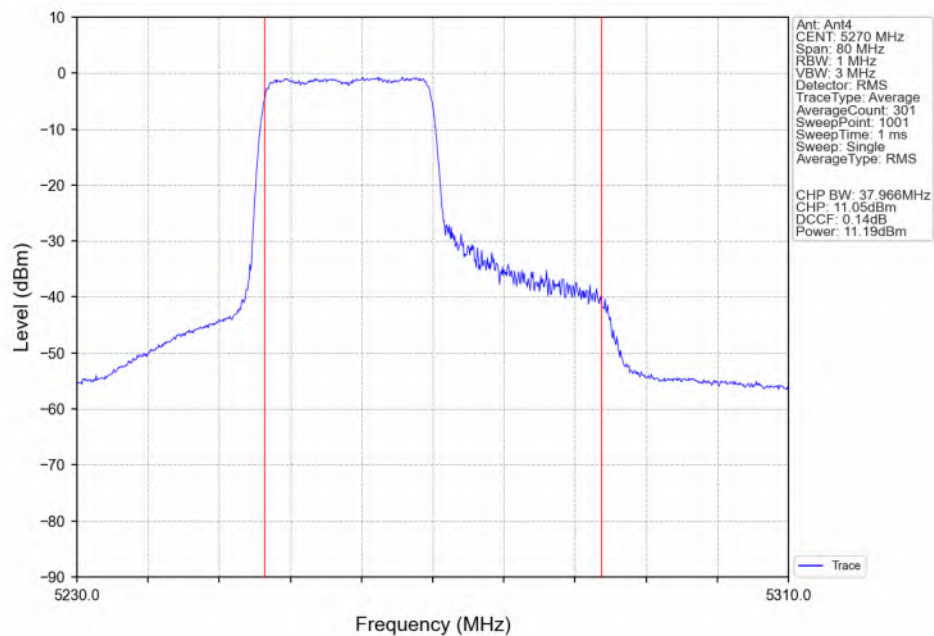
802.11be(EHT40) LCH_5270MHz_RU242_Left(61)_Ant4_NTNV
