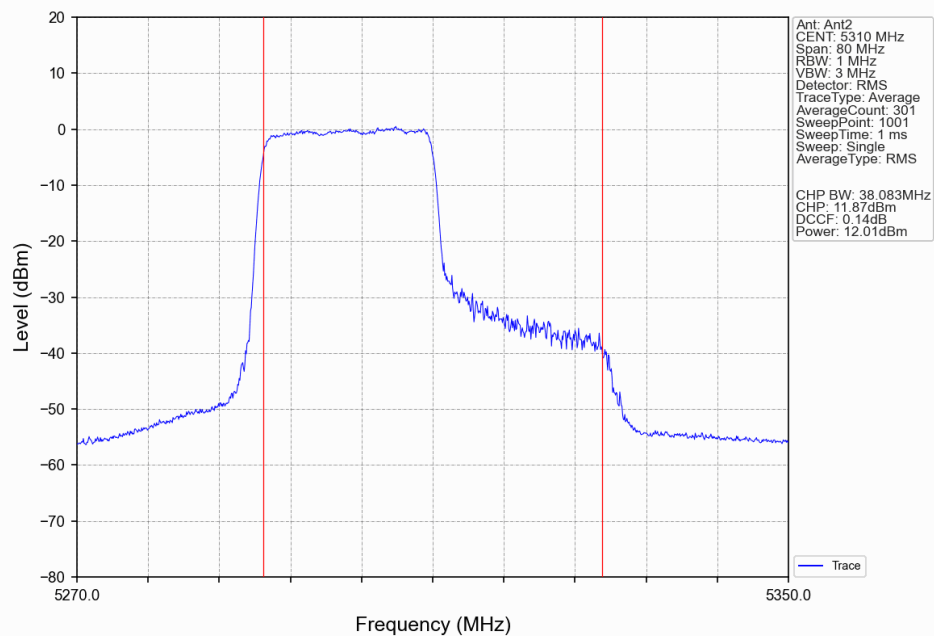
802.11be(EHT40)_HCH_5310MHz_RU242_Left(61)_Ant2_NTNV
