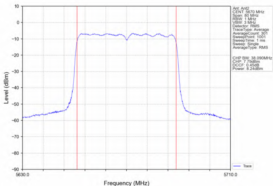
802.11be(EHT40)_HCH_5670MHz_RU484_Left(65)_Ant2_NTNV
