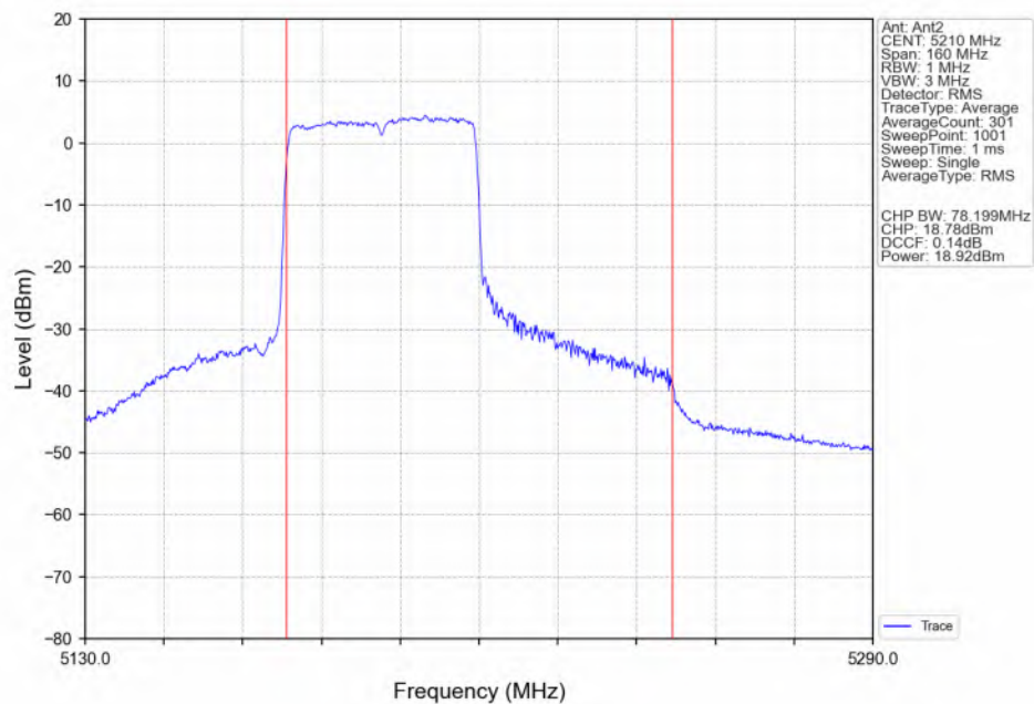
802.11be(EHT80)_MCH_5210MHz_RU484_Left(65)_Ant2_NTNV
