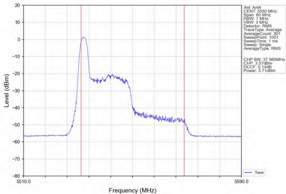
802.11be(EHT40)_MCH_5550MHz_RU26_Left(0)_Ant4_NTNV
