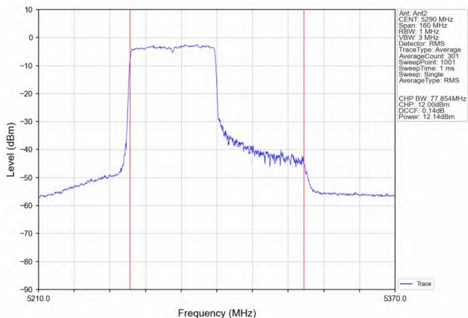
802.11be(EHT80)_MCH_5290MHz_RU484_Left(65)_Ant2_NTNV
