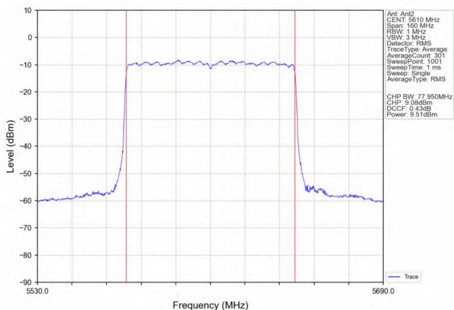
802.11be(EHT80)_HCH_5610MHz_RU996_Left(67)_Ant2_NTNV
