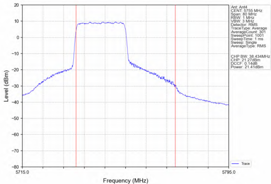
802.11be(EHT40) LCH_5755MHz_RU242_Left(61)_Ant4_NTNV
