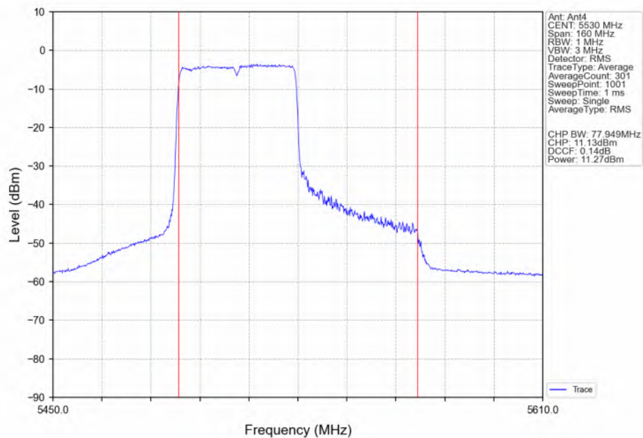
802.11be(EHT80) LCH_5530MHz_RU484_Left(65)_Ant4_NTNV
