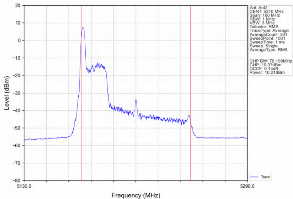
802.11be(EHT80)_MCH_5210MHz_RU26_Left(0)_Ant2_NTNV
