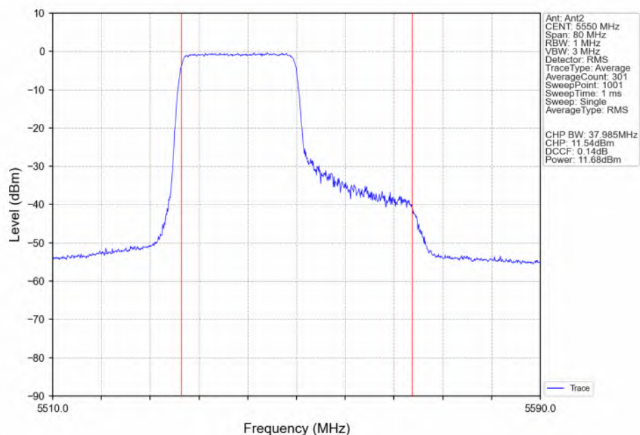
802.11be(EHT40)_MCH_5550MHz_RU242_Left(61)_Ant2_NTNV
