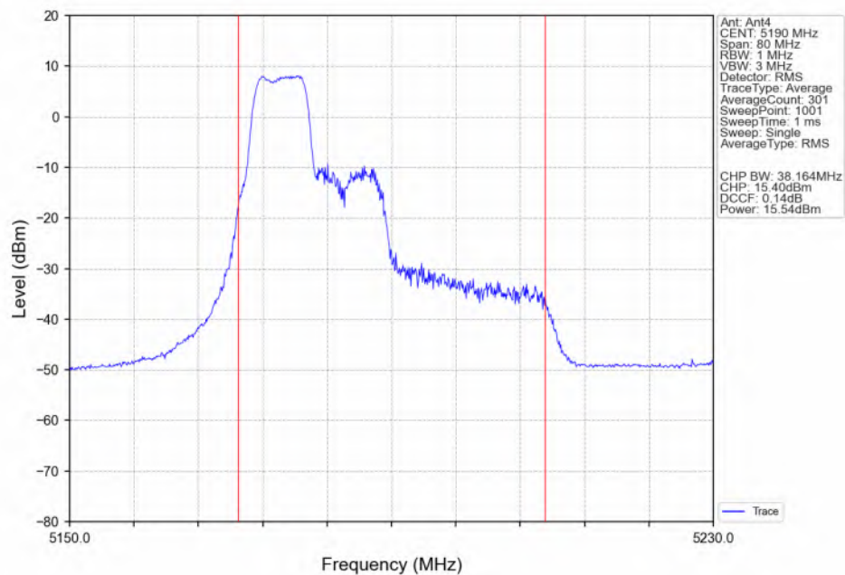
802.11be(EHT40)_LCH_5190MHz_26+52_ / Ant4_NTNV
