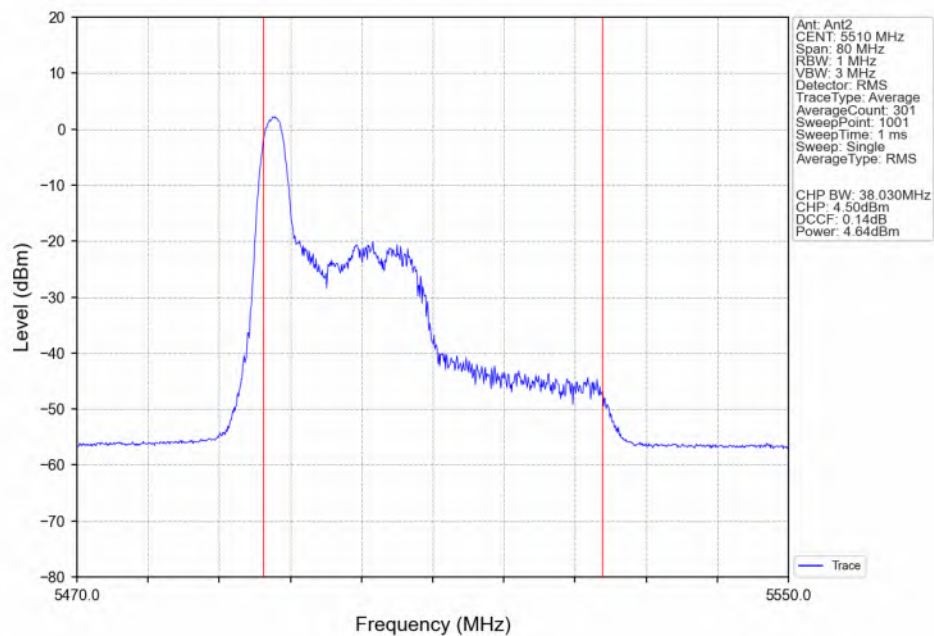
802.11be(EHT40) LCH_5510MHz_RU26_Left(0)_Ant2_NTNV
