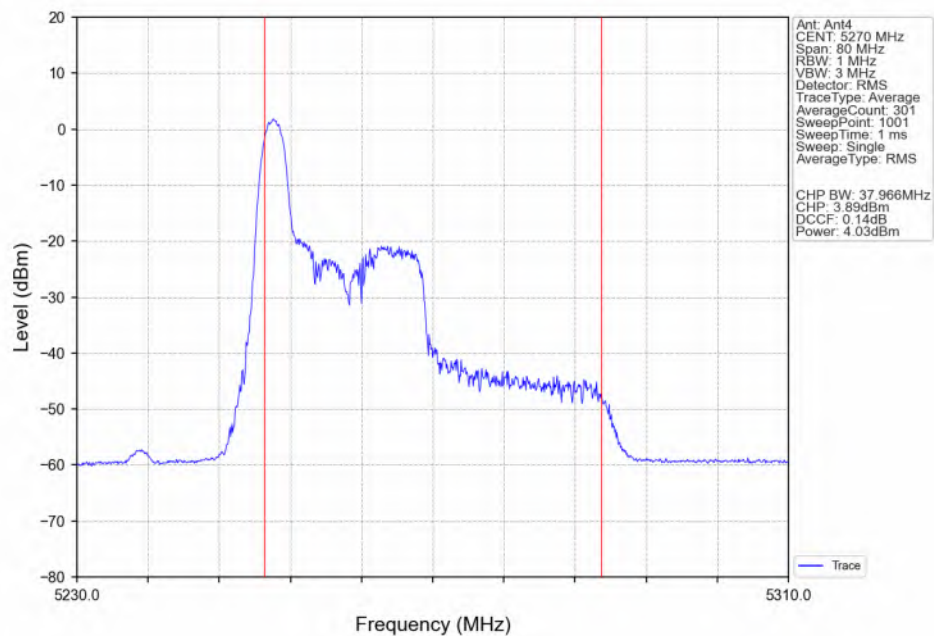
802.11be(EHT40) LCH_5270MHz_RU26_Left(0)_Ant4_NTNV
