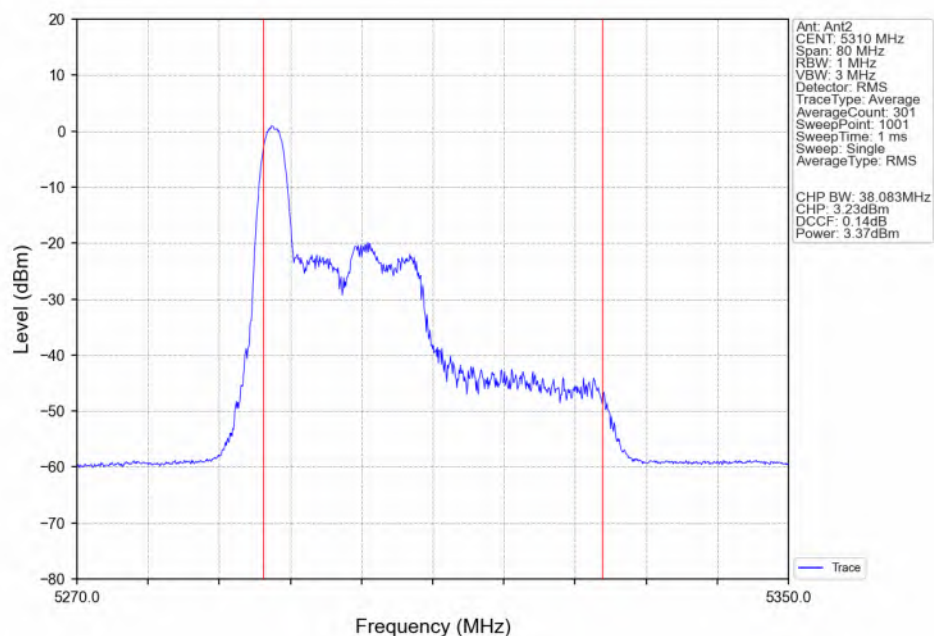
802.11be(EHT40)_HCH_5310MHz_RU26_Left(0)_Ant2_NTNV
