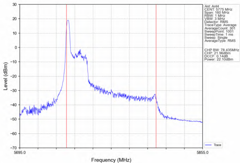
802.11be(EHT80)_MCH_5775MHz_RU26_Left(0)_Ant4_NTNV
