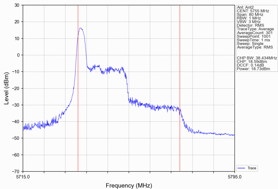
802.11be(EHT40) LCH_5755MHz_RU26_Left(0)_Ant2_NTNV
