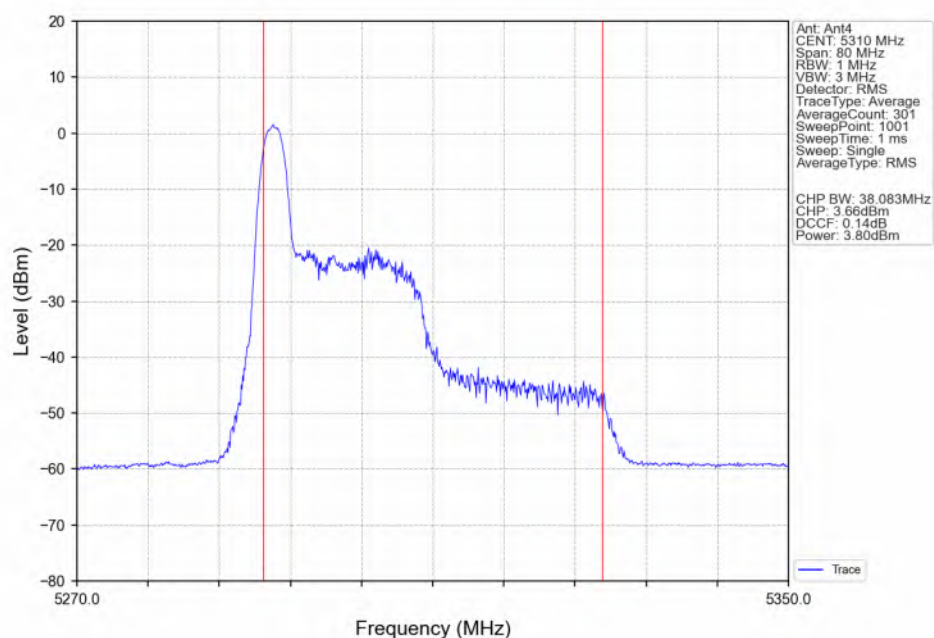
802.11be(EHT40)_HCH_5310MHz_RU26_Left(0)_Ant4_NTNV
