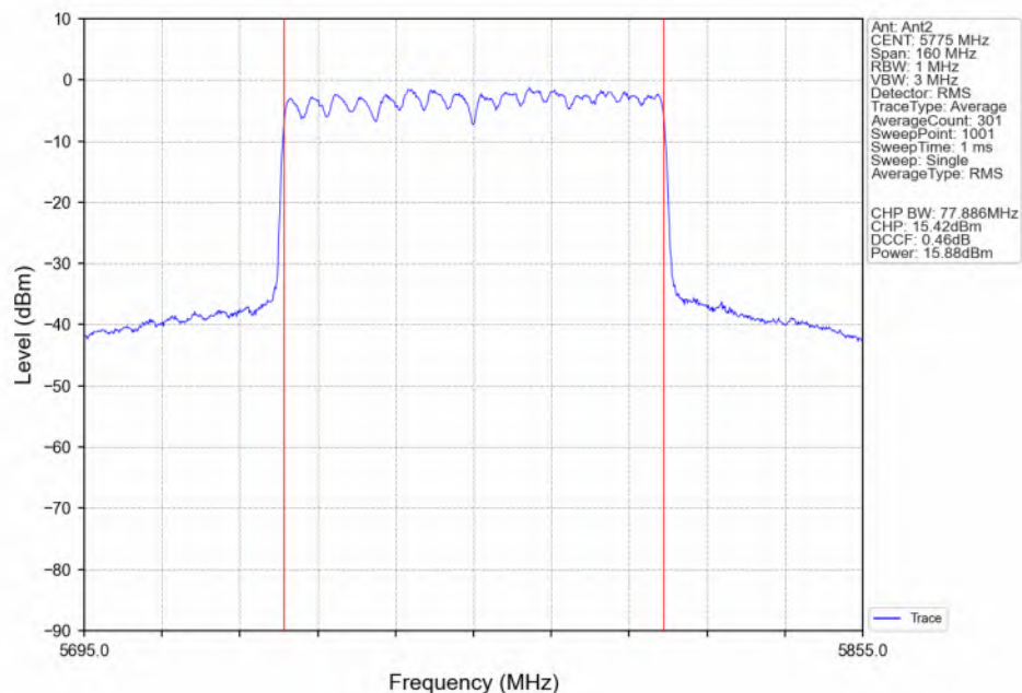
802.11be(EHT80)_MCH_5775MHz_RU996_Left(67)_Ant2_NTNV
