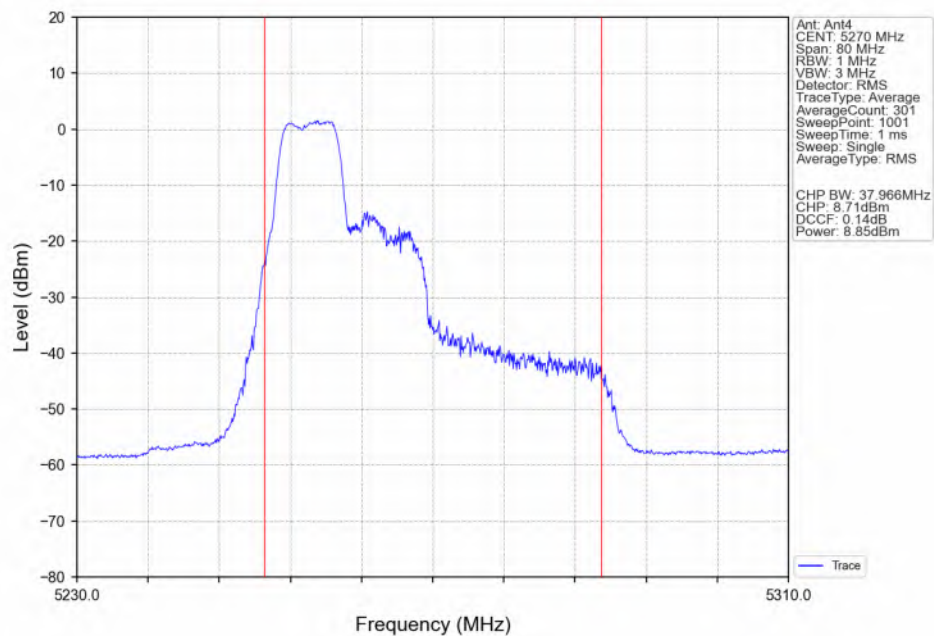
802.11be(EHT40)_LCH_5270MHz_26+52_ / Ant4_NTNV
