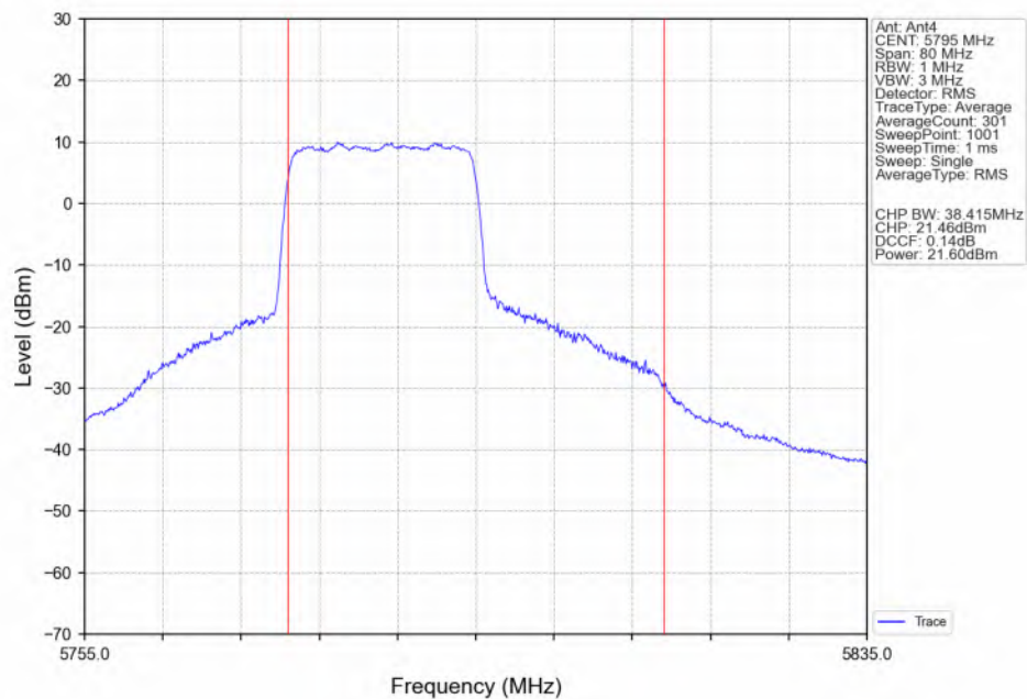
802.11be(EHT40)_HCH_5795MHz_RU242_Left(61)_Ant4_NTNV
