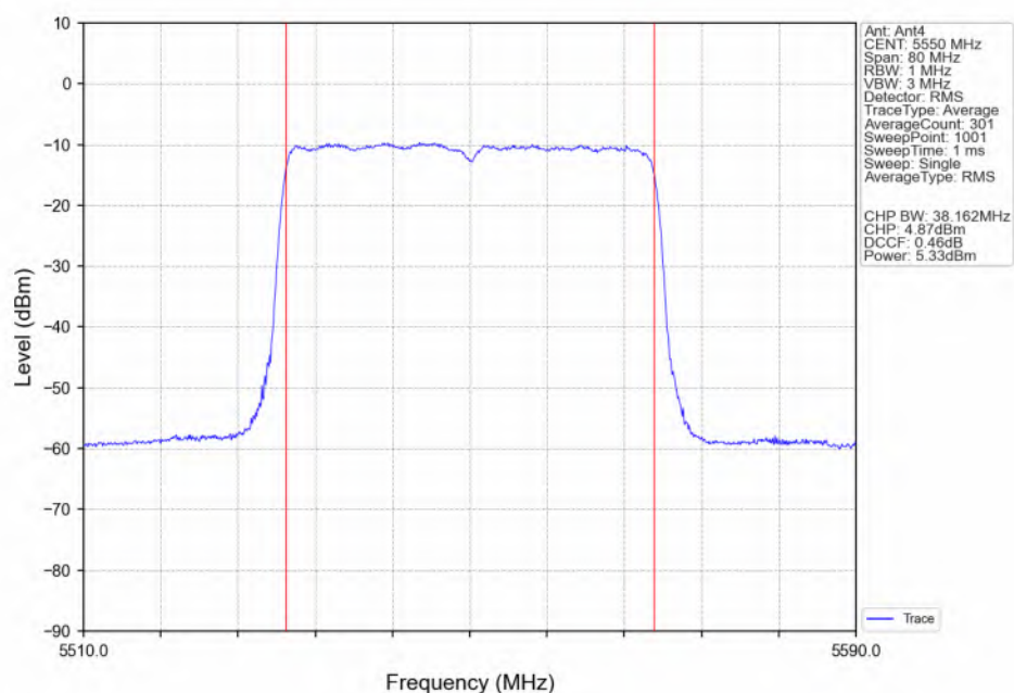
802.11be(EHT40)_MCH_5550MHz_RU484_Left(65)_Ant4_NTNV
