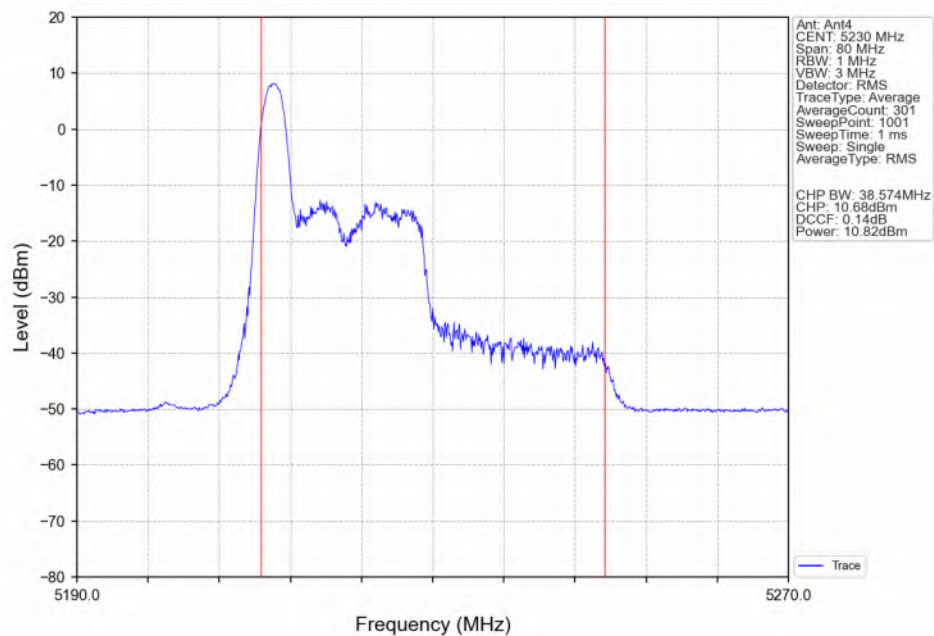
802.11be(EHT40)_HCH_5230MHz_RU26_Left(0)_Ant4_NTNV
