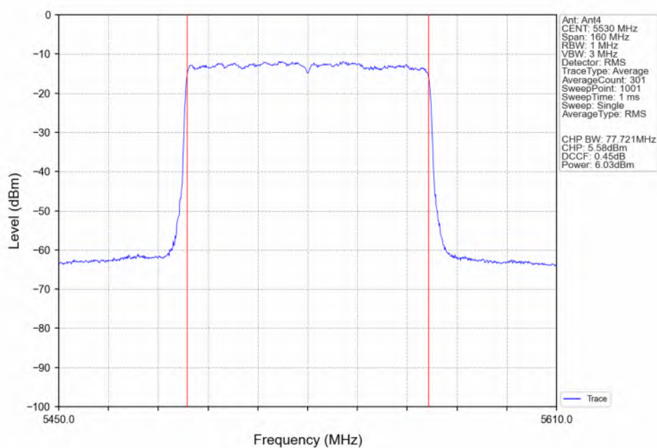
802.11be(EHT80) LCH_5530MHz_RU996_Left(67)_Ant4_NTNV
