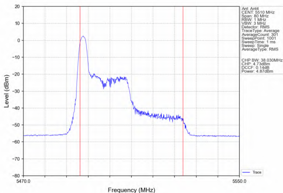
802.11be(EHT40) LCH_5510MHz_RU26_Left(0)_Ant4_NTNV
