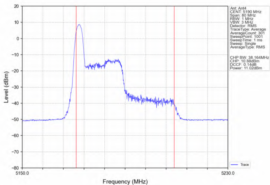
802.11be(EHT40) LCH_5190MHz_RU26_Left(0)_Ant4_NTNV
