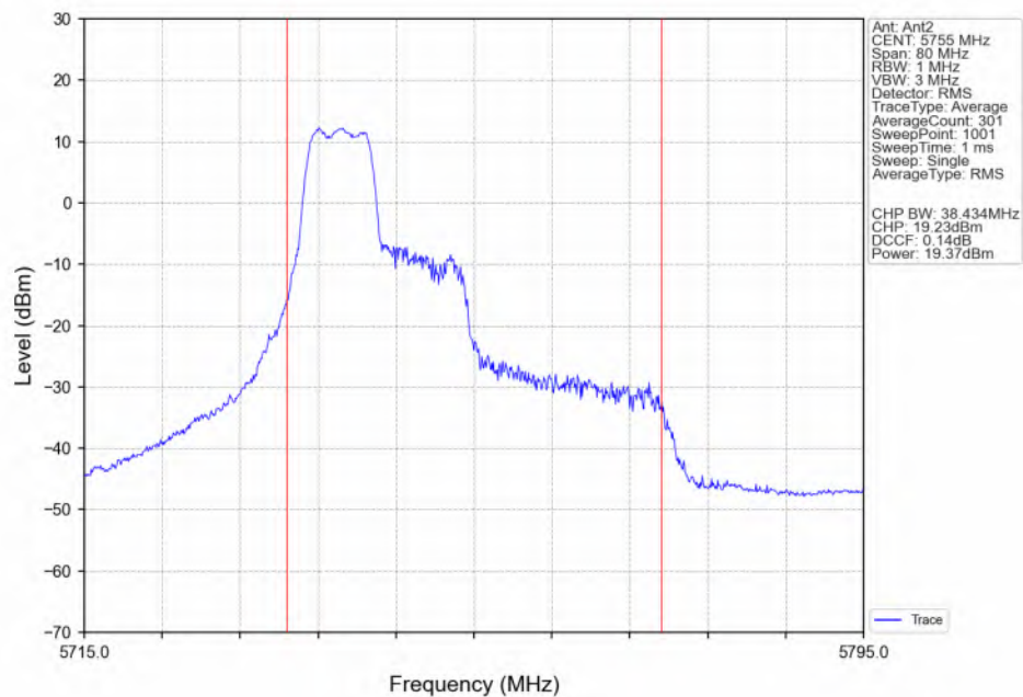
802.11be(EHT40)_LCH_5755MHz_26+52_ / Ant2_NTNV
