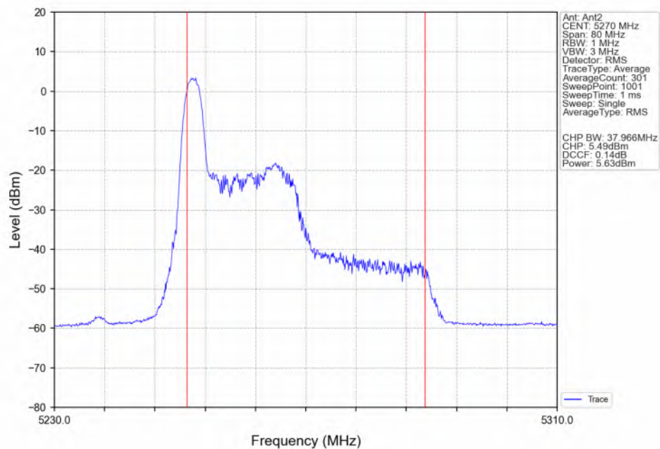
802.11be(EHT40) LCH_5270MHz_RU26_Left(0)_Ant2_NTNV
