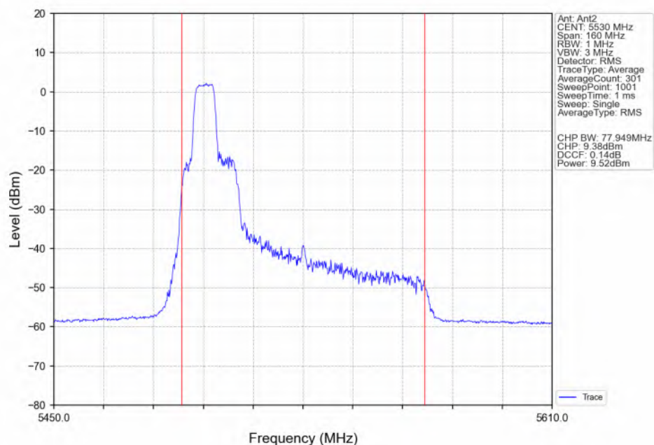
802.11be(EHT80)_LCH_5530MHz_26+52_ / Ant2_NTNV
