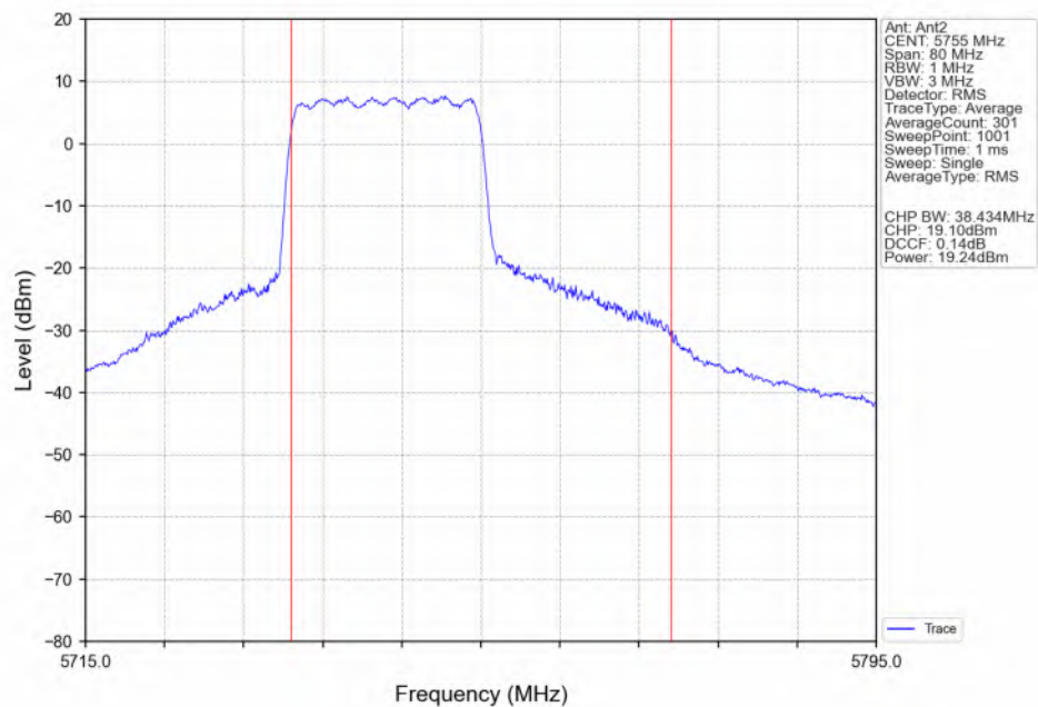
802.11be(EHT40) LCH_5755MHz_RU242_Left(61)_Ant2_NTNV
