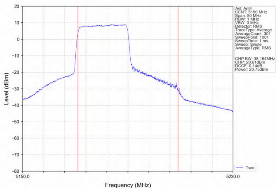
802.11be(EHT40) LCH_5190MHz_RU242_Left(61)_Ant4_NTNV
