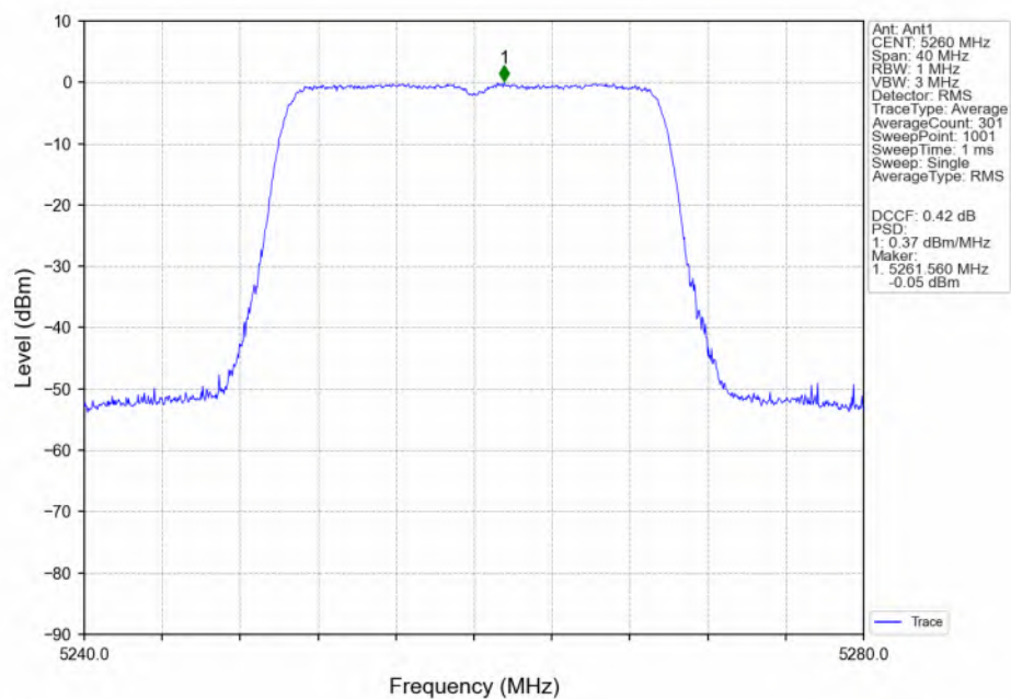
802.11ax(HEW20)_LCH_5260MHz_RU242_Left(61)_Ant1_NTNV
