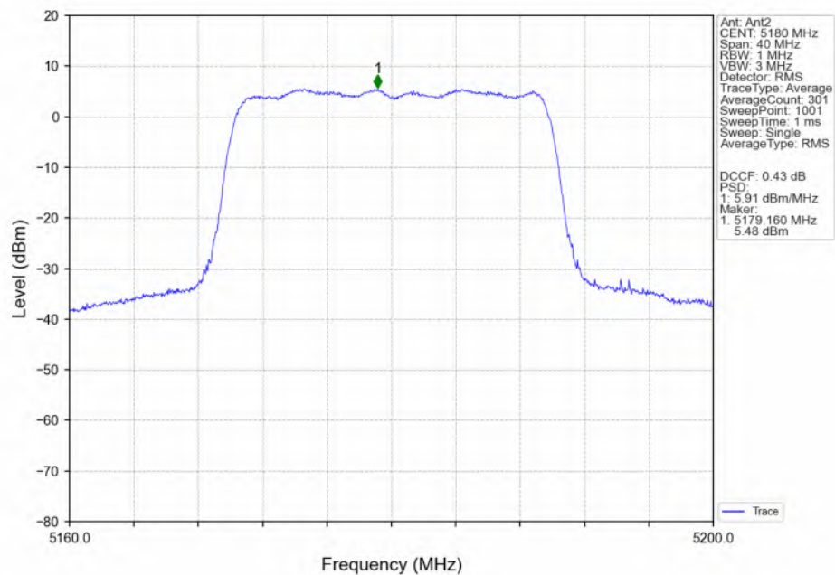
802.11ax(HEW20)_LCH_5180MHz_RU242_Left(61)_Ant2_NTNV
