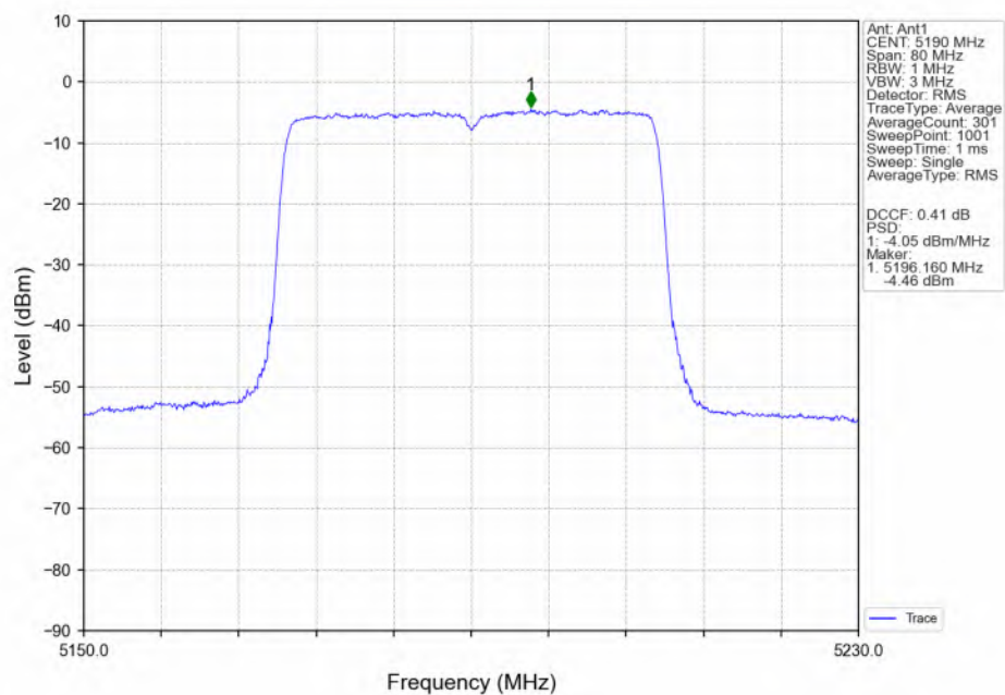
802.11ax(HEW40)_LCH_5190MHz_RU484_Left(65)_Ant1_NTNV
