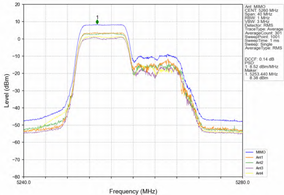
802.11ax(HEW20)_LCH_5260MHz_RU242_Left(61)_Ant1_NTNV
