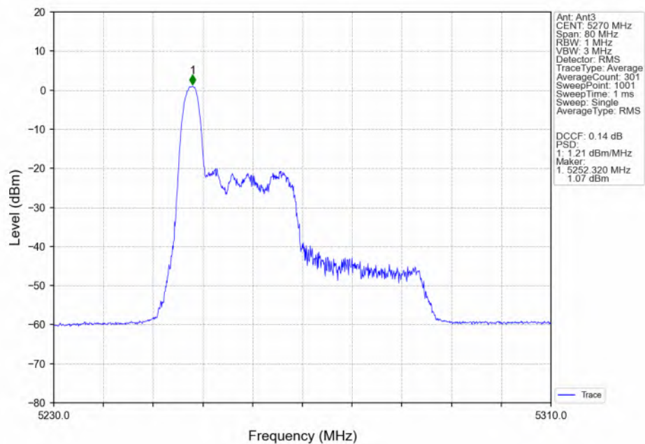
802.11ax(HEW40)_LCH_5270MHz_RU26_Left(0)_Ant3_NTNV
