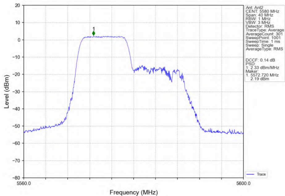
802.11ax(HEW20) MCH_5580MHz_RU106_Left(53)_Ant2_NTNV
