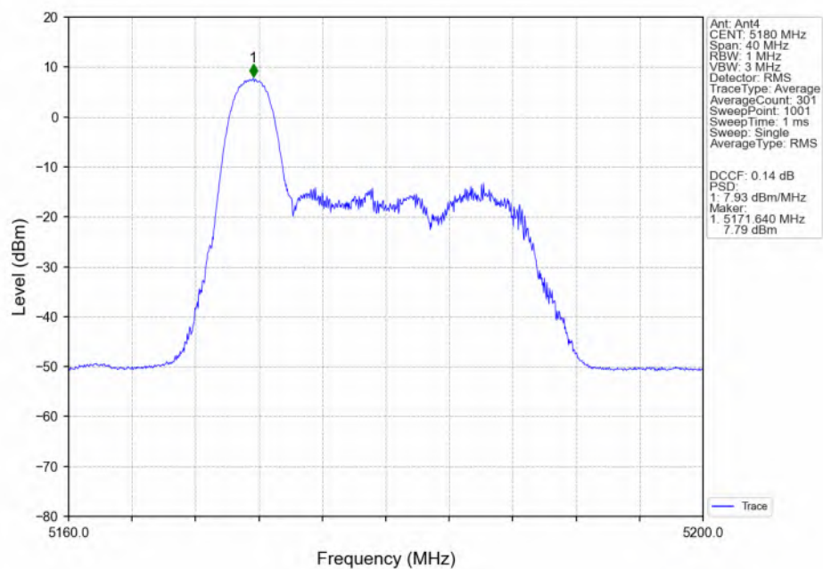
802.11ax(HEW20)_LCH_5180MHz_RU26_Left(0)_Ant4_NTNV
