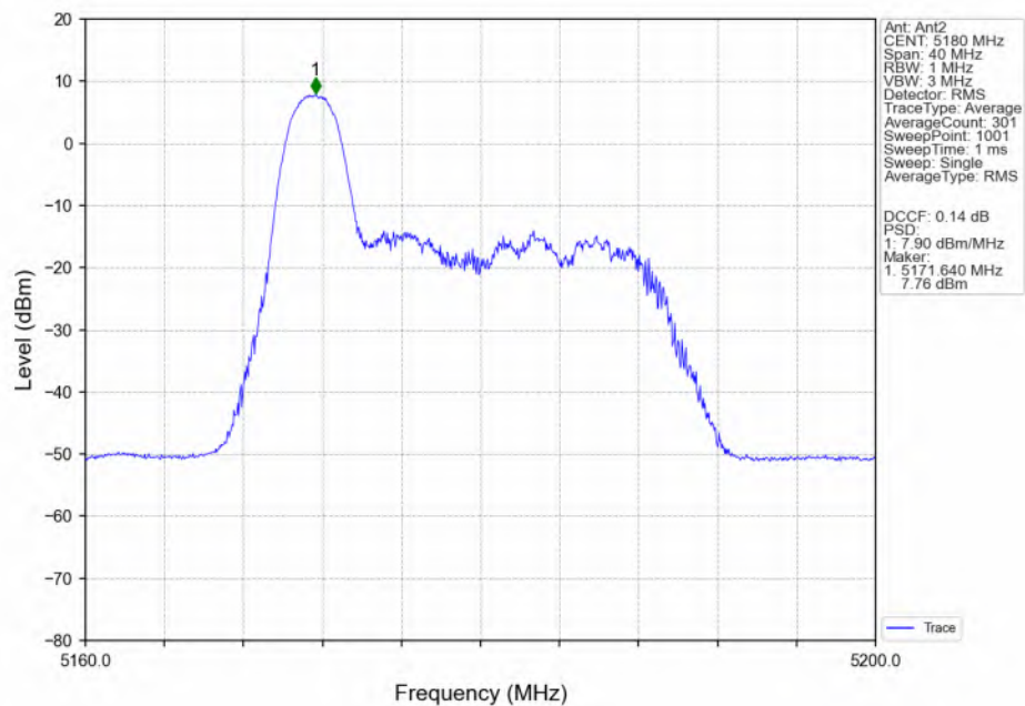
802.11ax(HEW20)_LCH_5180MHz_RU26_Left(0)_Ant2_NTNV
