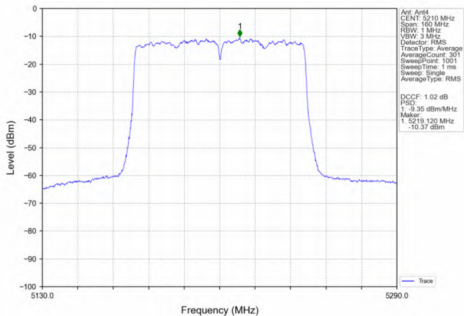
802.11ac(VHT80)_MCH_5210MHz_Ant4_NTNV
