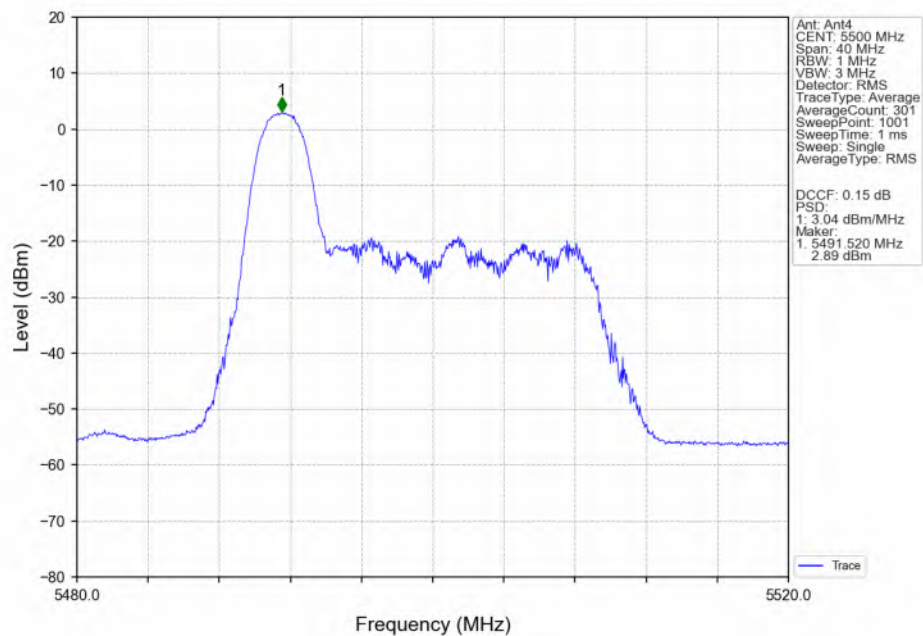
802.11ax(HEW20)_LCH_5500MHz_RU26_Left(0)_Ant4_NTNV
