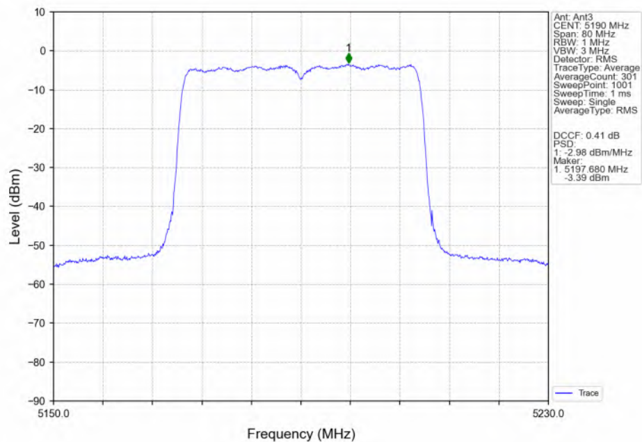
802.11ax(HEW40)_LCH_5190MHz_RU484_Left(65)_Ant3_NTNV
