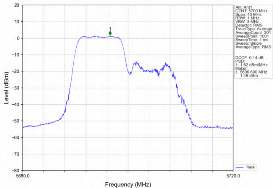
802.11ax(HEW20)_HCH_5700MHz_RU106_Left(53)_Ant1_NTNV
