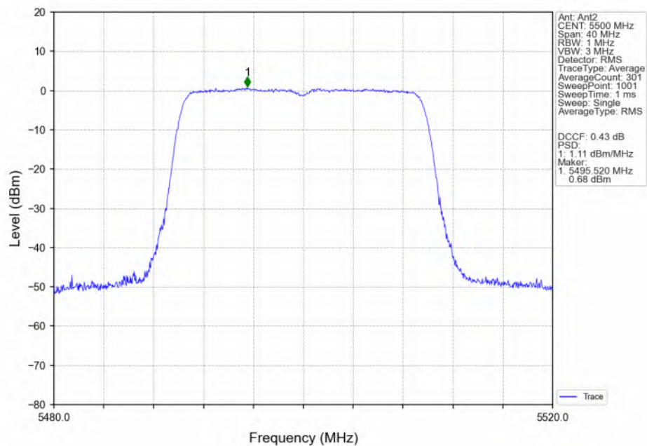
802.11ax(HEW20)_LCH_5500MHz_RU242_Left(61)_Ant2_NTNV
