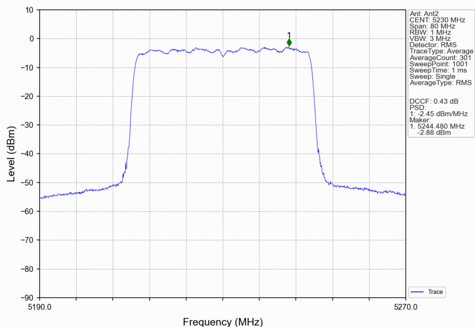
802.11ax(HEW40)_HCH_5230MHz_RU484_Left(65)_Ant2_NTNV
