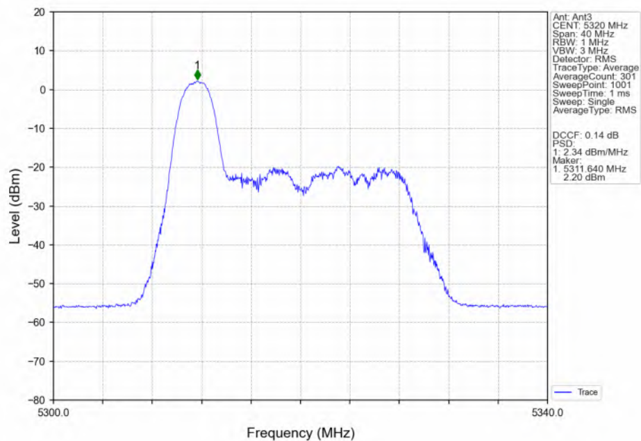
802.11ax(HEW20) HCH_5320MHz_RU26_Left(0)_Ant3_NTNV
