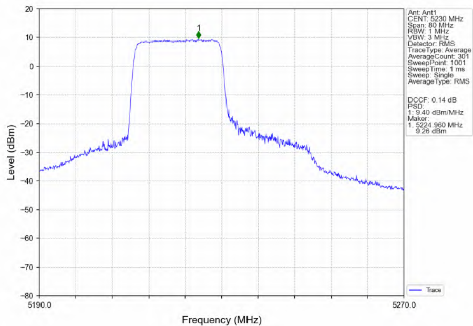
802.11ax(HEW40)_HCH_5230MHz_RU242_Left(61)_Ant1_NTNV
