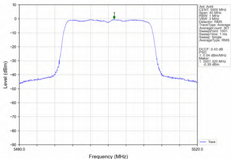
802.11ax(HEW20)_LCH_5500MHz_RU242_Left(61)_Ant4_NTNV
