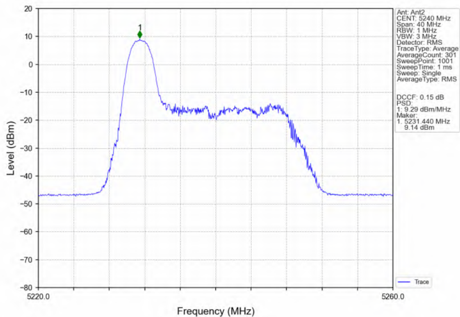
802.11ax(HEW20) HCH_5240MHz_RU26_Left(0)_Ant2_NTNV
