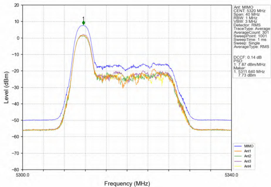
802.11ax(HEW20) HCH_5320MHz_RU26_Left(0)_MIMO_NTNV
