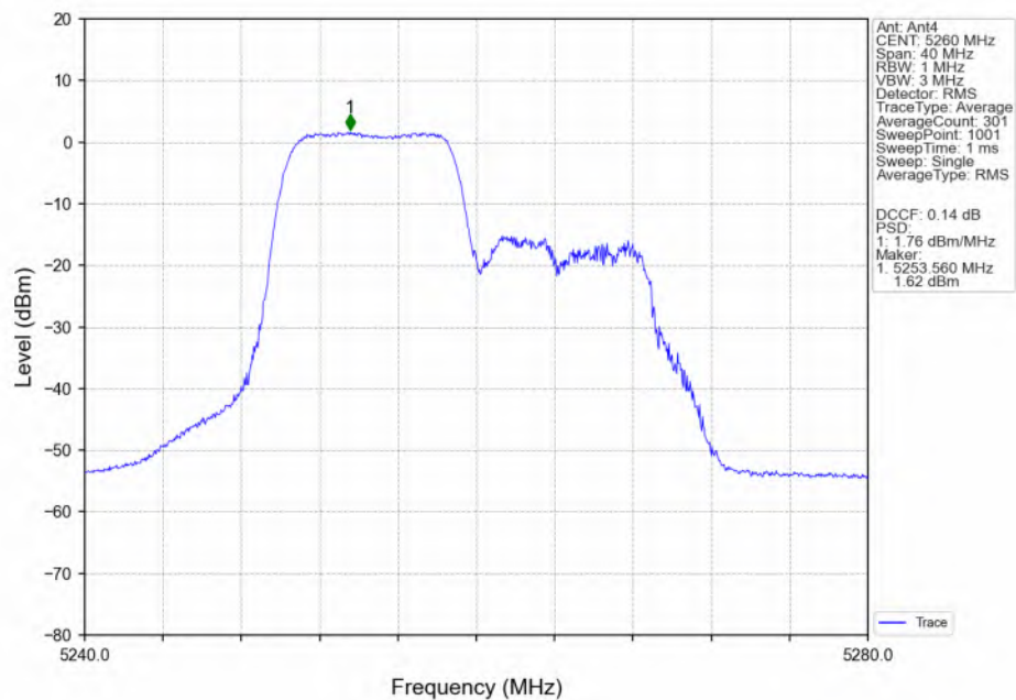
802.11ax(HEW20)_LCH_5260MHz_RU106_Left(53)_Ant4_NTNV
