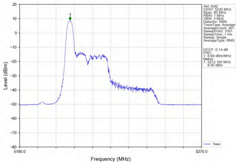
802.11ax(HEW40) HCH_5230MHz_RU26_Left(0)_Ant2_NTNV
