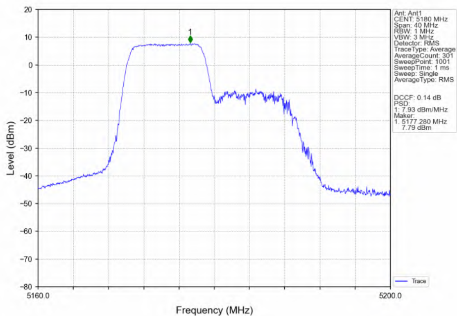
802.11ax(HEW20)_LCH_5180MHz_RU106_Left(53)_Ant1_NTNV
