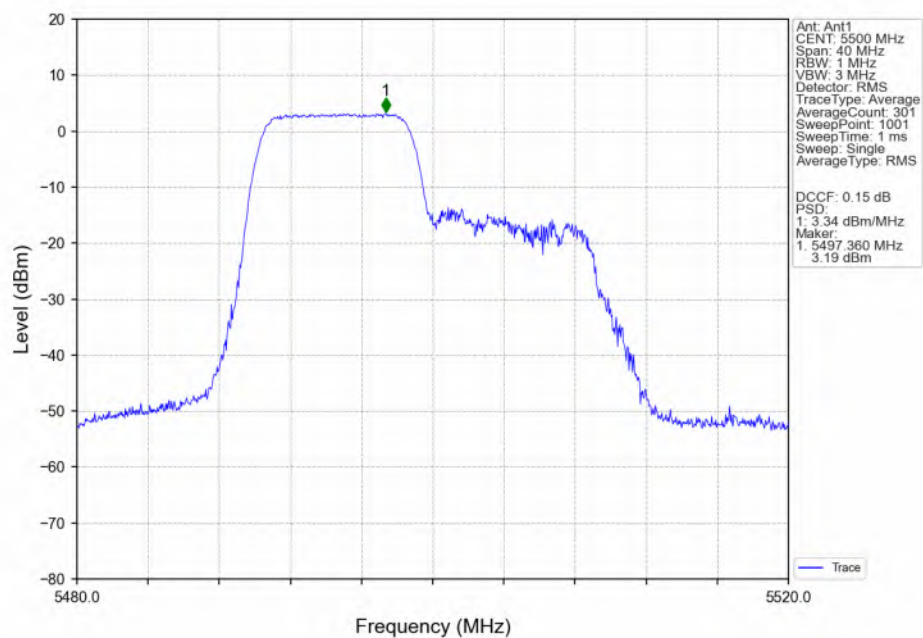
802.11ax(HEW20)_LCH_5500MHz_RU106_Left(53)_Ant1_NTNV
