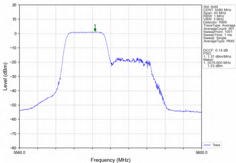
802.11ax(HEW20) MCH_5580MHz_RU106_Left(53)_Ant4_NTNV
