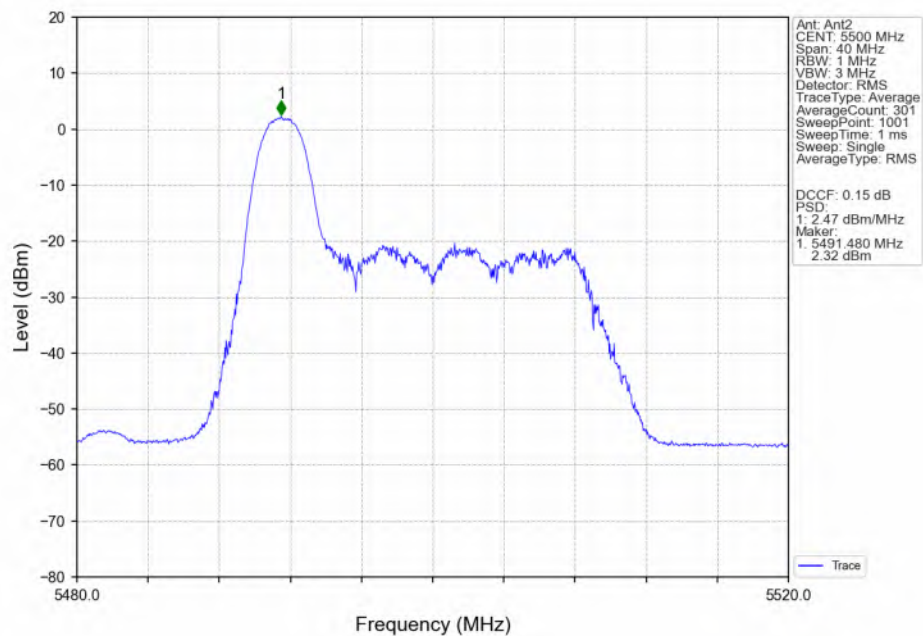
802.11ax(HEW20)_LCH_5500MHz_RU26_Left(0)_Ant2_NTNV
