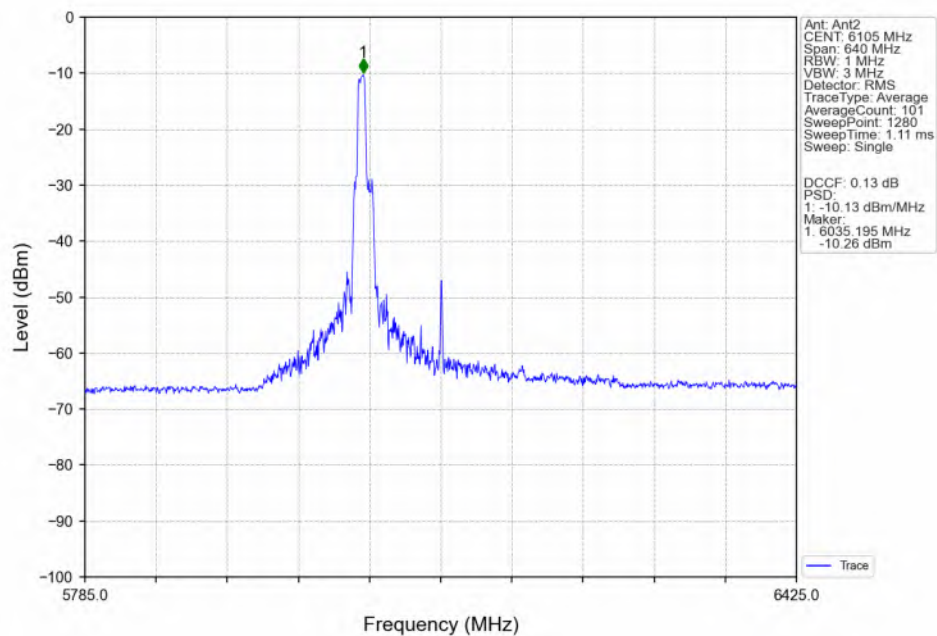
802.11be(EHT320) LCH_6105MHz_26+52 / Ant2_NTNV
