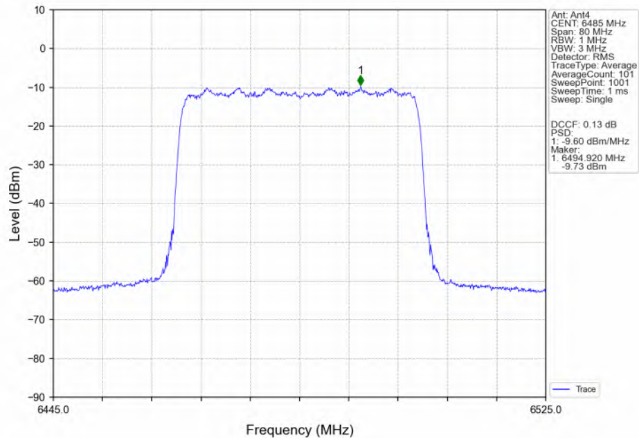
802.11be(EHT40)_MCH_6485MHz_RU484_Left(65)_MIMO_NTNV
