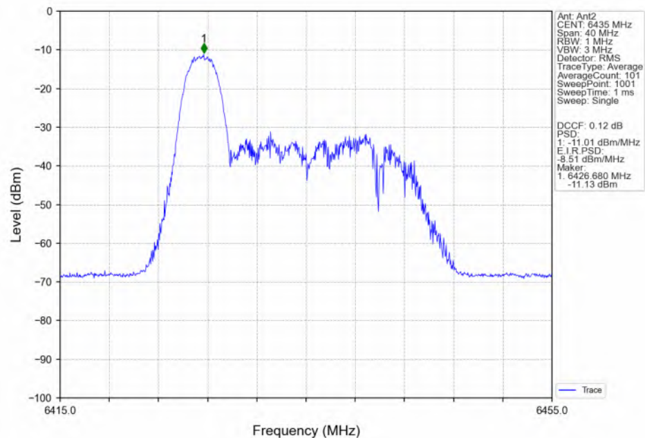
802.11be(EHT20)_LCH_6435MHz_RU26_Left(0)_Ant2_NTNV
