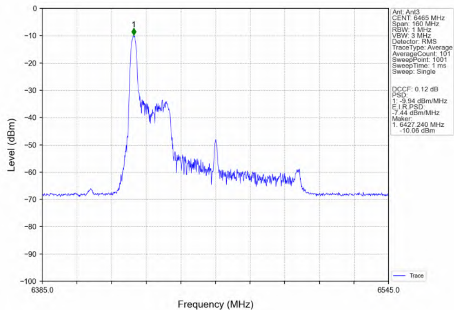
802.11be(EHT80) LCH_6465MHz_RU26_Left(0)_Ant3_NTNV
