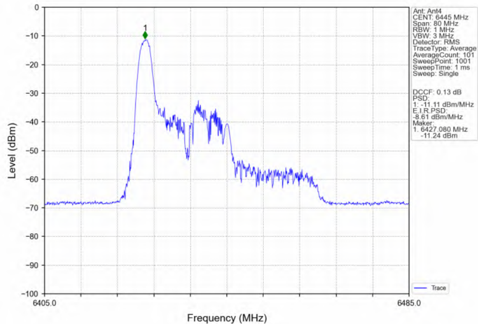
802.11be(EHT40) LCH 6445MHz RU26 Left(0) MIMO NTNV
