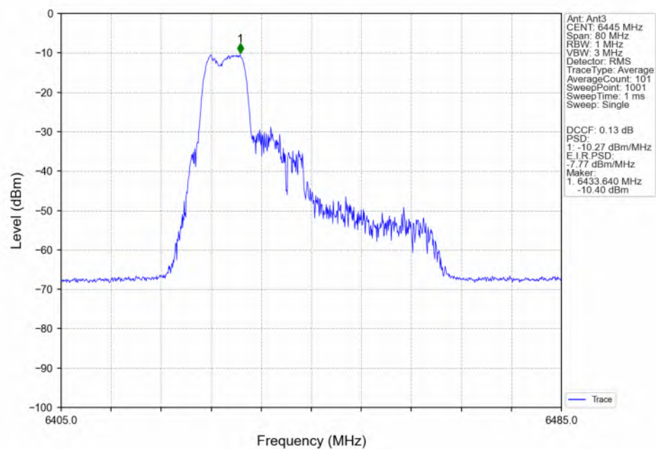
802.11be(EHT40)_LCH_6445MHz_26+52_ / Ant3_NTNV
