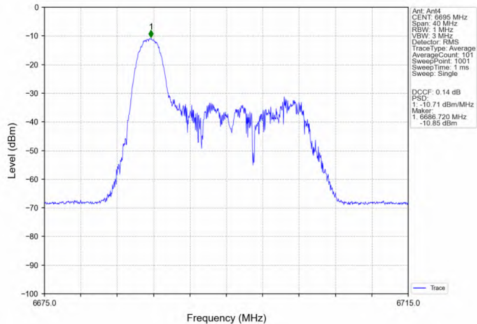
802.11be(EHT20)_MCH_6695MHz_RU26_Left(0)_MIMO_NTNV
