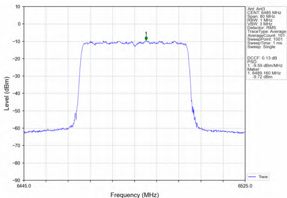
802.11be(EHT40)_MCH_6485MHz_RU484_Left(65)_Ant3_NTNV
