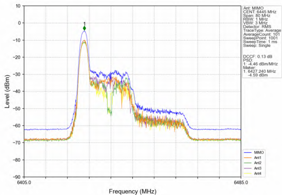
802.11be(EHT40) LCH 6445MHz RU26 Left(0) MIMO NTN
