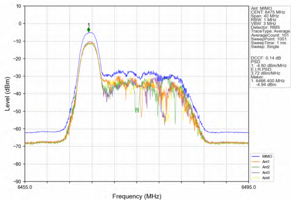
802.11be(EHT20)_MCH_6475MHz_RU26_Left(0)_MIMO_NTNV
