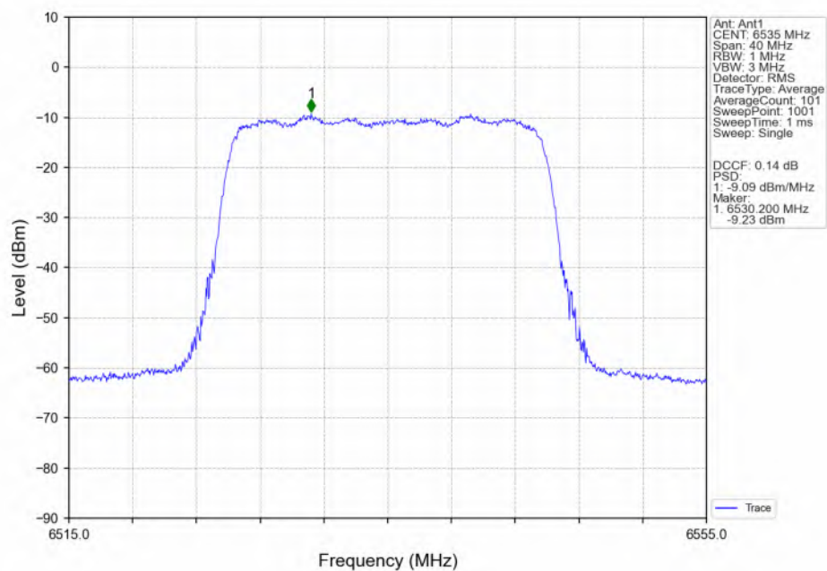
802.11be(EHT20) LCH_6535MHz_RU242_Left(61)_Ant1_NTNV
