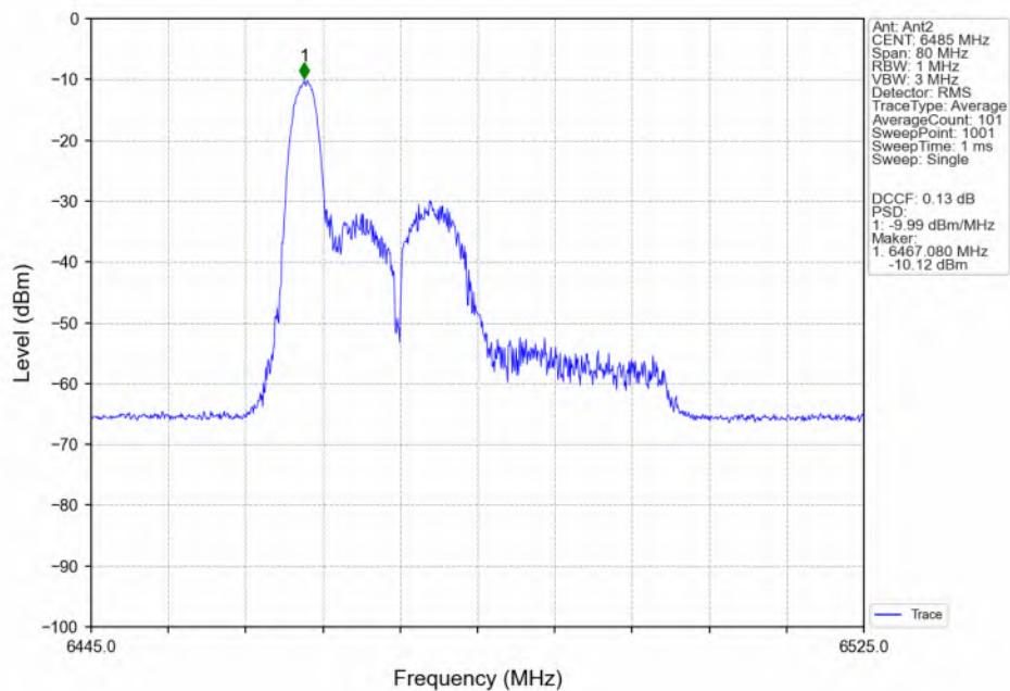
802.11be(EHT40)_MCH_6485MHz_RU26_Left(0)_Ant2_NTNV
