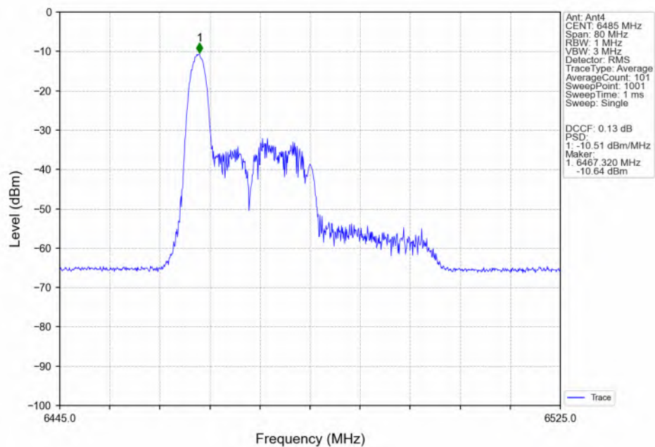
802.11be(EHT40)_MCH_6485MHz_RU26_Left(0)_Ant4_NTNV
