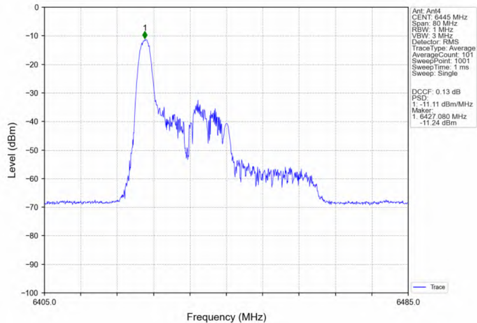
802.11be(EHT40) LCH 6445MHz RU26 Left(0) MIMO NTN
