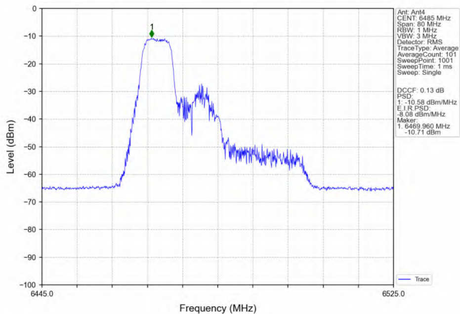
802.11be(EHT40)_MCH_6485MHz_26+52_/_Ant4_NTNV
