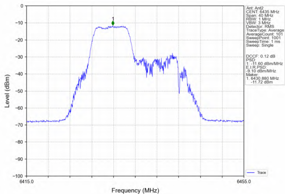
802.11be(EHT20)_LCH_6435MHz_26+52_ / Ant2_NTNV
