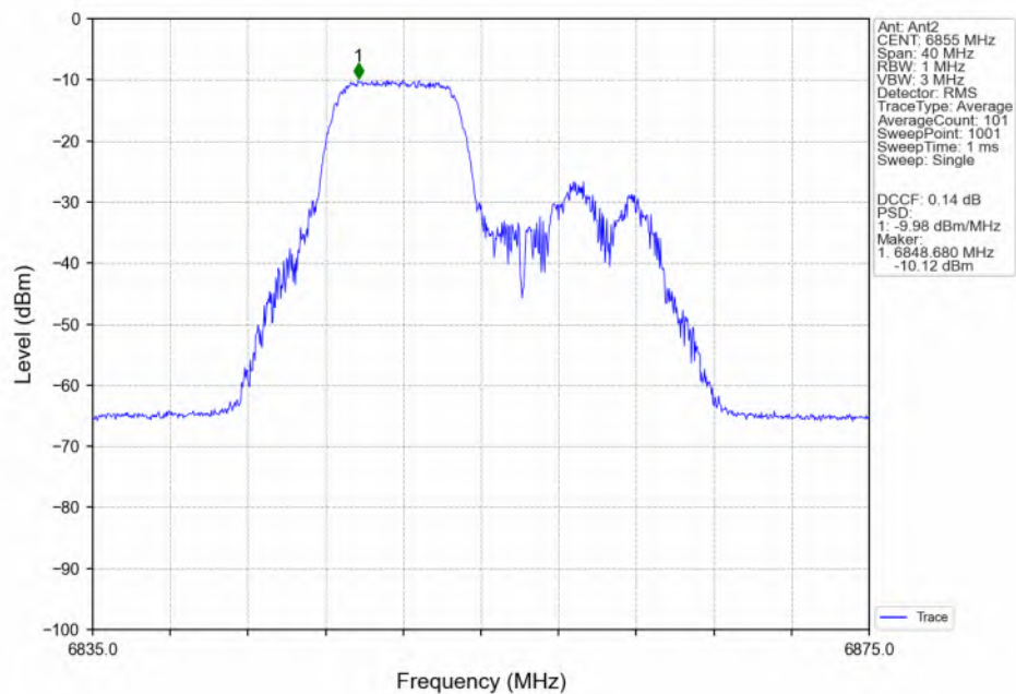
802.11be(EHT20)_HCH_6855MHz_26+52_ / Ant2_NTNV
