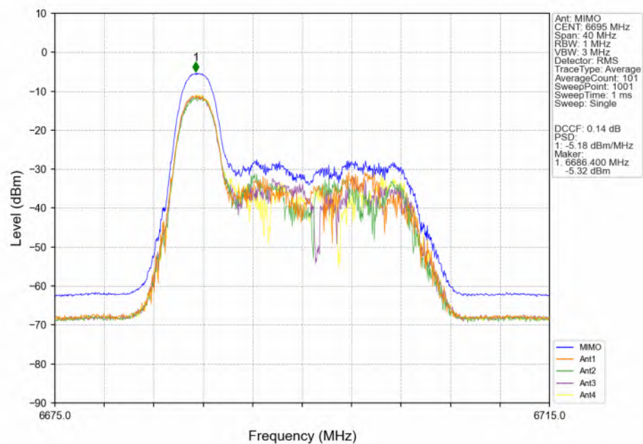
802.11be(EHT20)_MCH_6695MHz_RU26_Left(0)_MIMO_NTNV
