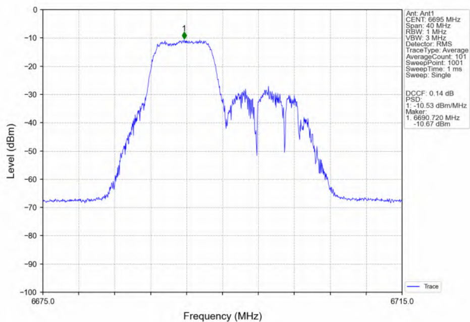
802.11be(EHT20)_MCH_6695MHz_26+52_/_Ant1_NTNV
