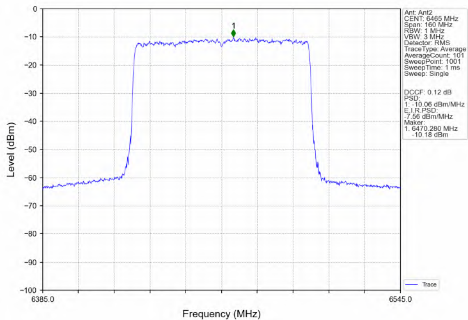
802.11be(EHT80) LCH_6465MHz_RU996_Left(67)_Ant2_NTNV
