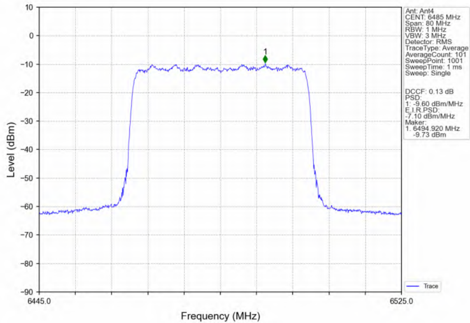
802.11be(EHT40)_MCH_6485MHz_RU484_Left(65)_MIMO_NTNV
