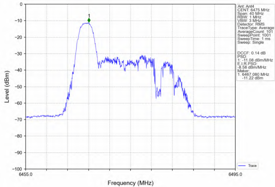
802.11be(EHT20)_MCH_6475MHz_RU26_Left(0)_MIMO_NTNV
