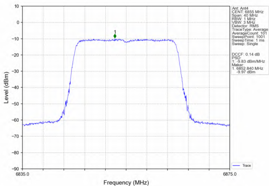
802.11be(EHT20)_HCH_6855MHz_RU242_Left(61)_MIMO_NTNV
