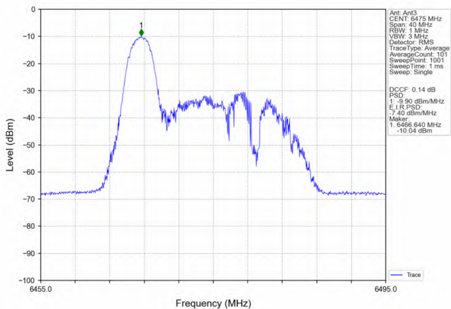
802.11be(EHT20)_MCH_6475MHz_RU26_Left(0)_Ant3_NTNV
