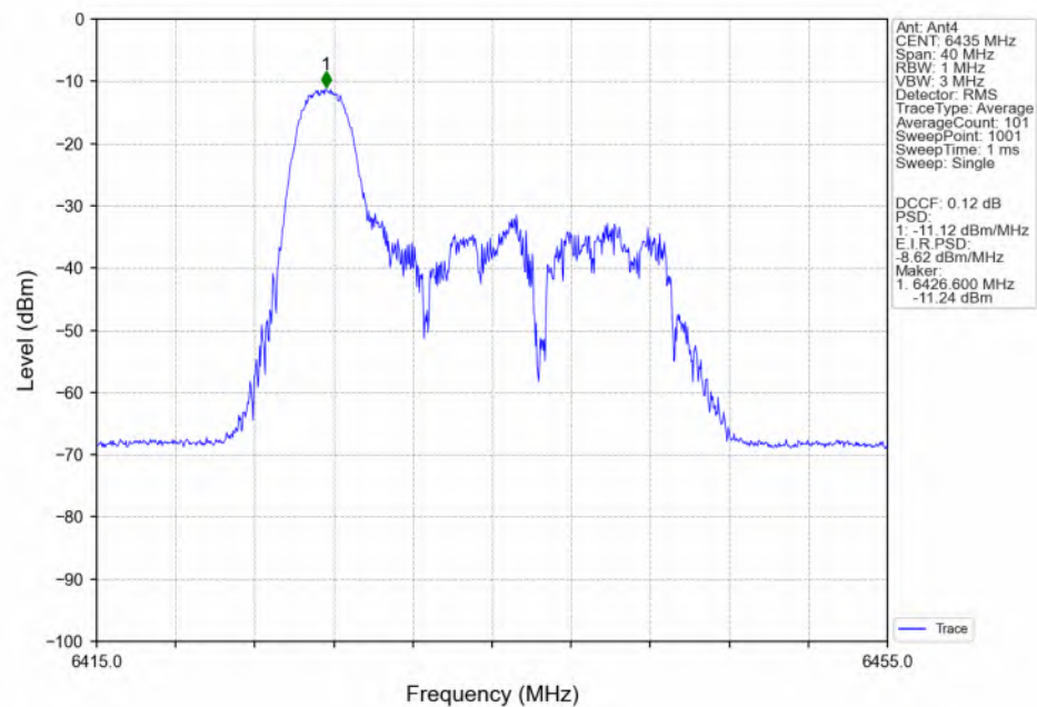
802.11be(EHT20) LCH_6435MHz_RU26_Left(0)_Ant4_NTNV
