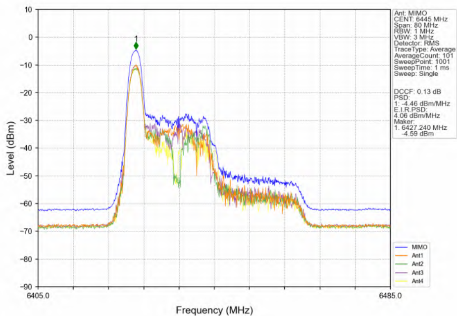
802.11be(EHT40) LCH 6445MHz RU26 Left(0) MIMO NTNV
