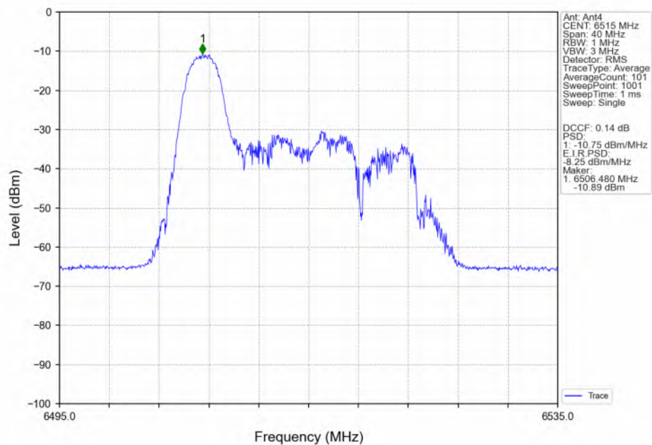
802.11be(EHT20)_HCH_6515MHz_RU26_Left(0)_Ant4_NTNV
