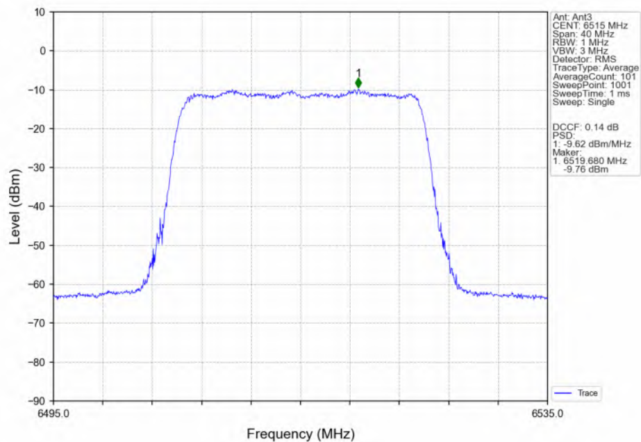
802.11be(EHT20)_HCH_6515MHz_RU242_Left(61)_Ant3_NTNV
