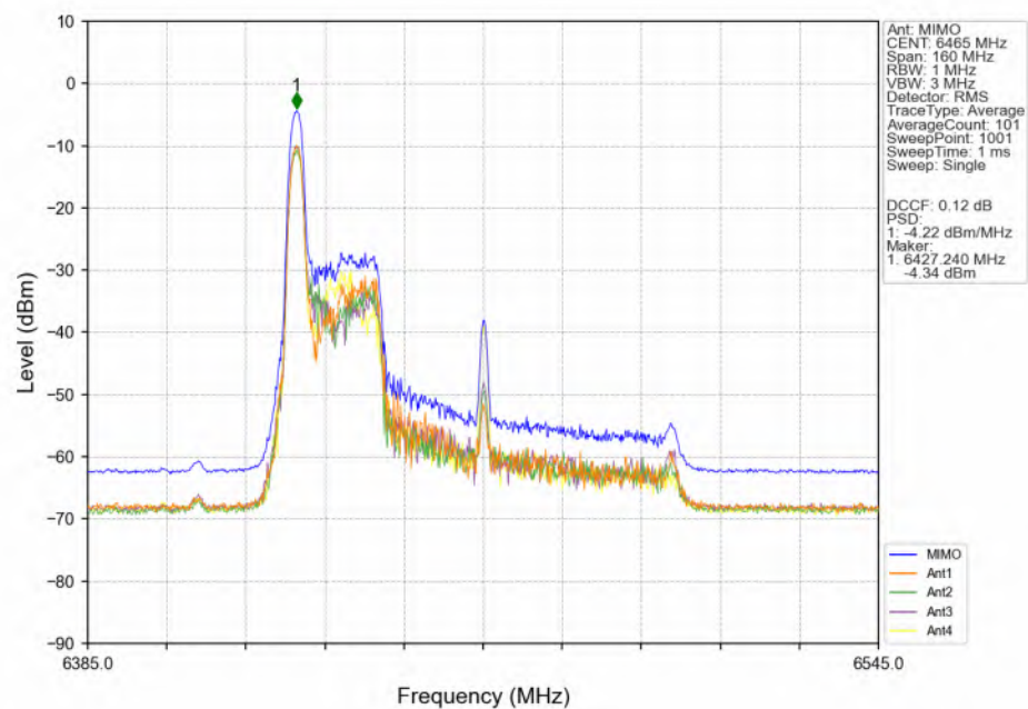
802.11be(EHT80) LCH_6465MHz_RU26_Left(0)_MIMO_NTNV
