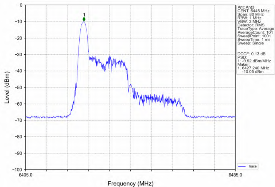
802.11be(EHT40) LCH_6445MHz_RU26_Left(0)_Ant3_NTNV
