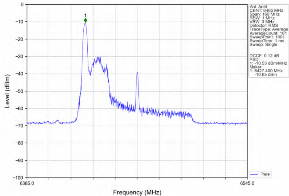
802.11be(EHT80) LCH_6465MHz_RU26_Left(0)_MIMO_NTNV
