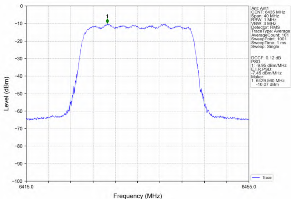
802.11be(EHT20) LCH_6435MHz_RU242_Left(61)_Ant1_NTNV
