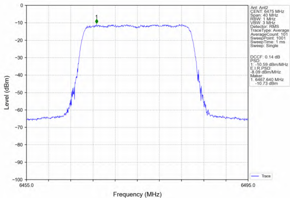
802.11be(EHT20)_MCH_6475MHz_RU242_Left(61)_Ant2_NTNV
