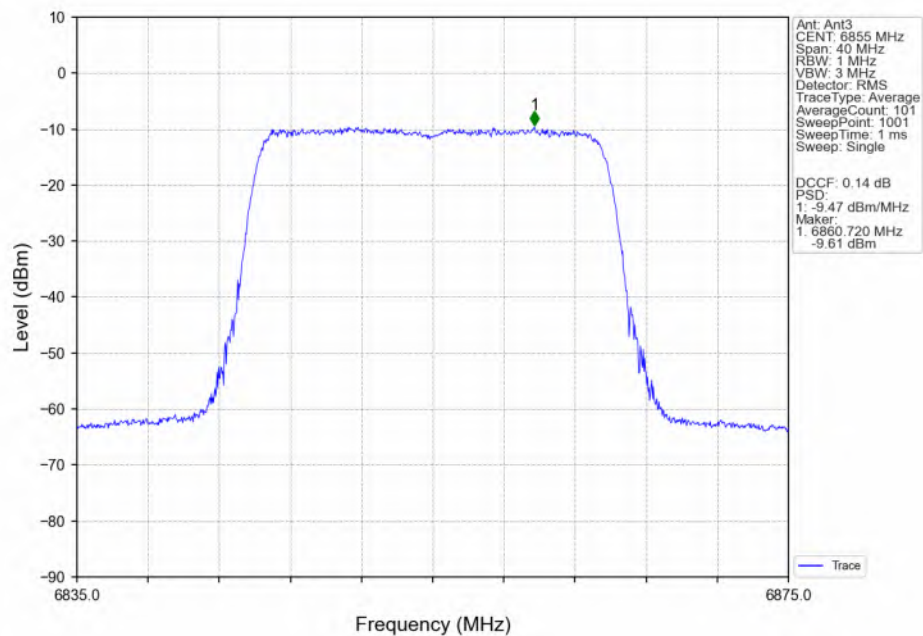
802.11be(EHT20)_HCH_6855MHz_RU242_Left(61)_Ant3_NTNV
