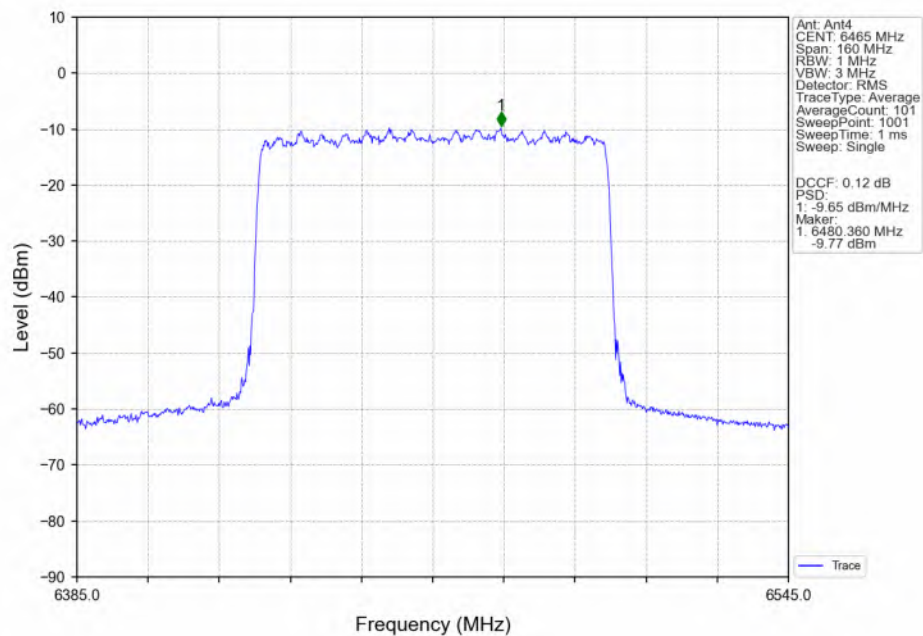
802.11be(EHT80) LCH_6465MHz_RU996_Left(67)_Ant4_NTNV
