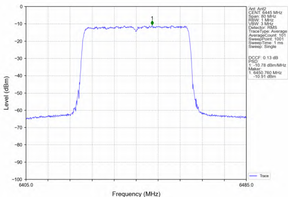
802.11be(EHT40) LCH_6445MHz_RU484_Left(65)_Ant2_NTNV
