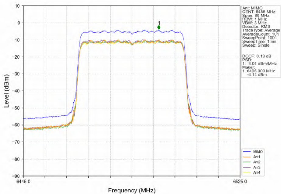
802.11be(EHT40)_MCH_6485MHz_RU484_Left(65)_MIMO_NTNV
