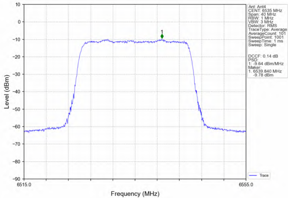
802.11be(EHT20)_LCH_6535MHz_RU242_Left(61)_MIMO_NTNV
