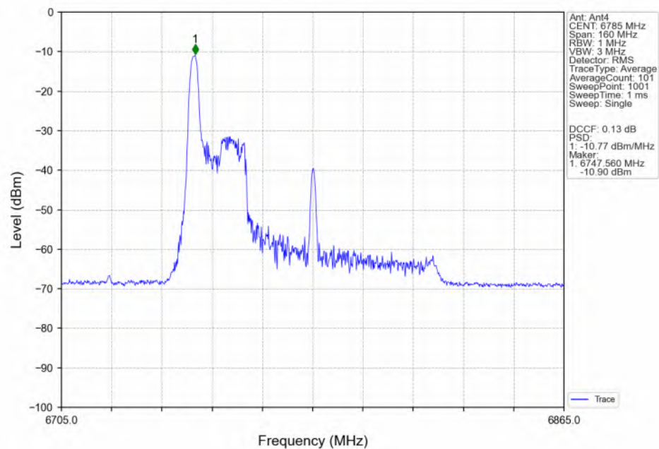
802.11be(EHT80)_HCH_6785MHz_RU26_Left(0)_Ant4_NTNV
