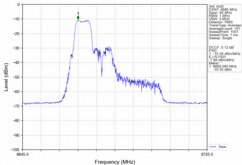
802.11be(EHT40) MCH 6685MHz 26+52 / Ant2_NTNV
