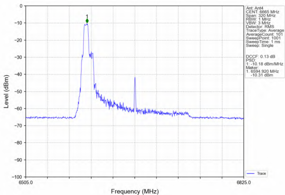
802.11be(EHT160)_MCH_6665MHz_26+52 / _Ant4_NTNV
