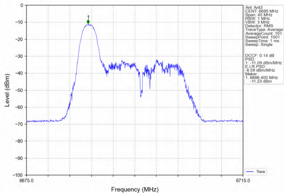
802.11be(EHT20)_MCH_6695MHz_RU26_Left(0)_Ant3_NTNV
