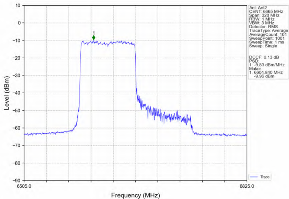
802.11be(EHT160)_MCH_6665MHz_RU996_Left(67)_Ant2_NTNV
