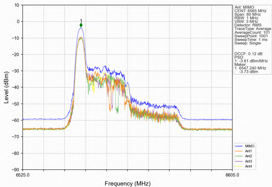
802.11be(EHT40) LCH_6565MHz_RU26_Left(0)_MIMO_NTNV
