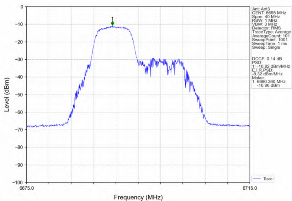
802.11be(EHT20)_MCH_6695MHz_26+52_ / Ant3_NTNV
