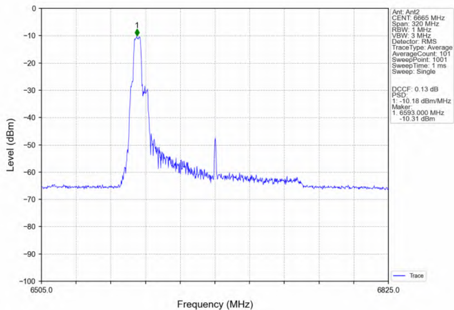
802.11be(EHT160)_MCH_6665MHz_26+52 / _Ant2_NTNV
