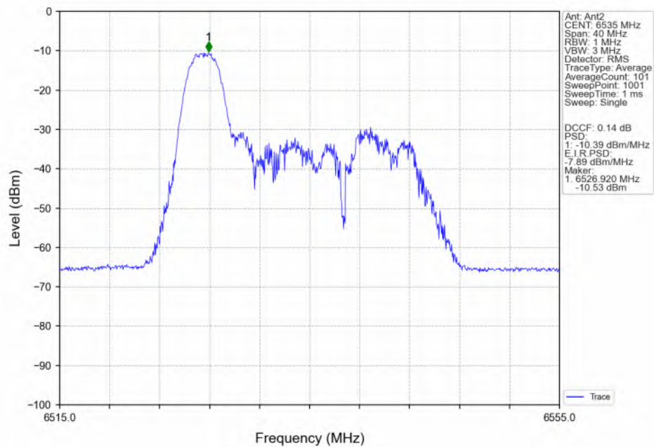
802.11be(EHT20)_LCH_6535MHz_RU26_Left(0)_Ant2_NTNV
