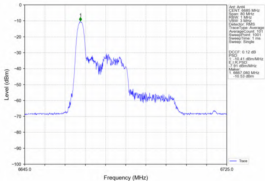
802.11be(EHT40)_MCH_6685MHz_RU26_Left(0)_Ant4_NTNV
