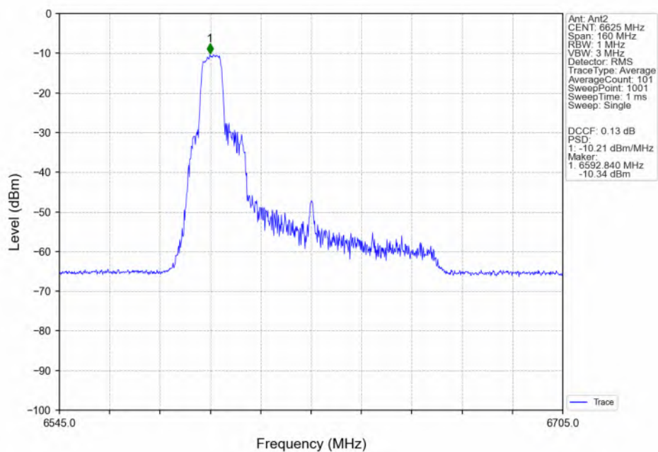
802.11be(EHT80)_LCH_6625MHz_26+52_ / Ant2_NTNV
