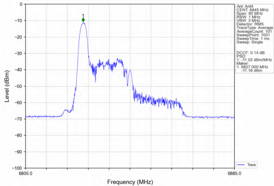
802.11be(EHT40)_HCH_6845MHz_RU26_Left(0)_MIMO_NTNV
