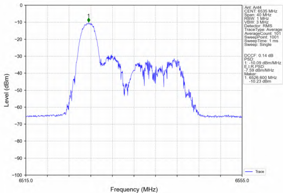
802.11be(EHT20) LCH_6535MHz_RU26_Left(0)_Ant4_NTNV
