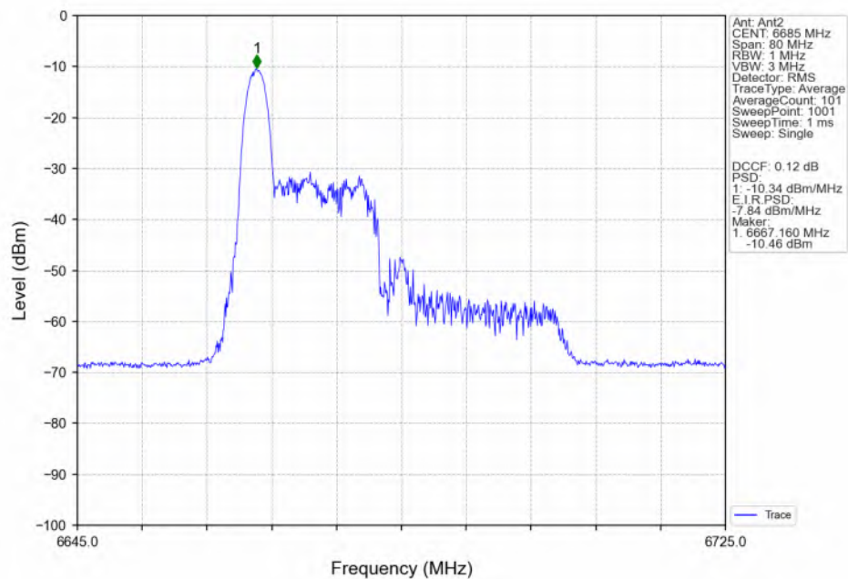
802.11be(EHT40)_MCH_6685MHz_RU26_Left(0)_Ant2_NTNV
