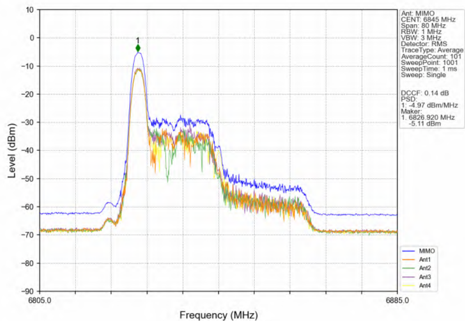
802.11be(EHT40)_HCH_6845MHz_RU26_Left(0)_MIMO_NTNV
