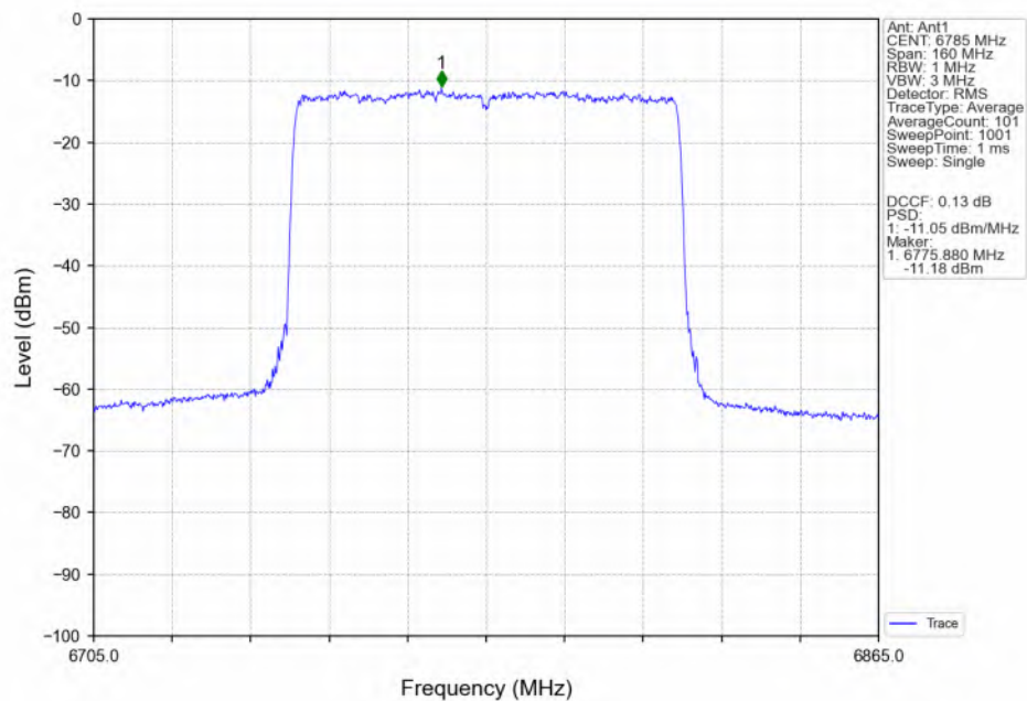
802.11be(EHT80)_HCH_6785MHz_RU996_Left(67)_Ant1_NTNV
