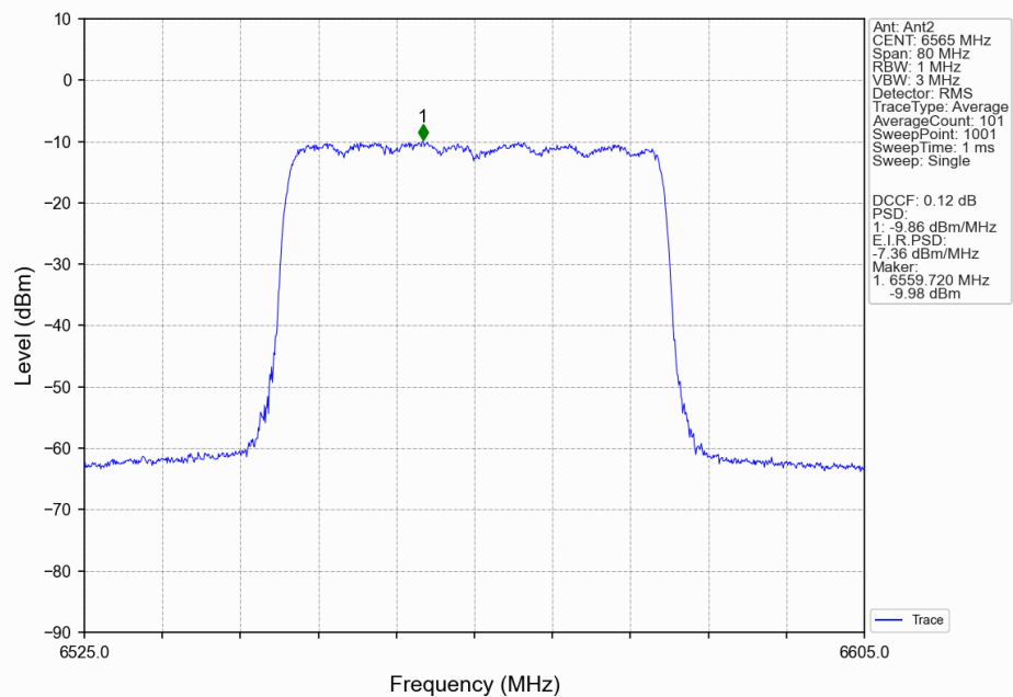
802.11be(EHT40) LCH_6565MHz_RU484_Left(65)_Ant2_NTNV
