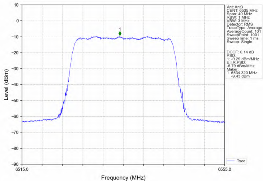
802.11be(EHT20) LCH_6535MHz_RU242_Left(61)_Ant3_NTNV
