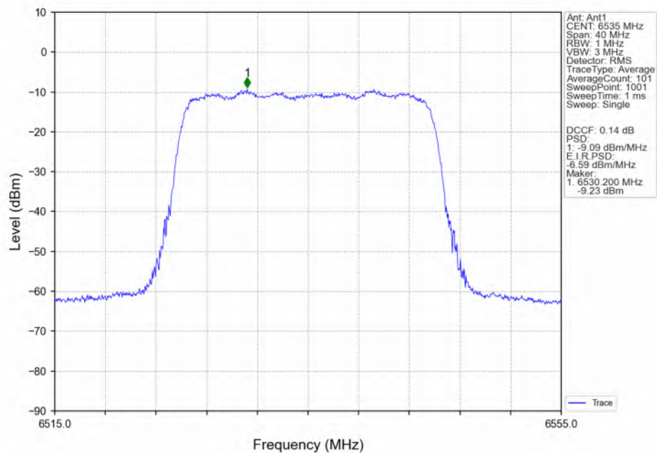
802.11be(EHT20) LCH_6535MHz_RU242_Left(61)_Ant1_NTNV
