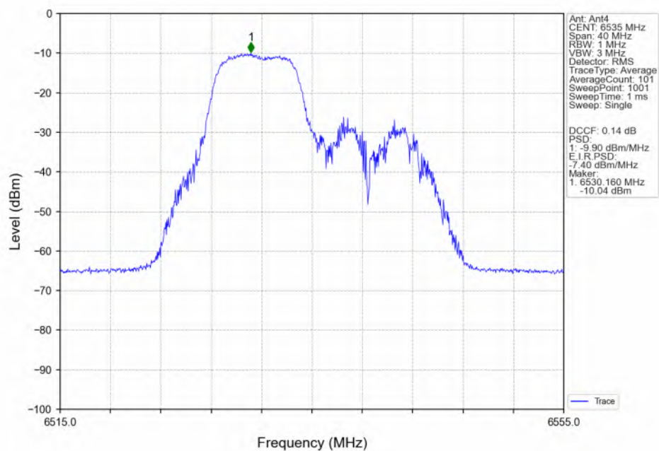
802.11be(EHT20)_LCH_6535MHz_26+52_ / Ant4_NTNV
