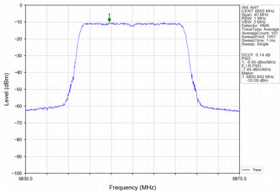
802.11be(EHT20)_HCH_6855MHz_RU242_Left(61)_Ant1_NTNV
