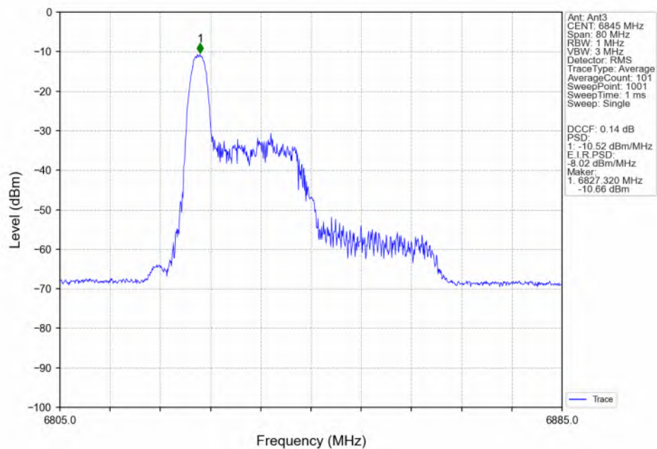
802.11be(EHT40)_HCH_6845MHz_RU26_Left(0)_Ant3_NTNV
