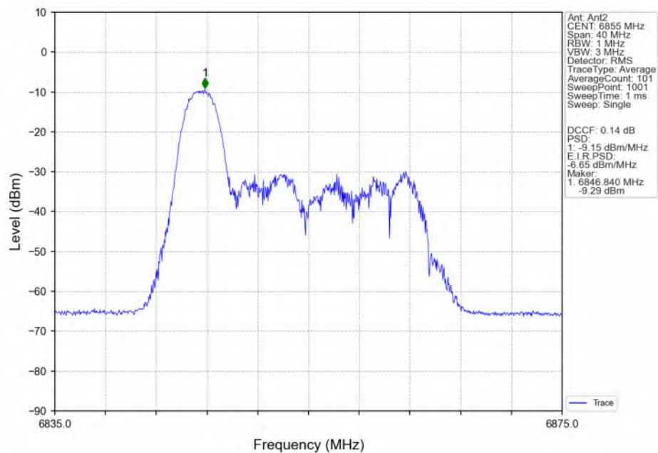
802.11be(EHT20)_HCH_6855MHz_RU26_Left(0)_Ant2_NTNV
