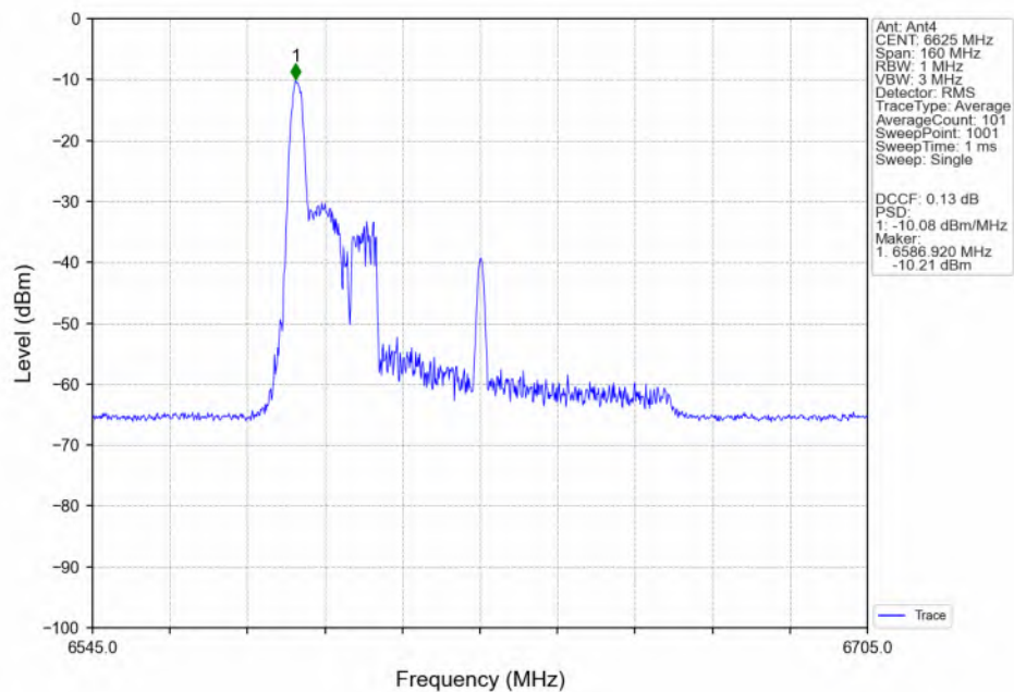
802.11be(EHT80) LCH_6625MHz_RU26_Left(0)_Ant4_NTNV
