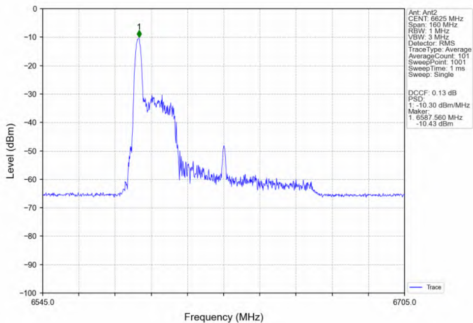
802.11be(EHT80) LCH_6625MHz_RU26_Left(0)_Ant2_NTNV
