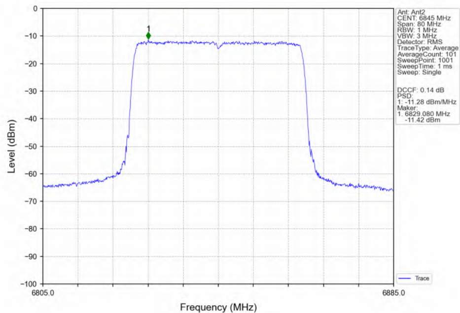
802.11be(EHT40)_HCH_6845MHz_RU484_Left(65)_Ant2_NTNV
