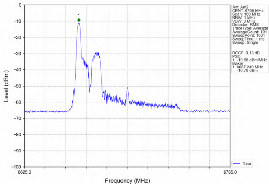
802.11be(EHT80)_MCH_6705MHz_RU26_Left(0)_Ant2_NTNV
