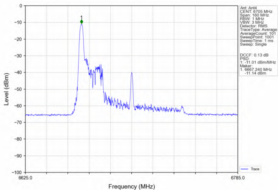
802.11be(EHT80)_MCH_6705MHz_RU26_Left(0)_Ant4_NTNV
