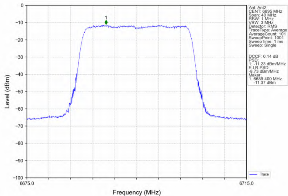
802.11be(EHT20)_MCH_6695MHz_RU242_Left(61)_Ant2_NTNV
