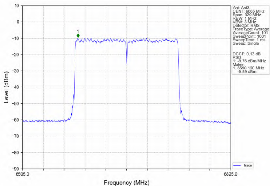
802.11be(EHT160)_MCH_6665MHz_2xRU996_Left(68)_Ant3_NTNV
