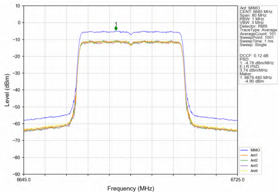
802.11be(EHT40)_MCH_6685MHz_RU484_Left(65)_MIMO_NTNV
