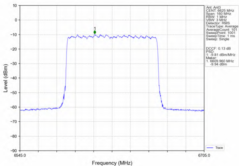
802.11be(EHT80) LCH_6625MHz_RU996_Left(67)_Ant3_NTNV
