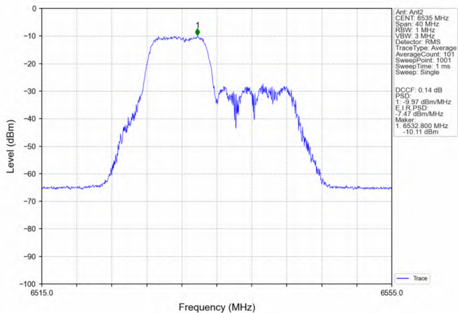
802.11be(EHT20)_LCH_6535MHz_26+52_ / Ant2_NTNV
