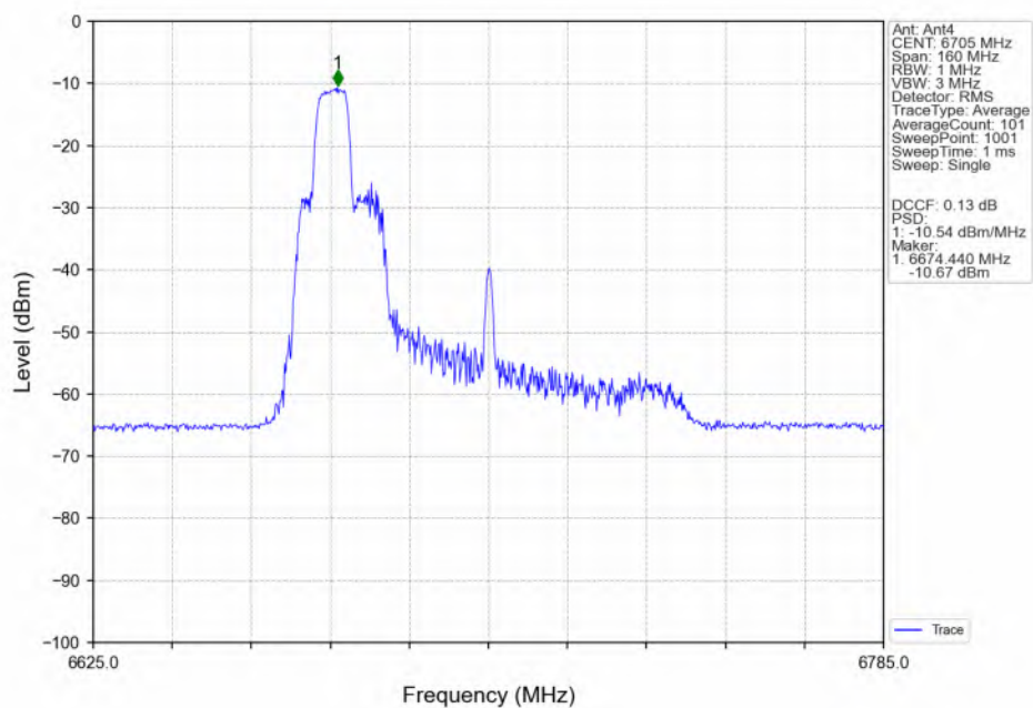
802.11be(EHT80)_MCH_6705MHz_26+52_/_Ant4_NTNV
