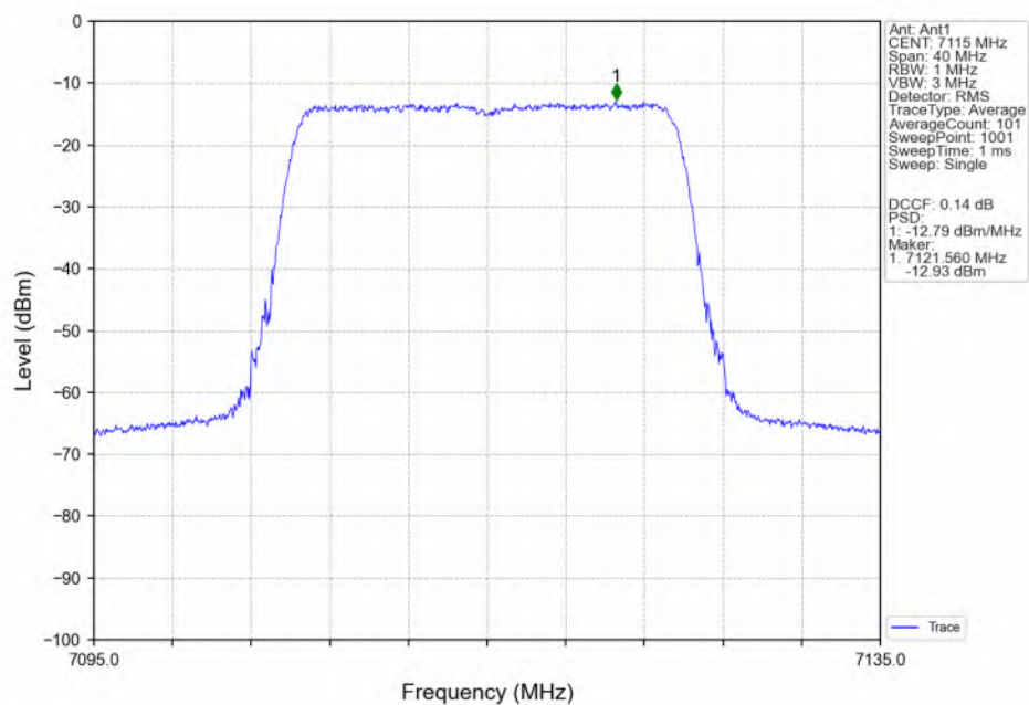
802.11be(EHT20)_HCH_7115MHz_RU242_Left(61)_Ant1_NTNV
