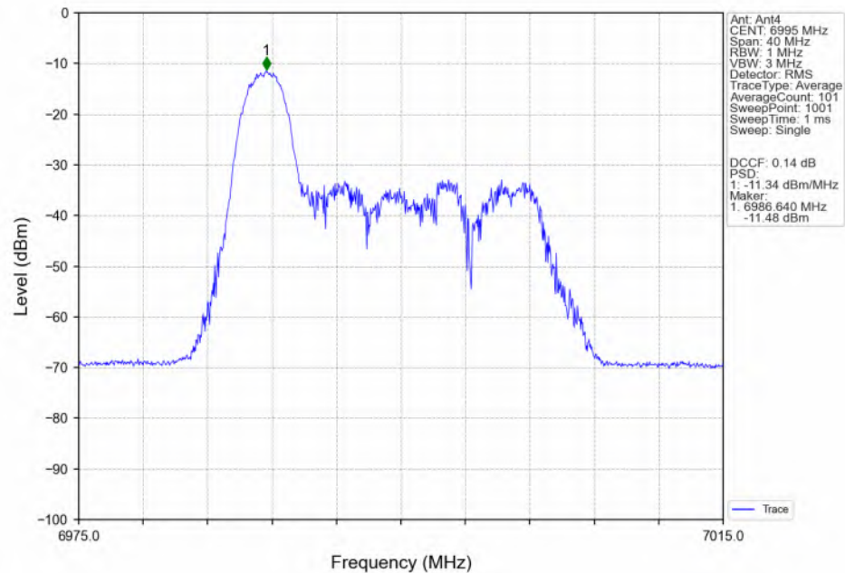
802.11be(EHT20)_MCH_6995MHz_RU26_Left(0)_MIMO_NTNV
