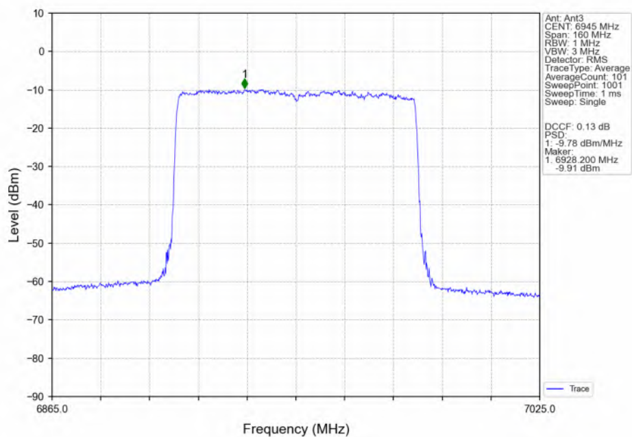
802.11be(EHT80) LCH_6945MHz_RU996_Left(67)_Ant3_NTNV
