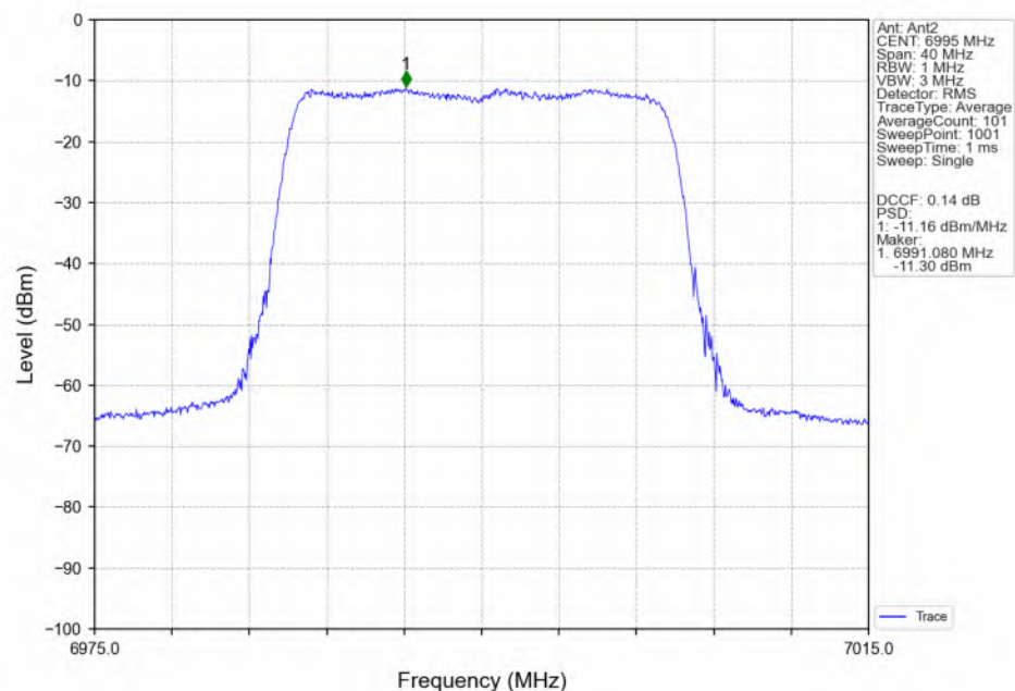
802.11be(EHT20)_MCH_6995MHz_RU242_Left(61)_Ant2_NTNV
