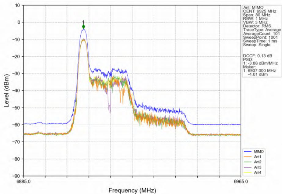
802.11be(EHT40) LCH_6925MHz_RU26_Left(0)_MIMO_NTNV
