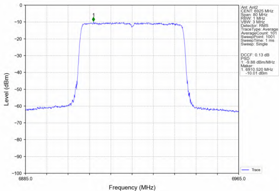
802.11be(EHT40) LCH_6925MHz_RU484_Left(65)_Ant2_NTNV
