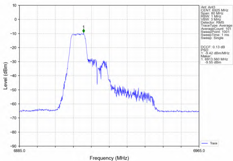
802.11be(EHT40)_LCH_6925MHz_26+52_/_Ant3_NTNV
