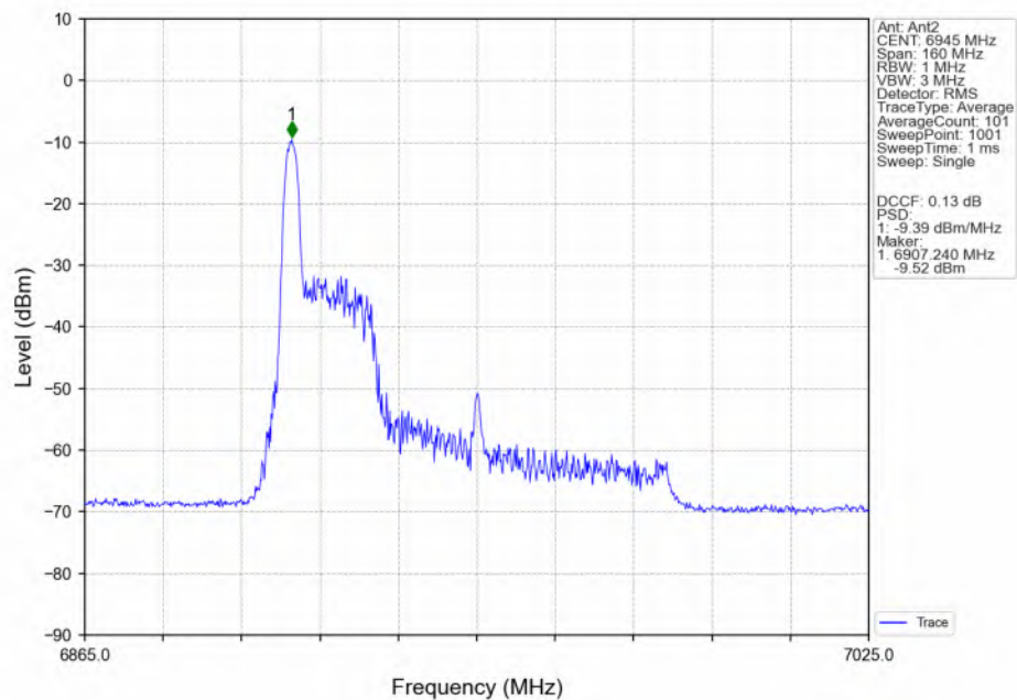
802.11be(EHT80) LCH_6945MHz_RU26_Left(0)_Ant2_NTNV
