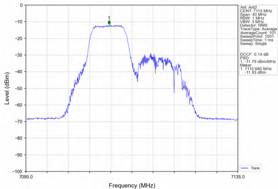
802.11be(EHT20)_HCH_7115MHz_26+52_ / Ant2_NTNV
