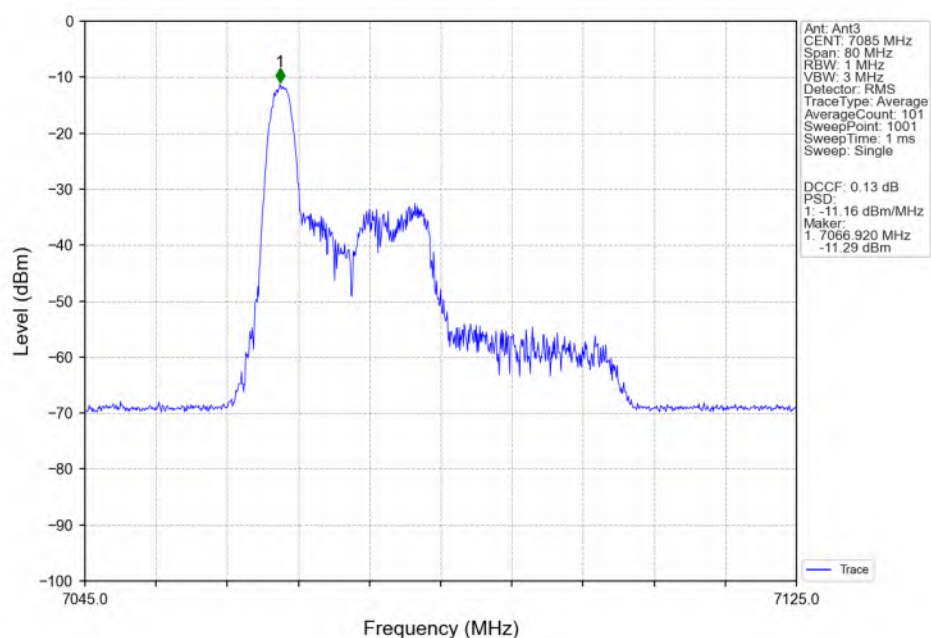
802.11be(EHT40)_HCH_7085MHz_RU26_Left(0)_Ant3_NTNV
