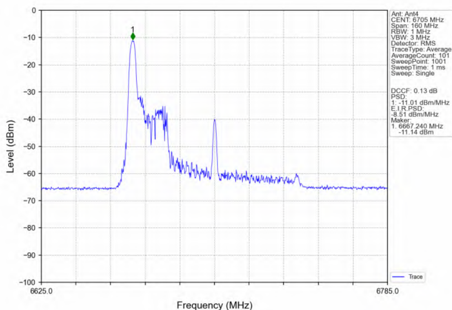
802.11be(EHT80)_MCH_6705MHz_RU26_Left(0)_Ant4_NTNV
