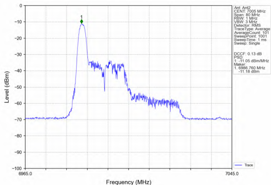
802.11be(EHT40)_MCH_7005MHz_RU26_Left(0)_Ant2_NTNV
