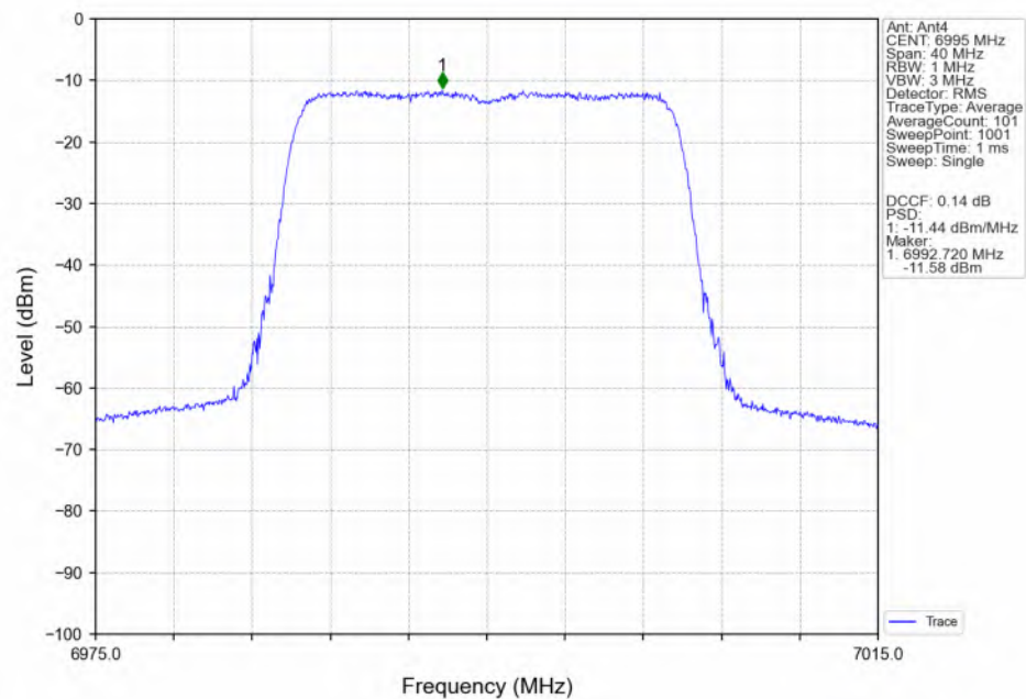
802.11be(EHT20)_MCH_6995MHz_RU242_Left(61)_Ant4_NTNV
