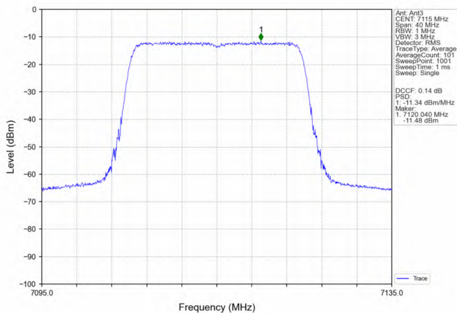
802.11be(EHT20)_HCH_7115MHz_RU242_Left(61)_Ant3_NTNV
