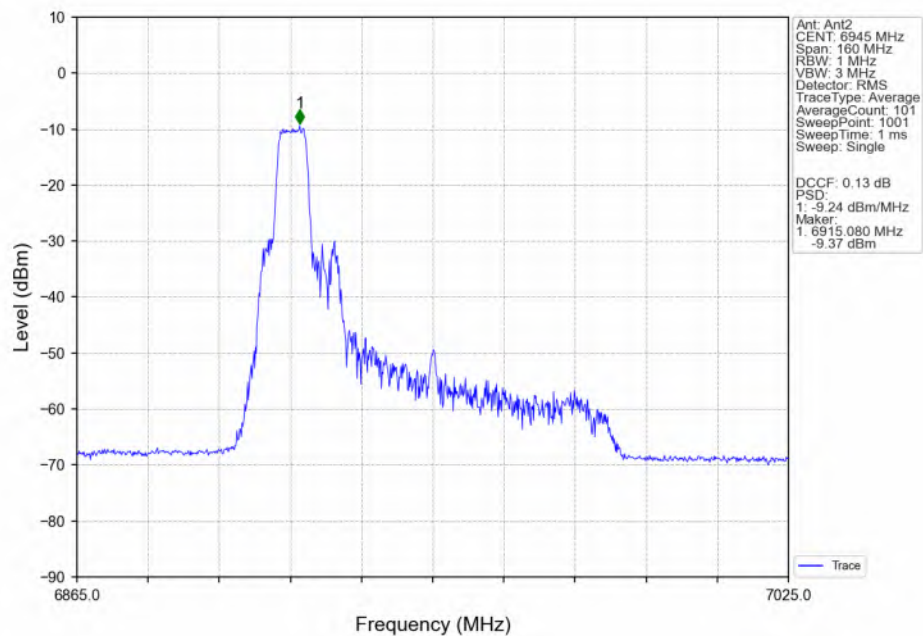
802.11be(EHT80)_LCH_6945MHz_26+52_ / Ant2_NTNV
