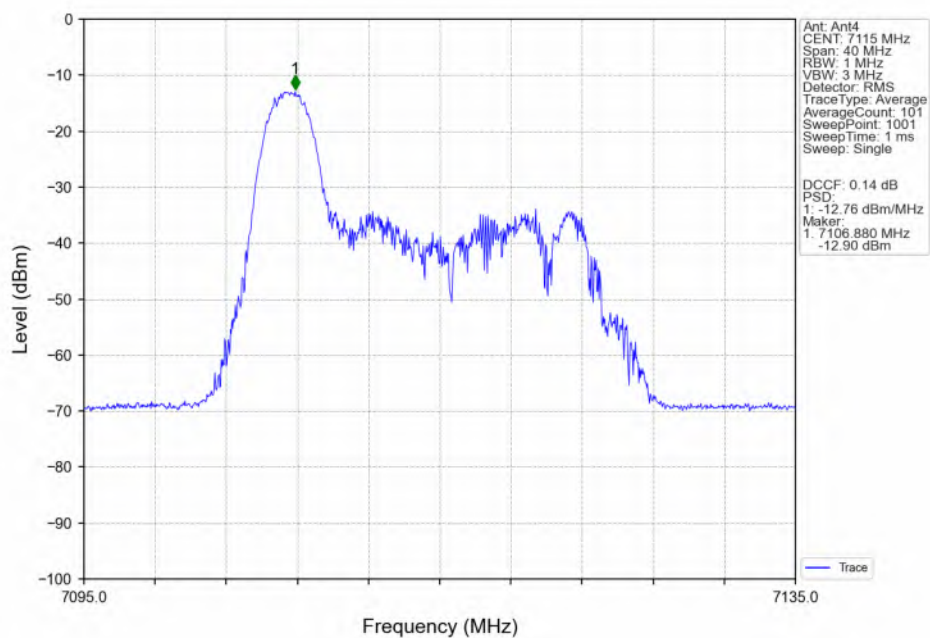
802.11be(EHT20)_HCH_7115MHz_RU26_Left(0)_Ant4_NTNV
