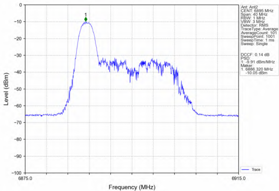
802.11be(EHT20)_LCH_6895MHz_RU26_Left(0)_Ant2_NTNV
