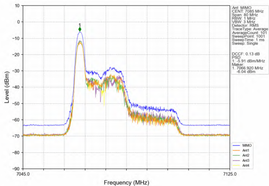
802.11be(EHT40)_HCH_7085MHz_RU26_Left(0)_MIMO_NTNV
