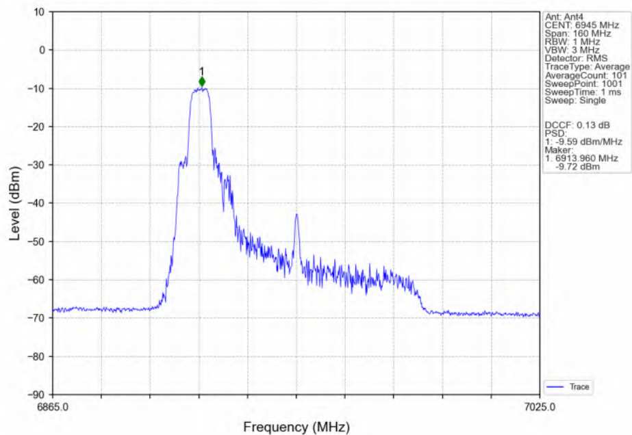
802.11be(EHT80)_LCH_6945MHz_26+52_/_Ant4_NTNV
