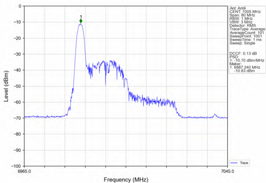
802.11be(EHT40)_MCH_7005MHz_RU26_Left(0)_Ant4_NTNV
