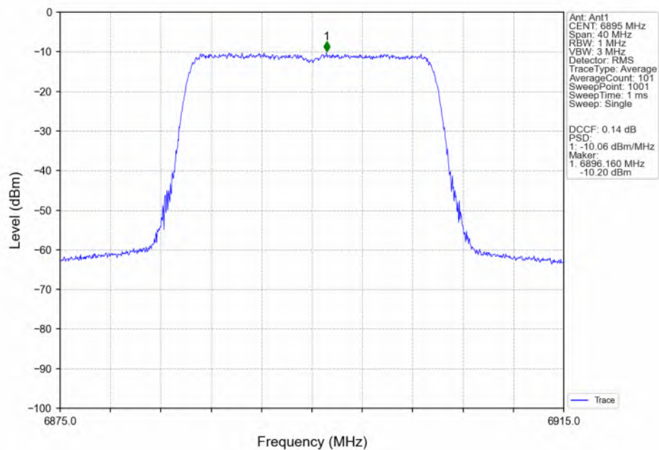
802.11be(EHT20) LCH_6895MHz_RU242_Left(61)_Ant1_NTNV
