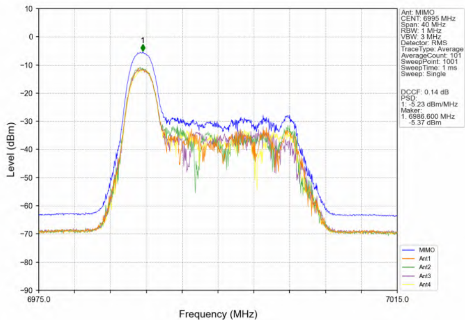
802.11be(EHT20)_MCH_6995MHz_RU26_Left(0)_MIMO_NTNV
