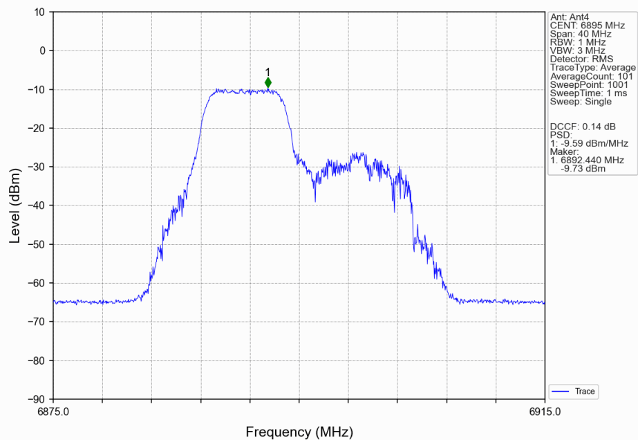
802.11be(EHT20)_LCH_6895MHz_26+52 / Ant4_NTNV
