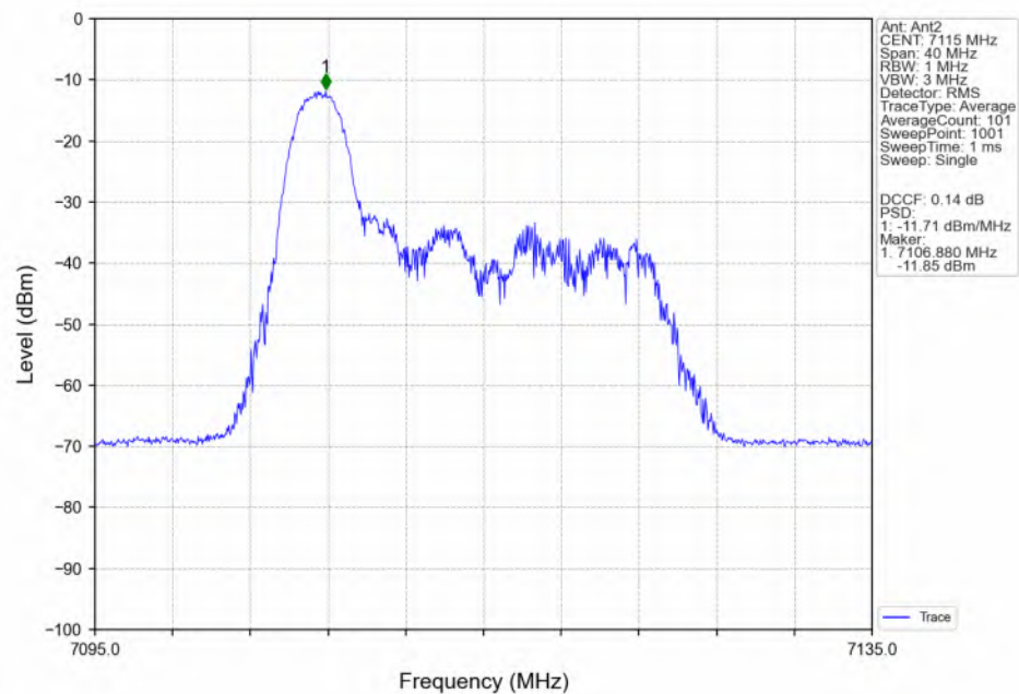
802.11be(EHT20)_HCH_7115MHz_RU26_Left(0)_Ant2_NTNV
