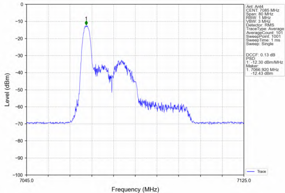
802.11be(EHT40)_HCH_7085MHz_RU26_Left(0)_MIMO_NTNV
