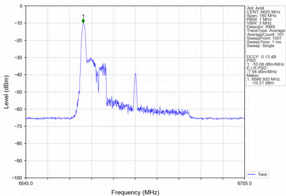
802.11be(EHT80) LCH_6625MHz_RU26_Left(0)_Ant4_NTNV
