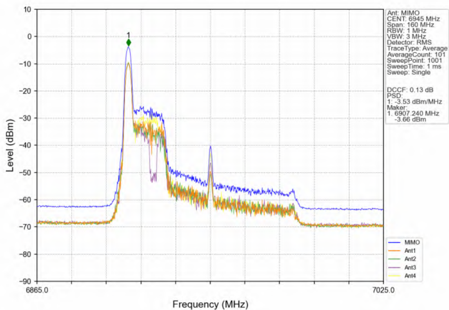
802.11be(EHT80)_LCH_6945MHz_RU996_Left(67)_Ant1_NTNV
