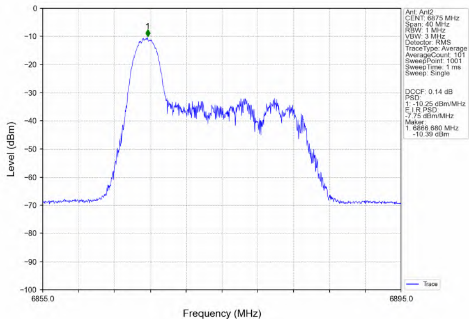
802.11be(EHT20)_HCH_6875MHz_RU26_Left(0)_Ant2_NTNV
