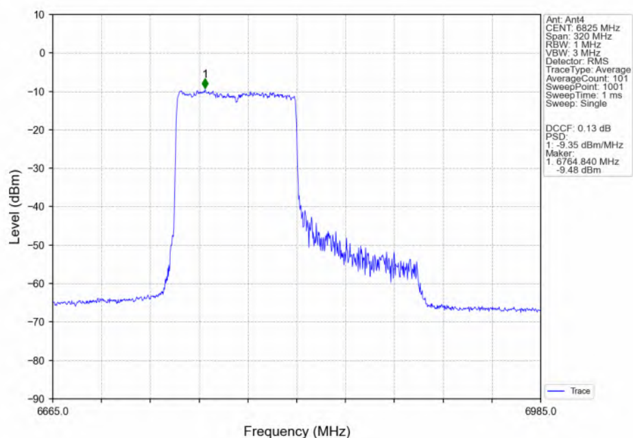
802.11be(EHT160)_HCH_6825MHz_RU996_Left(67)_Ant4_NTNV
