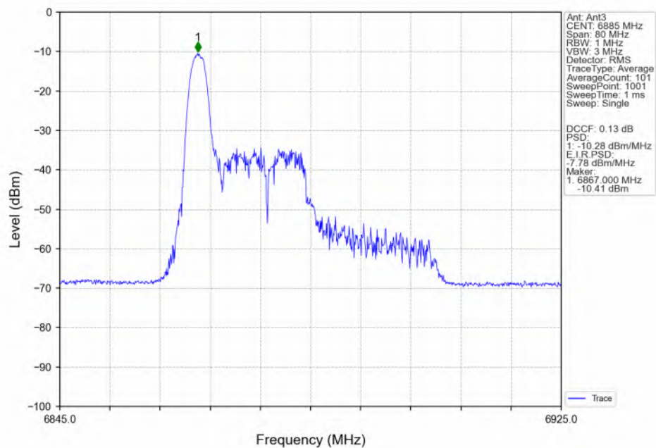
802.11be(EHT40)_HCH_6885MHz_RU26_Left(0)_Ant3_NTNV
