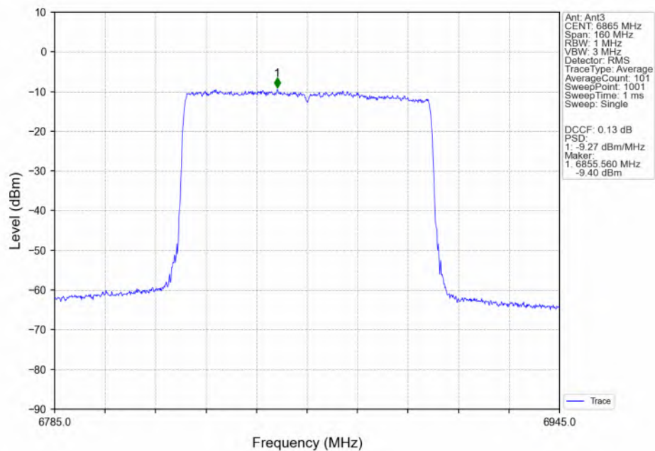
802.11be(EHT80)_HCH_6865MHz_RU996_Left(67)_Ant3_NTNV
