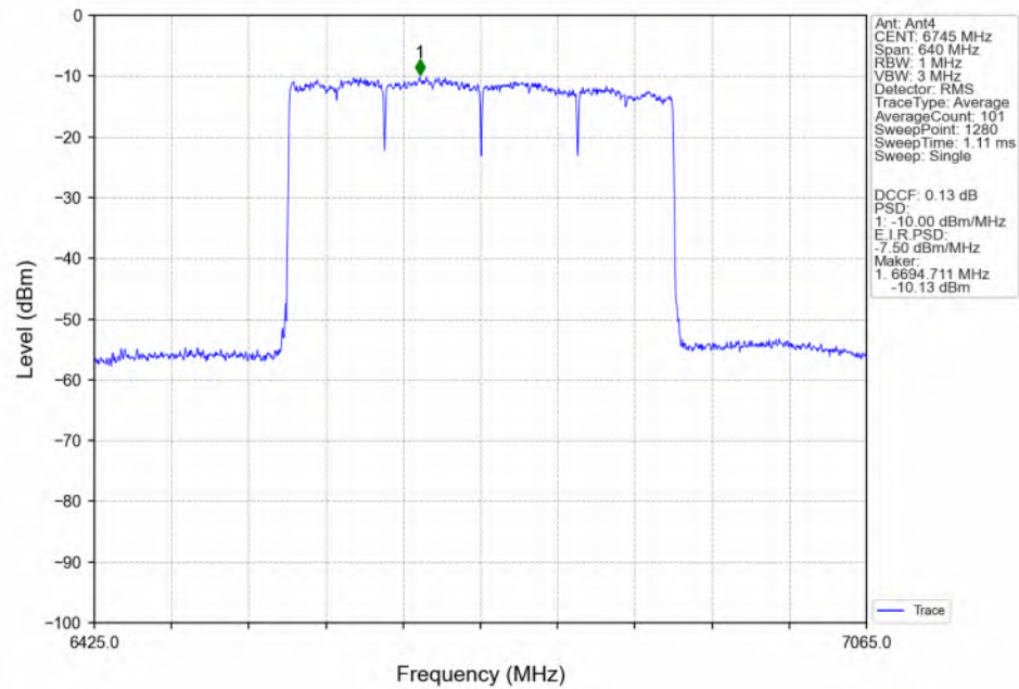
802.11be(EHT320)_LCH_6745MHz_4xRU996_Left(70)_MIMO_NTNV
