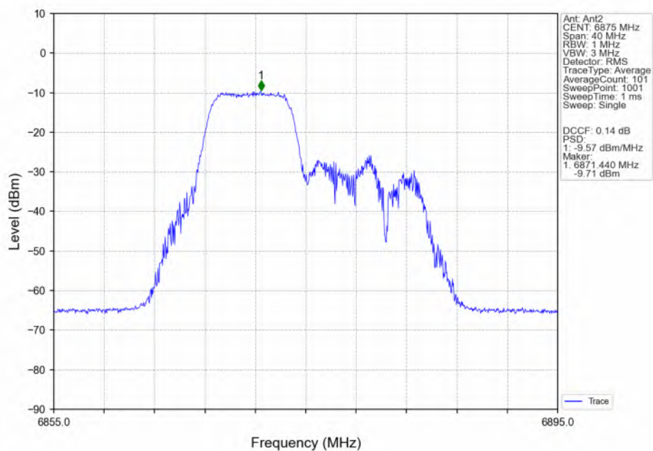
802.11be(EHT20)_HCH_6875MHz_26+52_ / Ant2_NTNV
