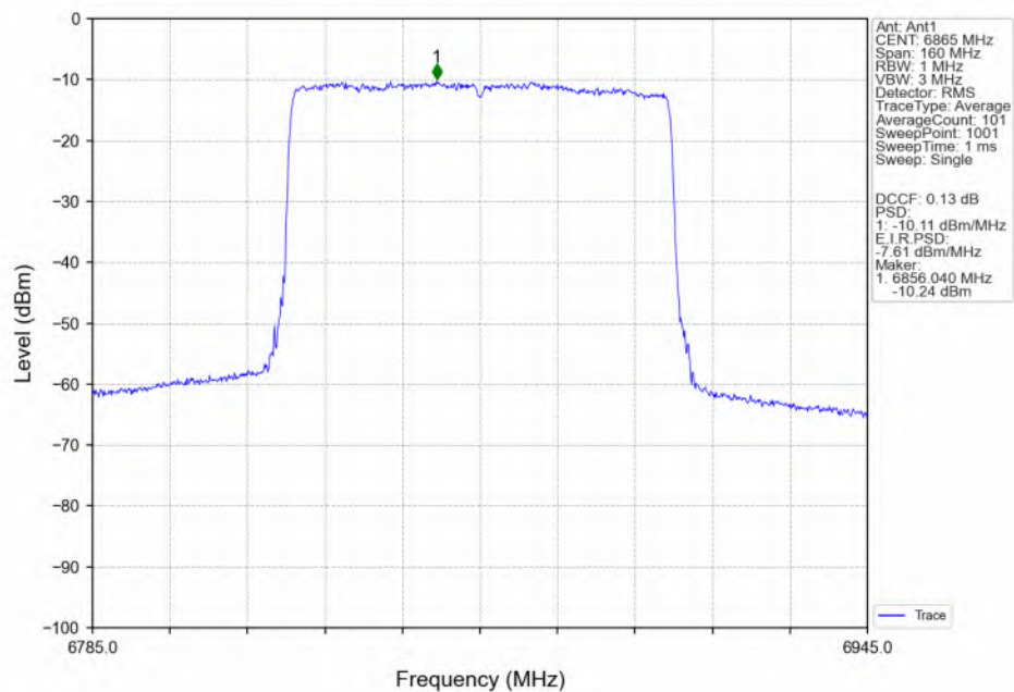
802.11be(EHT80)_HCH_6865MHz_RU996_Left(67)_Ant1_NTNV
