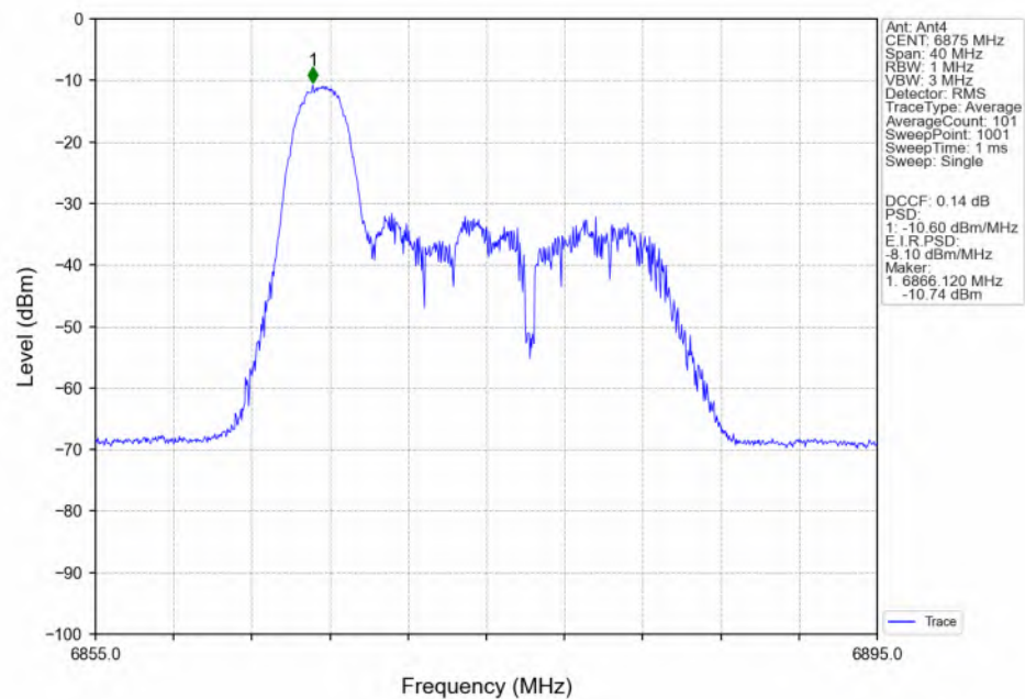
802.11be(EHT20)_HCH_6875MHz_RU26_Left(0)_Ant4_NTNV
