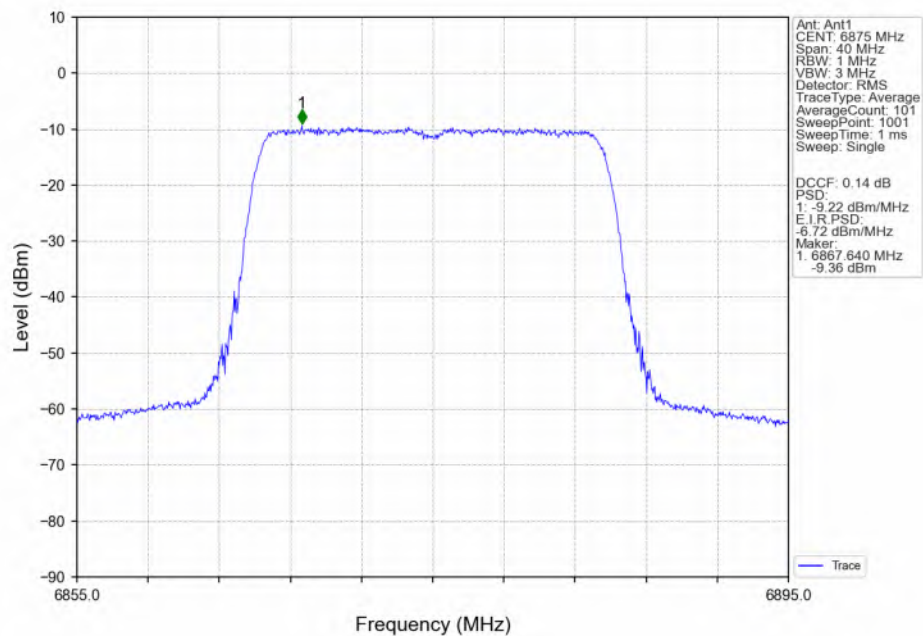
802.11be(EHT20)_HCH_6875MHz_RU242_Left(61)_Ant1_NTNV
