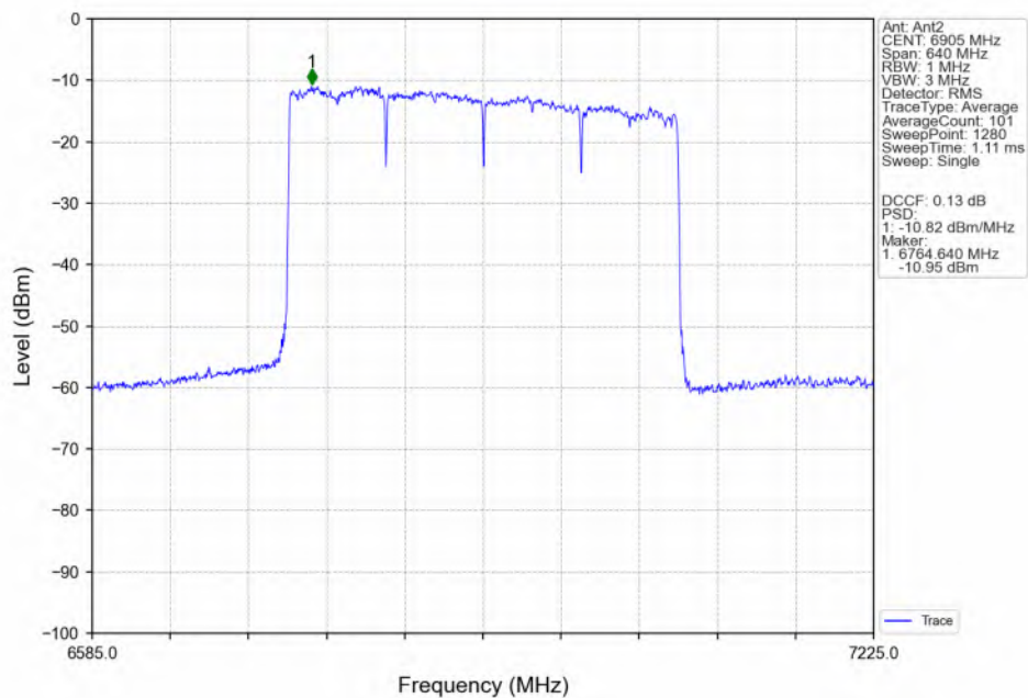
802.11be(EHT320)_HCH_6905MHz_4xRU996_Left(70)_Ant2_NTNV
