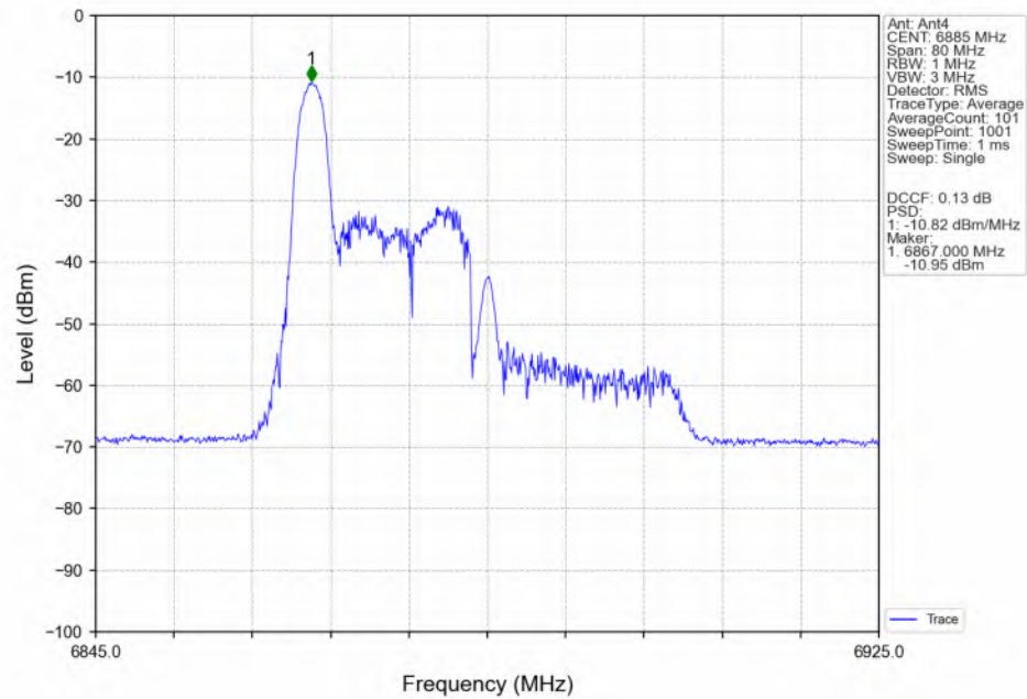
802.11be(EHT40)_HCH_6885MHz_RU26_Left(0)_MIMO_NTNV
