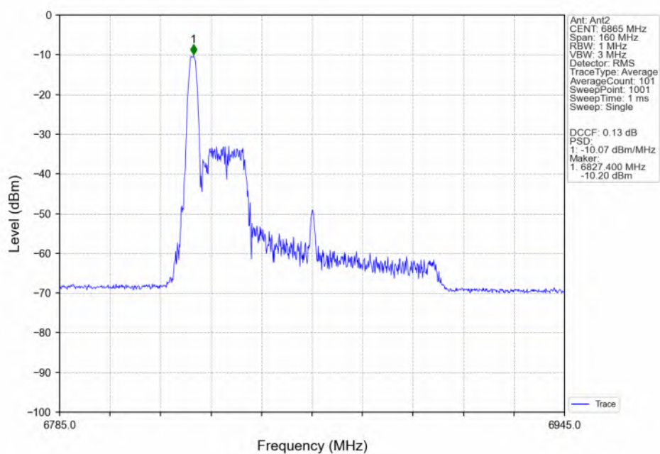
802.11be(EHT80)_HCH_6865MHz_RU26_Left(0)_Ant2_NTNV
