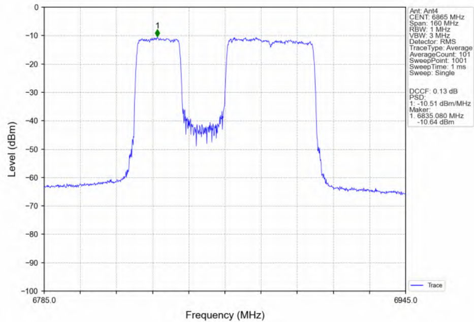
802.11be(EHT80)_HCH_6865MHz_P-20M-RU242+484 / MIMO_NTNV
