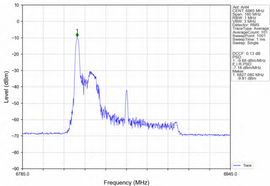
802.11be(EHT80)_HCH_6865MHz_RU26_Left(0)_Ant4_NTNV
