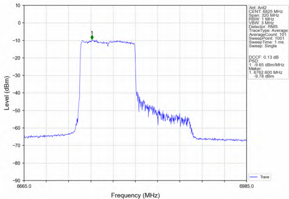
802.11be(EHT160)_HCH_6825MHz_RU996_Left(67)_Ant2_NTNV
