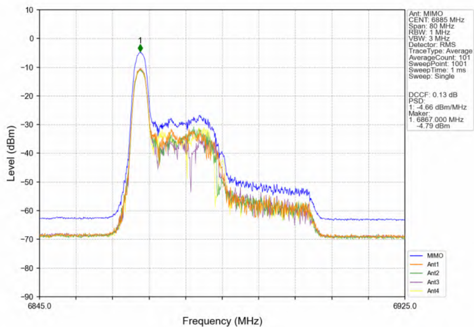
802.11be(EHT40)_HCH_6885MHz_RU26_Left(0)_MIMO_NTNV
