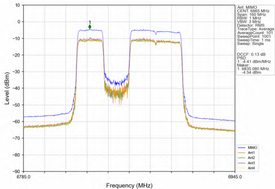
802.11be(EHT80)_HCH_6865MHz_P-20M-RU242+484 / MIMO_NTNV
