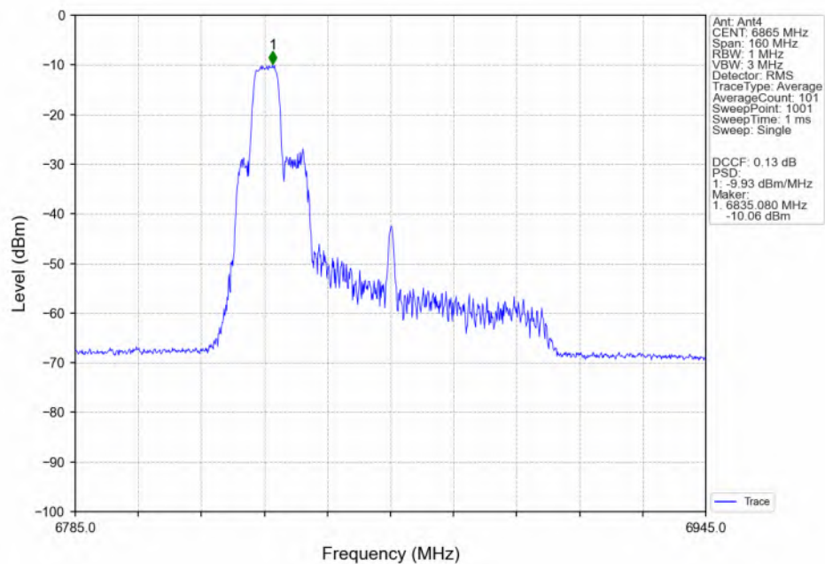
802.11be(EHT80)_HCH_6865MHz_26+52_ / Ant4_NTNV
