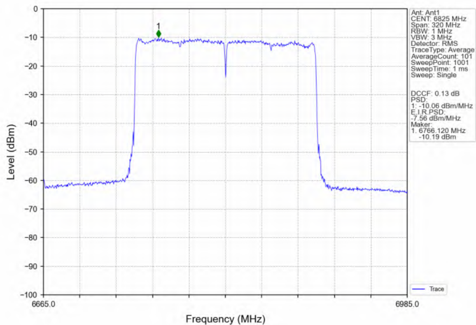
802.11be(EHT160)_HCH_6825MHz_2xRU996_Left(68)_Ant1_NTNV
