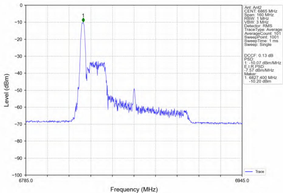
802.11be(EHT80)_HCH_6865MHz_RU26_Left(0)_Ant2_NTNV
