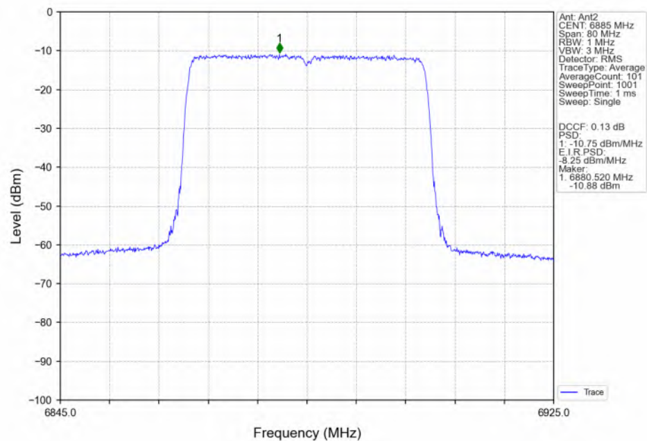
802.11be(EHT40)_HCH_6885MHz_RU484_Left(65)_Ant2_NTNV
