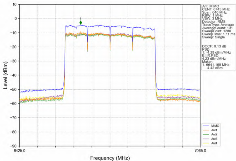
802.11be(EHT320)_LCH_6745MHz_4xRU996_Left(70)_MIMO_NTNV
