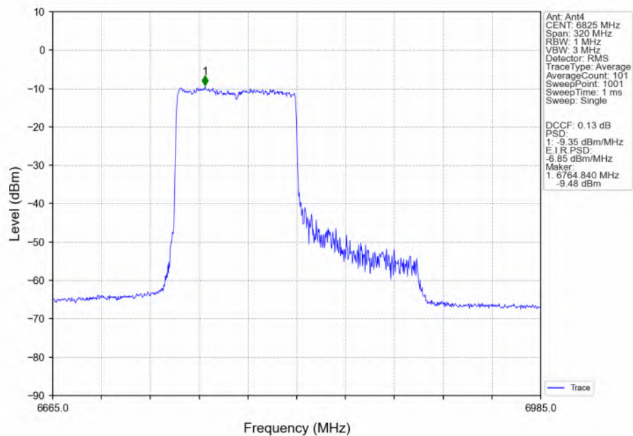
802.11be(EHT160)_HCH_6825MHz_RU996_Left(67)_Ant4_NTNV
