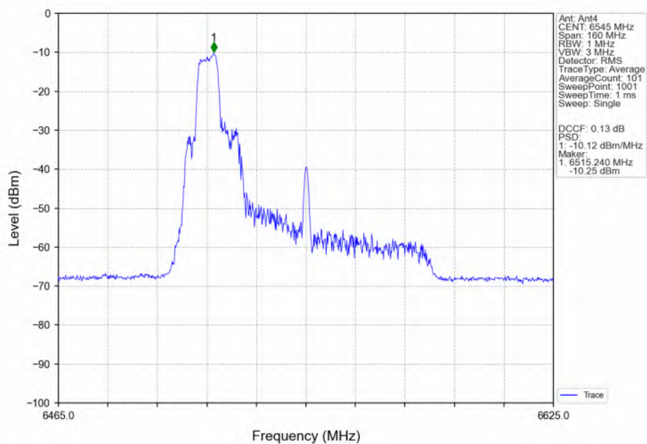
802.11be(EHT80)_HCH_6545MHz_26+52 / MIMO_NTNV
