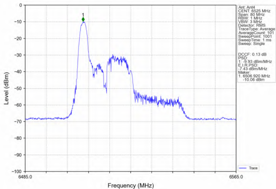
802.11be(EHT40)_HCH_6525MHz_RU26_Left(0)_Ant4_NTNV
