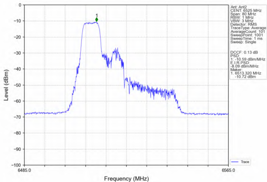
802.11be(EHT40)_HCH_6525MHz_26+52_ / Ant2_NTNV
