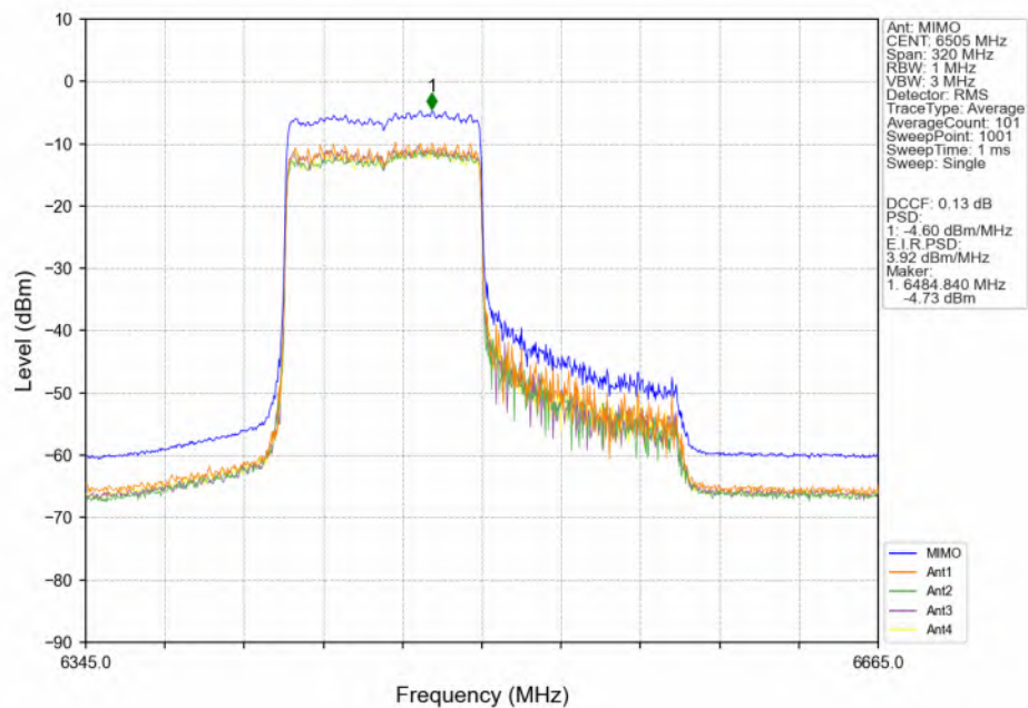
802.11be(EHT160)_HCH_6505MHz_RU996_Left(67)_MIMO_NTNV
