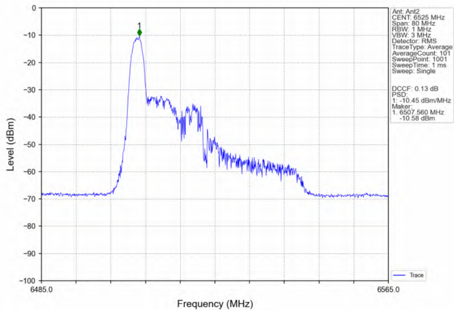
802.11be(EHT40)_HCH_6525MHz_RU26_Left(0)_Ant2_NTNV
