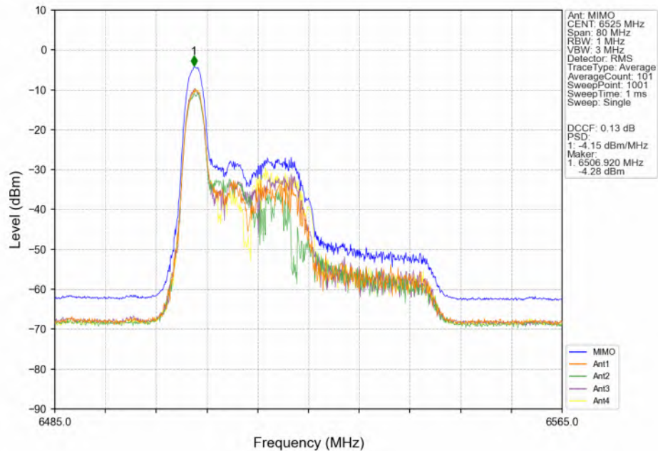
802.11be(EHT40)_HCH_6525MHz_RU484_Left(65)_Ant1_NTNV
