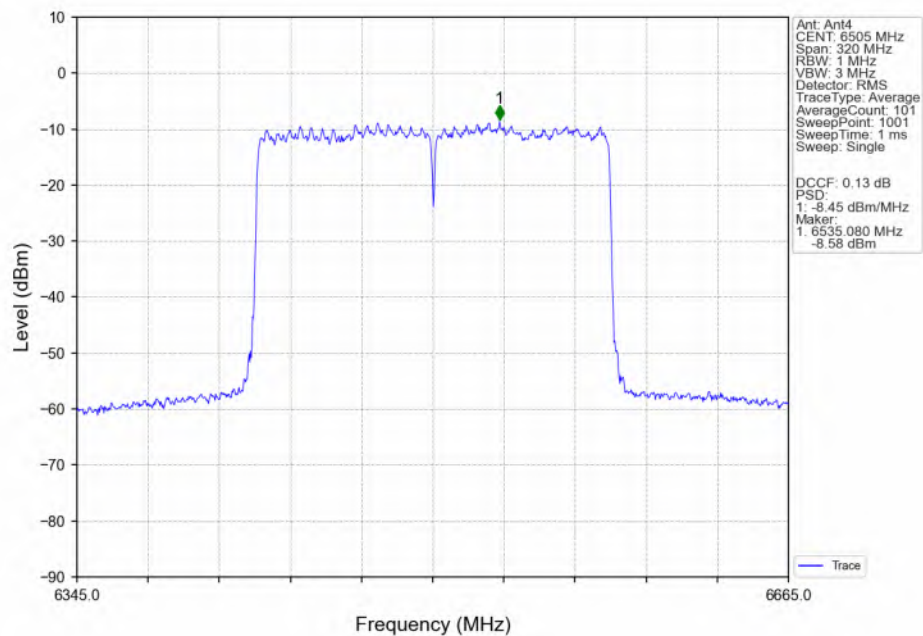
802.11be(EHT160)_HCH_6505MHz_2xRU996_Left(68)_Ant4_NTNV
