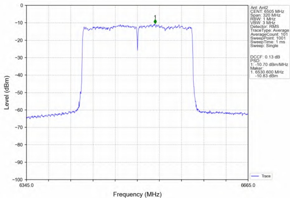
802.11be(EHT160)_HCH_6505MHz_2xRU996_Left(68)_Ant2_NTNV
