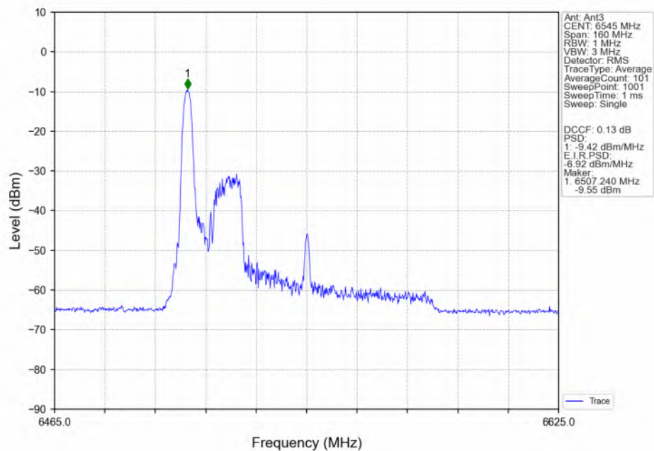
802.11be(EHT80)_HCH_6545MHz_RU26_Left(0)_Ant3_NTNV
