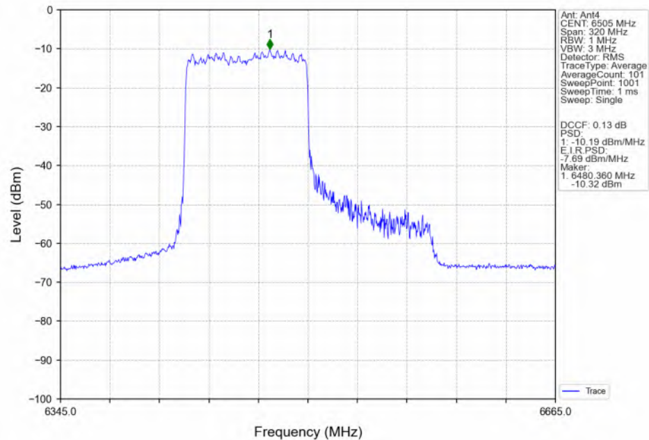
802.11be(EHT160)_HCH_6505MHz_RU996_Left(67)_MIMO_NTNV
