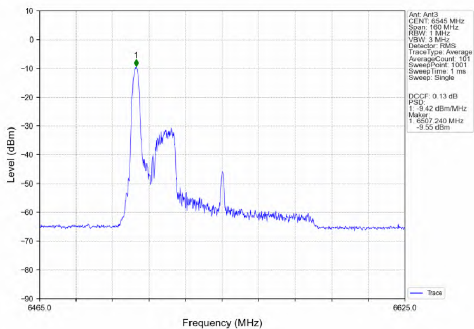
802.11be(EHT80)_HCH_6545MHz_RU26_Left(0)_Ant3_NTNV
