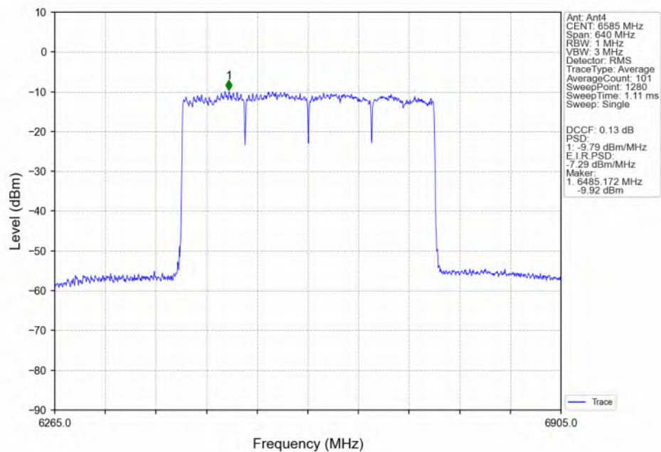
802.11be(EHT320)_MCH_6585MHz_4xRU996_Left(70)_Ant4_NTNV
