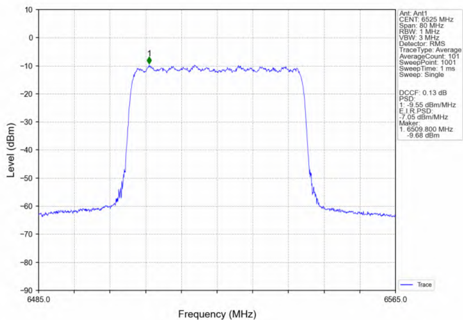
802.11be(EHT40)_HCH_6525MHz_RU484_Left(65)_Ant1_NTNV
