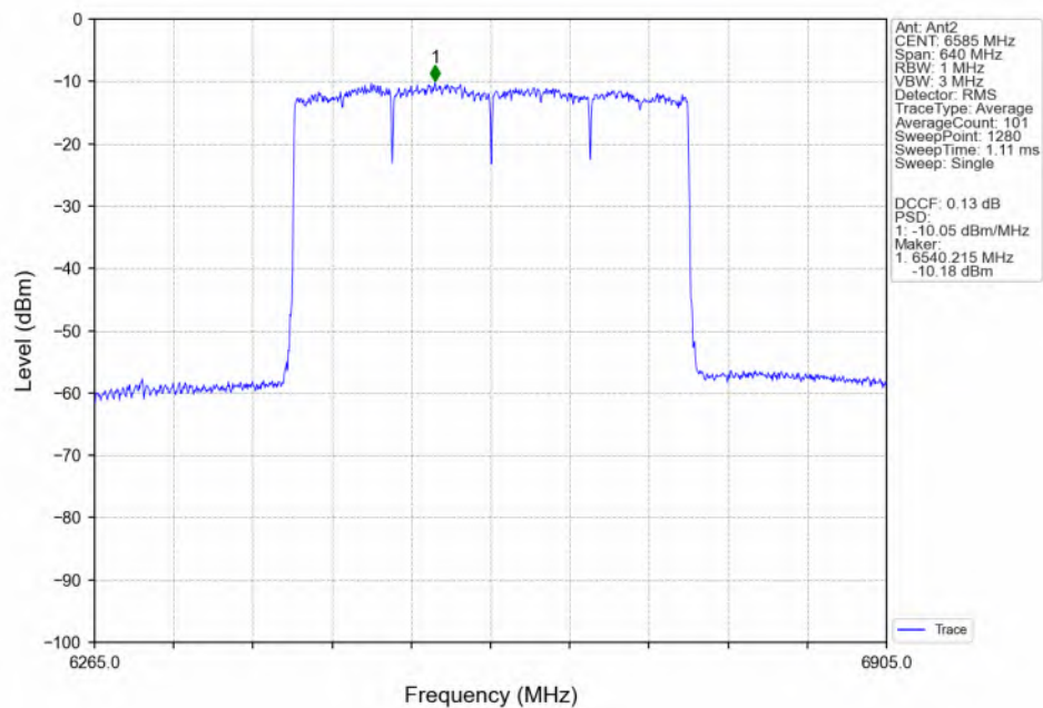
802.11be(EHT320)_MCH_6585MHz_4xRU996_Left(70)_Ant2_NTNV
