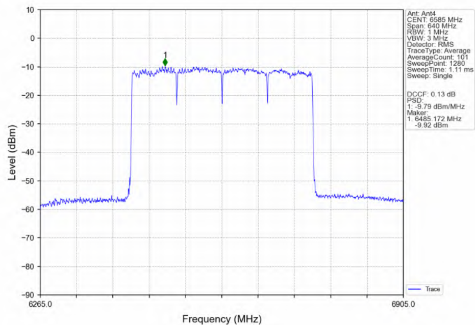
802.11be(EHT320)_MCH_6585MHz_4xRU996_Left(70)_Ant4_NTNV
