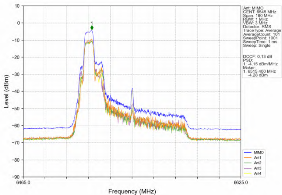
802.11be(EHT80)_HCH_6545MHz_26+52 / MIMO_NTNV
