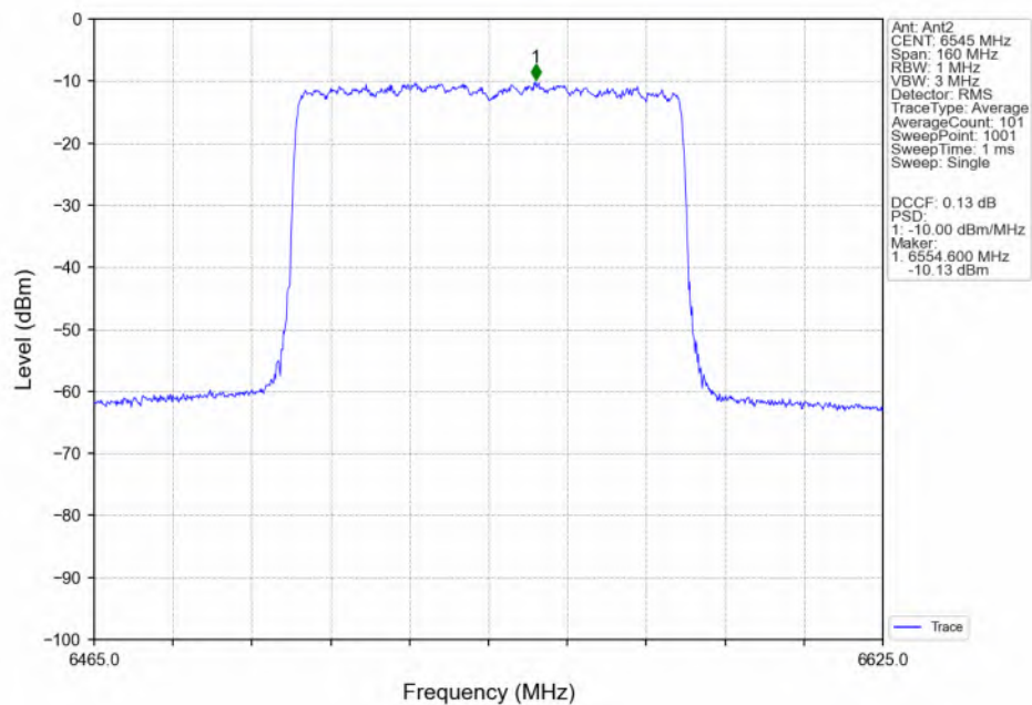
802.11be(EHT80)_HCH_6545MHz_RU996_Left(67)_Ant2_NTNV
