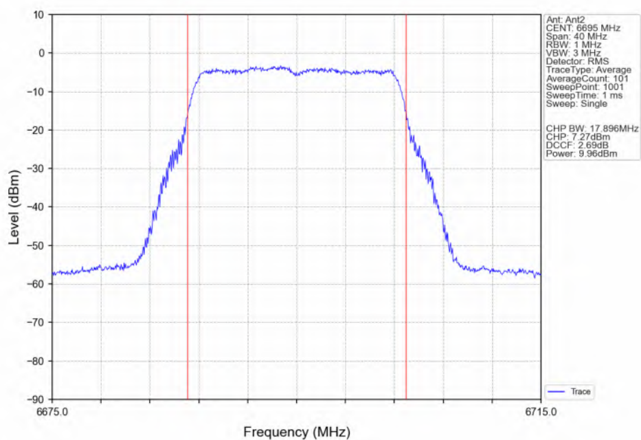
802.11a_MCH_6695MHz_Ant2_NTNV
