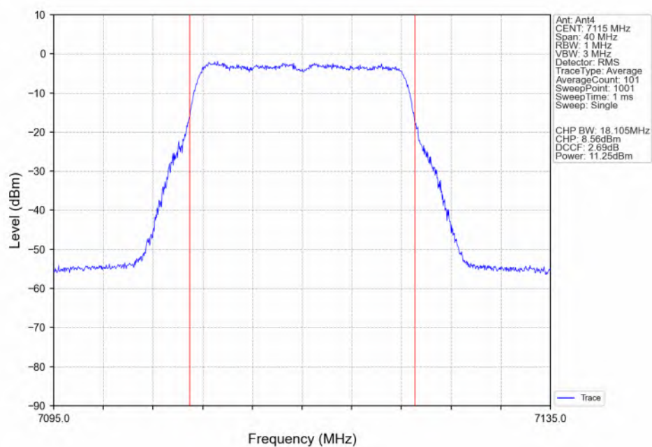
802.11a_HCH_7115MHz_Ant4_NTNV
