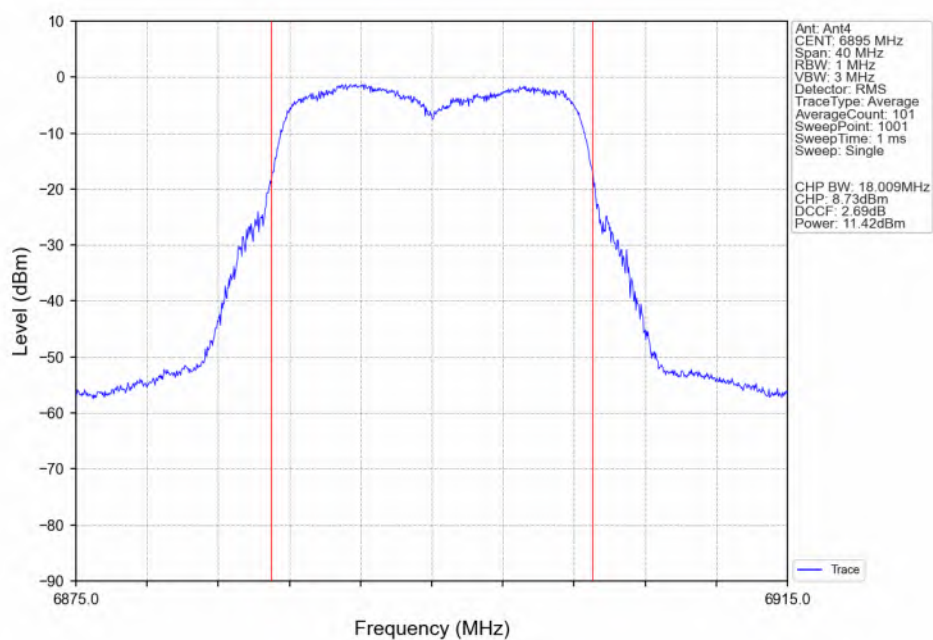
802.11a_LCH_6895MHz_Ant4_NTNV
