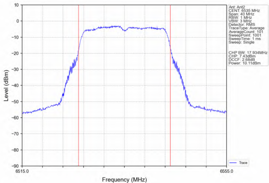
802.11a_LCH_6535MHz_Ant2_NTNV
