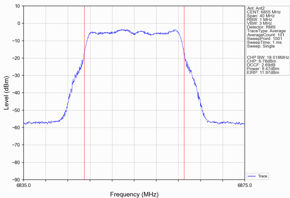
802.11a_HCH_6855MHz_Ant2_NTNV
