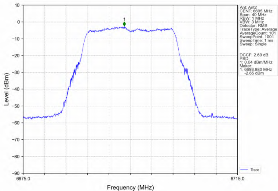
802.11a_MCH_6695MHz_Ant2_NTNV
