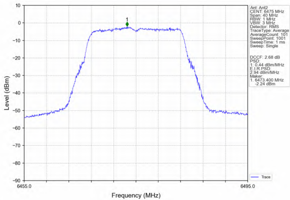
802.11a_MCH_6475MHz_Ant2_NTNV
