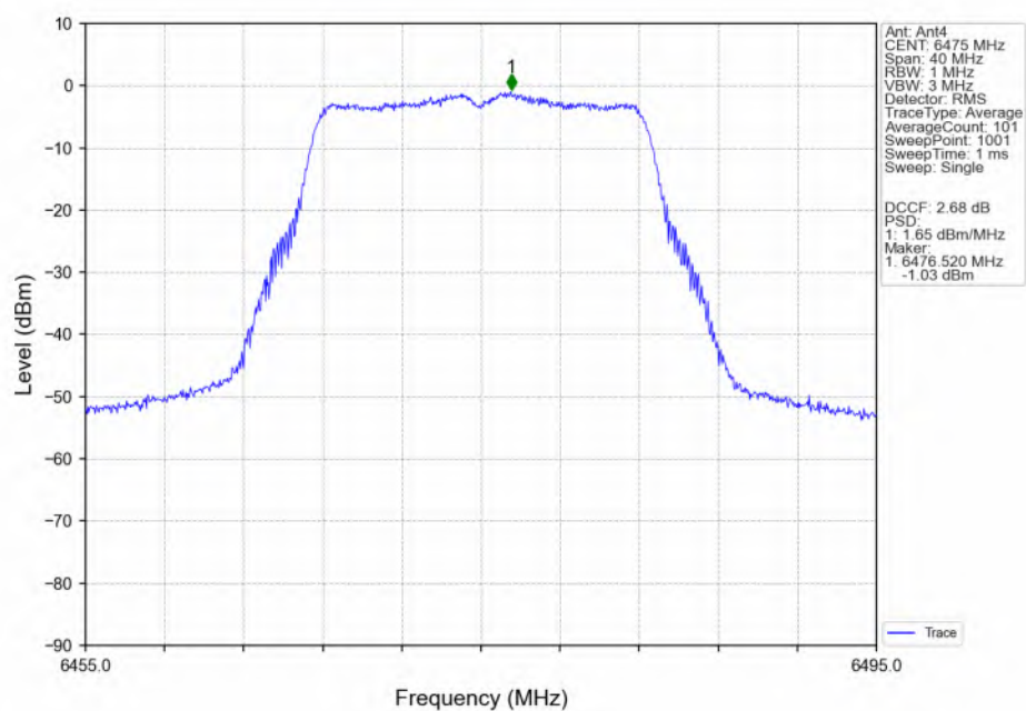
802.11a_MCH_6475MHz_Ant4_NTNV
