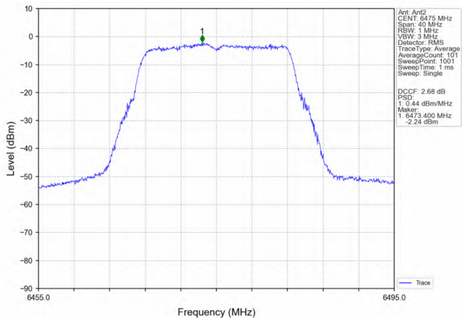
802.11a_MCH_6475MHz_Ant2_NTNV
