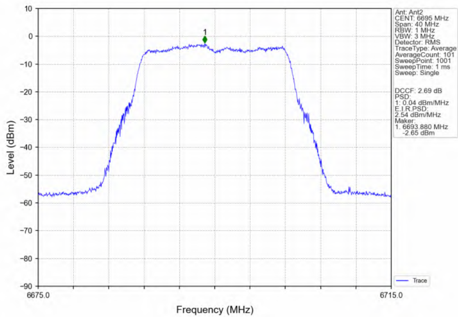
802.11a_MCH_6695MHz_Ant2_NTNV
