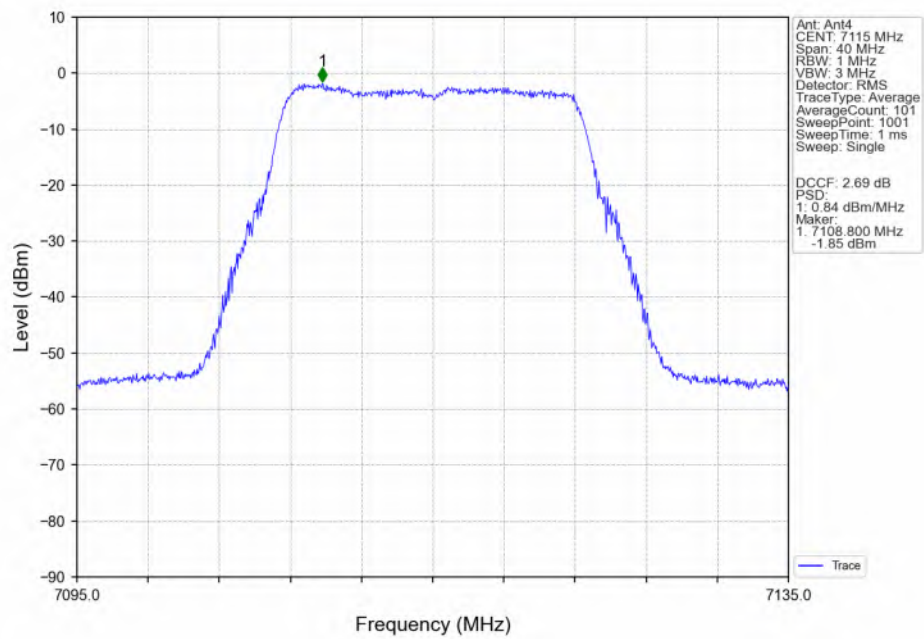
802.11a_HCH_7115MHz_Ant4_NTNV
