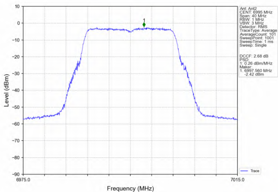
802.11a_MCH_6995MHz_Ant2_NTNV
