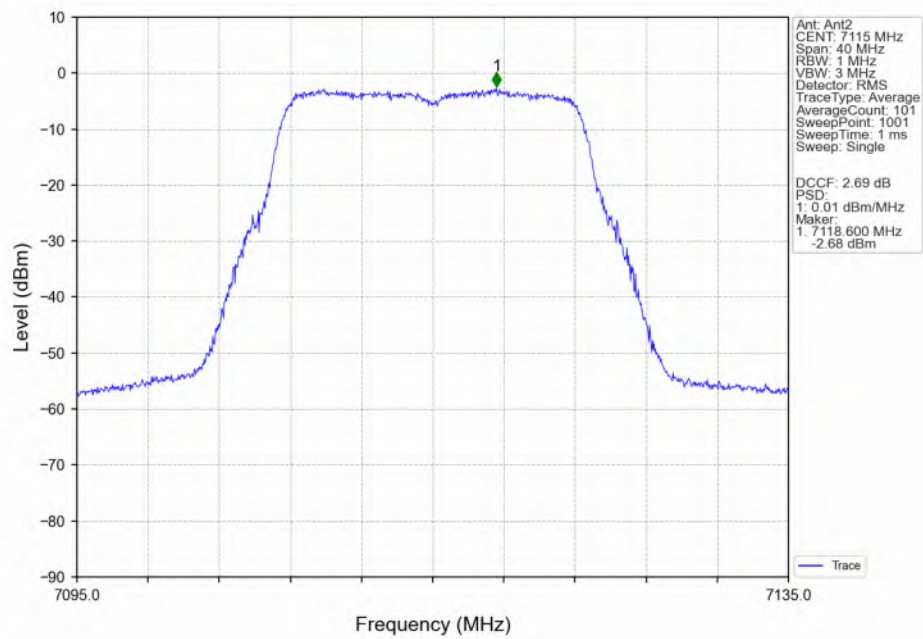
802.11a_HCH_7115MHz_Ant2_NTNV
