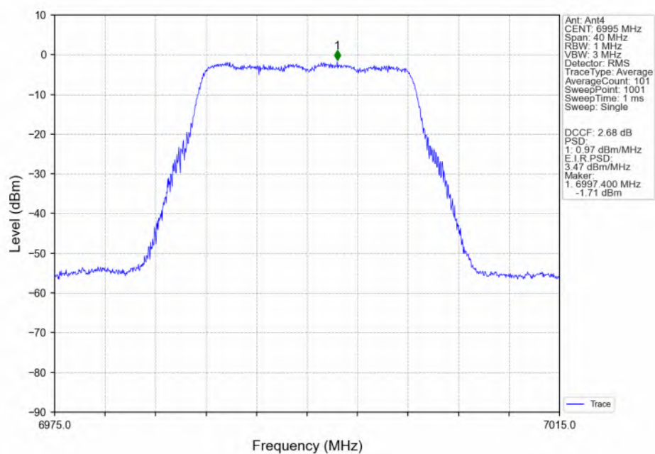
802.11a_MCH_6995MHz_Ant4_NTNV
