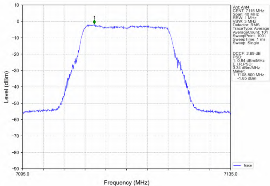
802.11a_HCH_7115MHz_Ant4_NTNV
