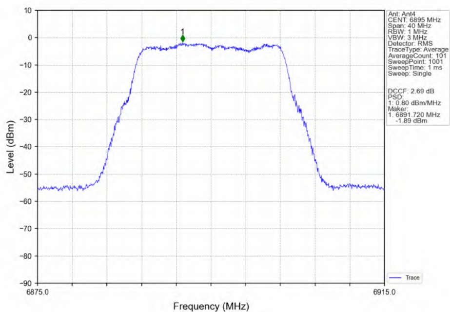
802.11a_LCH_6895MHz_Ant4_NTNV
