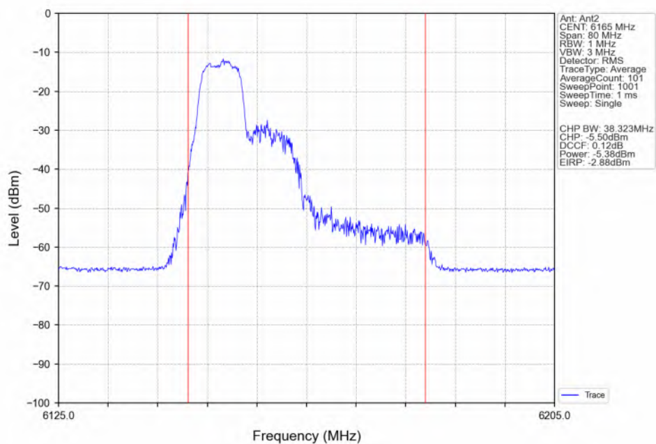
802.11be(EHT40)_MCH_6165MHz_26+52_/_Ant2_NTNV
