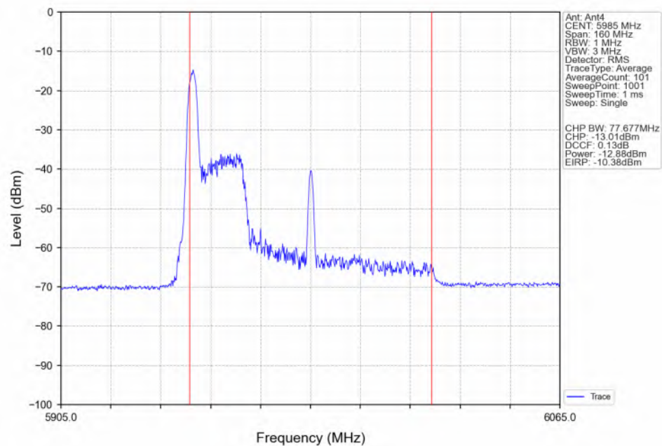
802.11be(EHT80) LCH_5985MHz_RU26_Left(0)_Ant4_NTNV
