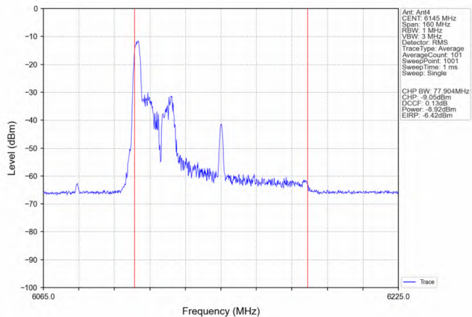
802.11be(EHT80)_MCH_6145MHz_RU26_Left(0)_Ant4_NTNV
