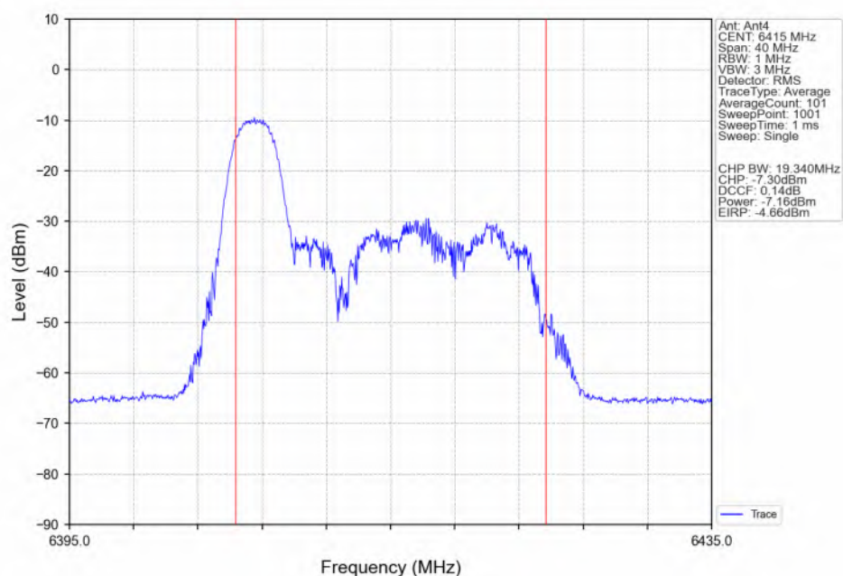
802.11be(EHT20)_HCH_6415MHz_RU26_Left(0)_Ant4_NTNV
