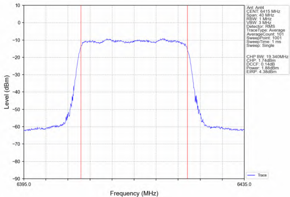
802.11be(EHT20)_HCH_6415MHz_RU242_Left(61)_Ant4_NTNV
