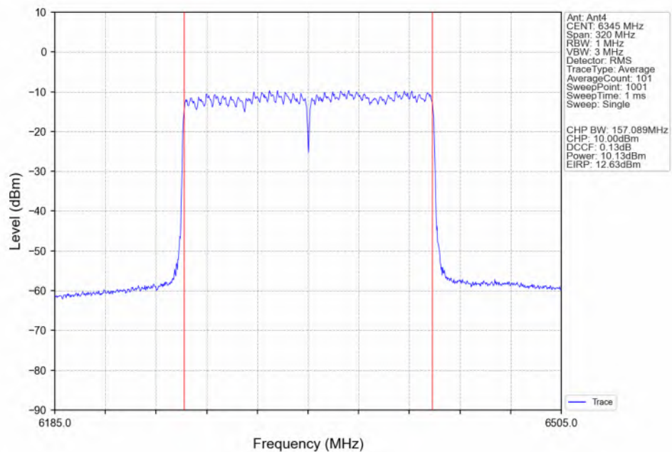
802.11be(EHT160)_HCH_6345MHz_2xRU996_Left(68)_Ant4_NTNV
