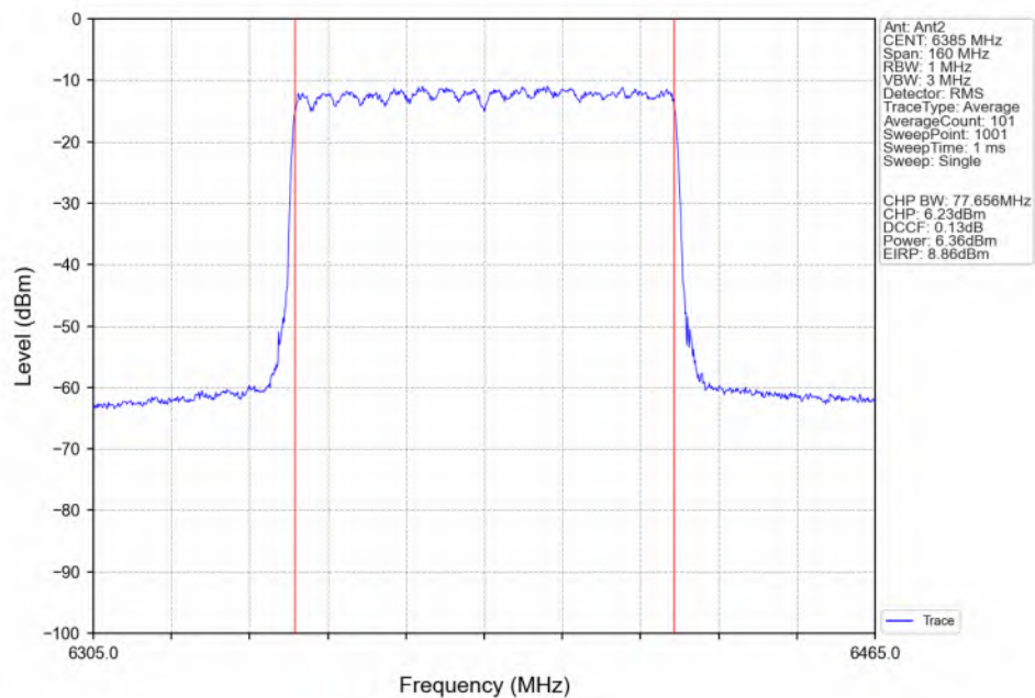
802.11be(EHT80)_HCH_6385MHz_RU996_Left(67)_Ant2_NTNV
