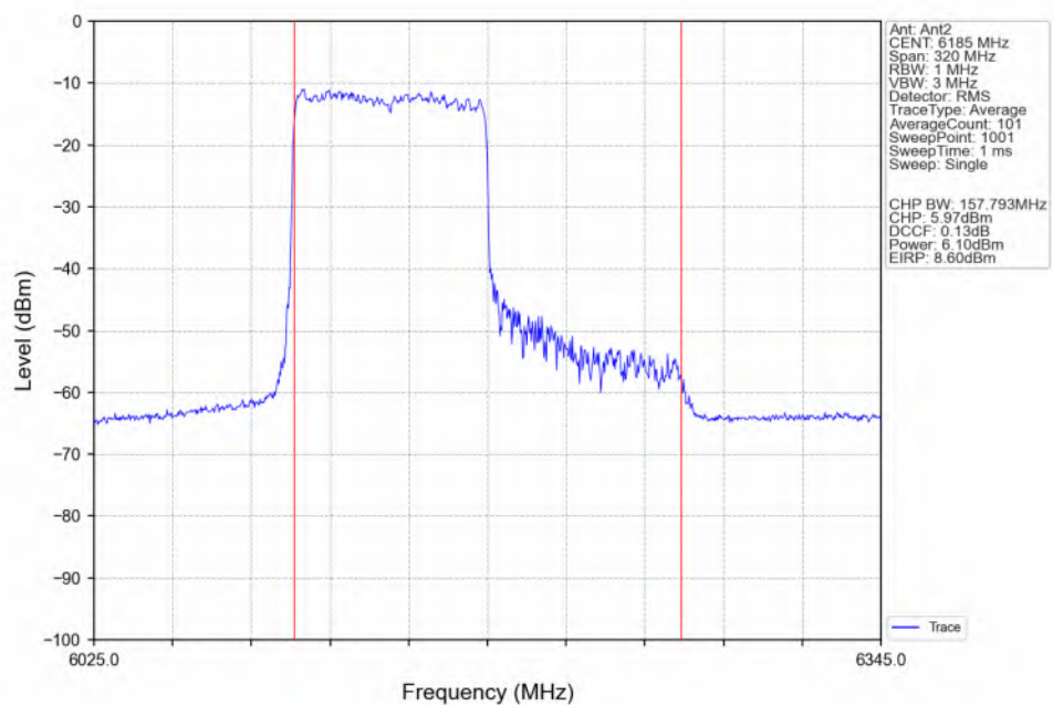
802.11be(EHT160)_MCH_6185MHz_RU996_Left(67)_Ant2_NTNV
