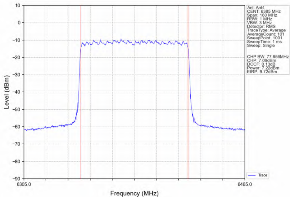
802.11be(EHT80)_HCH_6385MHz_RU996_Left(67)_Ant4_NTNV
