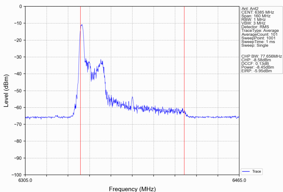
802.11be(EHT80)_HCH_6385MHz_RU26_Left(0)_Ant2_NTNV
