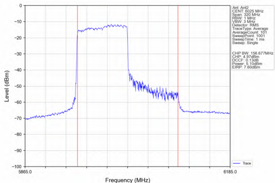
802.11be(EHT160)_LCH_6025MHz_RU996_Left(67)_Ant2_NTNV
