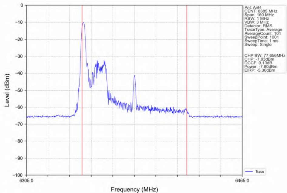
802.11be(EHT80)_HCH_6385MHz_RU26_Left(0)_Ant4_NTNV
