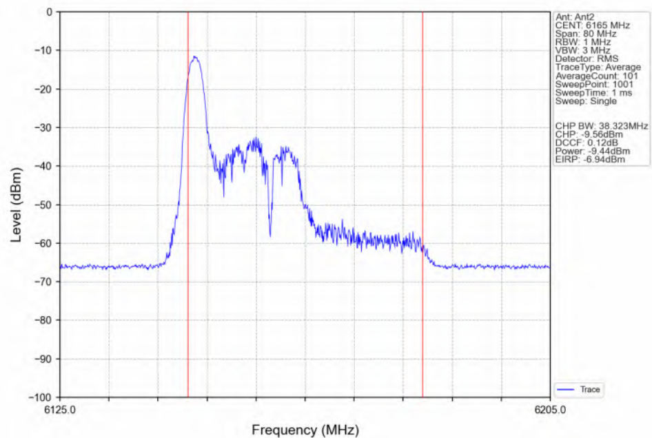
802.11be(EHT40)_MCH_6165MHz_RU26_Left(0)_Ant2_NTNV
