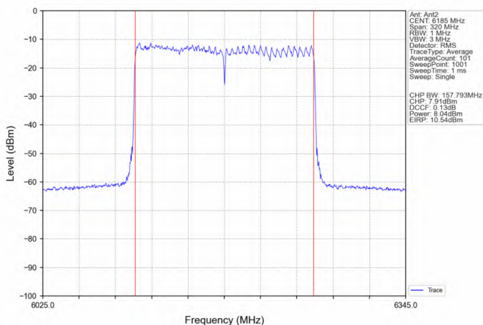
802.11be(EHT160)_MCH_6185MHz_2xRU996_Left(68)_Ant2_NTNV
