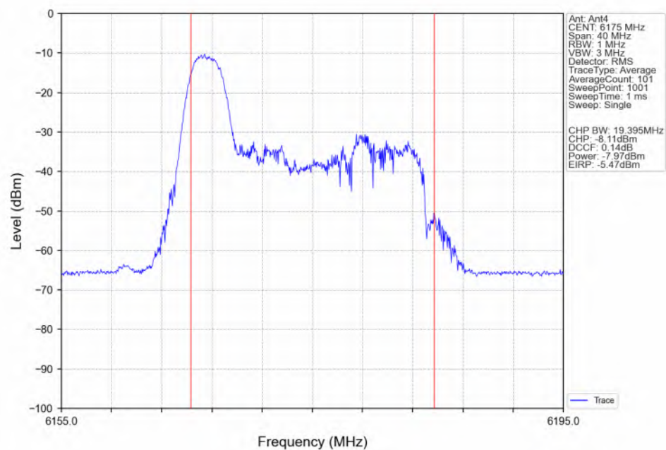
802.11be(EHT20)_MCH_6175MHz_RU26_Left(0)_Ant4_NTNV
