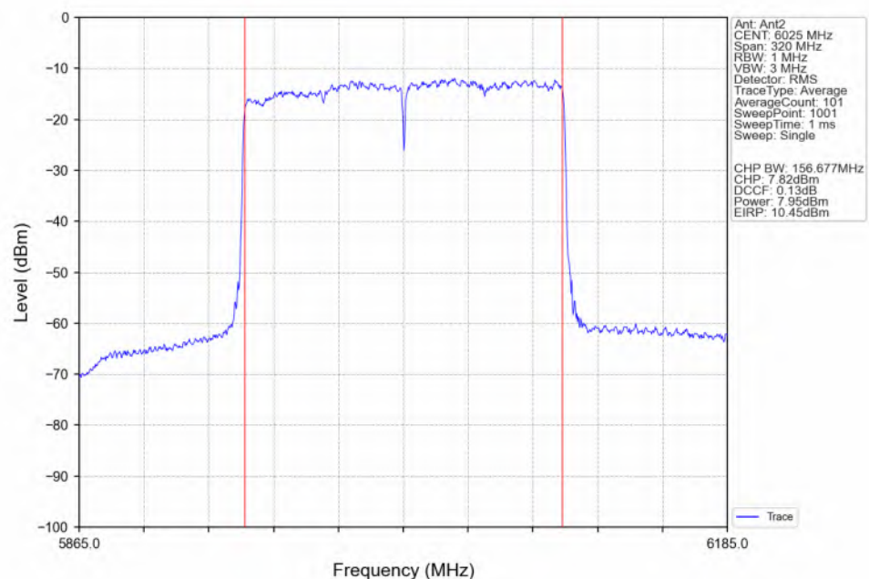
802.11be(EHT160)_LCH_6025MHz_2xRU996_Left(68)_Ant2_NTNV
