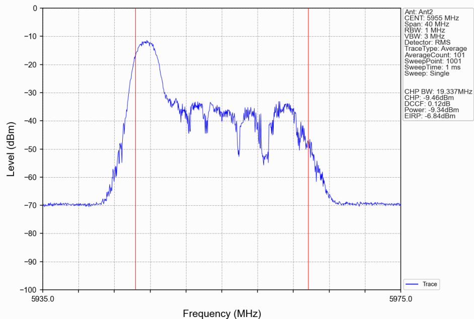
802.11be(EHT20)_LCH_5955MHz_RU26_Left(0)_Ant2_NTNV
