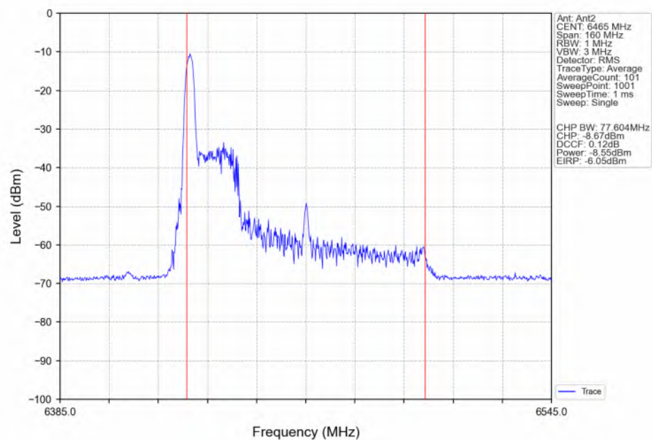
802.11be(EHT80) LCH_6465MHz_RU26_Left(0)_Ant2_NTNV
