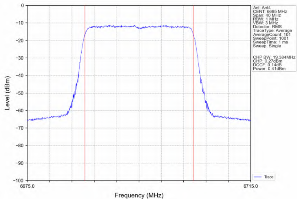
802.11be(EHT20)_MCH_6695MHz_RU242_Left(61)_Ant4_NTNV
