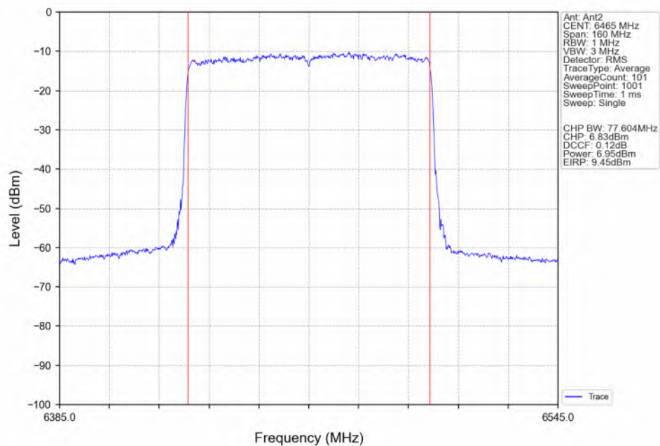
802.11be(EHT80) LCH_6465MHz_RU996_Left(67)_Ant2_NTNV
