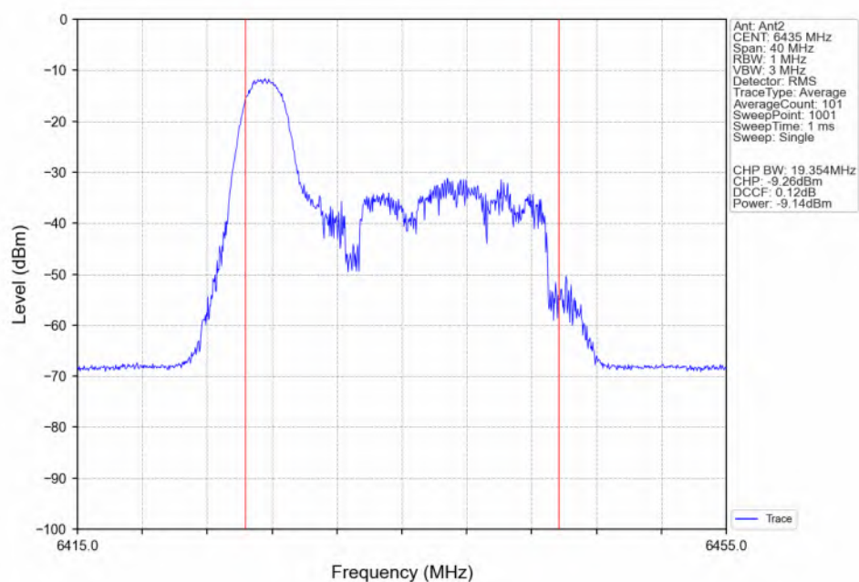
802.11be(EHT20)_LCH_6435MHz_RU26_Left(0)_Ant2_NTNV
