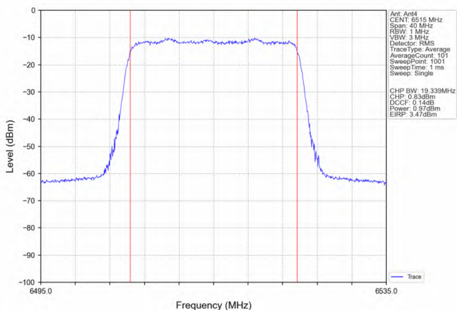
802.11be(EHT20)_HCH_6515MHz_RU242_Left(61)_Ant4_NTNV
