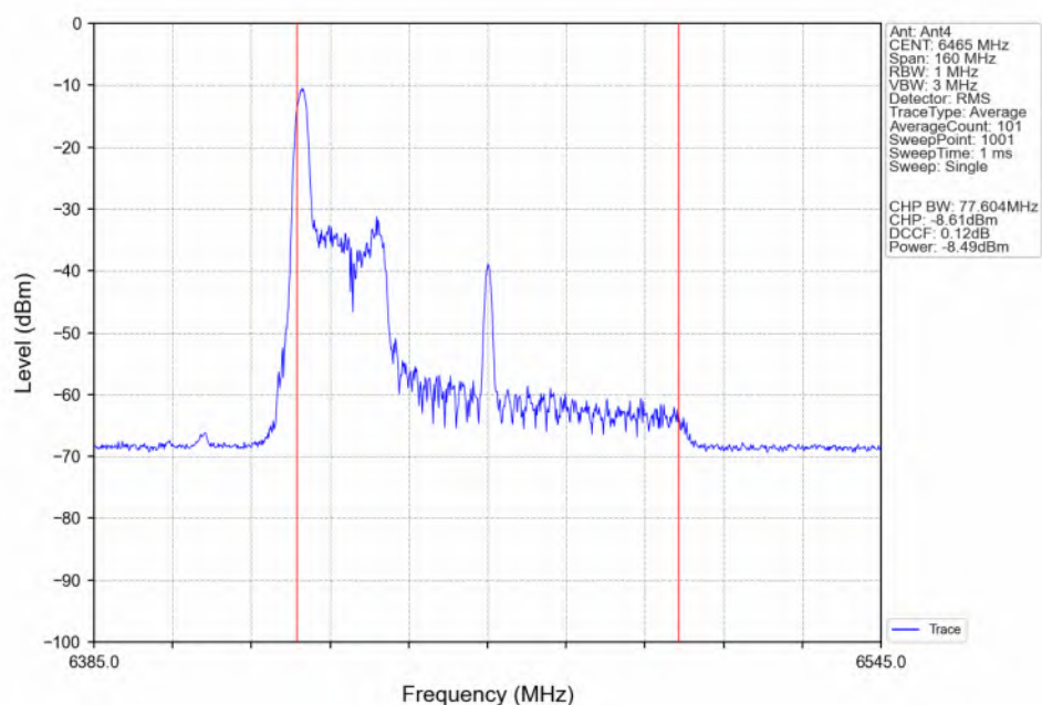
802.11be(EHT80) LCH_6465MHz_RU26_Left(0)_Ant4_NTNV
