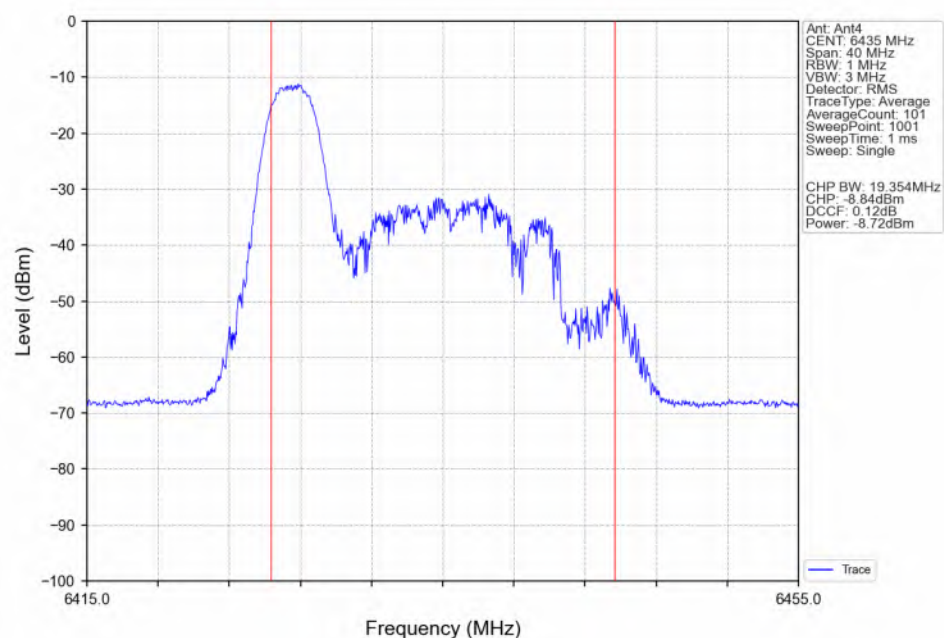
802.11be(EHT20) LCH_6435MHz_RU26_Left(0)_Ant4_NTNV
