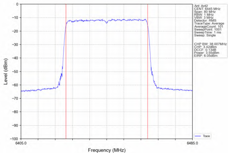
802.11be(EHT40) LCH_6445MHz_RU484_Left(65)_Ant2_NTNV
