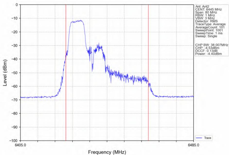
802.11be(EHT40)_LCH_6445MHz_26+52_/_Ant2_NTNV
