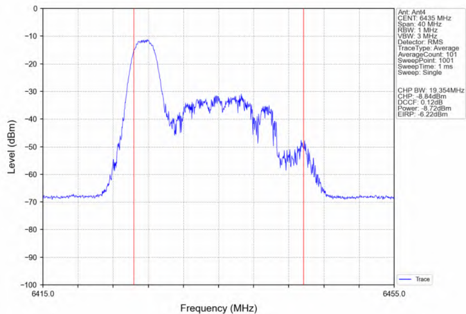
802.11be(EHT20) LCH_6435MHz_RU26_Left(0)_Ant4_NTNV
