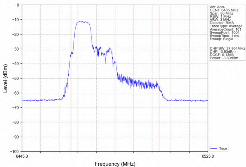
802.11be(EHT40)_MCH_6485MHz_26+52_/_Ant4_NTNV
