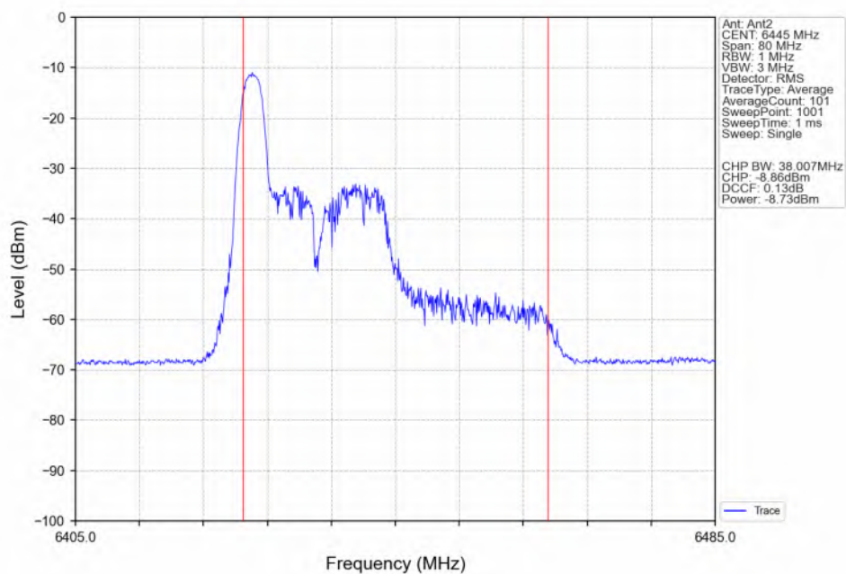
802.11be(EHT40) LCH_6445MHz_RU26_Left(0)_Ant2_NTNV
