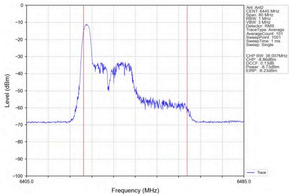
802.11be(EHT40) LCH_6445MHz_RU26_Left(0)_Ant2_NTNV
