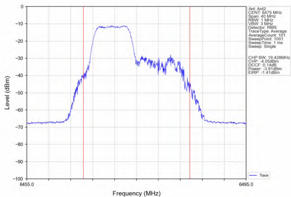
802.11be(EHT20)_MCH_6475MHz_26+52_ / Ant2_NTNV
