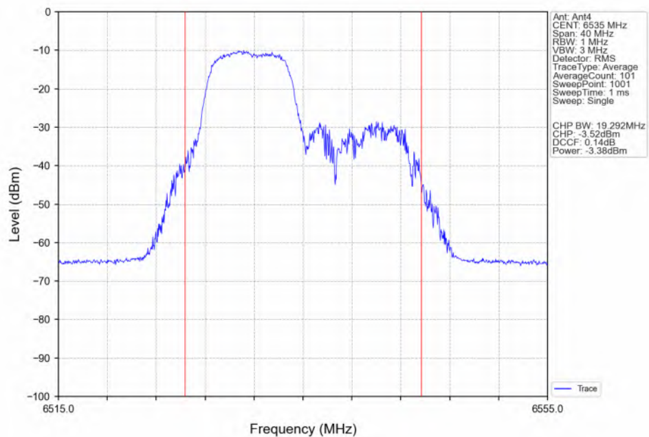
802.11be(EHT20)_LCH_6535MHz_26+52_ / Ant4_NTNV
