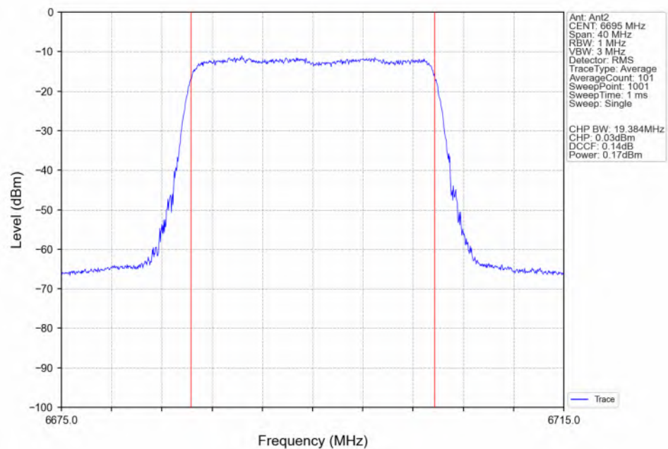
802.11be(EHT20)_MCH_6695MHz_RU242_Left(61)_Ant2_NTNV
