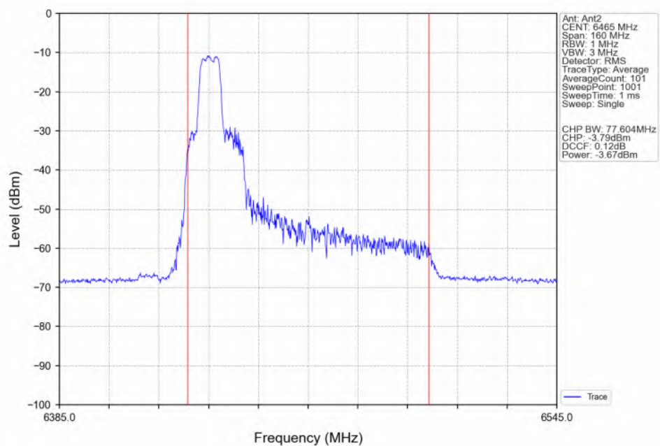
802.11be(EHT80)_LCH_6465MHz_26+52_/_Ant2_NTNV
