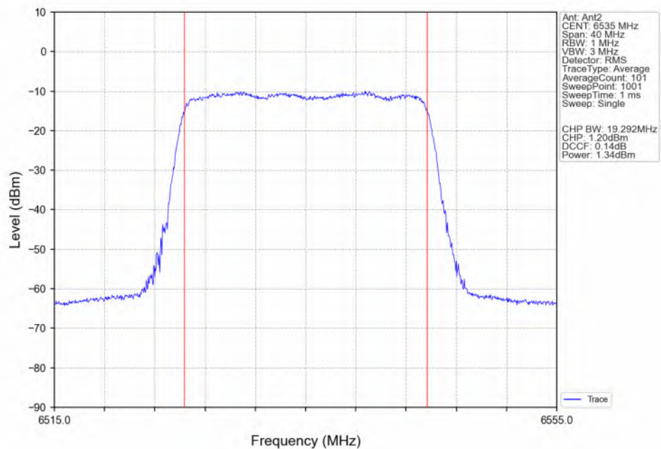
802.11be(EHT20) LCH_6535MHz_RU242_Left(61)_Ant2_NTNV
