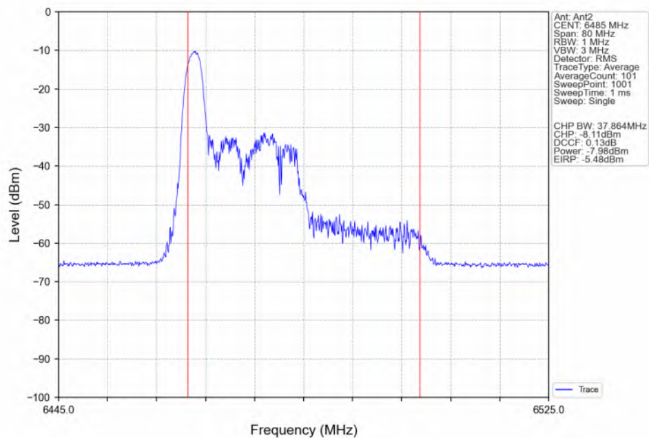
802.11be(EHT40)_MCH_6485MHz_RU26_Left(0)_Ant2_NTNV
