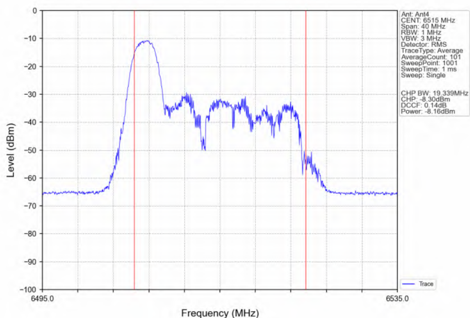
802.11be(EHT20)_HCH_6515MHz_RU26_Left(0)_Ant4_NTNV
