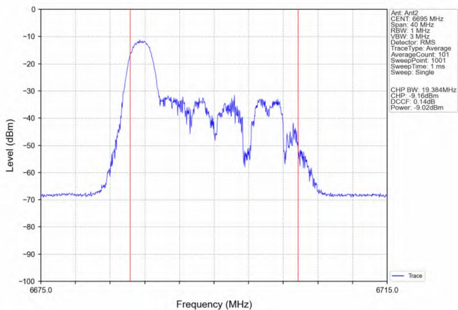
802.11be(EHT20)_MCH_6695MHz_RU26_Left(0)_Ant2_NTNV
