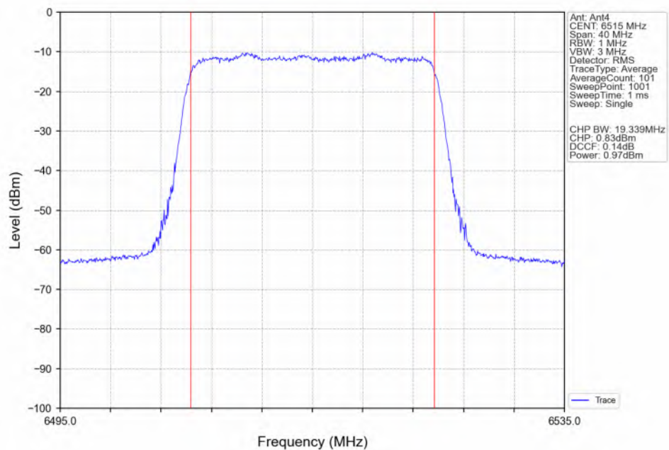
802.11be(EHT20)_HCH_6515MHz_RU242_Left(61)_Ant4_NTNV
