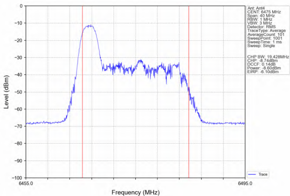
802.11be(EHT20)_MCH_6475MHz_RU26_Left(0)_Ant4_NTNV
