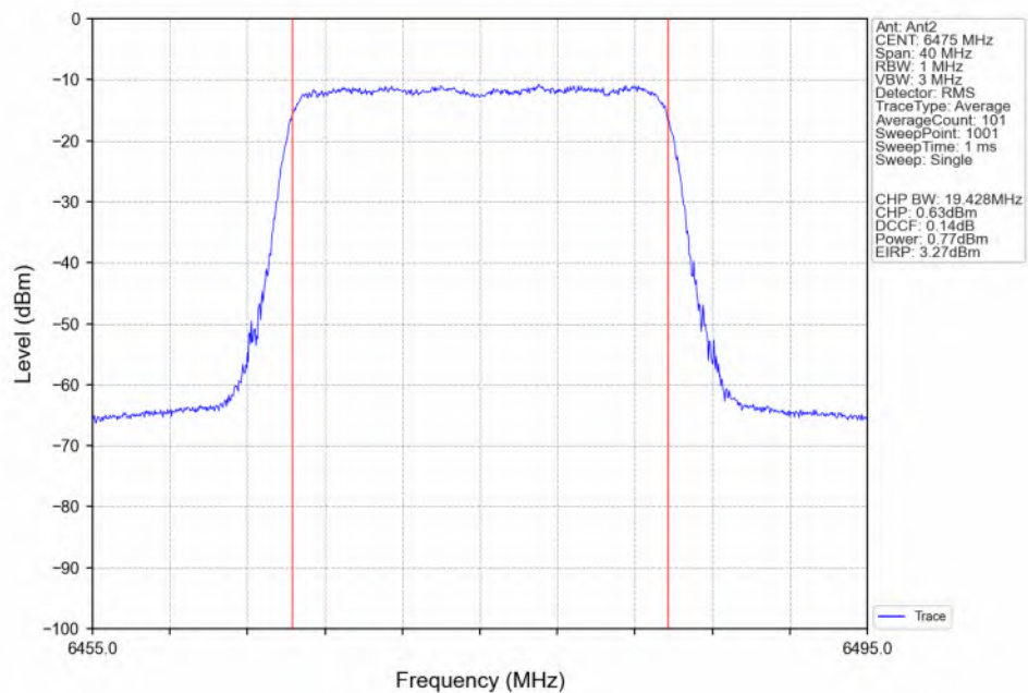
802.11be(EHT20)_MCH_6475MHz_RU242_Left(61)_Ant2_NTNV
