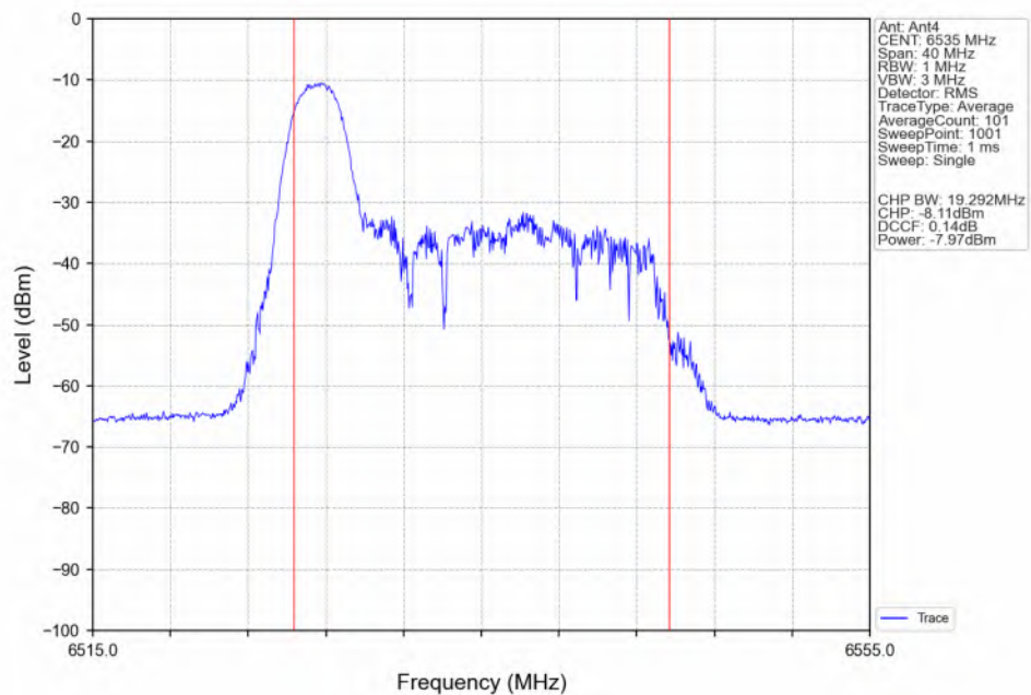
802.11be(EHT20) LCH_6535MHz_RU26_Left(0)_Ant4_NTNV
