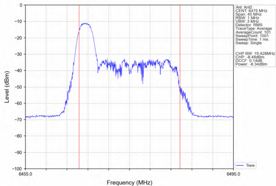
802.11be(EHT20)_MCH_6475MHz_RU26_Left(0)_Ant2_NTNV
