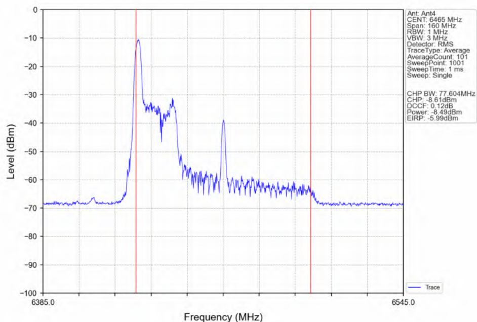
802.11be(EHT80) LCH_6465MHz_RU26_Left(0)_Ant4_NTNV
