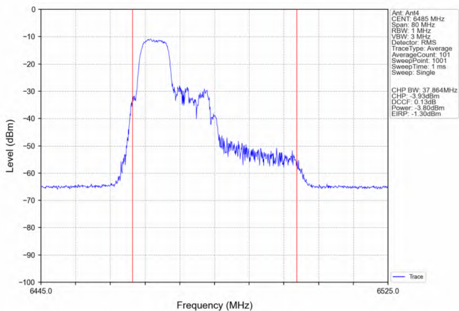
802.11be(EHT40) MCH 6485MHz 26+52 / Ant4_NTNV
