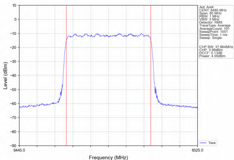
802.11be(EHT40)_MCH_6485MHz_RU484_Left(65)_Ant4_NTNV
