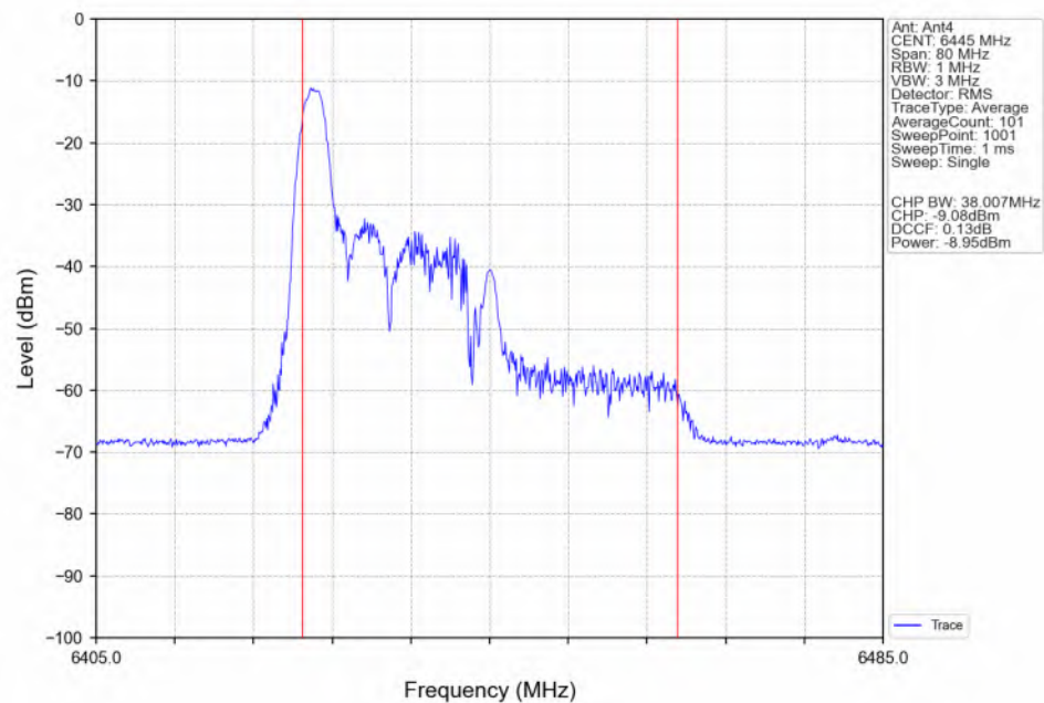
802.11be(EHT40) LCH_6445MHz_RU26_Left(0)_Ant4_NTNV
