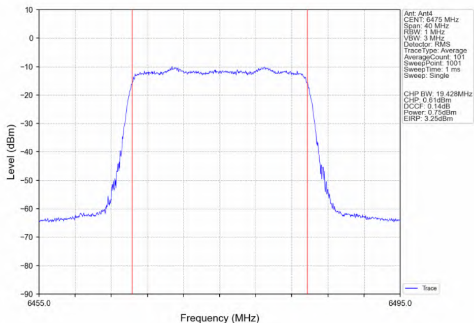
802.11be(EHT20)_MCH_6475MHz_RU242_Left(61)_Ant4_NTNV
