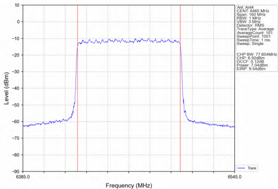
802.11be(EHT80) LCH_6465MHz_RU996_Left(67)_Ant4_NTNV
