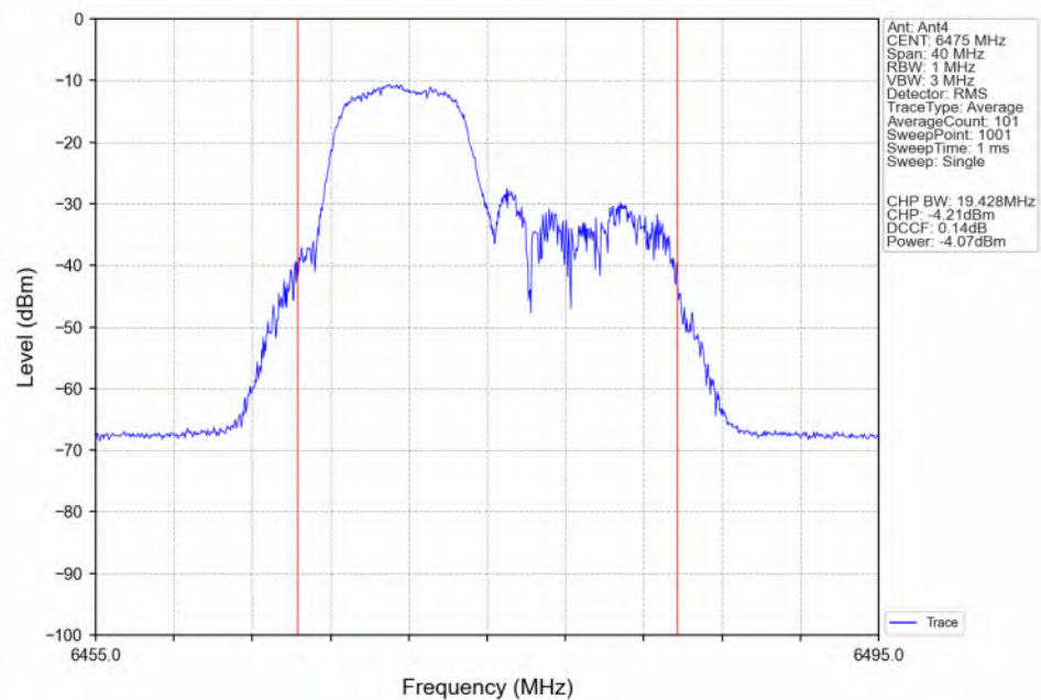
802.11be(EHT20)_MCH_6475MHz_26+52_/_Ant4_NTNV
