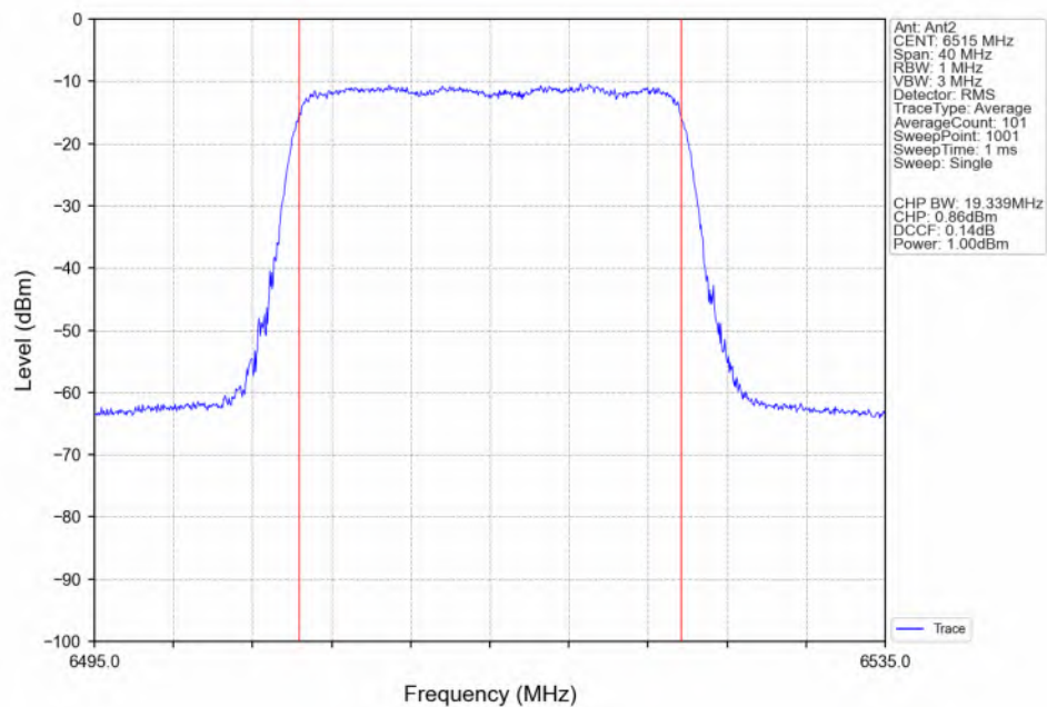
802.11be(EHT20)_HCH_6515MHz_RU242_Left(61)_Ant2_NTNV
