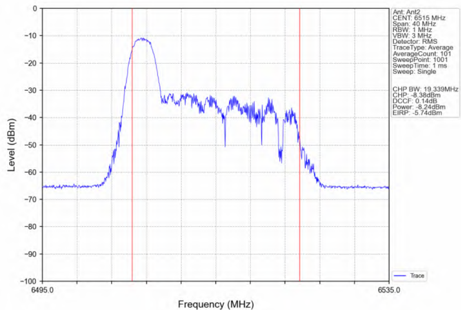
802.11be(EHT20)_HCH_6515MHz_RU26_Left(0)_Ant2_NTNV
