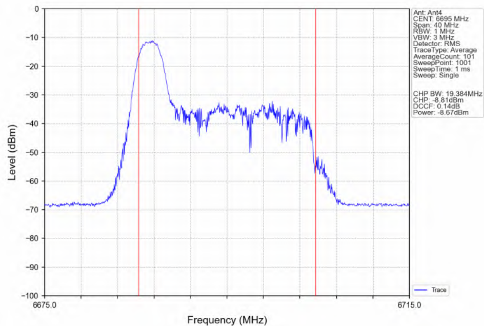
802.11be(EHT20)_MCH_6695MHz_RU26_Left(0)_Ant4_NTNV
