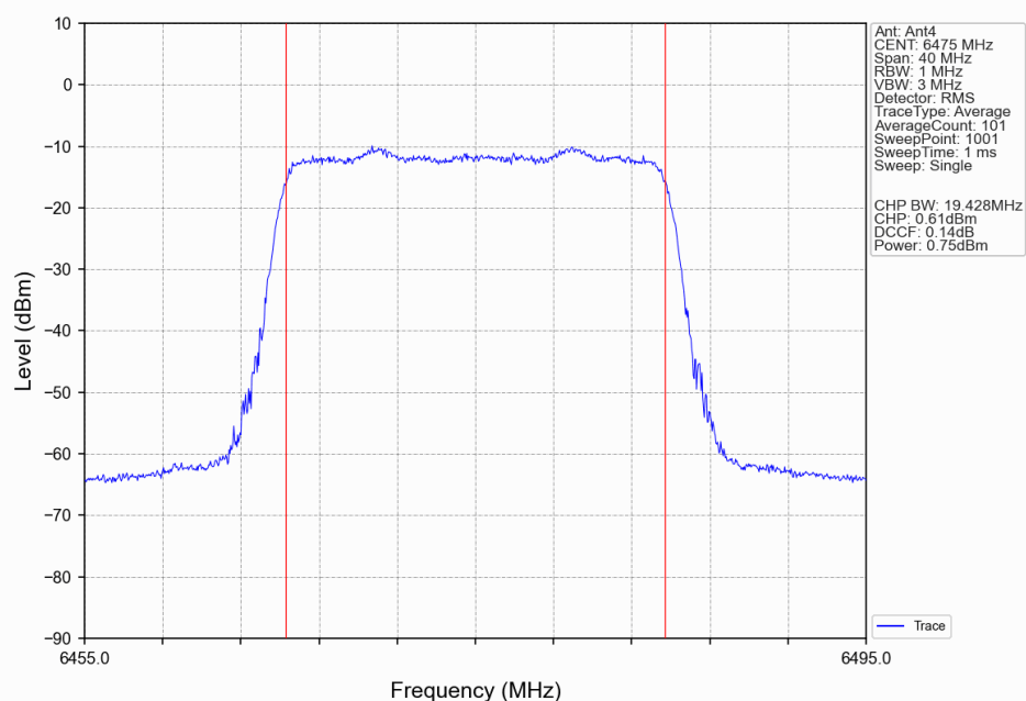
802.11be(EHT20)_MCH_6475MHz_RU242_Left(61)_Ant4_NTNV
