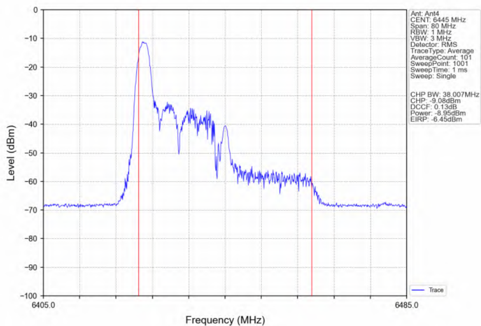
802.11be(EHT40) LCH_6445MHz_RU26_Left(0)_Ant4_NTNV
