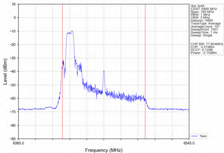
802.11be(EHT80)_LCH_6465MHz_26+52_ / Ant4_NTNV
