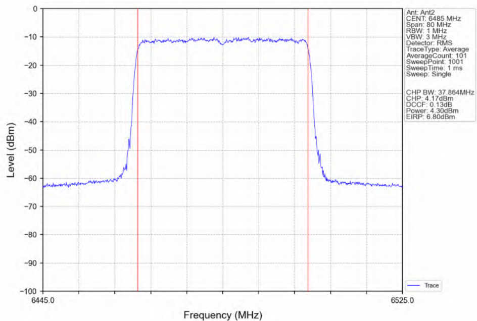
802.11be(EHT40)_MCH_6485MHz_RU484_Left(65)_Ant2_NTNV
