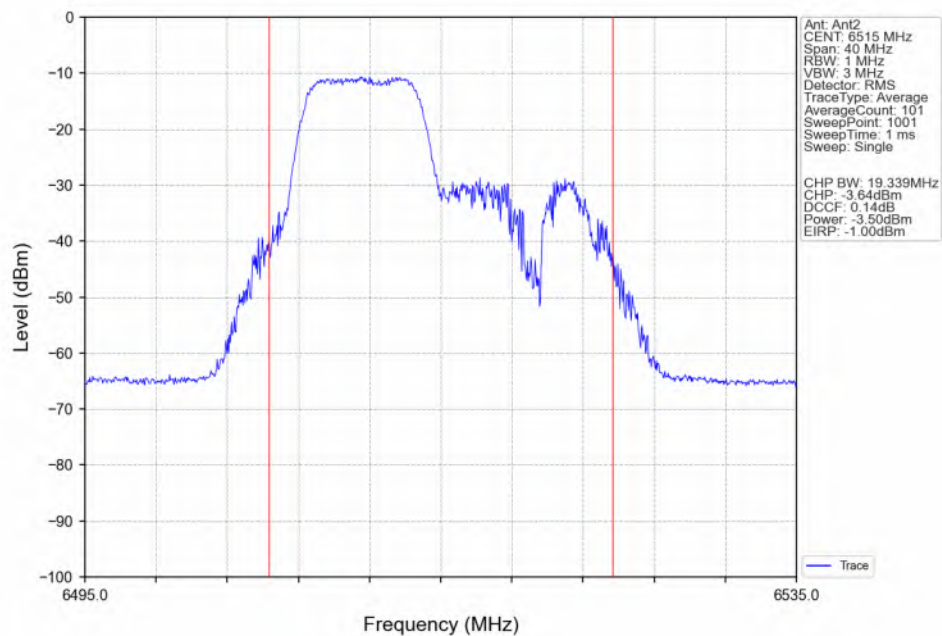
802.11be(EHT20)_HCH_6515MHz_26+52_ / Ant2_NTNV
