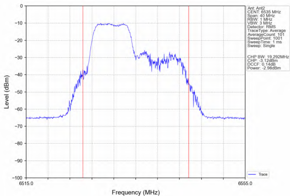
802.11be(EHT20)_LCH_6535MHz_26+52_ / Ant2_NTNV
