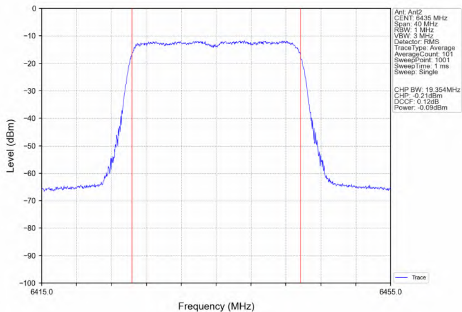
802.11be(EHT20) LCH_6435MHz_RU242_Left(61)_Ant2_NTNV
