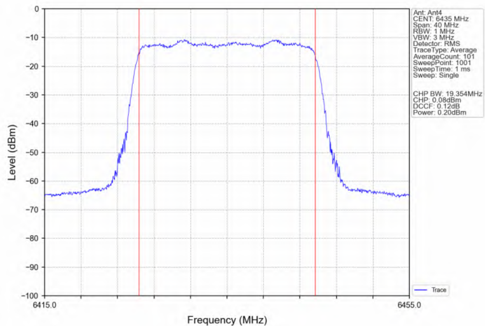
802.11be(EHT20) LCH_6435MHz_RU242_Left(61)_Ant4_NTNV
