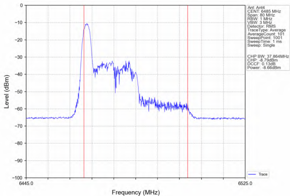
802.11be(EHT40)_MCH_6485MHz_RU26_Left(0)_Ant4_NTNV
