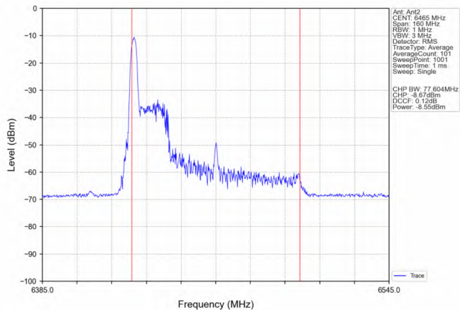
802.11be(EHT80) LCH_6465MHz_RU26_Left(0)_Ant2_NTNV
