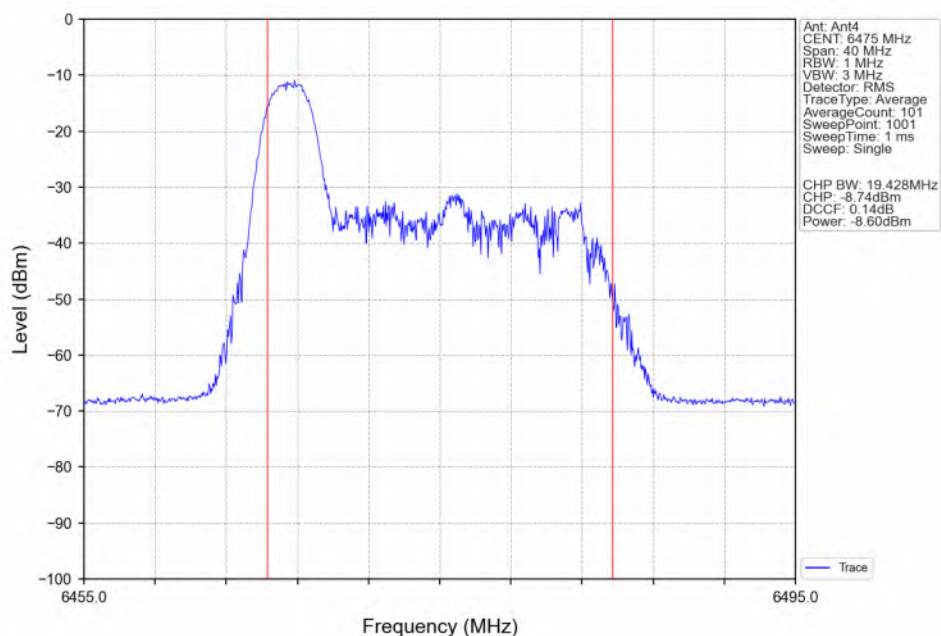
802.11be(EHT20)_MCH_6475MHz_RU26_Left(0)_Ant4_NTNV
