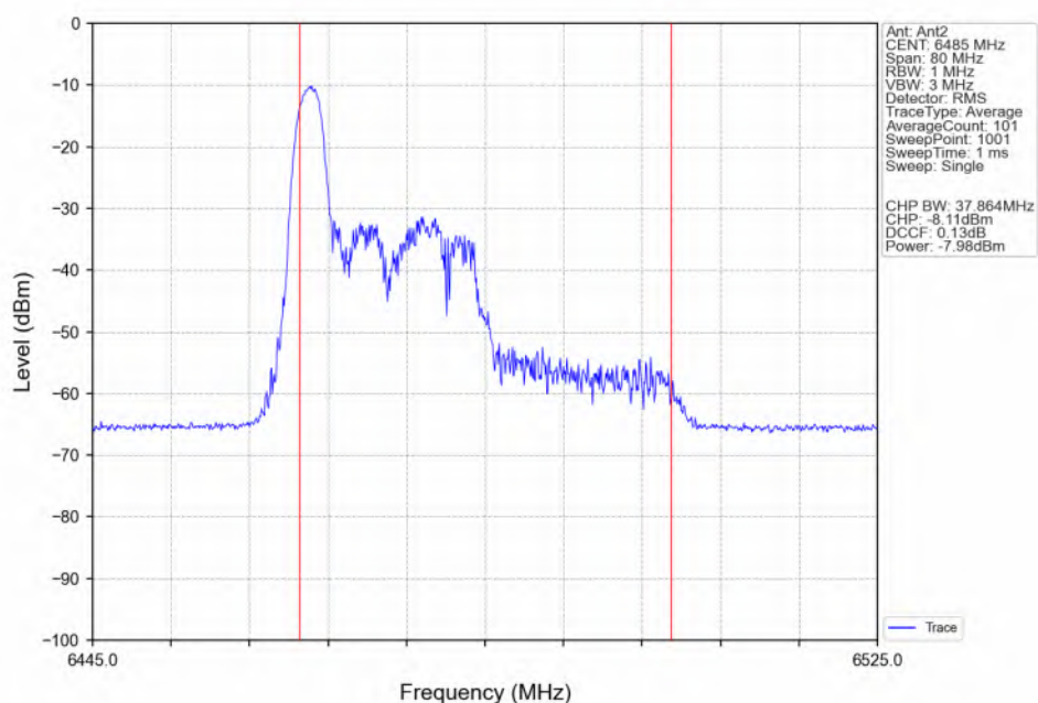
802.11be(EHT40)_MCH_6485MHz_RU26_Left(0)_Ant2_NTNV
