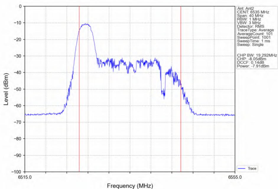
802.11be(EHT20)_LCH_6535MHz_RU26_Left(0)_Ant2_NTNV
