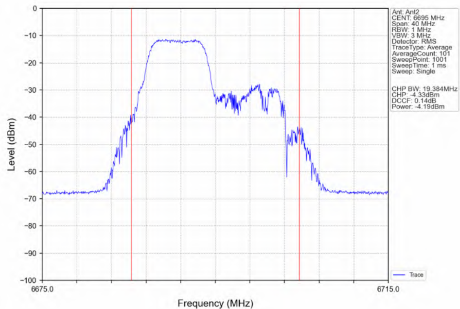
802.11be(EHT20)_MCH_6695MHz_26+52_ / Ant2_NTNV
