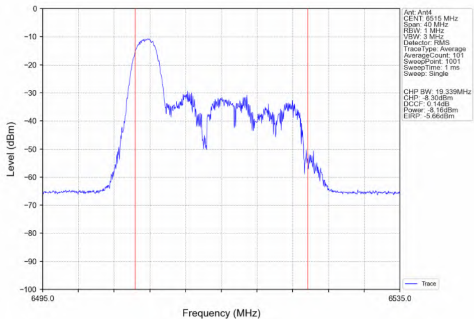
802.11be(EHT20)_HCH_6515MHz_RU26_Left(0)_Ant4_NTNV
