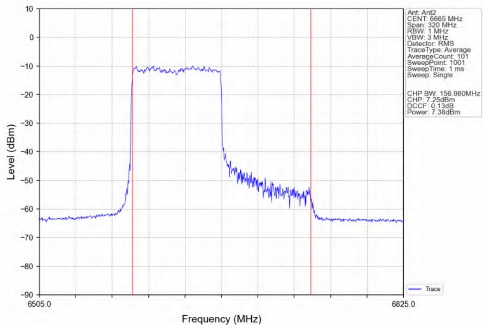
802.11be(EHT160)_MCH_6665MHz_RU996_Left(67)_Ant2_NTNV
