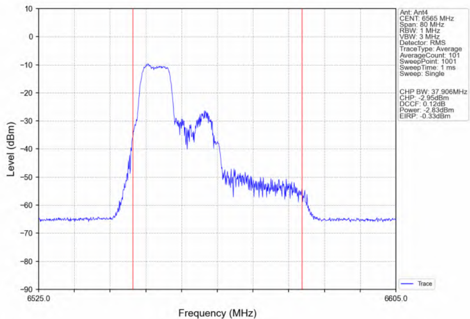
802.11be(EHT40)_LCH_6565MHz_26+52 / Ant4_NTNV
