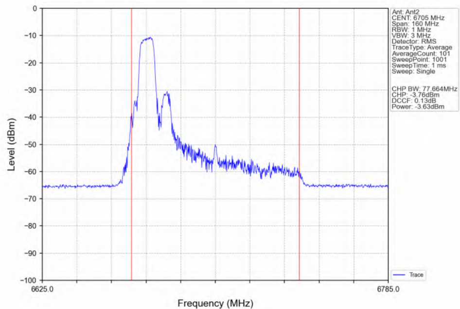
802.11be(EHT80)_MCH_6705MHz_26+52_ / Ant2_NTNV
