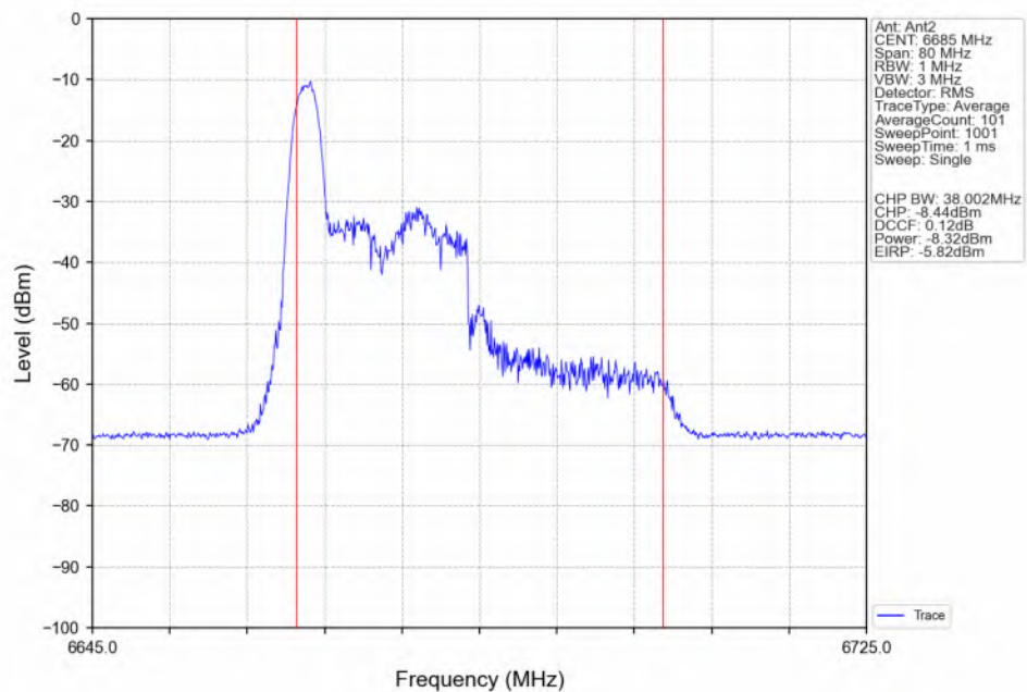
802.11be(EHT40)_MCH_6685MHz_RU26_Left(0)_Ant2_NTNV
