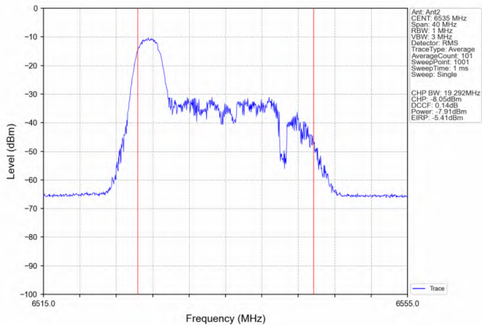
802.11be(EHT20)_LCH_6535MHz_RU26_Left(0)_Ant2_NTNV
