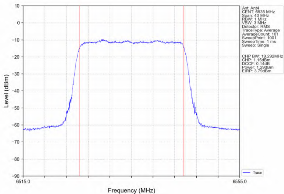
802.11be(EHT20) LCH_6535MHz_RU242_Left(61)_Ant4_NTNV
