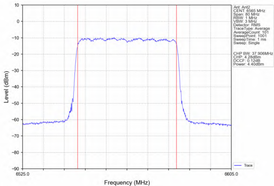
802.11be(EHT40) LCH_6565MHz_RU484_Left(65)_Ant2_NTNV
