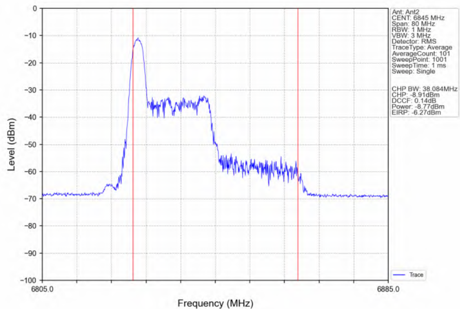
802.11be(EHT40)_HCH_6845MHz_RU26_Left(0)_Ant2_NTNV
