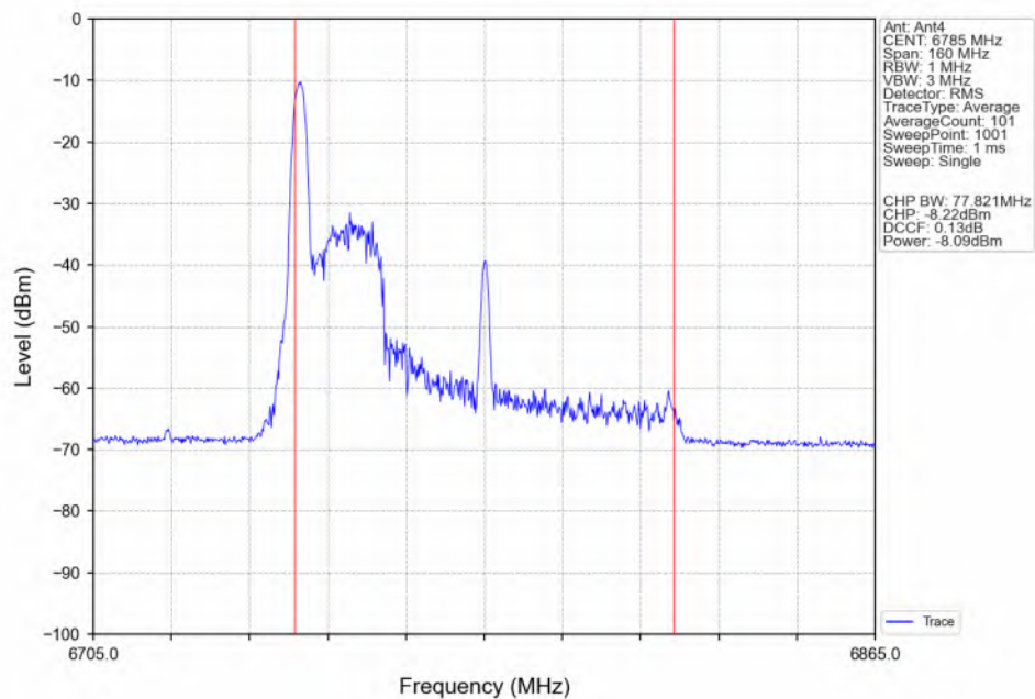
802.11be(EHT80)_HCH_6785MHz_RU26_Left(0)_Ant4_NTNV
