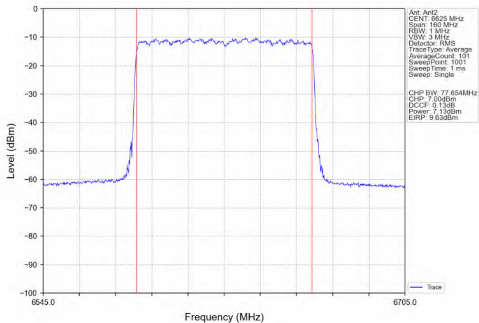
802.11be(EHT80) LCH_6625MHz_RU996_Left(67)_Ant2_NTNV
