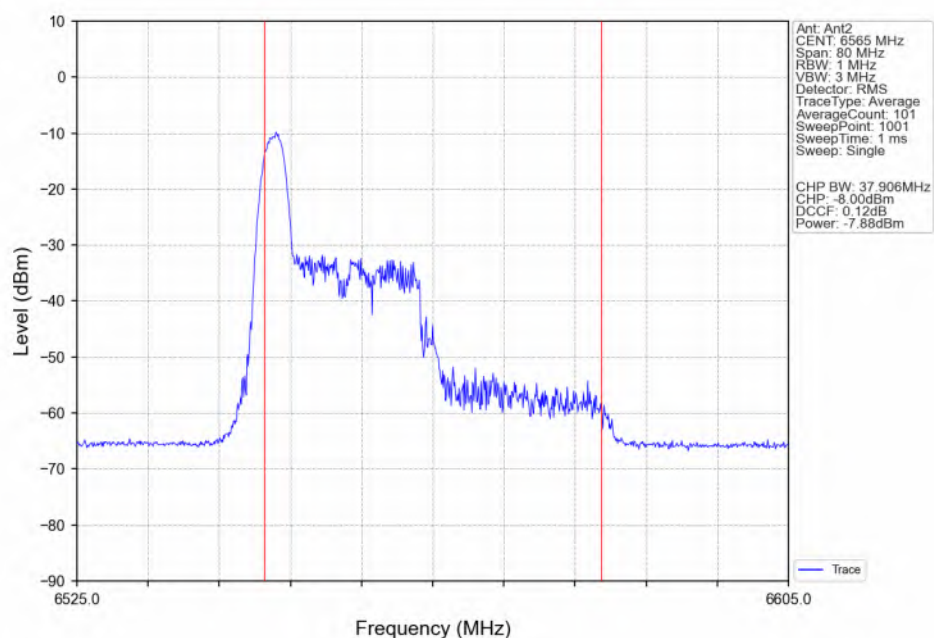
802.11be(EHT40) LCH_6565MHz_RU26_Left(0)_Ant2_NTNV
