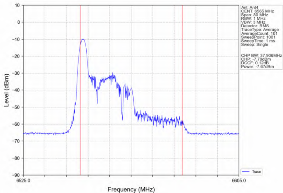
802.11be(EHT40) LCH_6565MHz_RU26_Left(0)_Ant4_NTNV
