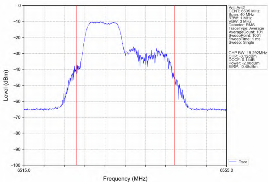
802.11be(EHT20)_LCH_6535MHz_26+52_ / Ant2_NTNV
