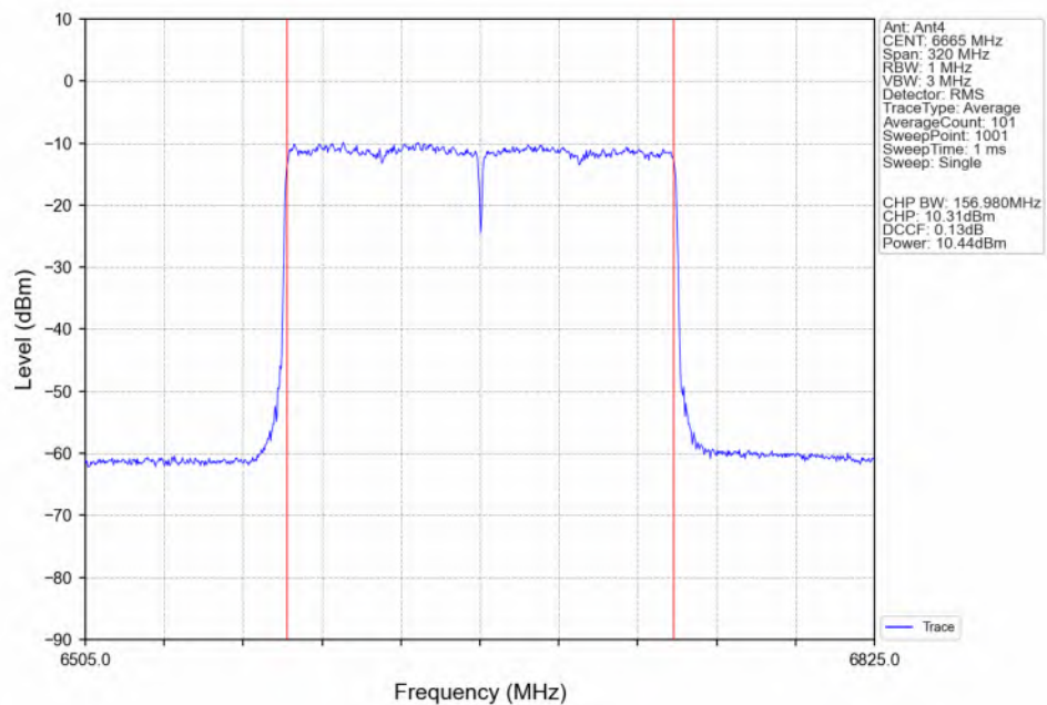
802.11be(EHT160)_MCH_6665MHz_2xRU996_Left(68)_Ant4_NTNV
