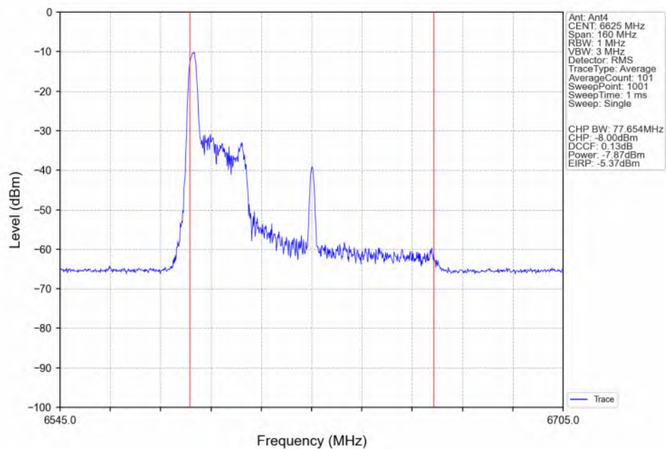
802.11be(EHT80) LCH_6625MHz_RU26_Left(0)_Ant4_NTNV
