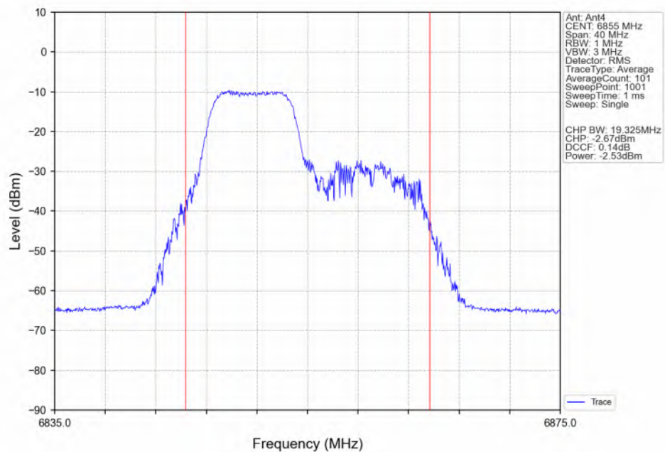
802.11be(EHT20) HCH 6855MHz 26+52 / Ant4_NTNV
