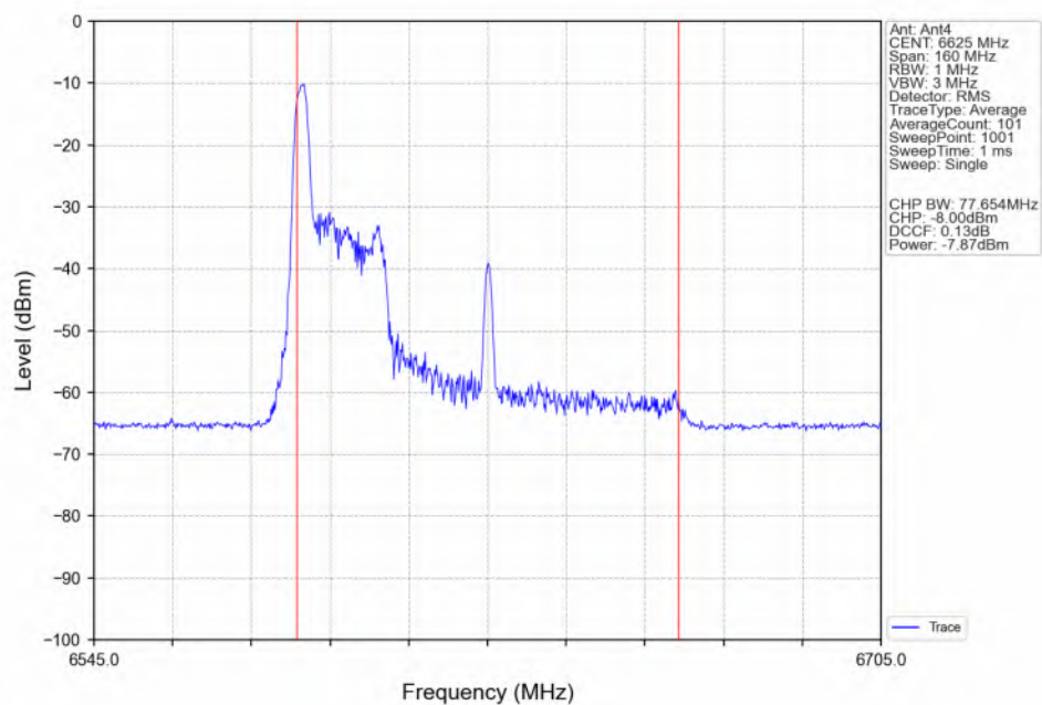
802.11be(EHT80) LCH_6625MHz_RU26_Left(0)_Ant4_NTNV
