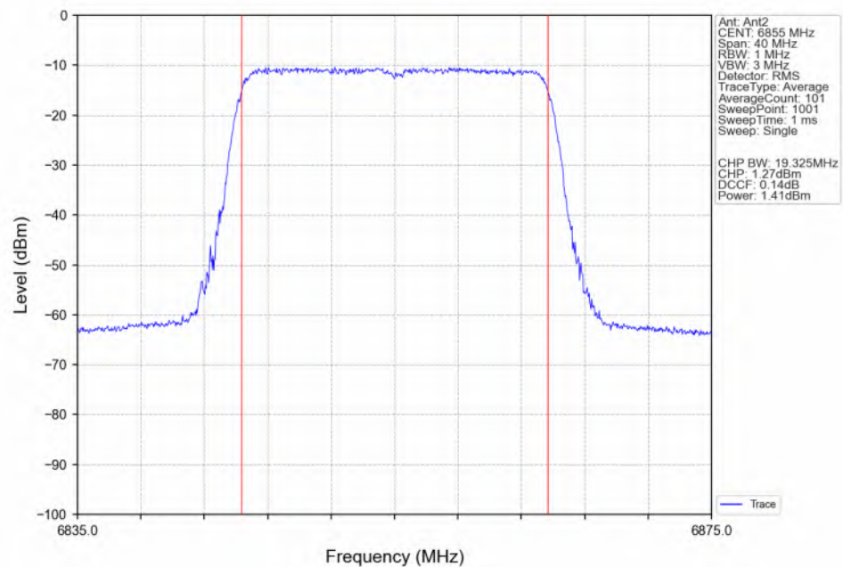
802.11be(EHT20)_HCH_6855MHz_RU242_Left(61)_Ant2_NTNV
