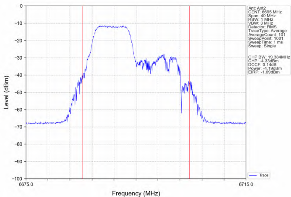
802.11be(EHT20)_MCH_6695MHz_26+52_/_Ant2_NTNV
