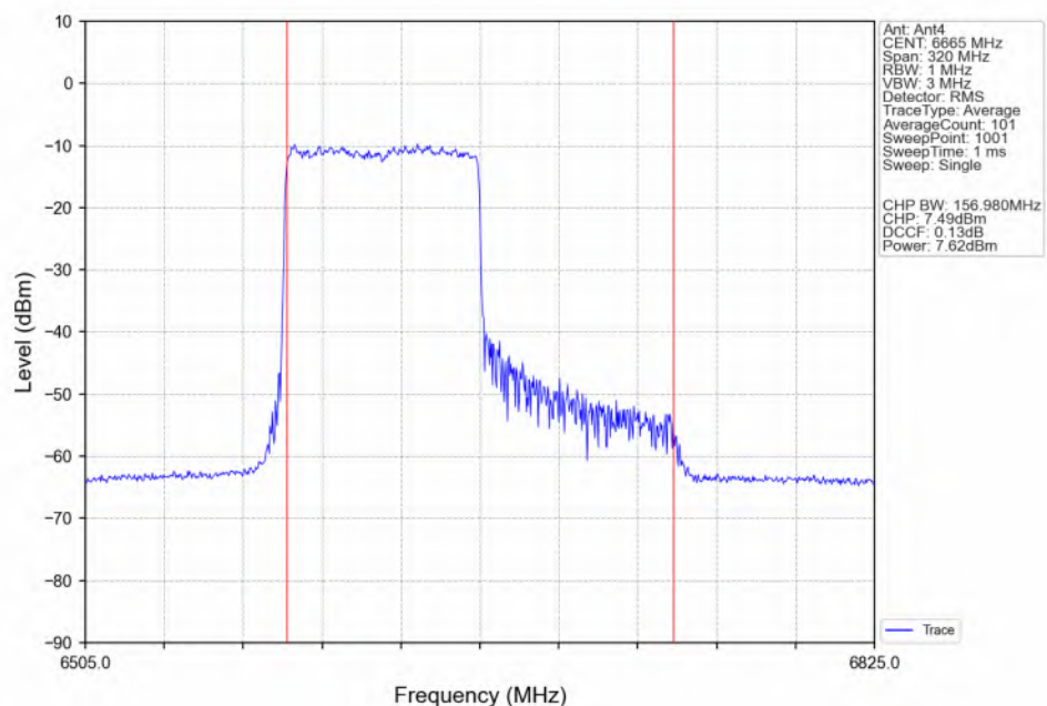
802.11be(EHT160)_MCH_6665MHz_RU996_Left(67)_Ant4_NTNV
