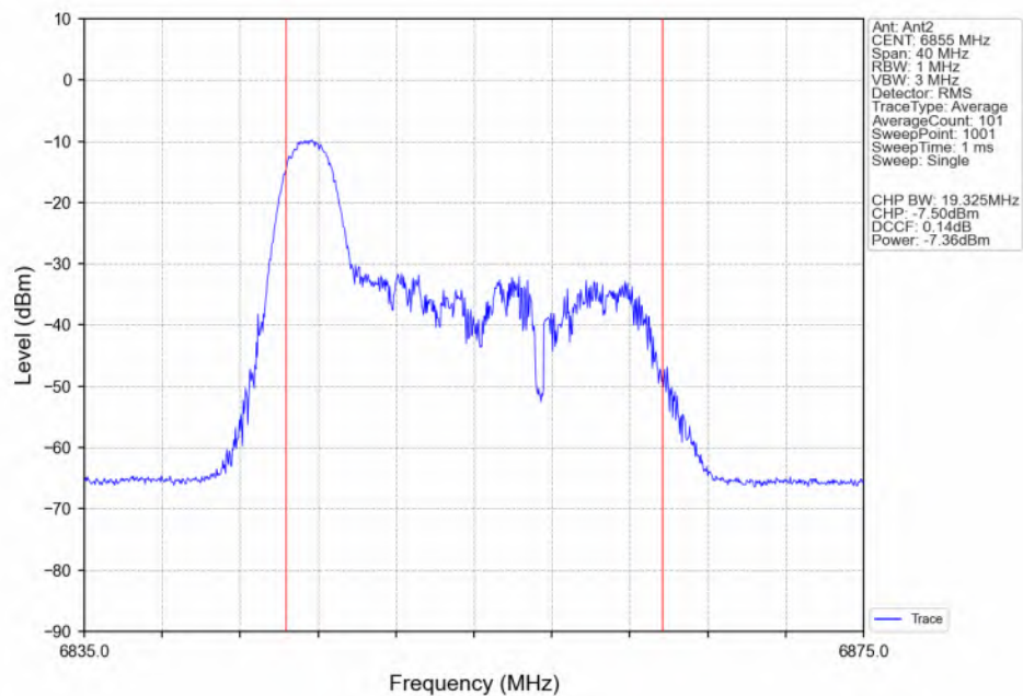
802.11be(EHT20)_HCH_6855MHz_RU26_Left(0)_Ant2_NTNV
