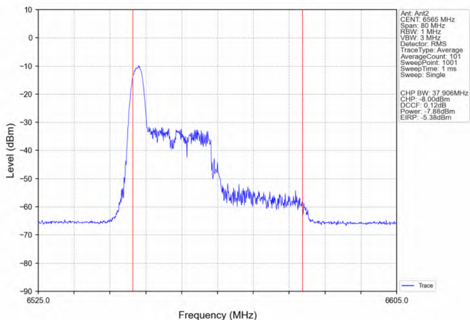
802.11be(EHT40) LCH_6565MHz_RU26_Left(0)_Ant2_NTNV
