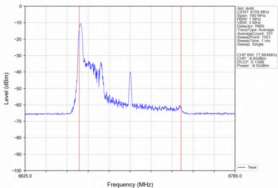
802.11be(EHT80)_MCH_6705MHz_RU26_Left(0)_Ant4_NTNV
