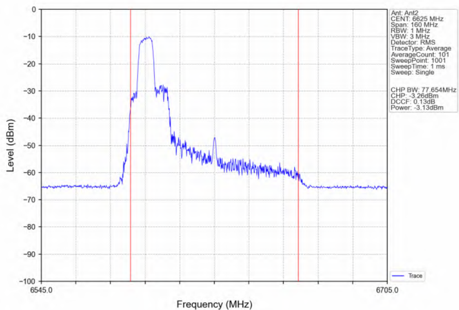
802.11be(EHT80)_LCH_6625MHz_26+52_/_Ant2_NTNV
