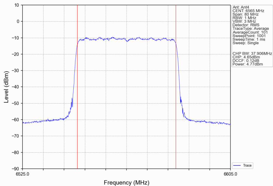
802.11be(EHT40) LCH_6565MHz_RU484_Left(65)_Ant4_NTNV
