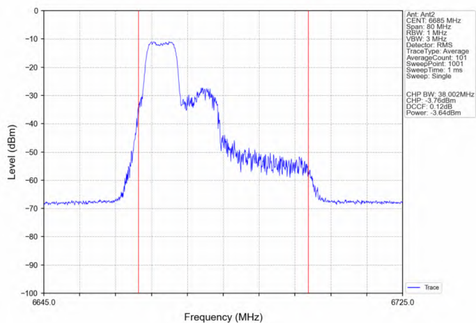
802.11be(EHT40) MCH 6685MHz 26+52 / Ant2_NTNV
