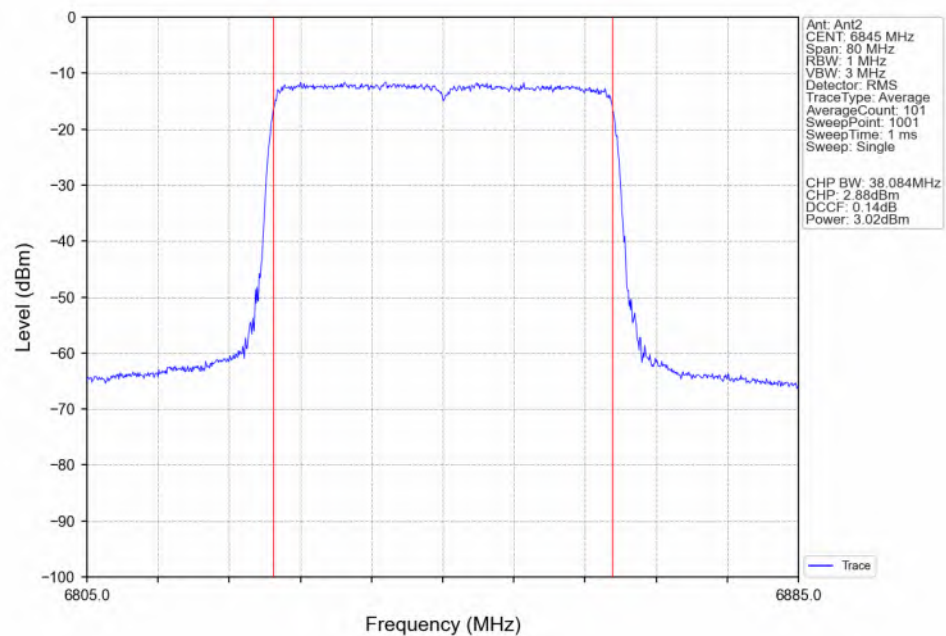
802.11be(EHT40)_HCH_6845MHz_RU484_Left(65)_Ant2_NTNV
