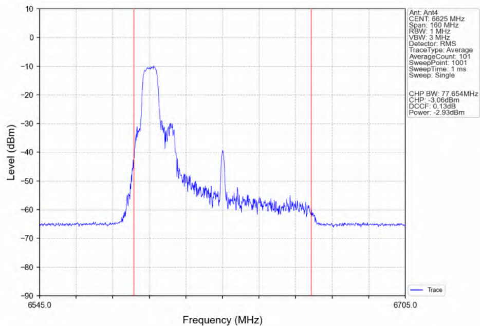
802.11be(EHT80)_LCH_6625MHz_26+52_ / Ant4_NTNV
