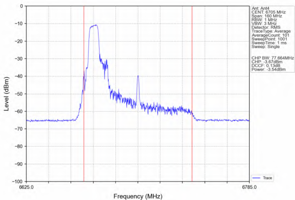
802.11be(EHT80) MCH 6705MHz 26+52 / Ant4_NTNV
