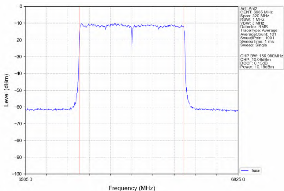
802.11be(EHT160)_MCH_6665MHz_2xRU996_Left(68)_Ant2_NTNV
