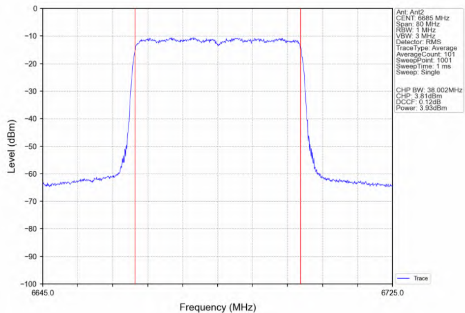
802.11be(EHT40)_MCH_6685MHz_RU484_Left(65)_Ant2_NTNV
