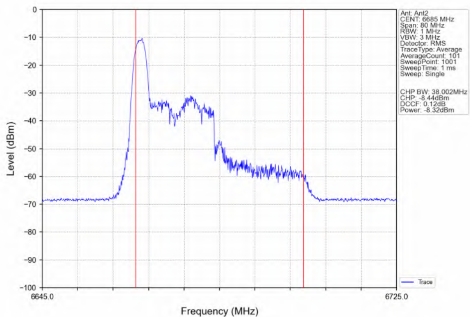
802.11be(EHT40)_MCH_6685MHz_RU26_Left(0)_Ant2_NTNV
