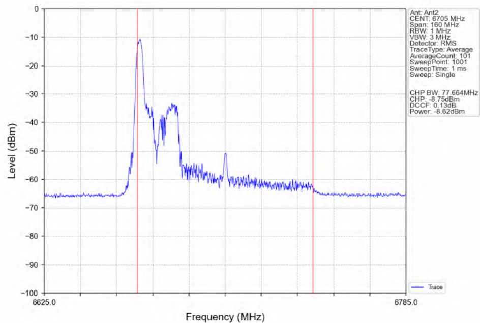
802.11be(EHT80)_MCH_6705MHz_RU26_Left(0)_Ant2_NTNV
