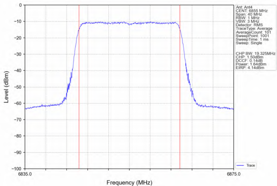
802.11be(EHT20)_HCH_6855MHz_RU242_Left(61)_Ant4_NTNV
