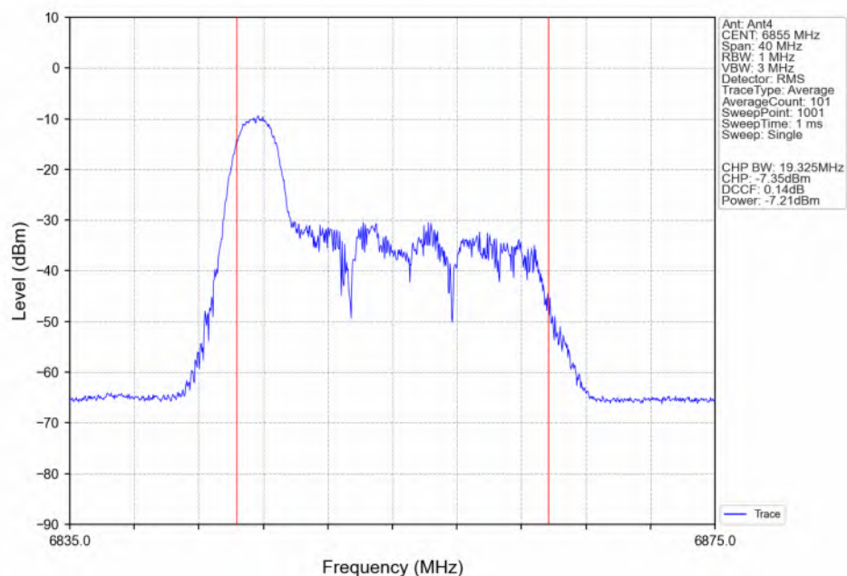
802.11be(EHT20)_HCH_6855MHz_RU26_Left(0)_Ant4_NTNV
