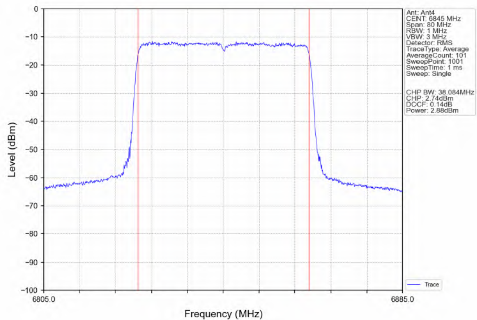
802.11be(EHT40)_HCH_6845MHz_RU484_Left(65)_Ant4_NTNV
