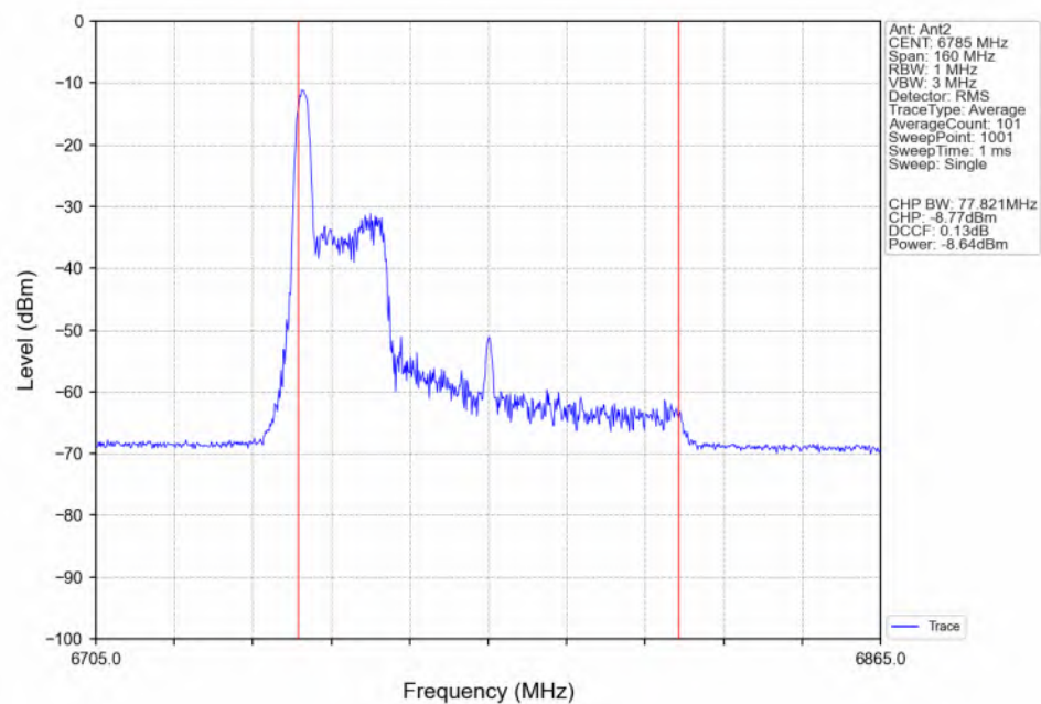
802.11be(EHT80)_HCH_6785MHz_RU26_Left(0)_Ant2_NTNV
