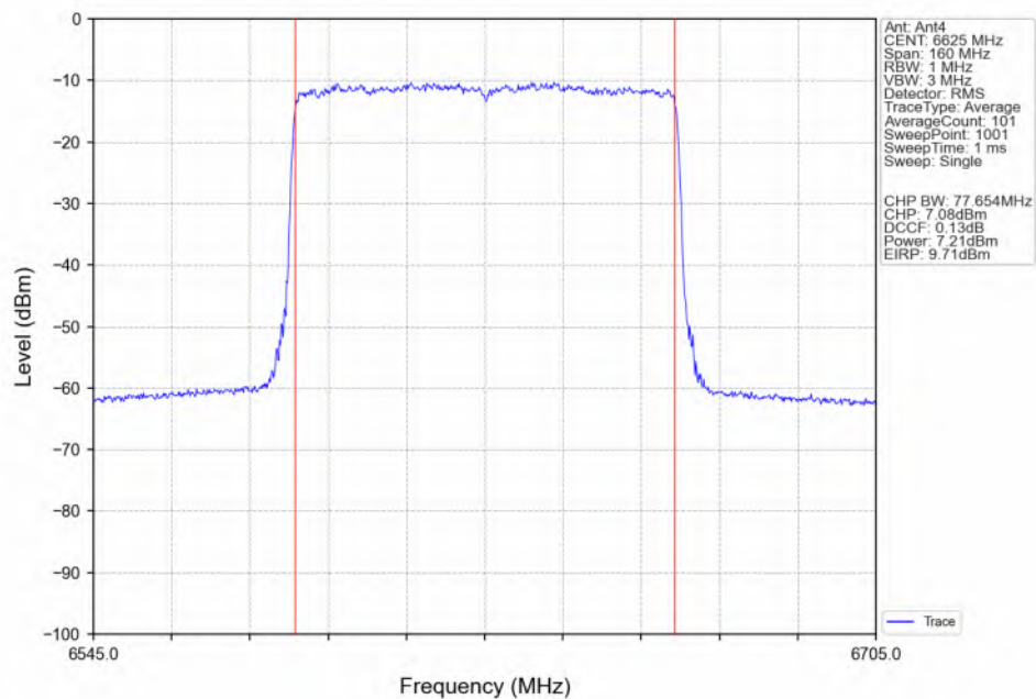
802.11be(EHT80) LCH_6625MHz_RU996_Left(67)_Ant4_NTNV
