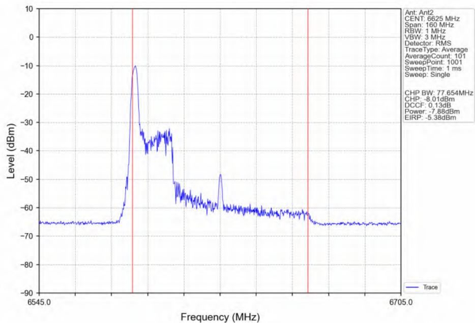
802.11be(EHT80) LCH_6625MHz_RU26_Left(0)_Ant2_NTNV
