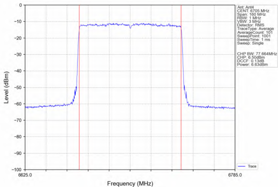
802.11be(EHT80)_MCH_6705MHz_RU996_Left(67)_Ant4_NTNV
