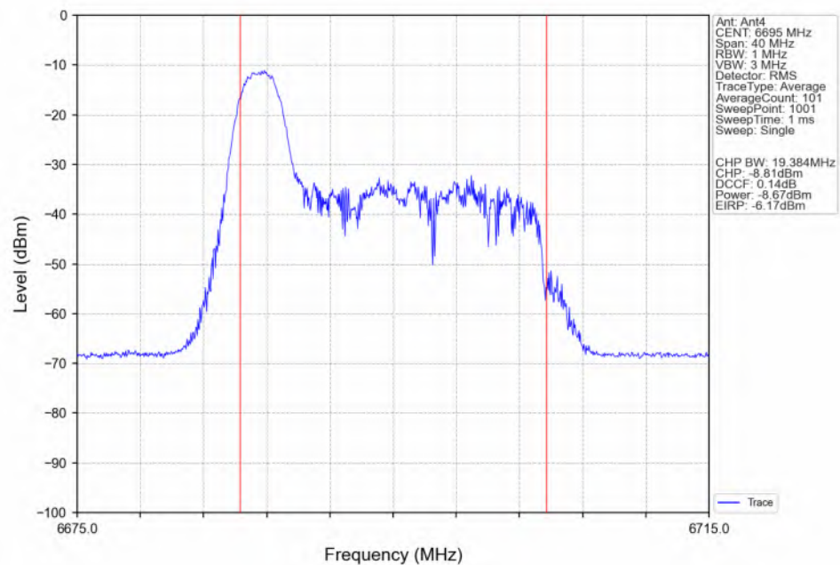
802.11be(EHT20)_MCH_6695MHz_RU26_Left(0)_Ant4_NTNV
