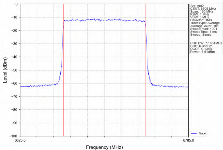
802.11be(EHT80)_MCH_6705MHz_RU996_Left(67)_Ant2_NTNV
