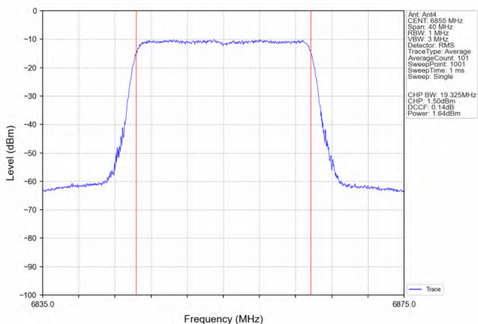
802.11be(EHT20)_HCH_6855MHz_RU242_Left(61)_Ant4_NTNV
