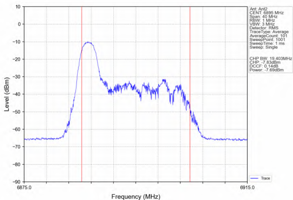
802.11be(EHT20)_LCH_6895MHz_RU26_Left(0)_Ant2_NTNV
