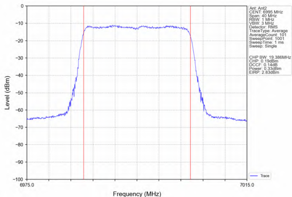
802.11be(EHT20)_MCH_6995MHz_RU242_Left(61)_Ant2_NTNV
