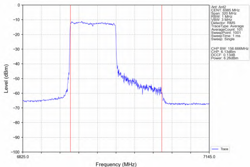
802.11be(EHT160)_MCH_6985MHz_RU996_Left(67)_Ant2_NTNV
