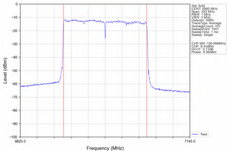
802.11be(EHT160)_MCH_6985MHz_2xRU996_Left(68)_Ant2_NTNV
