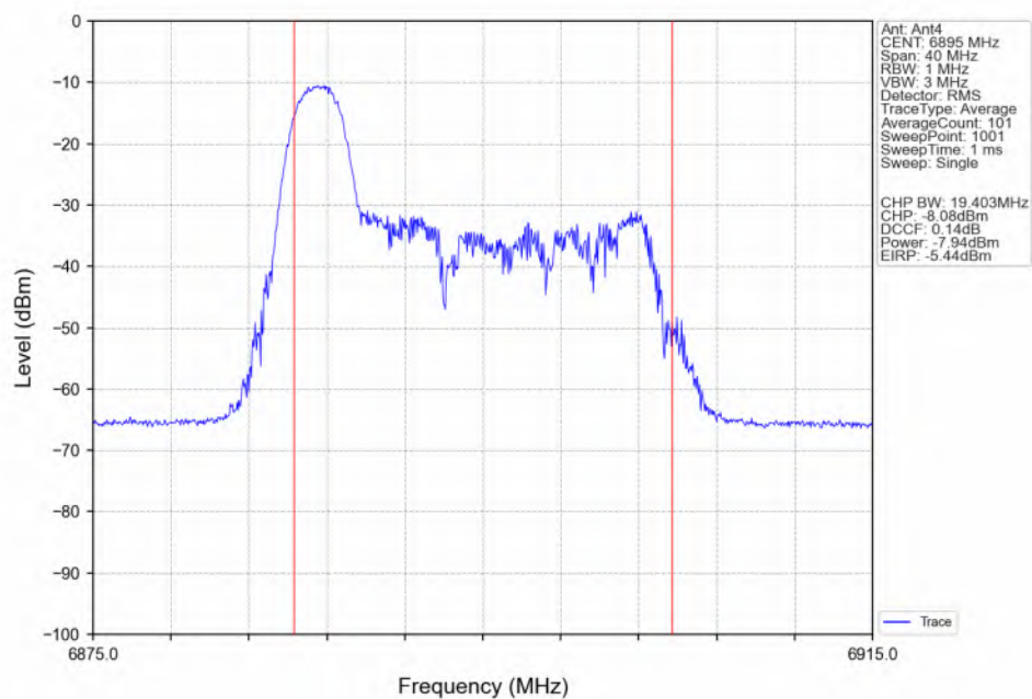
802.11be(EHT20) LCH_6895MHz_RU26_Left(0)_Ant4_NTNV
