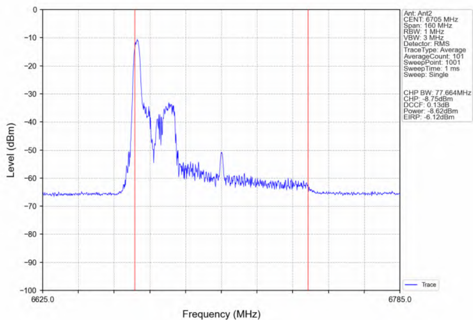
802.11be(EHT80)_MCH_6705MHz_RU26_Left(0)_Ant2_NTNV
