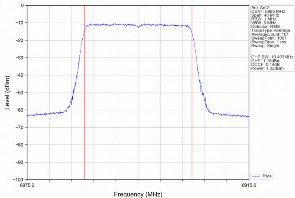
802.11be(EHT20) LCH_6895MHz_RU242_Left(61)_Ant2_NTNV
