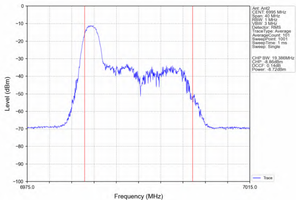
802.11be(EHT20)_MCH_6995MHz_RU26_Left(0)_Ant2_NTNV
