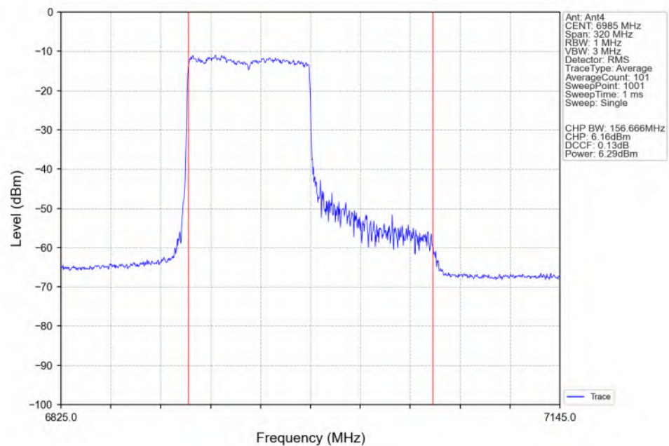
802.11be(EHT160)_MCH_6985MHz_RU996_Left(67)_Ant4_NTNV
