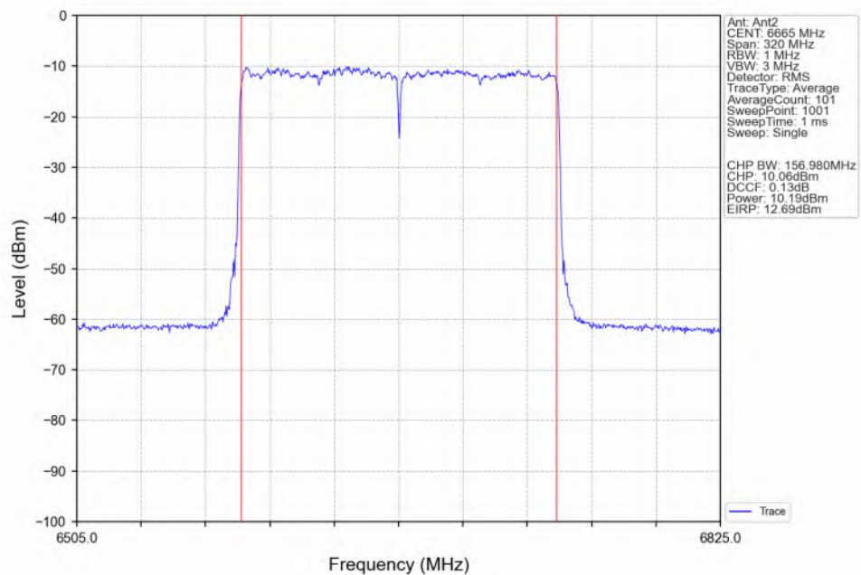
802.11be(EHT160)_MCH_6665MHz_2xRU996_Left(68)_Ant2_NTNV
