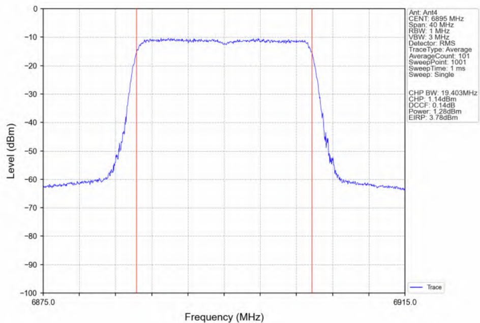
802.11be(EHT20) LCH_6895MHz_RU242_Left(61)_Ant4_NTNV
