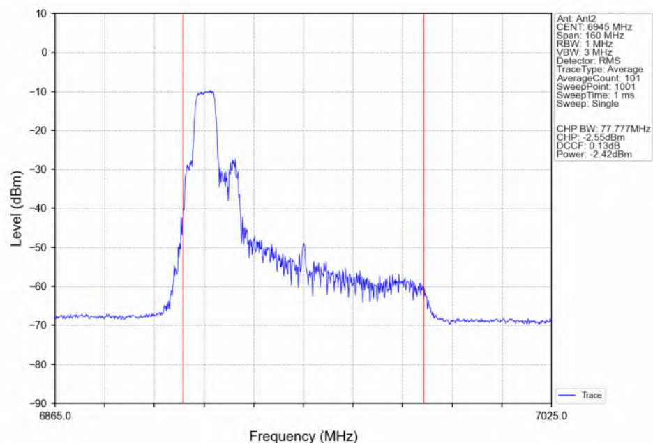
802.11be(EHT80)_LCH_6945MHz_26+52_ / Ant2_NTNV
