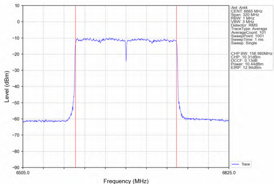
802.11be(EHT160)_MCH_6665MHz_2xRU996_Left(68)_Ant4_NTNV
