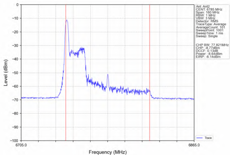
802.11be(EHT80)_HCH_6785MHz_RU26_Left(0)_Ant2_NTNV
