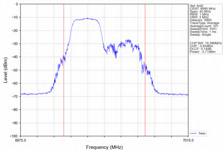
802.11be(EHT20)_MCH_6995MHz_26+52_ / Ant2_NTNV
