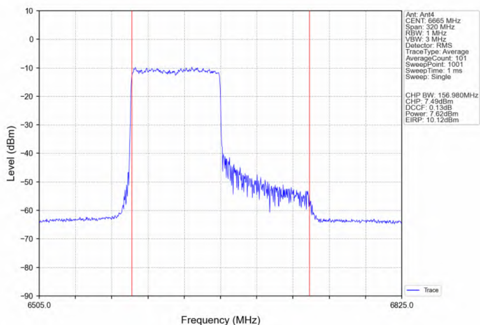
802.11be(EHT160)_MCH_6665MHz_RU996_Left(67)_Ant4_NTNV
