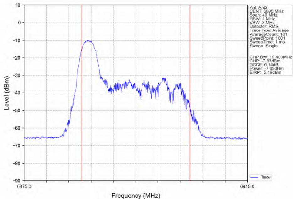
802.11be(EHT20)_LCH_6895MHz_RU26_Left(0)_Ant2_NTNV
