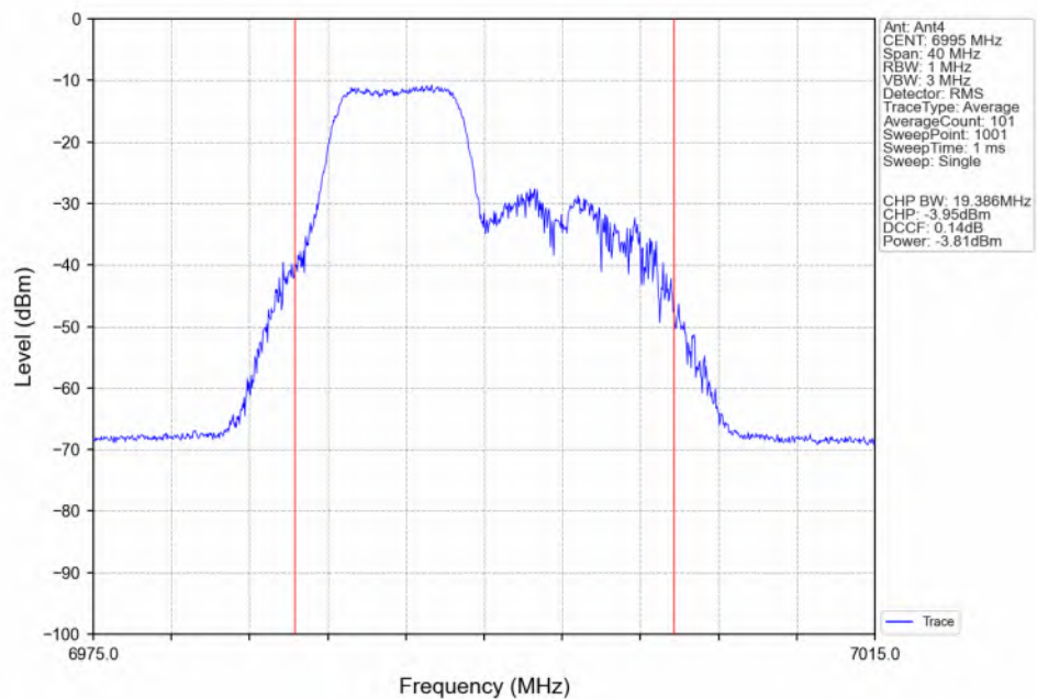
802.11be(EHT20)_MCH_6995MHz_26+52_ / Ant4_NTNV
