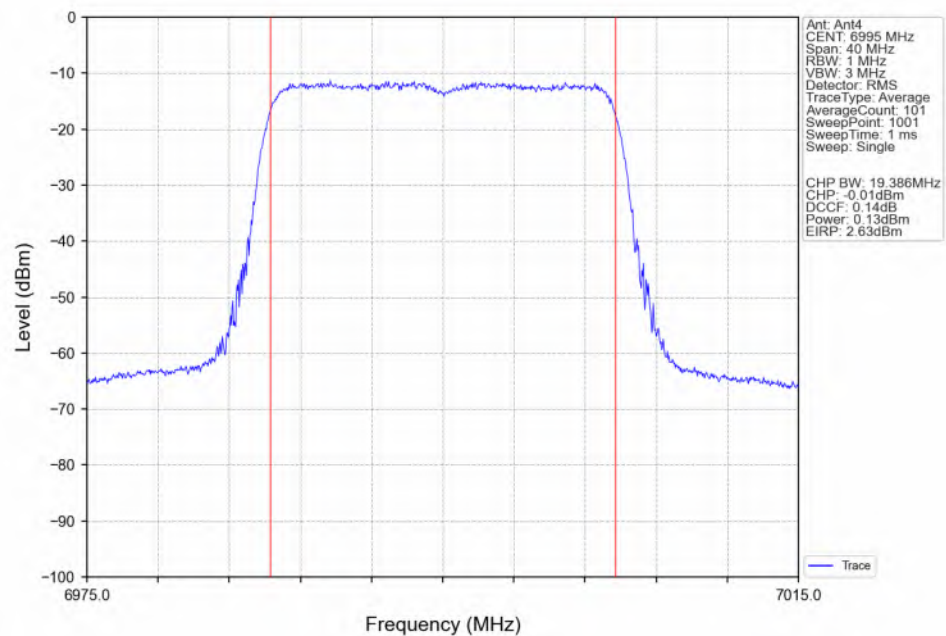
802.11be(EHT20)_MCH_6995MHz_RU242_Left(61)_Ant4_NTNV
