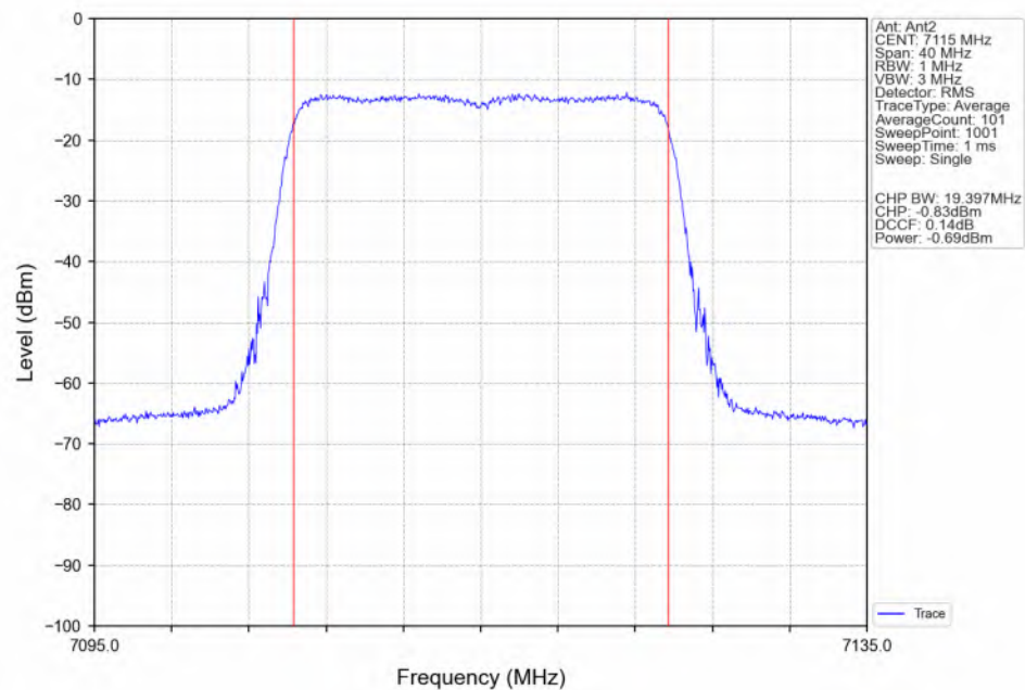
802.11be(EHT20)_HCH_7115MHz_RU242_Left(61)_Ant2_NTNV
