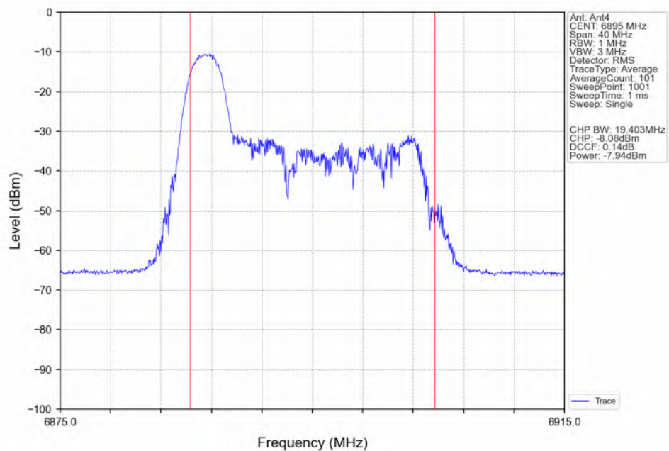
802.11be(EHT20) LCH_6895MHz_RU26_Left(0)_Ant4_NTNV
