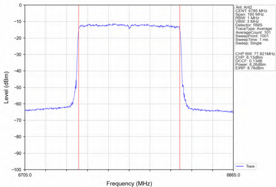
802.11be(EHT80)_HCH_6785MHz_RU996_Left(67)_Ant2_NTNV
