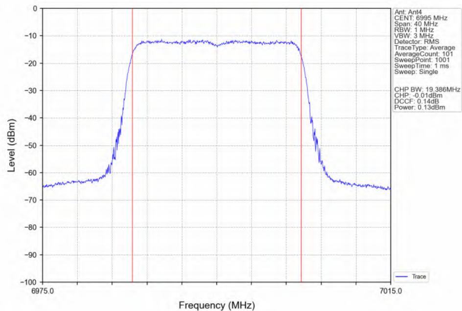
802.11be(EHT20)_MCH_6995MHz_RU242_Left(61)_Ant4_NTNV
