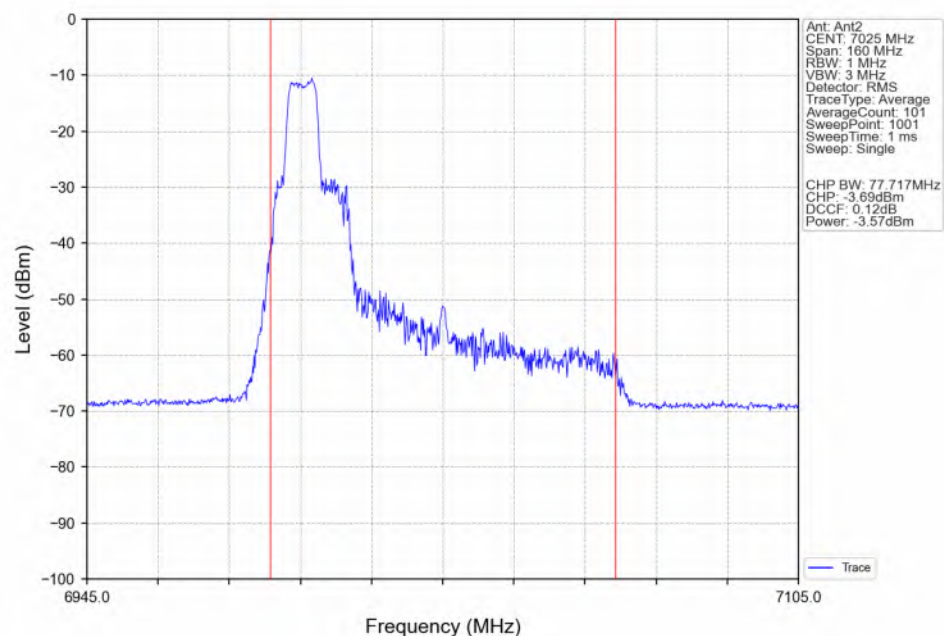
802.11be(EHT80)_HCH_7025MHz_26+52_ / Ant2_NTNV
