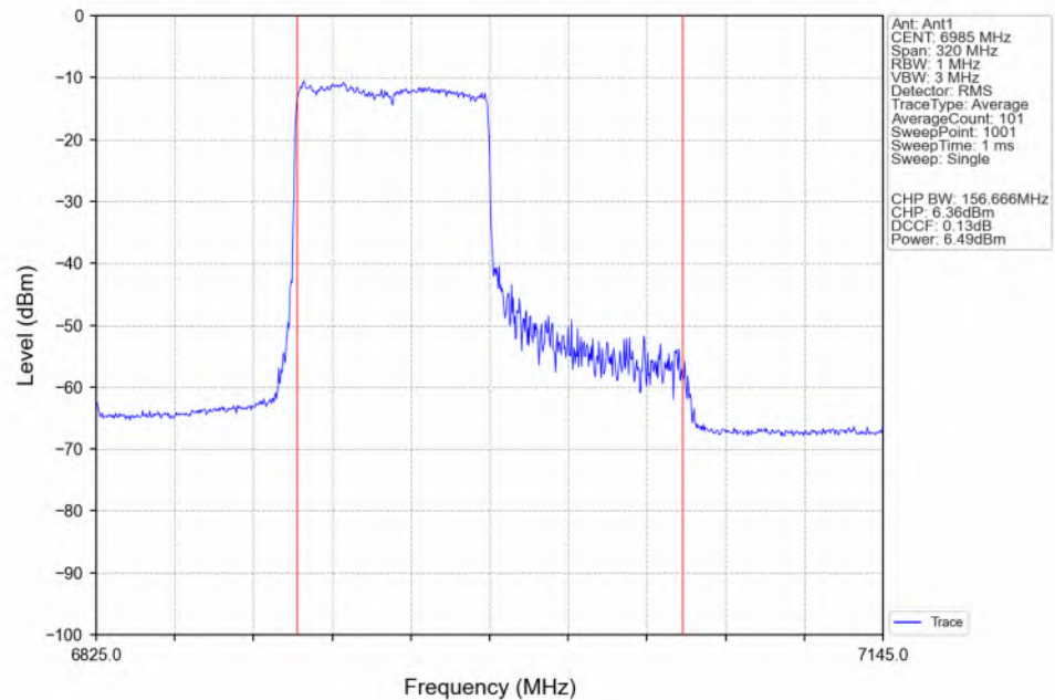
802.11be(EHT160)_MCH_6985MHz_RU996_Left(67)_Ant2_NTNV
