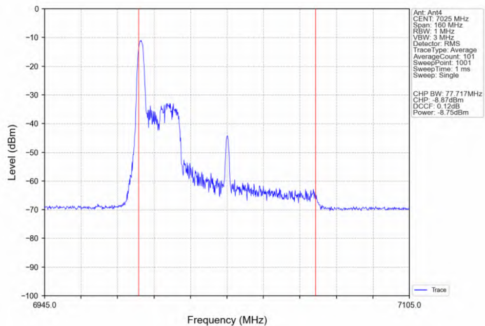
802.11be(EHT80)_HCH_7025MHz_RU26_Left(0)_Ant4_NTNV
