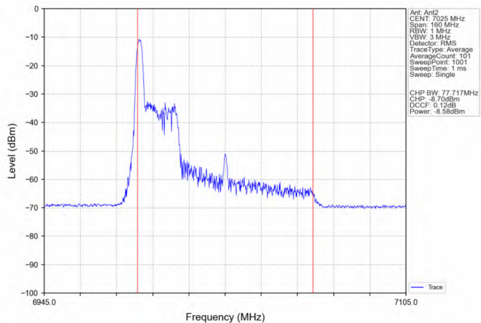
802.11be(EHT80)_HCH_7025MHz_RU26_Left(0)_Ant2_NTNV
