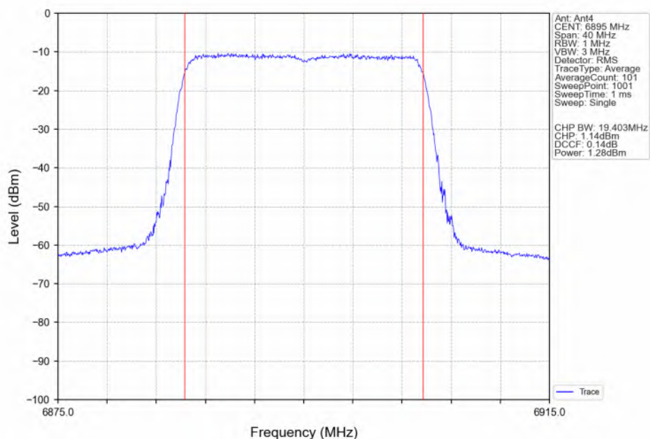
802.11be(EHT20) LCH_6895MHz_RU242_Left(61)_Ant4_NTNV
