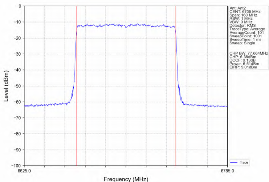
802.11be(EHT80)_MCH_6705MHz_RU996_Left(67)_Ant2_NTNV
