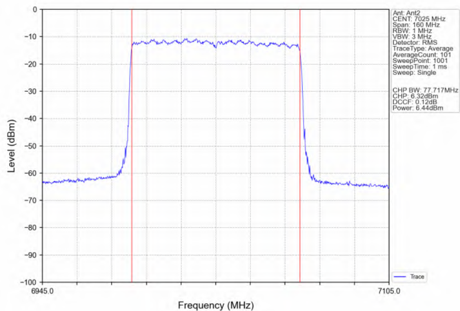
802.11be(EHT80)_HCH_7025MHz_RU996_Left(67)_Ant2_NTNV
