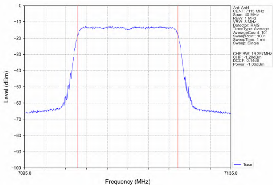
802.11be(EHT20)_HCH_7115MHz_RU242_Left(61)_Ant4_NTNV
