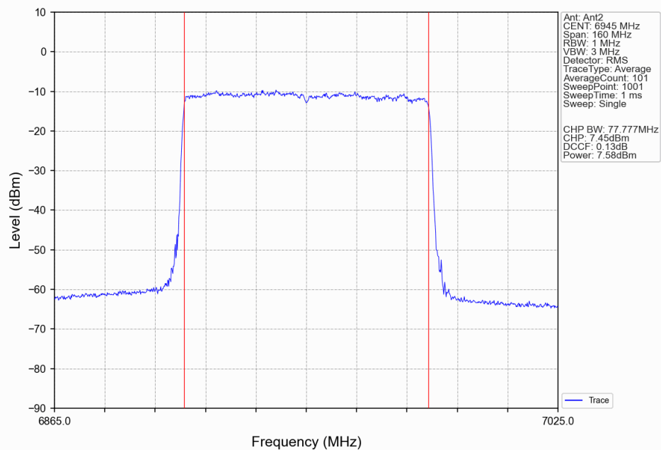
802.11be(EHT80) LCH_6945MHz_RU996_Left(67)_Ant2_NTNV
