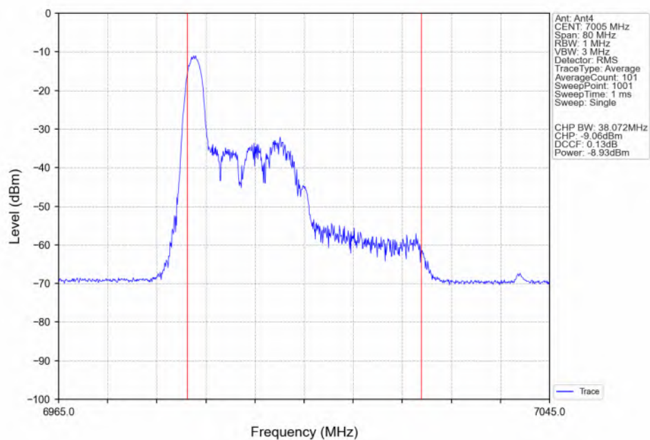
802.11be(EHT40)_MCH_7005MHz_RU26_Left(0)_Ant4_NTNV
