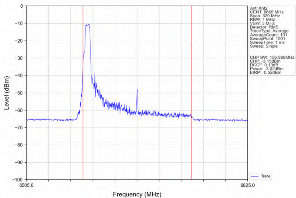
802.11be(EHT160)_MCH_6665MHz_26+52 / _Ant2_NTNV
