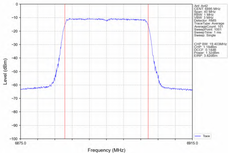
802.11be(EHT20) LCH_6895MHz_RU242_Left(61)_Ant2_NTNV
