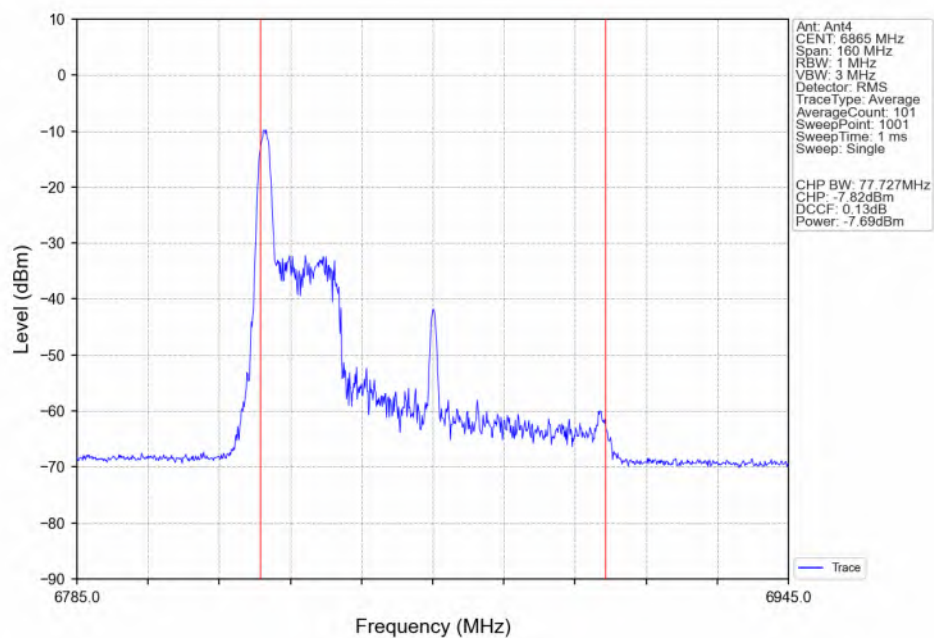
802.11be(EHT80)_HCH_6865MHz_RU26_Left(0)_Ant4_NTNV
