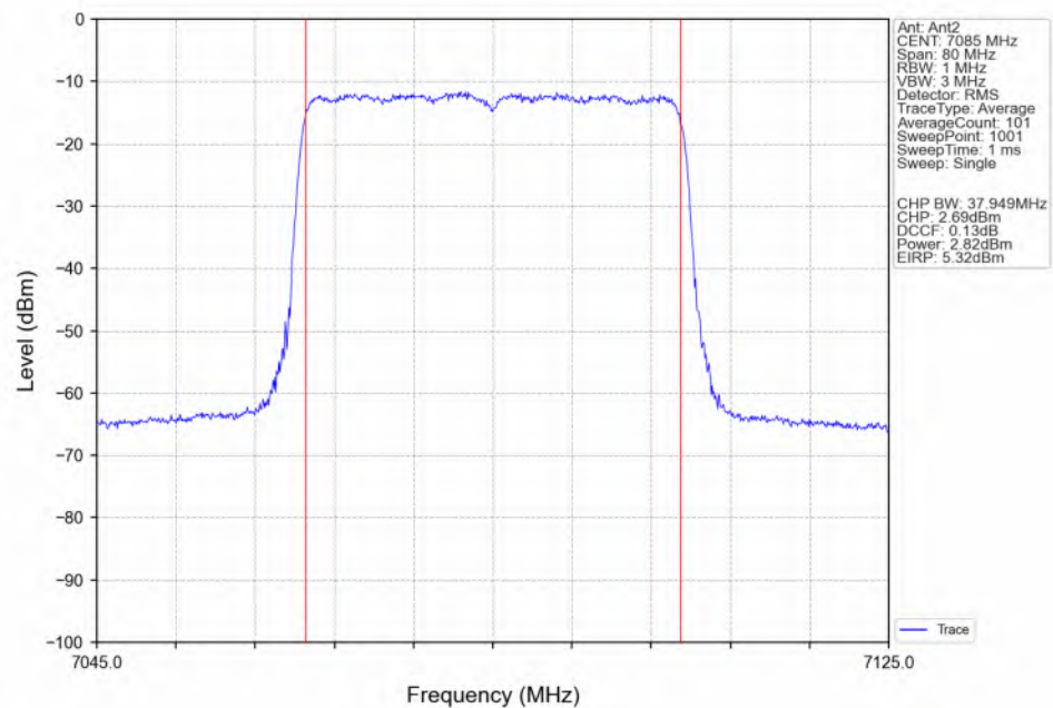
802.11be(EHT40)_HCH_7085MHz_RU484_Left(65)_Ant2_NTNV
