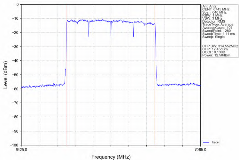
802.11be(EHT320)_LCH_6745MHz_4xRU996_Left(70)_Ant2_NTNV
