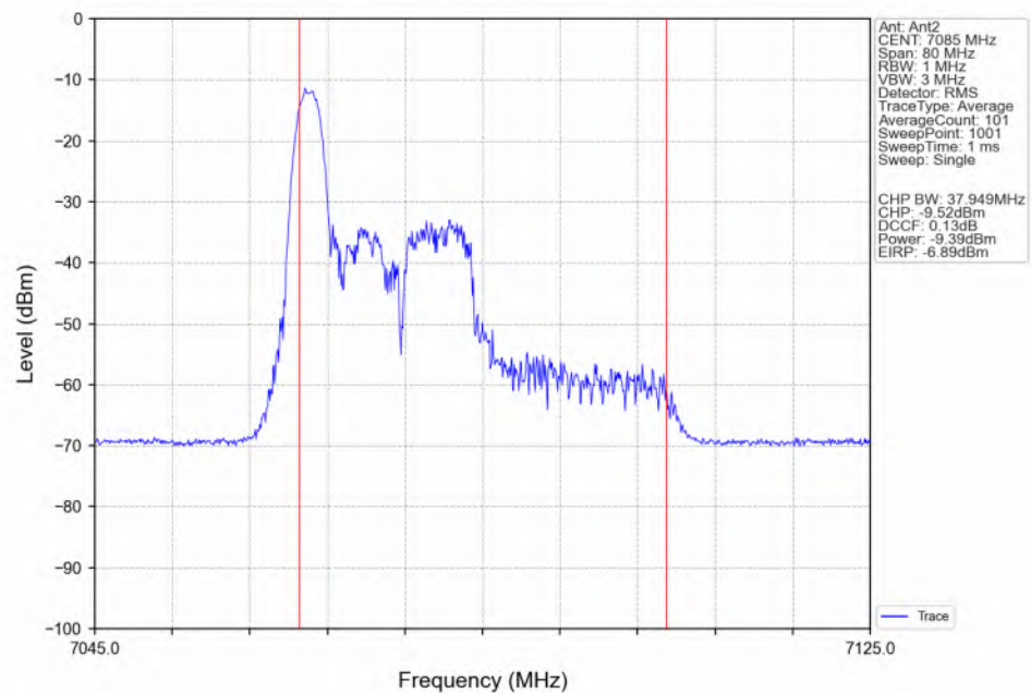
802.11be(EHT40)_HCH_7085MHz_RU26_Left(0)_Ant2_NTNV
