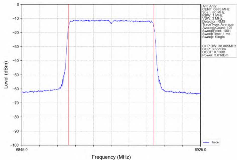
802.11be(EHT40)_HCH_6885MHz_RU484_Left(65)_Ant2_NTNV
