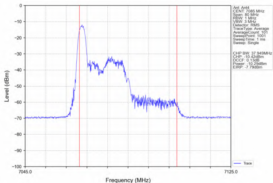
802.11be(EHT40)_HCH_7085MHz_RU26_Left(0)_Ant4_NTNV
