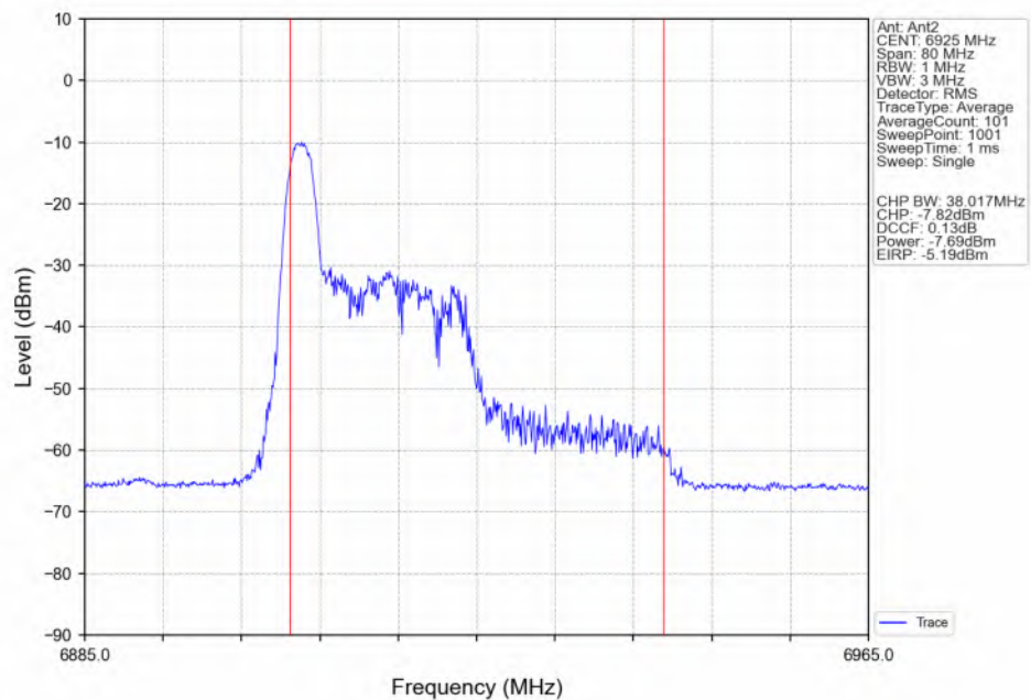
802.11be(EHT40) LCH_6925MHz_RU26_Left(0)_Ant2_NTNV
