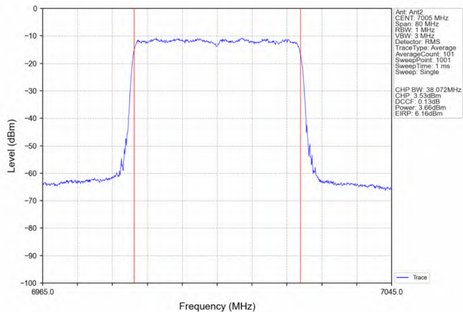
802.11be(EHT40)_MCH_7005MHz_RU484_Left(65)_Ant2_NTNV
