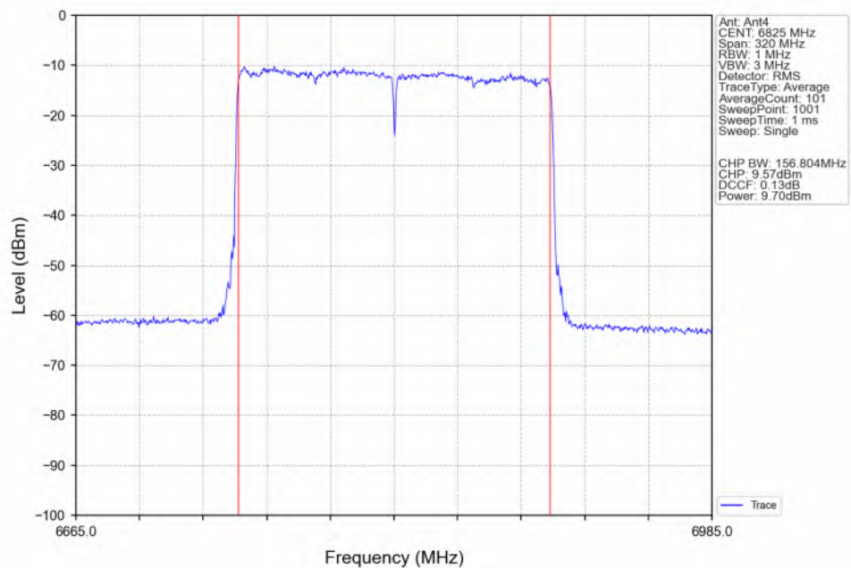
802.11be(EHT160)_HCH_6825MHz_2xRU996_Left(68)_Ant4_NTNV
