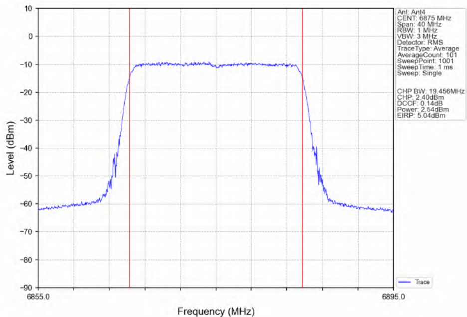
802.11be(EHT20)_HCH_6875MHz_RU242_Left(61)_Ant4_NTNV
