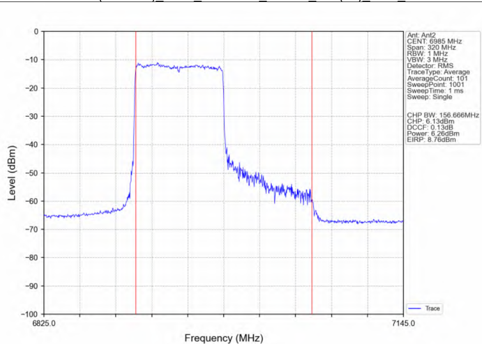
802.11be(EHT160)_MCH_6985MHz_RU996_Left(67)_Ant2_NTNV
