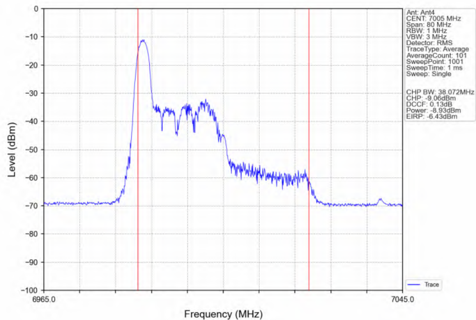
802.11be(EHT40)_MCH_7005MHz_RU26_Left(0)_Ant4_NTNV
