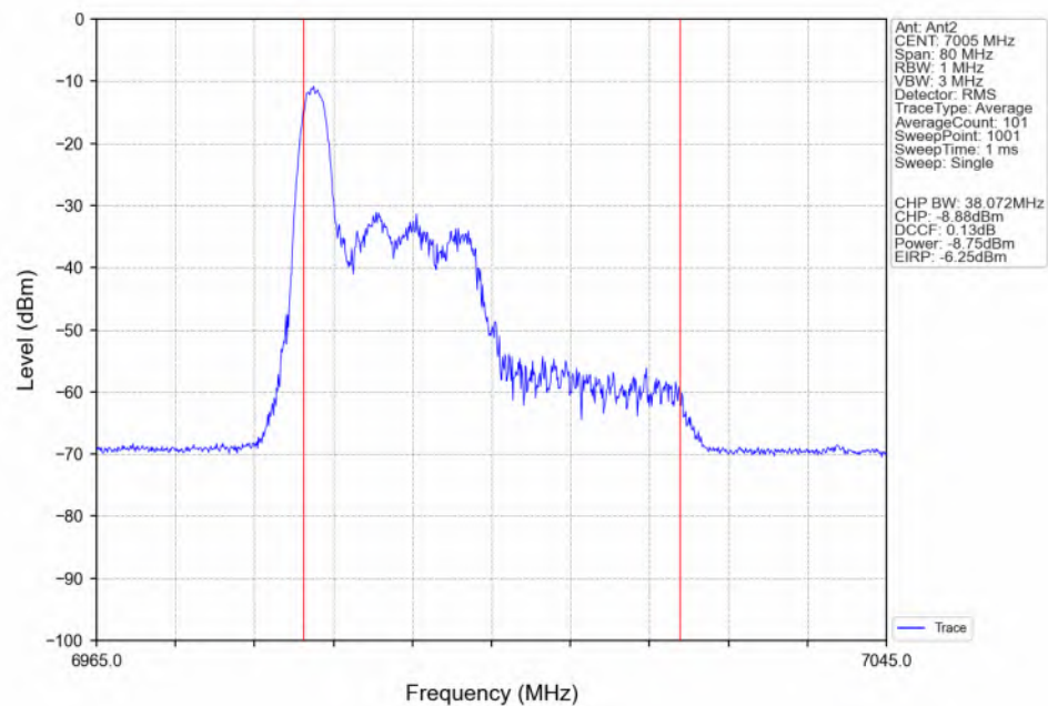
802.11be(EHT40)_MCH_7005MHz_RU26_Left(0)_Ant2_NTNV
