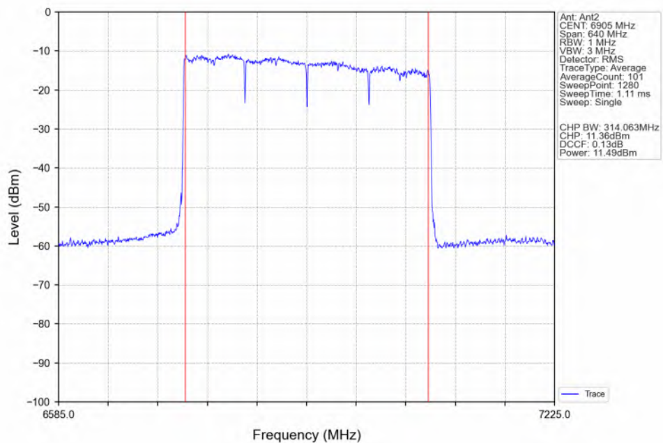
802.11be(EHT320)_HCH_6905MHz_4xRU996_Left(70)_Ant2_NTNV
