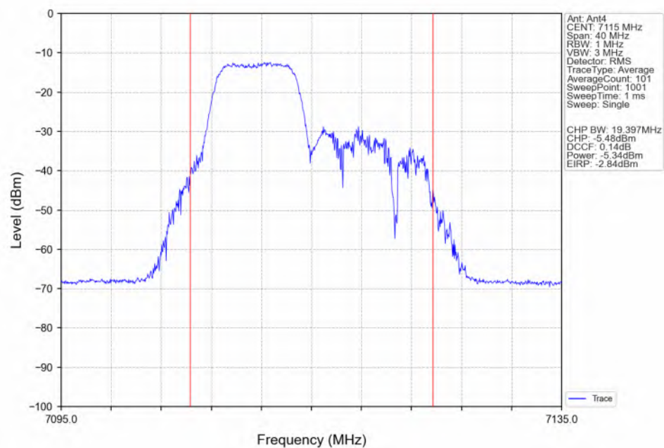
802.11be(EHT20)_HCH_7115MHz_26+52_ / Ant4_NTNV
