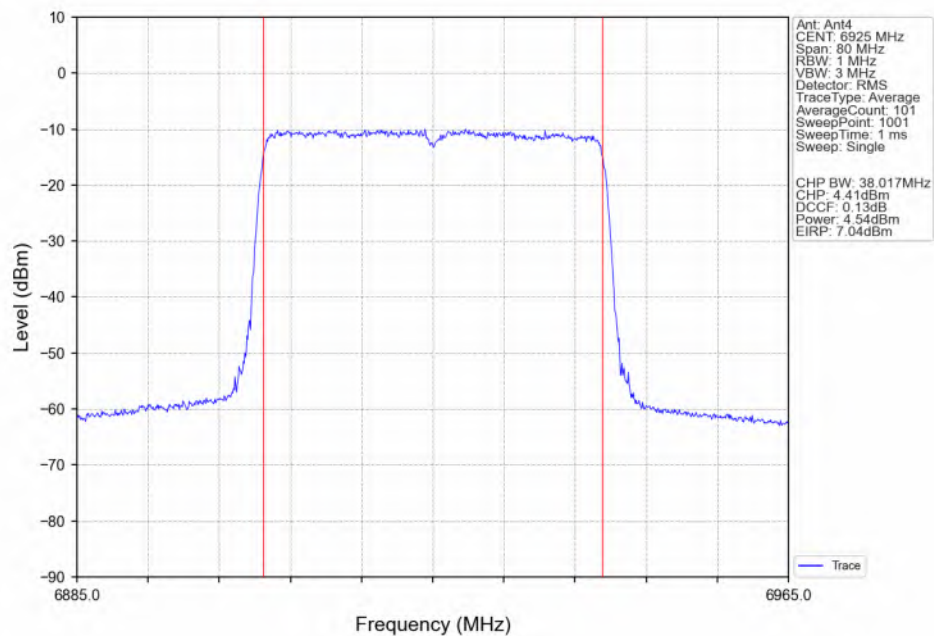
802.11be(EHT40) LCH_6925MHz_RU484_Left(65)_Ant4_NTNV
