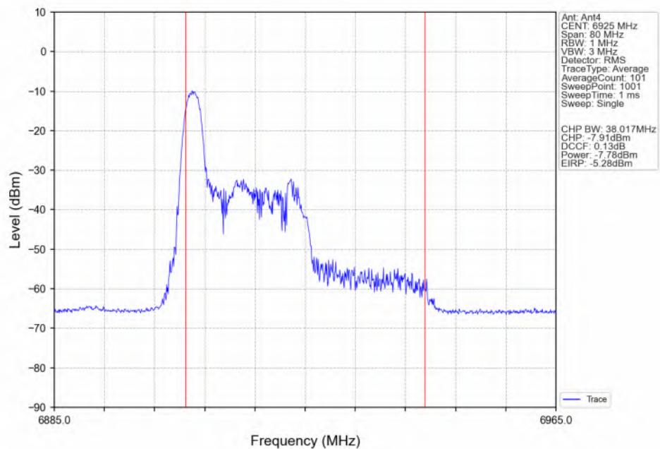
802.11be(EHT40) LCH_6925MHz_RU26_Left(0)_Ant4_NTNV
