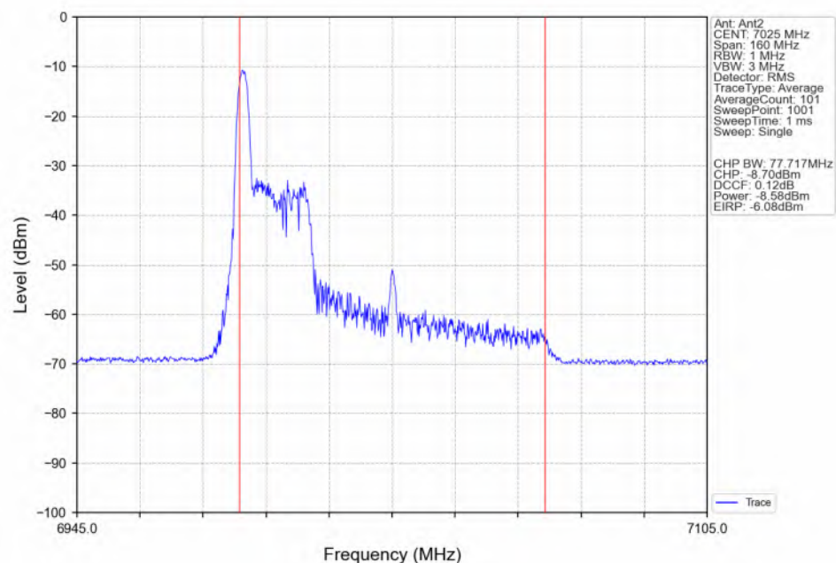
802.11be(EHT80)_HCH_7025MHz_RU26_Left(0)_Ant2_NTNV
