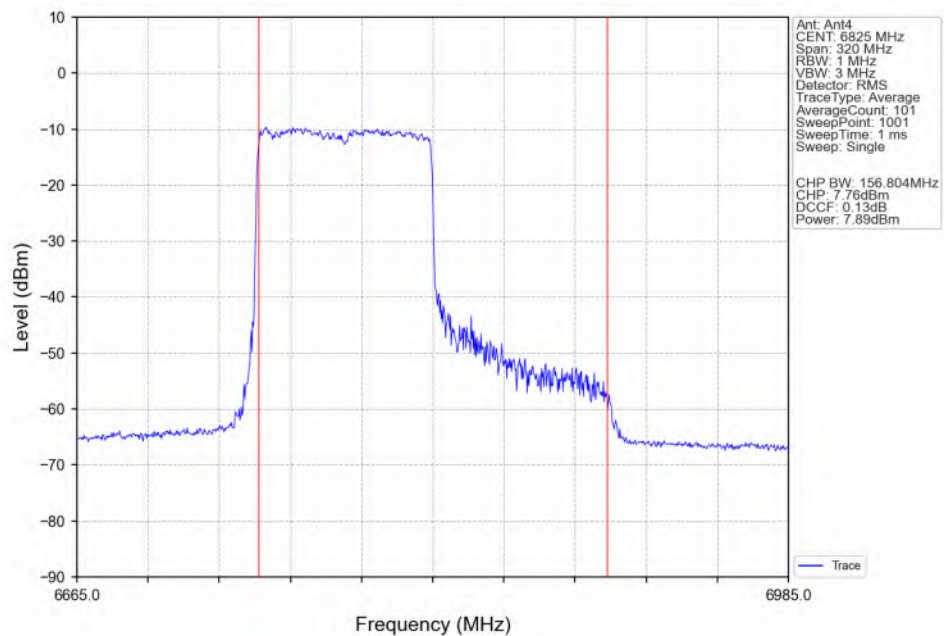
802.11be(EHT160)_HCH_6825MHz_RU996_Left(67)_Ant4_NTNV
