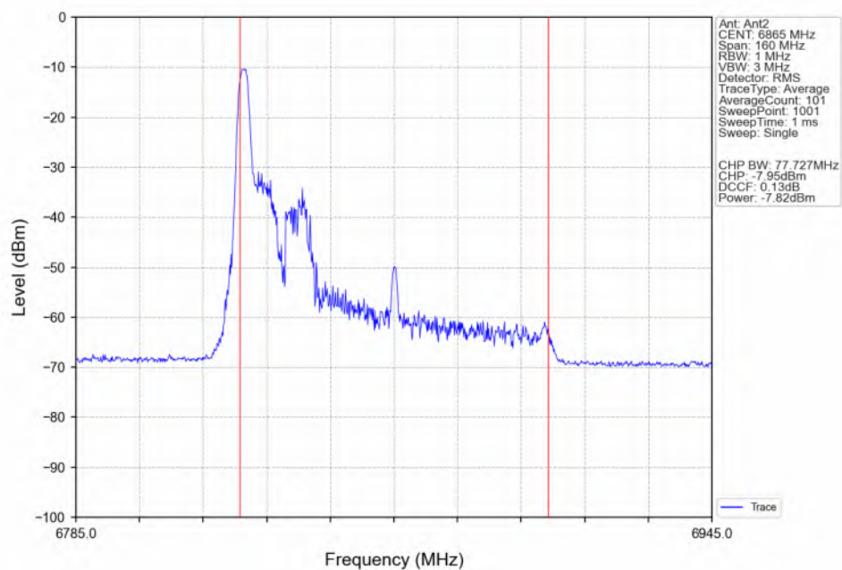
802.11be(EHT80)_HCH_6865MHz_RU26_Left(0)_Ant2_NTNV
