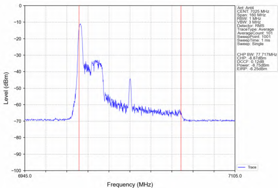
802.11be(EHT80)_HCH_7025MHz_RU26_Left(0)_Ant4_NTNV
