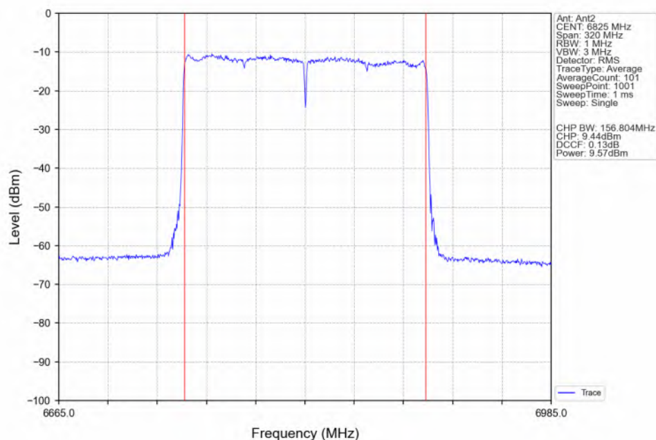
802.11be(EHT160)_HCH_6825MHz_2xRU996_Left(68)_Ant2_NTNV
