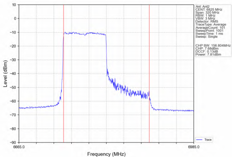
802.11be(EHT160)_HCH_6825MHz_RU996_Left(67)_Ant2_NTNV
