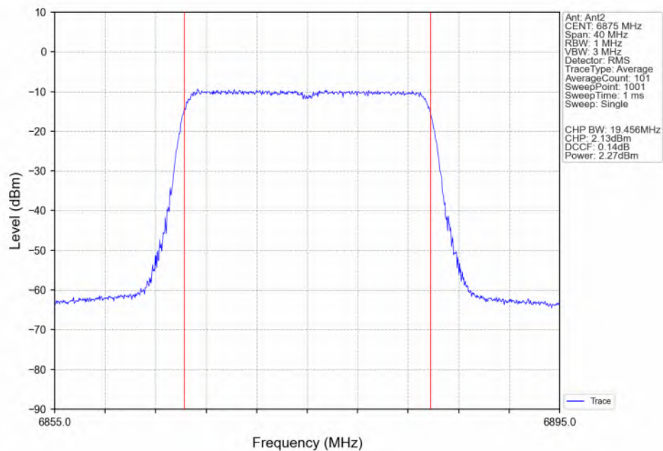
802.11be(EHT20)_HCH_6875MHz_RU242_Left(61)_Ant2_NTNV
