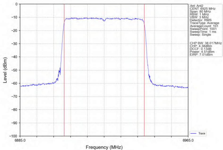
802.11be(EHT40) LCH_6925MHz_RU484_Left(65)_Ant2_NTNV
