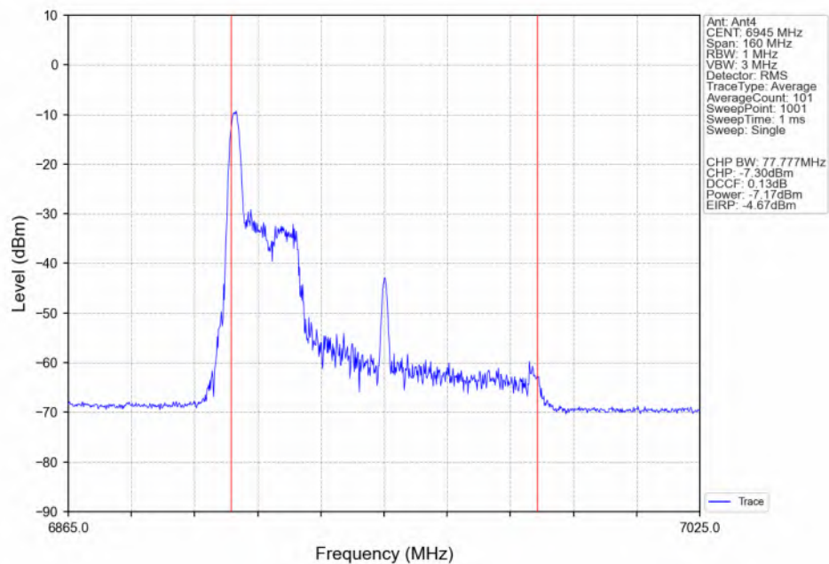
802.11be(EHT80) LCH_6945MHz_RU26_Left(0)_Ant4_NTNV
