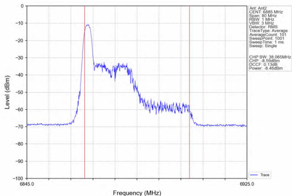
802.11be(EHT40)_HCH_6885MHz_RU26_Left(0)_Ant2_NTNV
