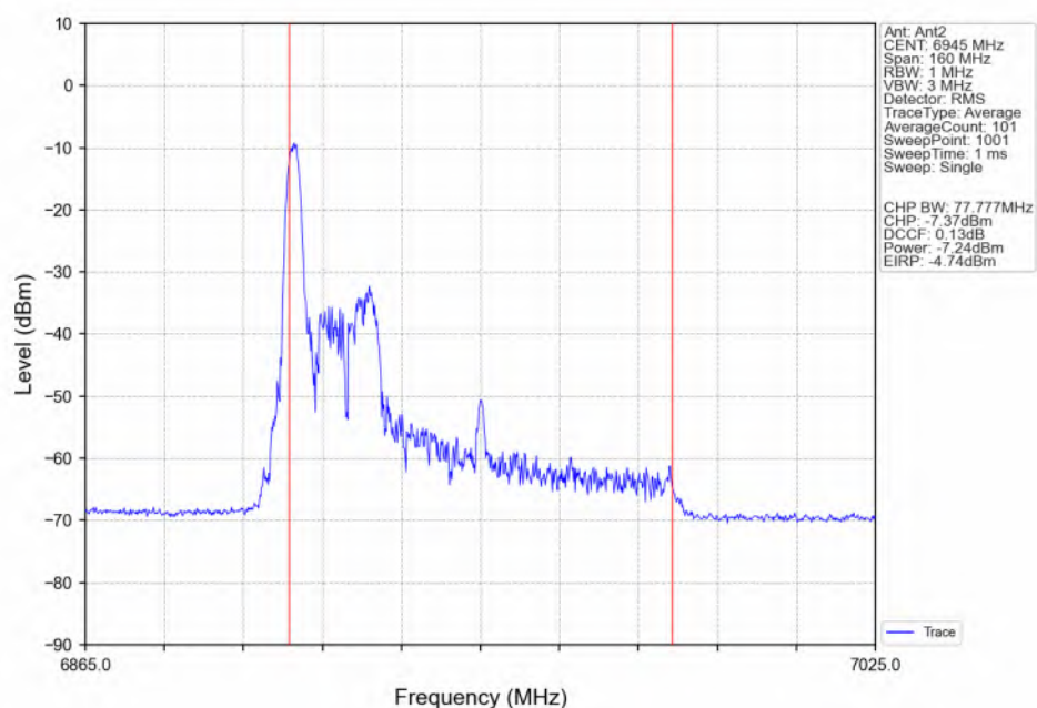
802.11be(EHT80) LCH_6945MHz_RU26_Left(0)_Ant2_NTNV
