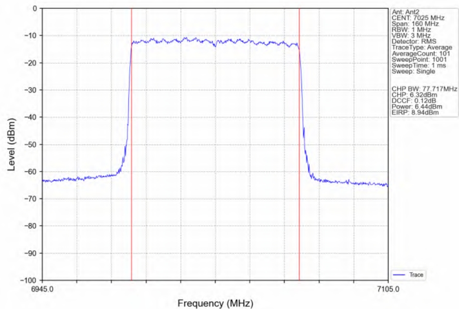
802.11be(EHT80)_HCH_7025MHz_RU996_Left(67)_Ant2_NTNV
