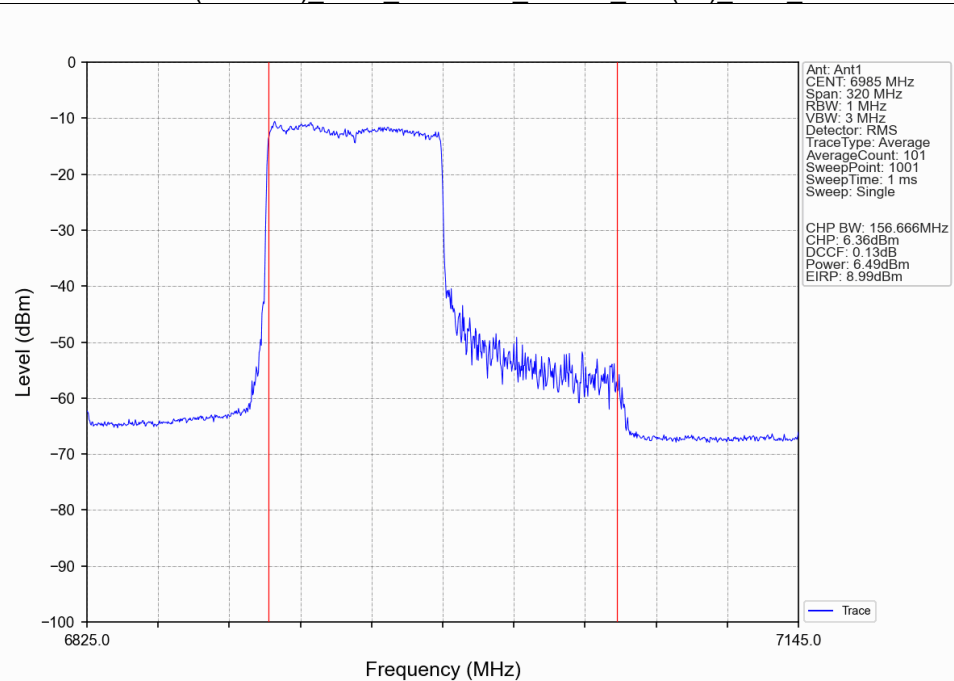
802.11be(EHT160)_MCH_6985MHz_RU996_Left(67)_Ant1_NTNV
