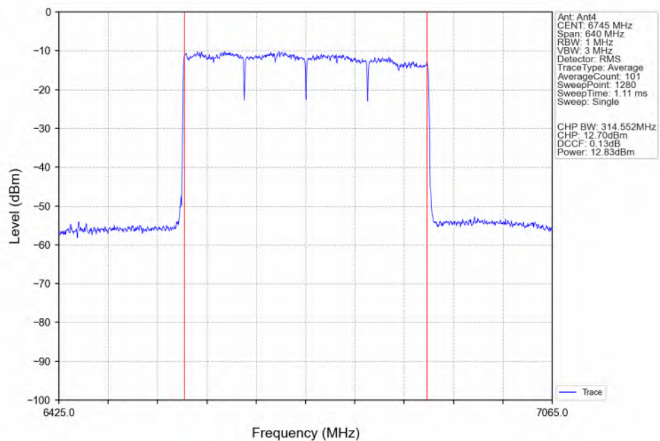
802.11be(EHT320)_LCH_6745MHz_4xRU996_Left(70)_Ant4_NTNV
