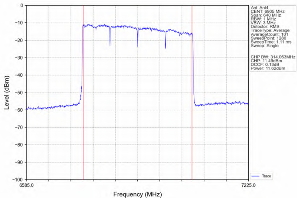
802.11be(EHT320)_HCH_6905MHz_4xRU996_Left(70)_Ant4_NTNV
