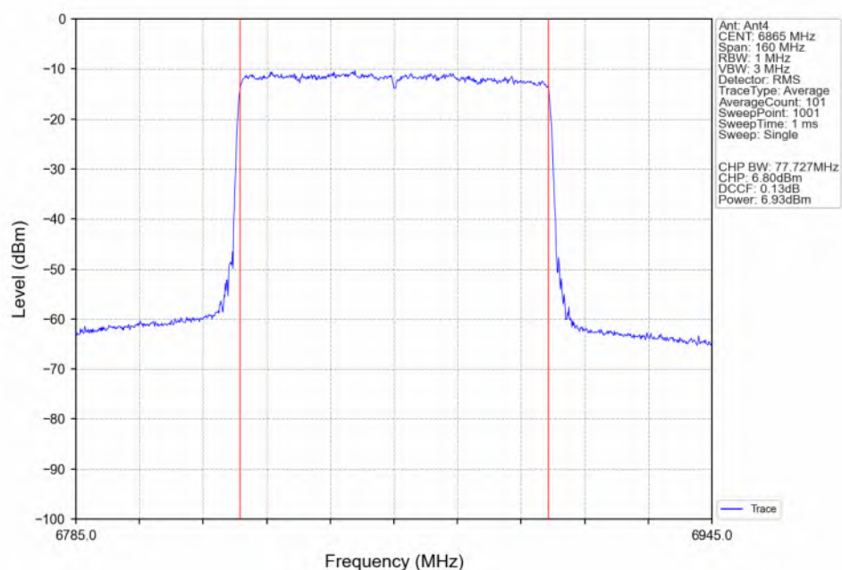
802.11be(EHT80)_HCH_6865MHz_RU996_Left(67)_Ant4_NTNV
