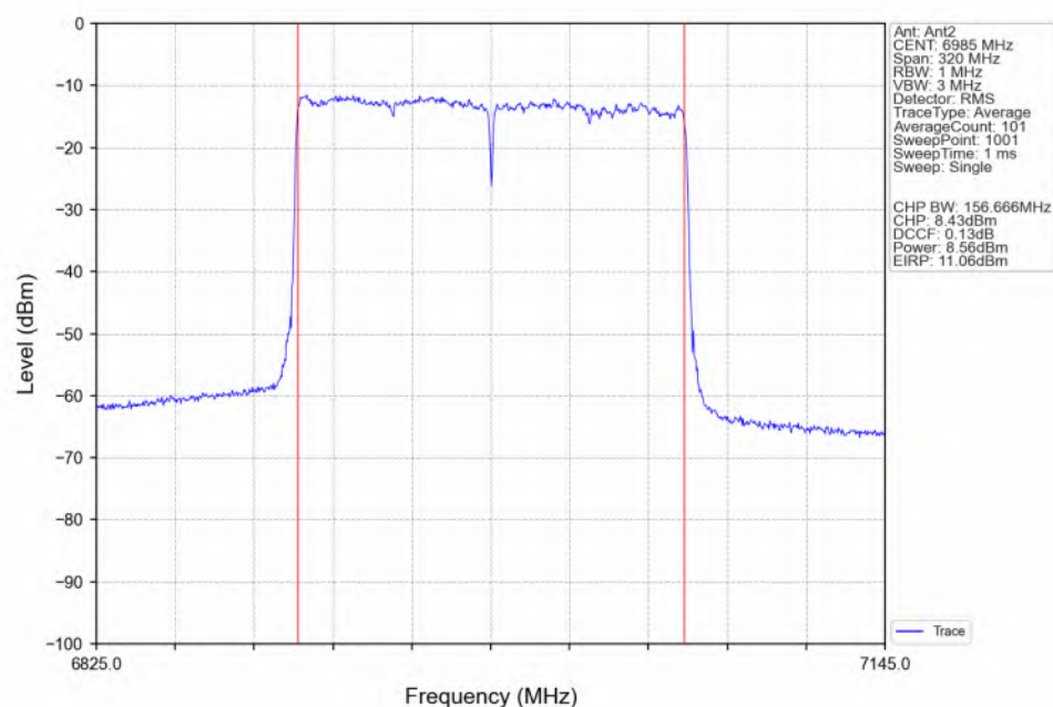
802.11be(EHT160)_MCH_6985MHz_2xRU996_Left(68)_Ant2_NTNV
