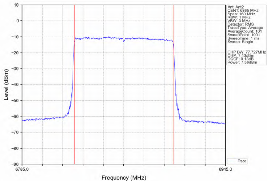
802.11be(EHT80)_HCH_6865MHz_RU996_Left(67)_Ant2_NTNV
