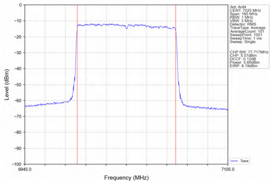
802.11be(EHT80)_HCH_7025MHz_RU996_Left(67)_Ant4_NTNV
