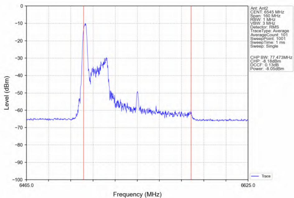
802.11be(EHT80)_HCH_6545MHz_RU26_Left(0)_Ant2_NTNV
