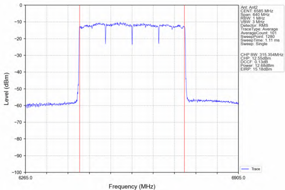
802.11be(EHT320)_MCH_6585MHz_4xRU996_Left(70)_Ant2_NTNV
