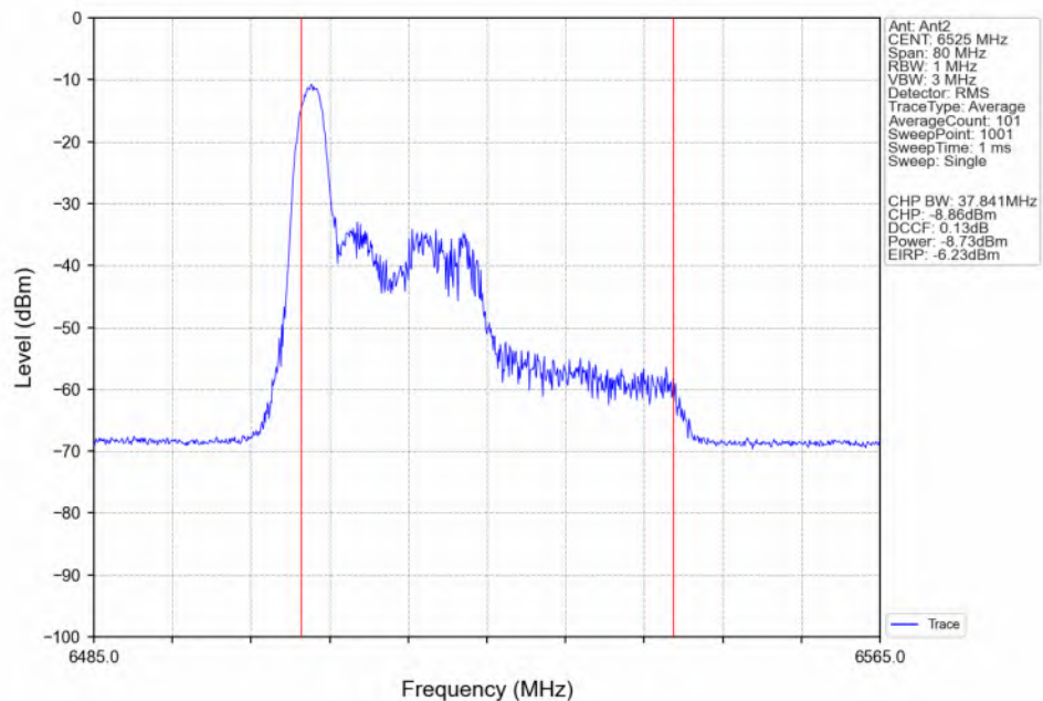
802.11be(EHT40)_HCH_6525MHz_RU26_Left(0)_Ant2_NTNV
