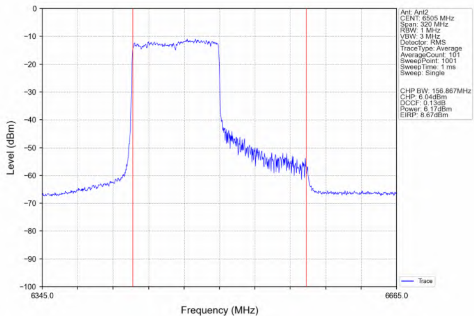
802.11be(EHT160)_HCH_6505MHz_RU996_Left(67)_Ant2_NTNV
