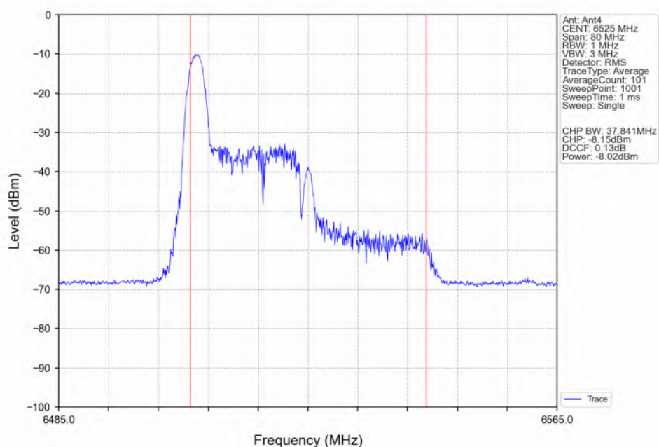
802.11be(EHT40)_HCH_6525MHz_RU26_Left(0)_Ant4_NTNV
