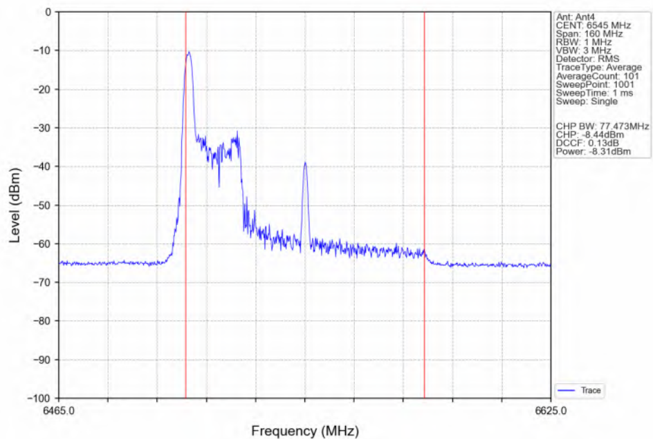
802.11be(EHT80)_HCH_6545MHz_RU26_Left(0)_Ant4_NTNV
