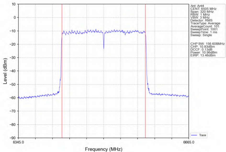
802.11be(EHT160)_HCH_6505MHz_2xRU996_Left(68)_Ant4_NTNV
