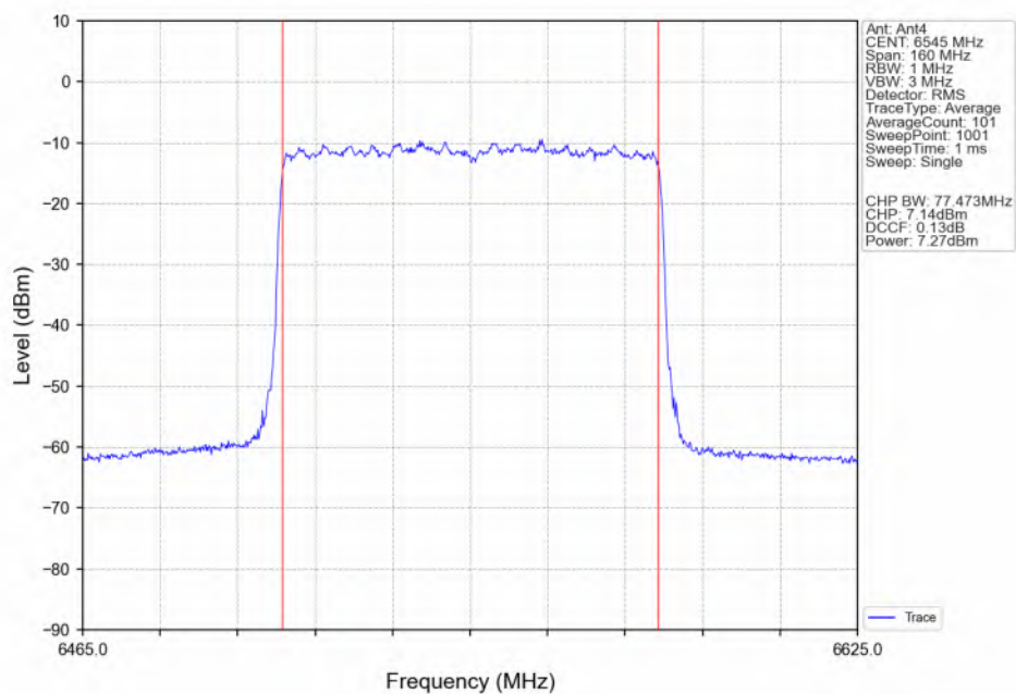
802.11be(EHT80)_HCH_6545MHz_RU996_Left(67)_Ant4_NTNV
