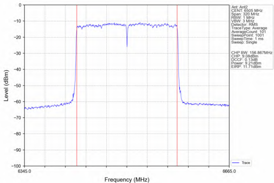
802.11be(EHT160)_HCH_6505MHz_2xRU996_Left(68)_Ant2_NTNV
