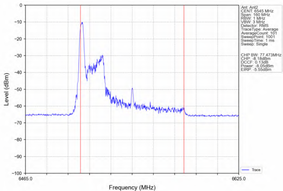
802.11be(EHT80)_HCH_6545MHz_RU26_Left(0)_Ant2_NTNV
