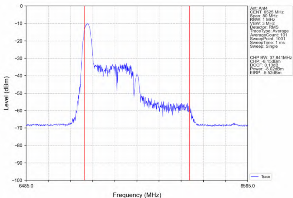
802.11be(EHT40)_HCH_6525MHz_RU26_Left(0)_Ant4_NTNV
