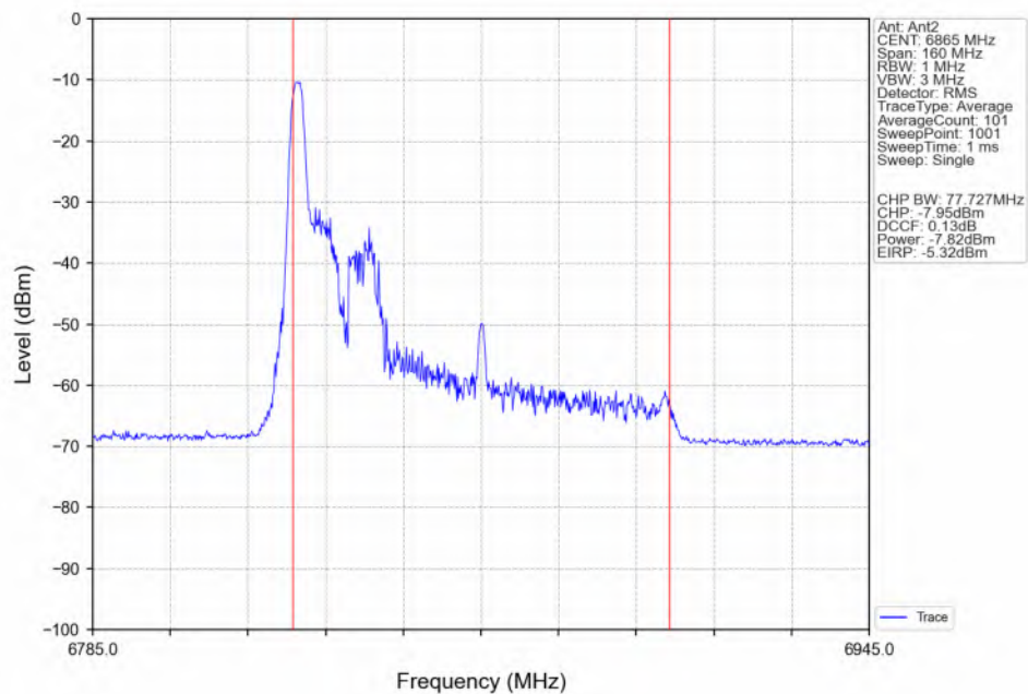
802.11be(EHT80)_HCH_6865MHz_RU26_Left(0)_Ant2_NTNV
