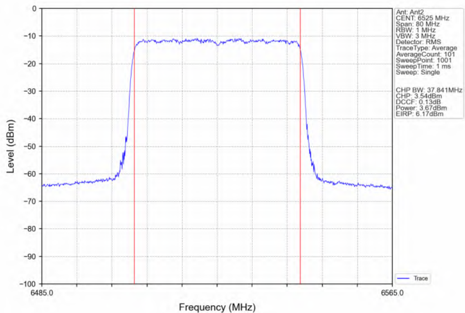
802.11be(EHT40)_HCH_6525MHz_RU484_Left(65)_Ant2_NTNV
