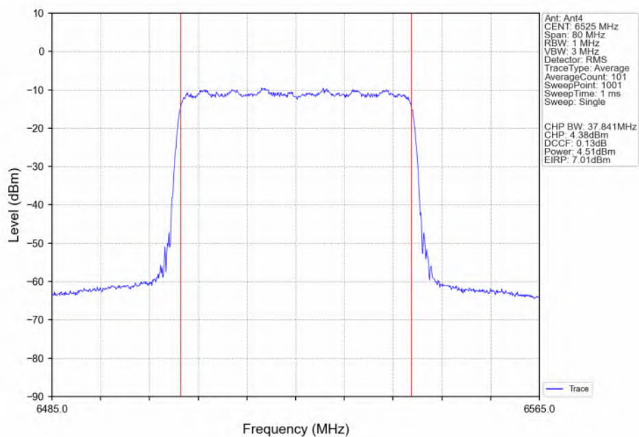
802.11be(EHT40)_HCH_6525MHz_RU484_Left(65)_Ant4_NTNV
