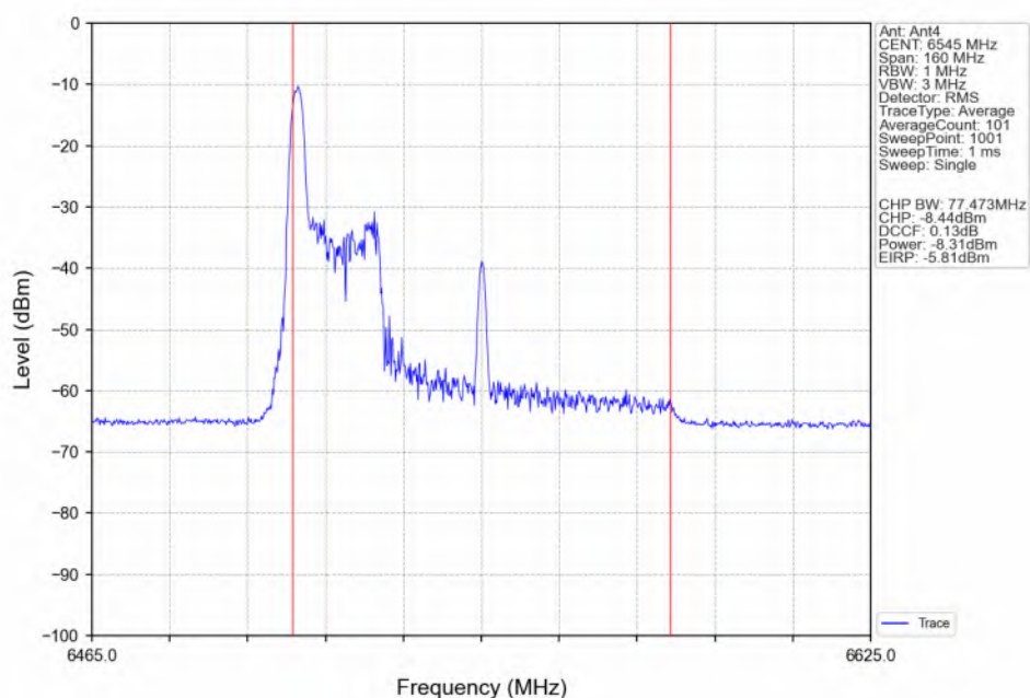
802.11be(EHT80)_HCH_6545MHz_RU26_Left(0)_Ant4_NTNV
