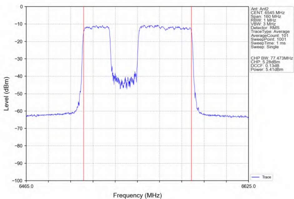
802.11be(EHT80)_HCH_6545MHz_P-20M-RU242+484_ / Ant2_NTNV
