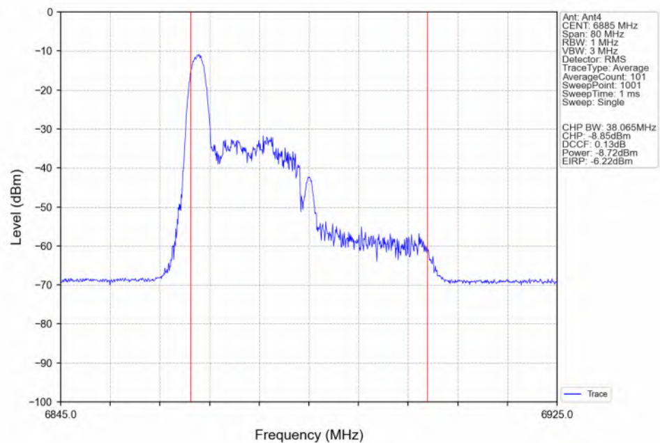
802.11be(EHT40)_HCH_6885MHz_RU26_Left(0)_Ant4_NTNV
