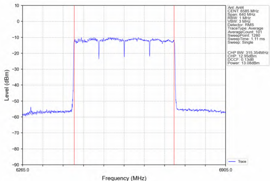
802.11be(EHT320)_MCH_6585MHz_4xRU996_Left(70)_Ant4_NTNV
