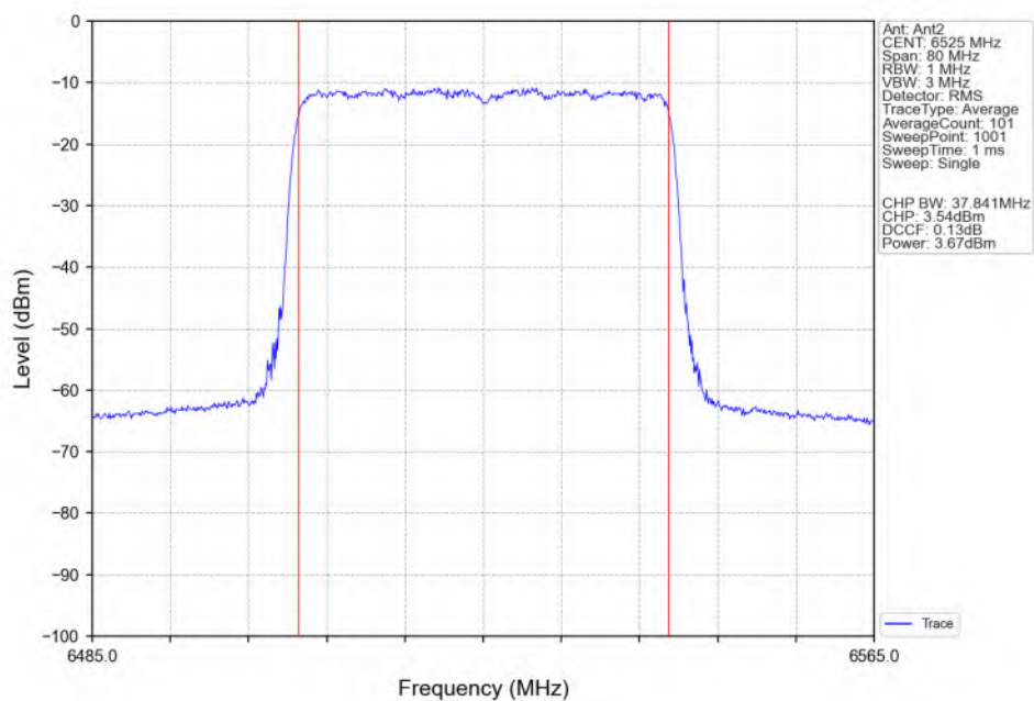
802.11be(EHT40)_HCH_6525MHz_RU484_Left(65)_Ant2_NTNV
