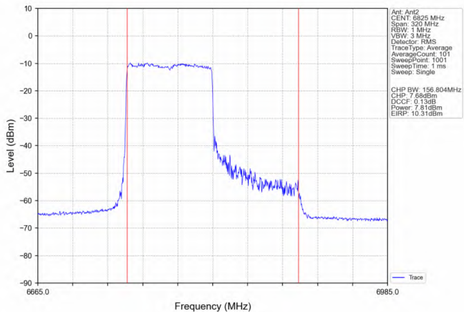
802.11be(EHT160)_HCH_6825MHz_RU996_Left(67)_Ant2_NTNV
