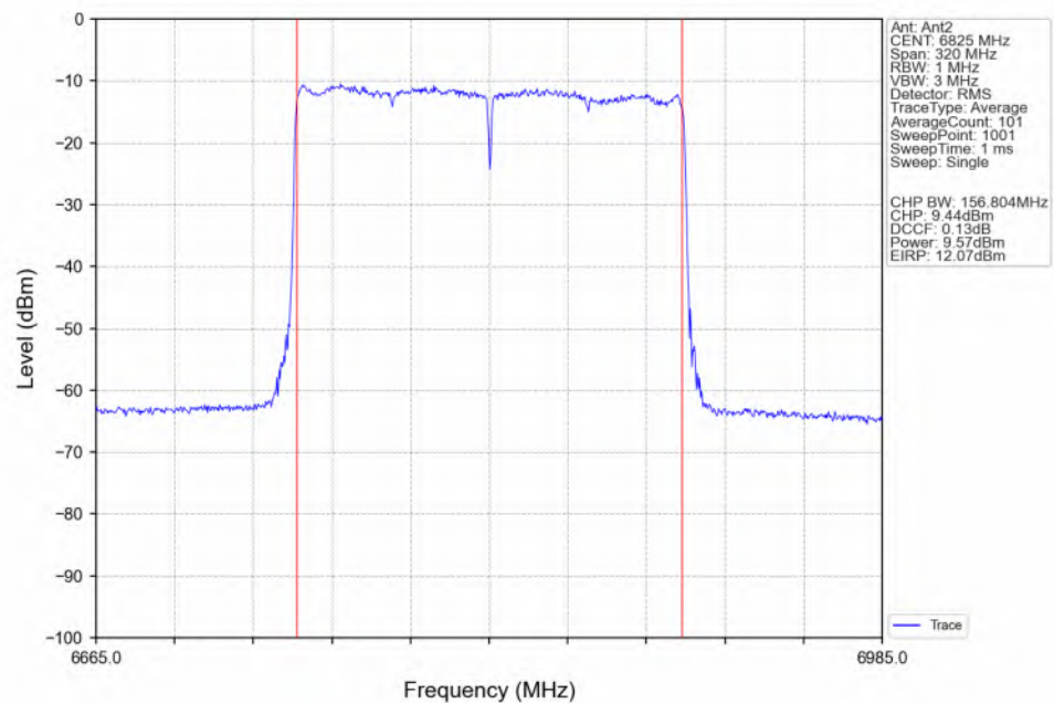
802.11be(EHT160)_HCH_6825MHz_2xRU996_Left(68)_Ant2_NTNV
