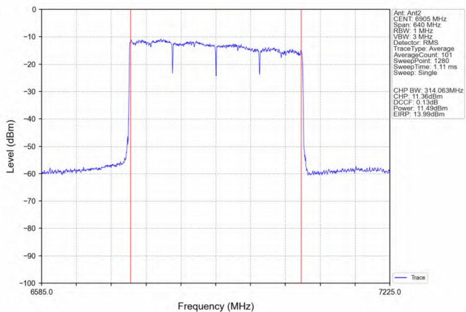
802.11be(EHT320)_HCH_6905MHz_4xRU996_Left(70)_Ant2_NTNV
