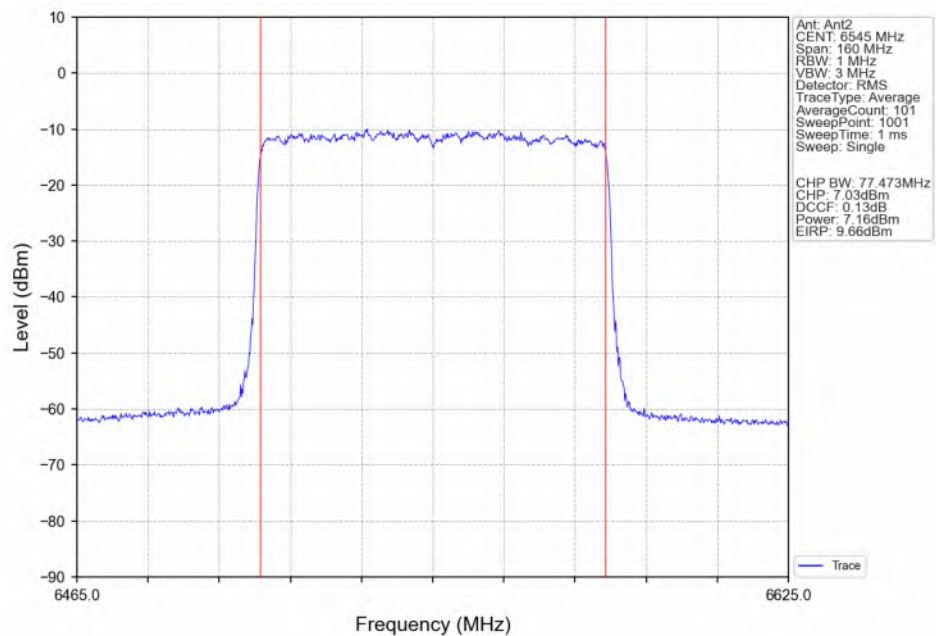
802.11be(EHT80)_HCH_6545MHz_RU996_Left(67)_Ant2_NTNV
