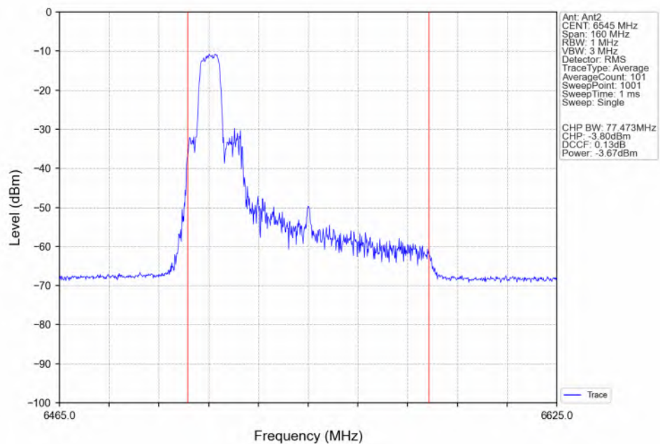
802.11be(EHT80) HCH 6545MHz 26+52 / Ant2_NTNV
