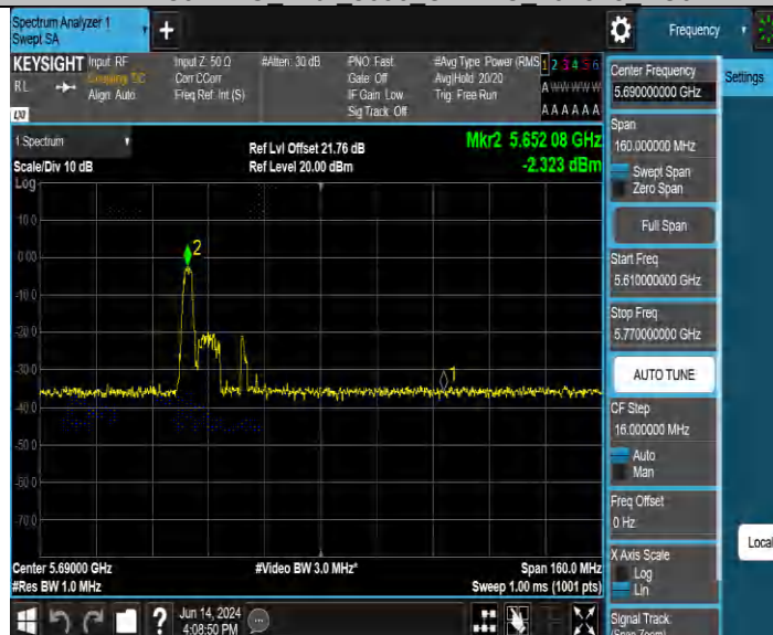
11AX80MIMO_Ant2_5690_UNII-2C_484Tone_RU65
