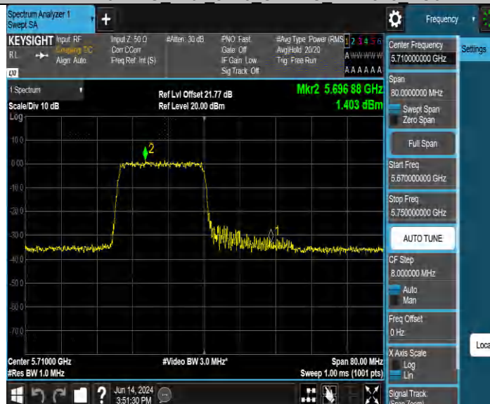
11AX40MIMO_Ant3_5710_UNII-2C_26Tone_RU0
