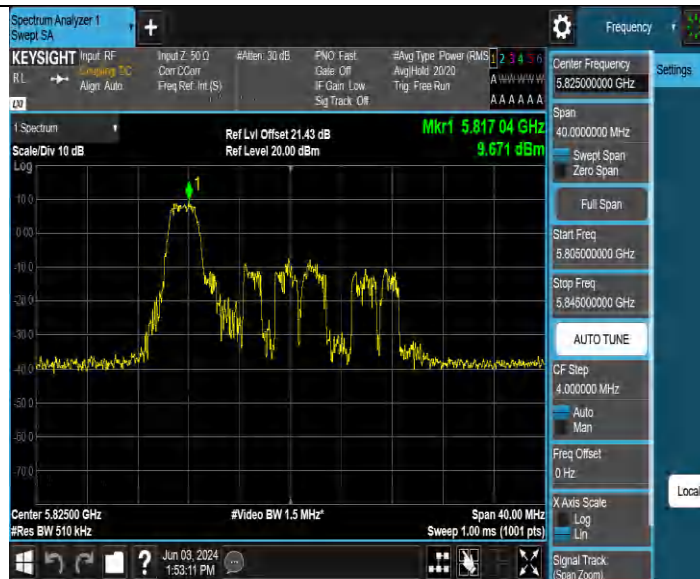
11AX20MIMO_Ant1_5825_106Tone_RU53
