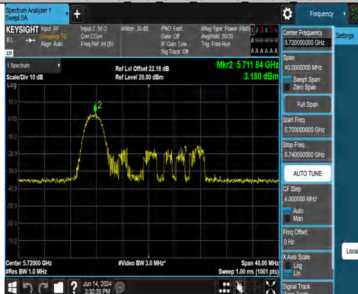
11AX20MIMO_Ant1_5720_UNII-2C_106Tone_RU53
