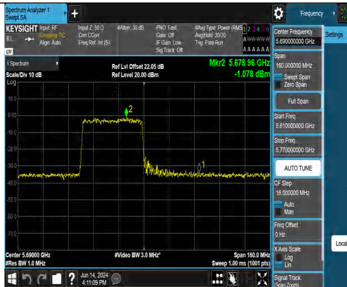
11AX80MIMO_Ant2_5690_UNII-2C_26Tone_RU0
