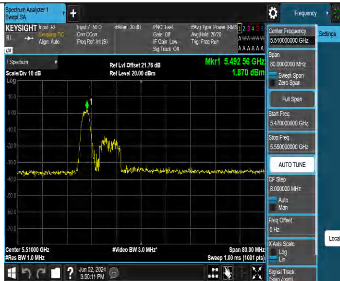
11AX40MIMO_Ant2_5510_242Tone_RU61
