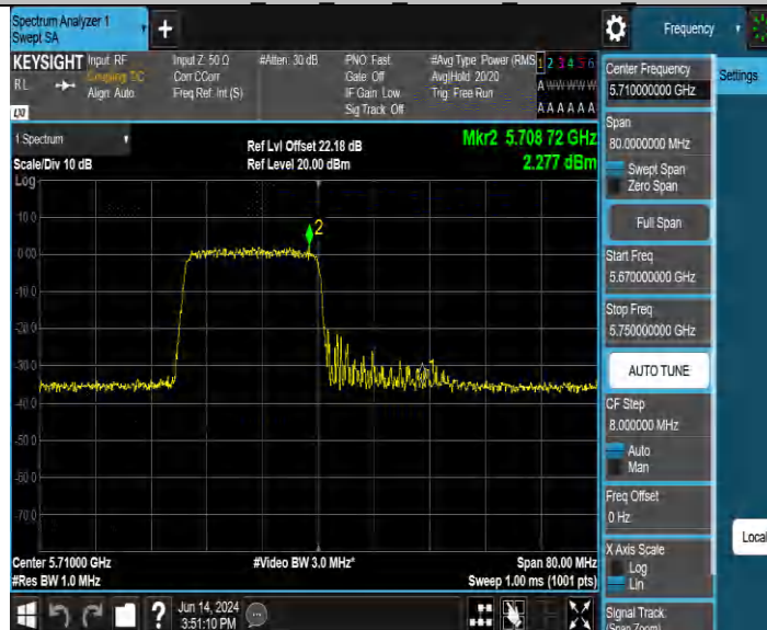
11AX40MIMO_Ant2_5710_UNII-2C_26Tone_RU0
