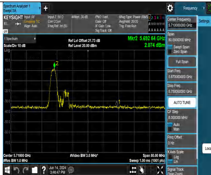
11AX40MIMO_Ant2_5710_UNII-2C_242Tone_RU61
