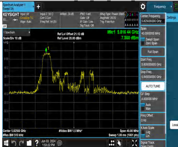
11AX20MIMO_Ant2_5825_106Tone_RU53
