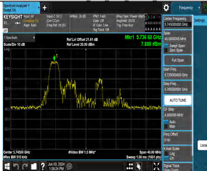
11AX20MIMO_Ant1_5745_106Tone_RU53
