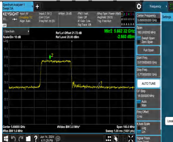
11AX80MIMO_Ant3_5690_UNII-2C_26Tone_RU0
