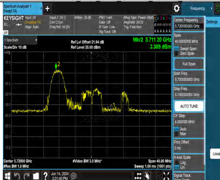
11AX20MIMO_Ant4_5720_UNII-2C_106Tone_RU53
