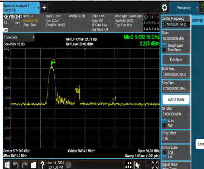
11AX40MIMO_Ant3_5710_UNII-2C_242Tone_RU61
