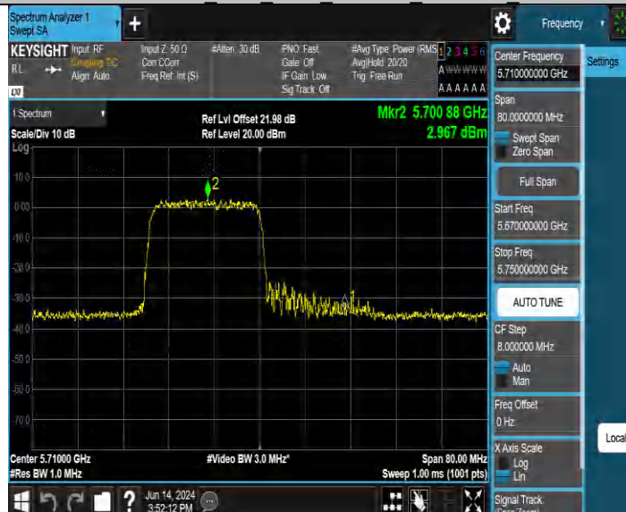
11AX40MIMO_Ant1_5710_UNII-3_26Tone_RU0
