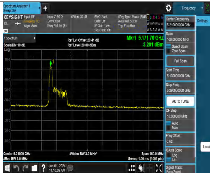
11AX80MIMO_Ant1_5210_484Tone_RU65
