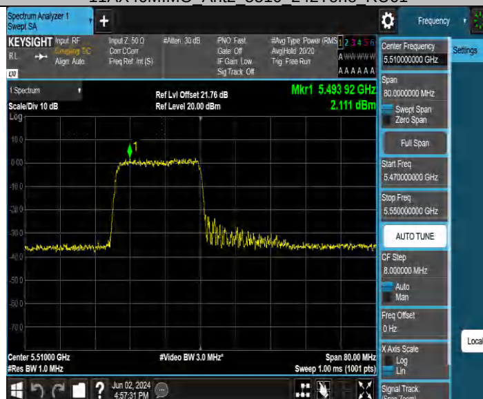
11AX40MIMO_Ant3_5510_26Tone_RU0
