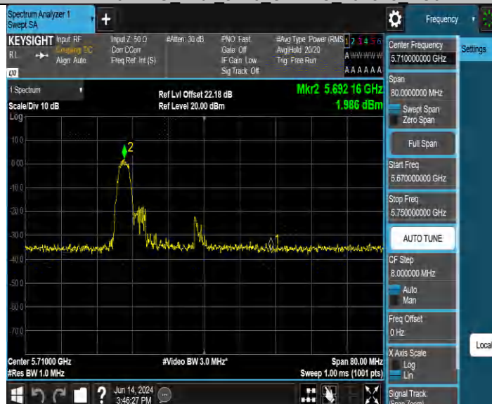
11AX40MIMO_Ant1_5710_UNII-2C_242Tone_RU61
