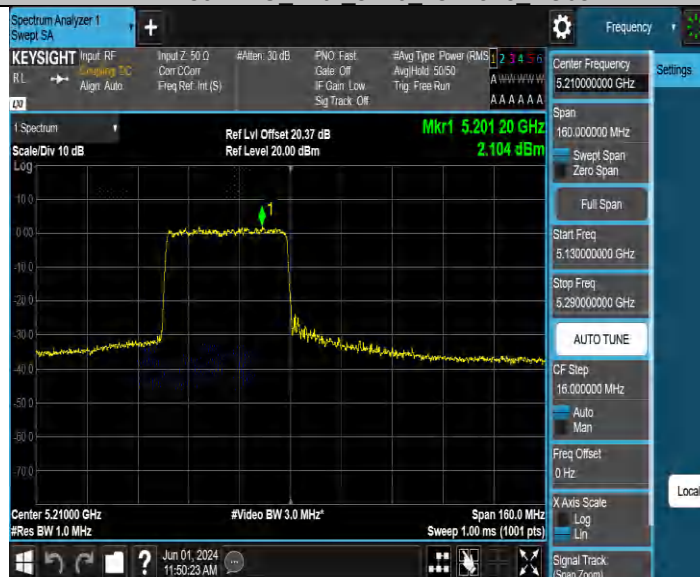
11AX80MIMO_Ant2_5210_26Tone_RU0
