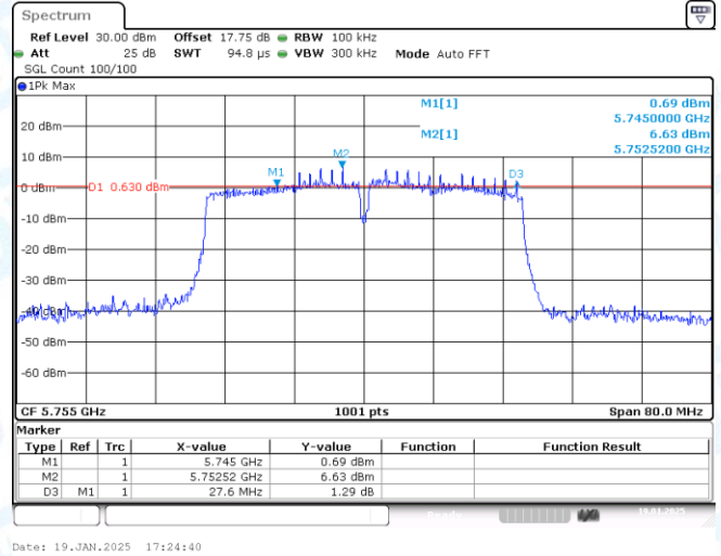
11N40-CDD-Ant2-5755-PASS
