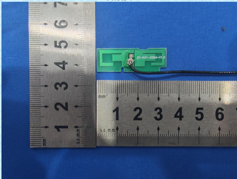
ANT 1
