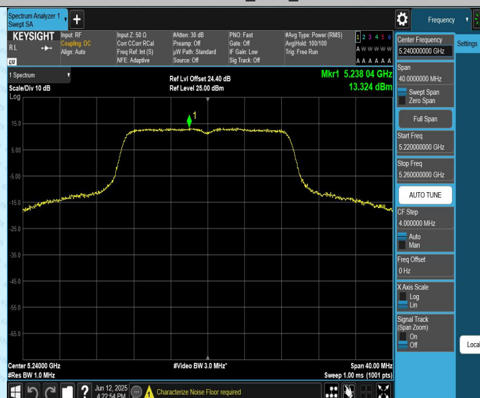
11N20CDD_Ant2_5240
