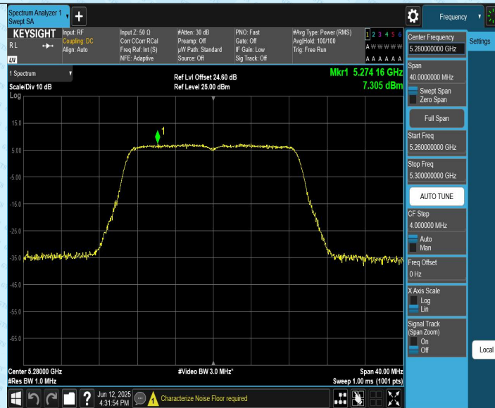
11N20CDD_Ant2_5280
