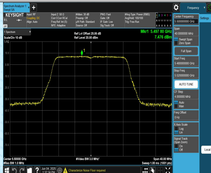
11N20CDD_Ant2_5500
