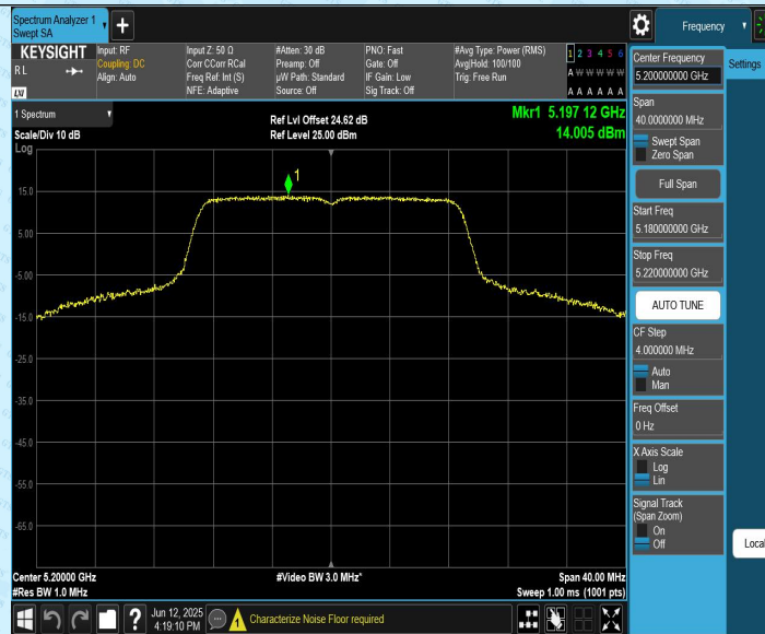
11N20CDD_Ant2_5200
