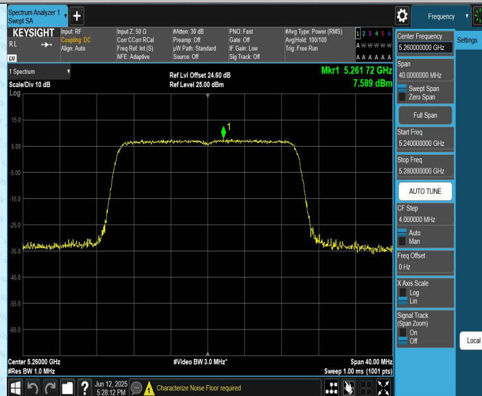
11AX20CDD_Ant2_5260
