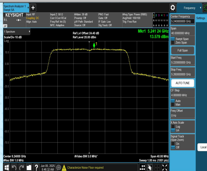
11AX20CDD_Ant2_5240
