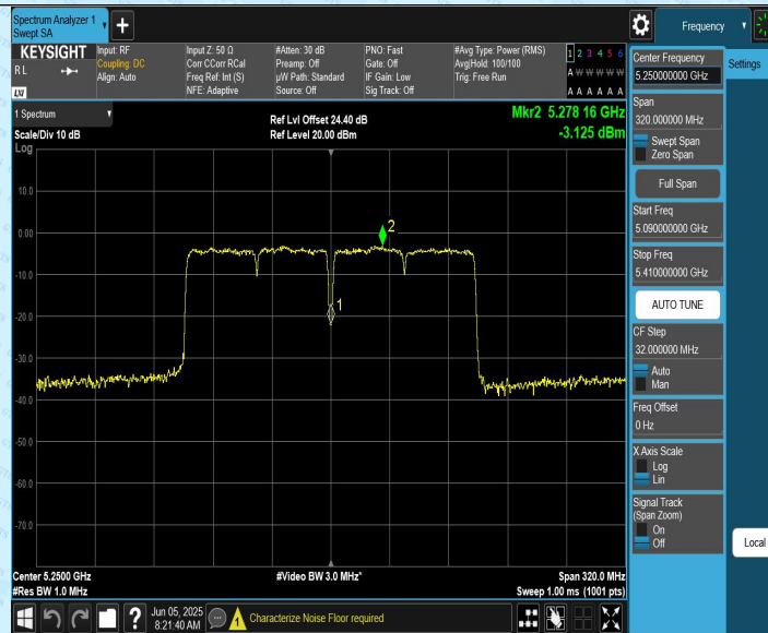
11AC160CDD_Ant2_5250_UNII-2A
