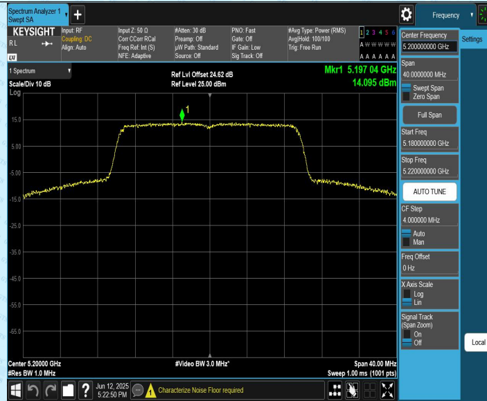
11AX20CDD_Ant2_5200
