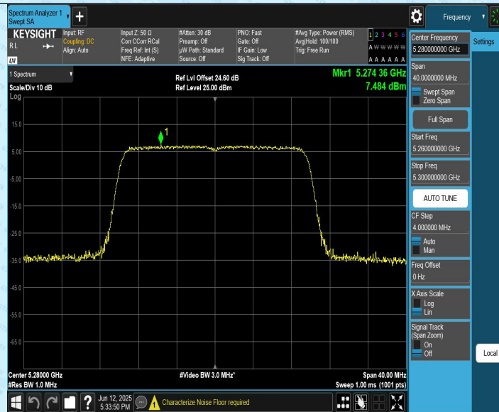
11AX20CDD_Ant2_5280
