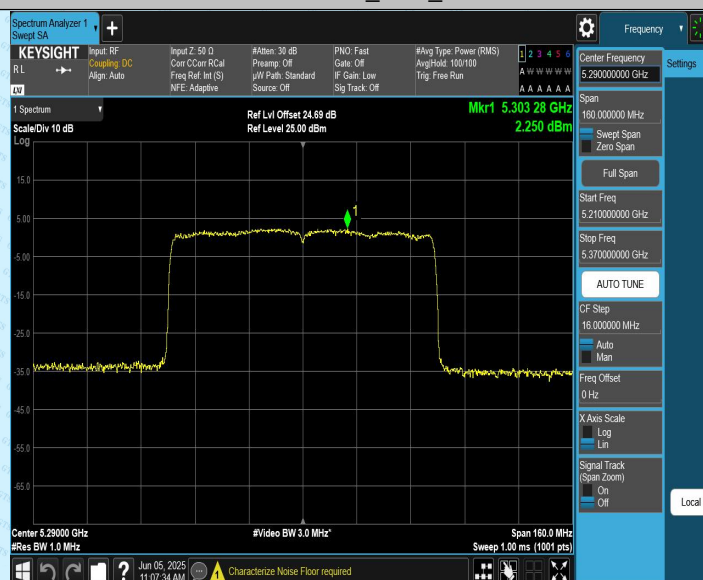
11AX80CDD_Ant2_5290
