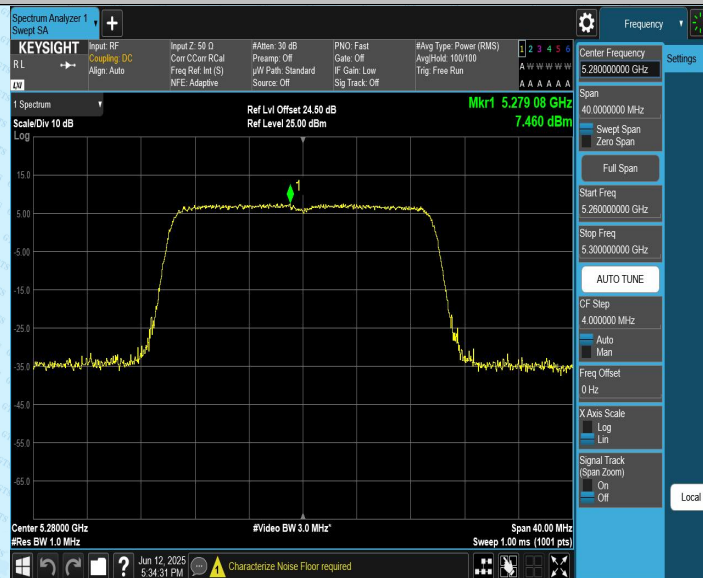
11AX20CDD_Ant1_5320
