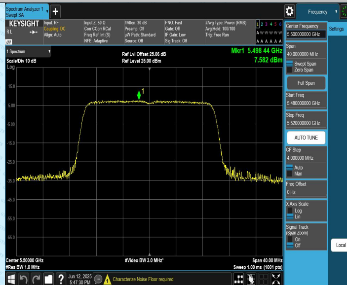
11AX20CDD_Ant2_5500
