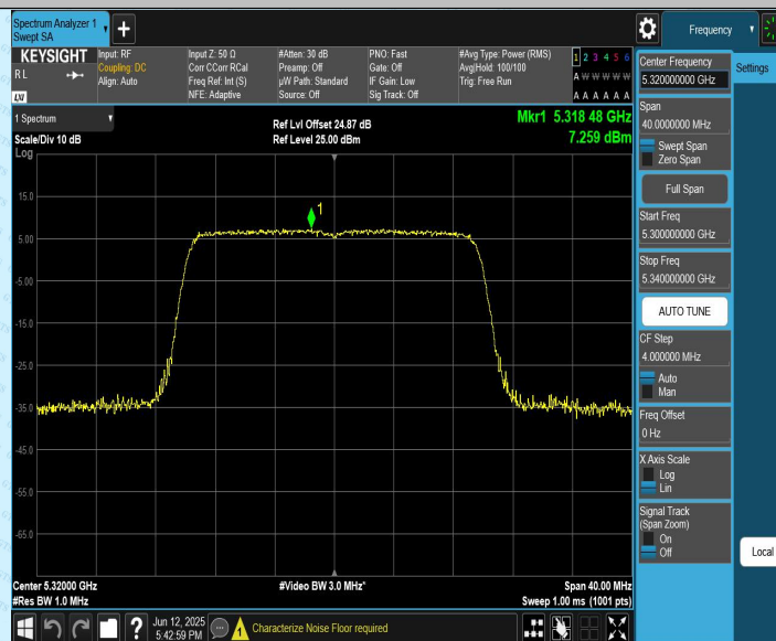
11AX20CDD_Ant2_5320
