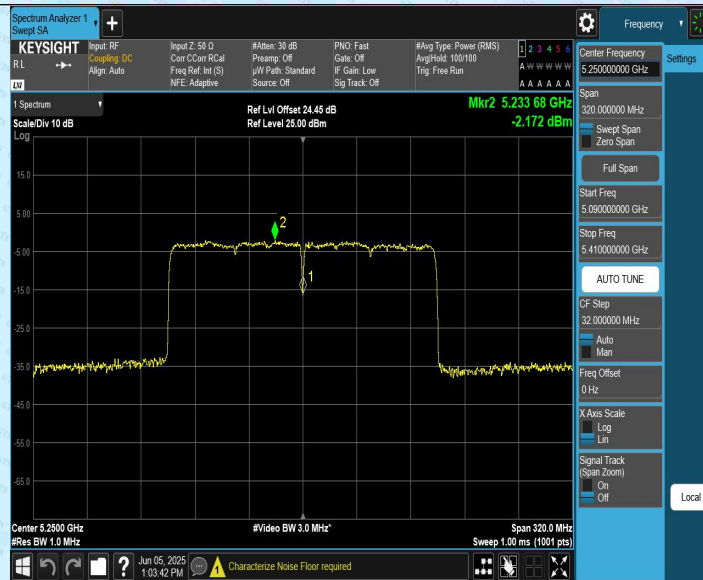
11AX160CDD_Ant1_5250_UNII-2A
