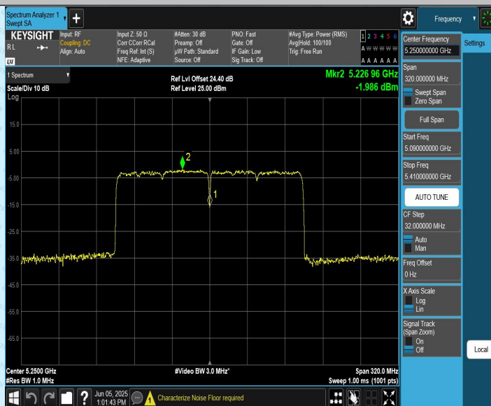
11AX160CDD_Ant2_5250_UNII-1
