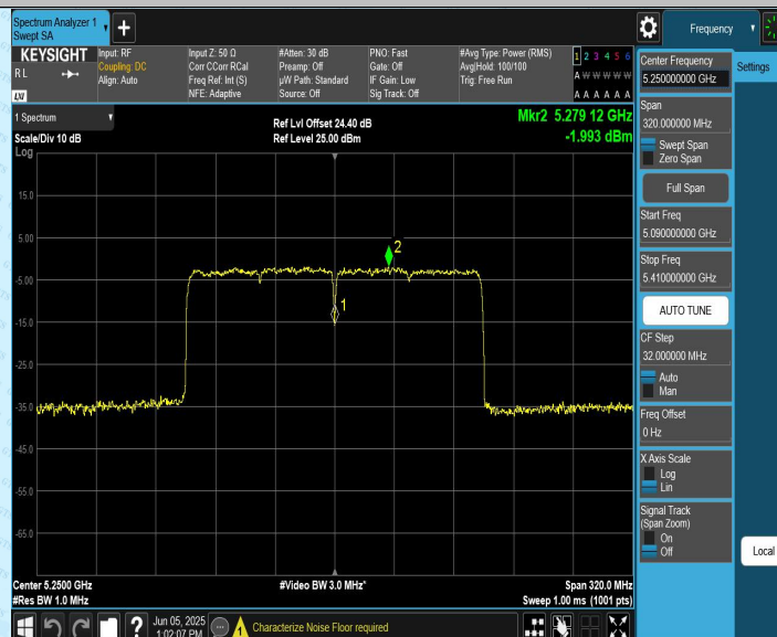
11AX160CDD_Ant2_5250_UNII-2A
