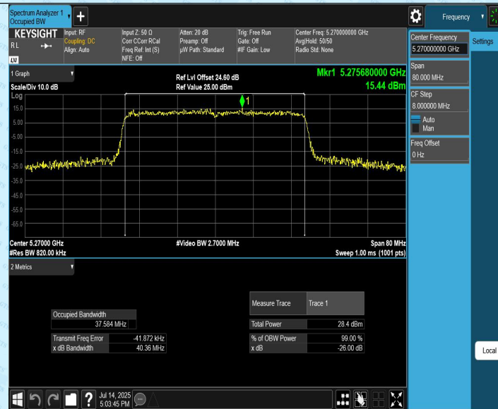
11AX40MIMO_Ant2_5270
