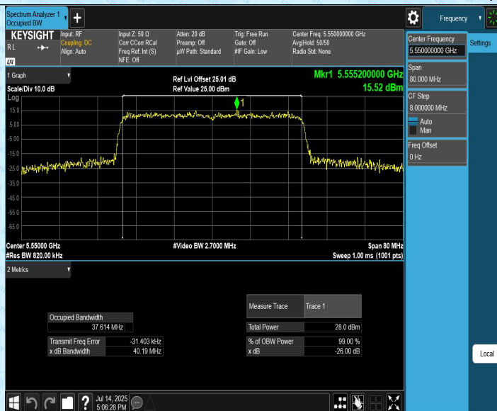
11AX40MIMO_Ant2_5550
