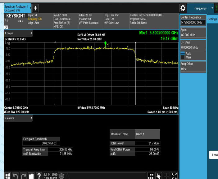
11AX40MIMO_Ant2_5795
