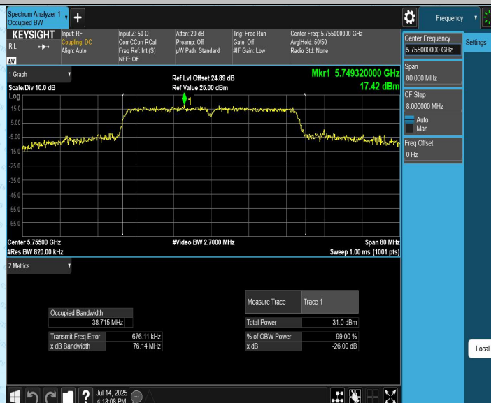
11N40MIMO_Ant2_5755
