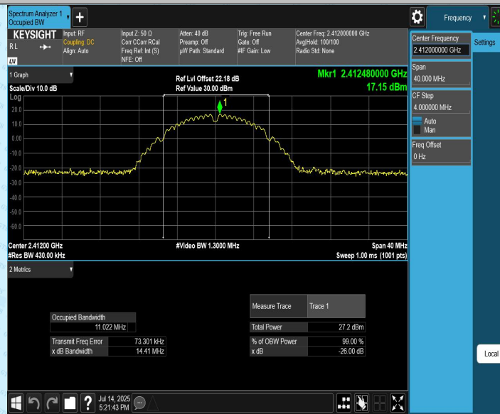
11B-CDD_Ant2_2412
