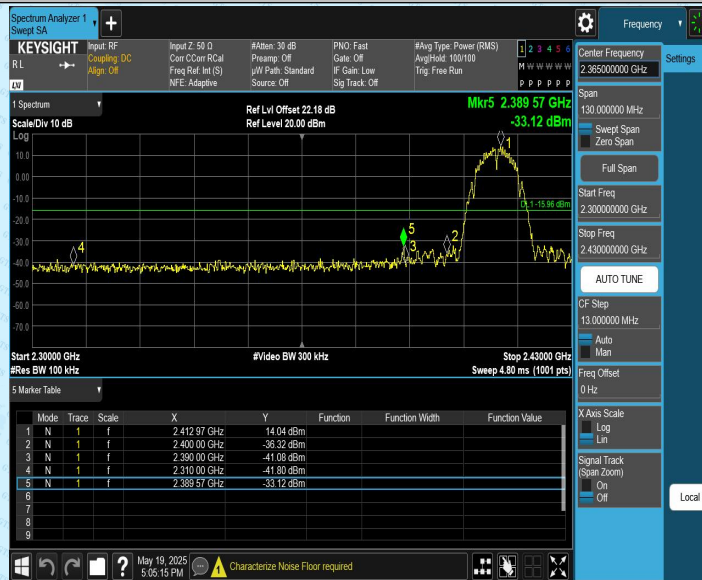
11B-CDD_Ant2_Low_2412
