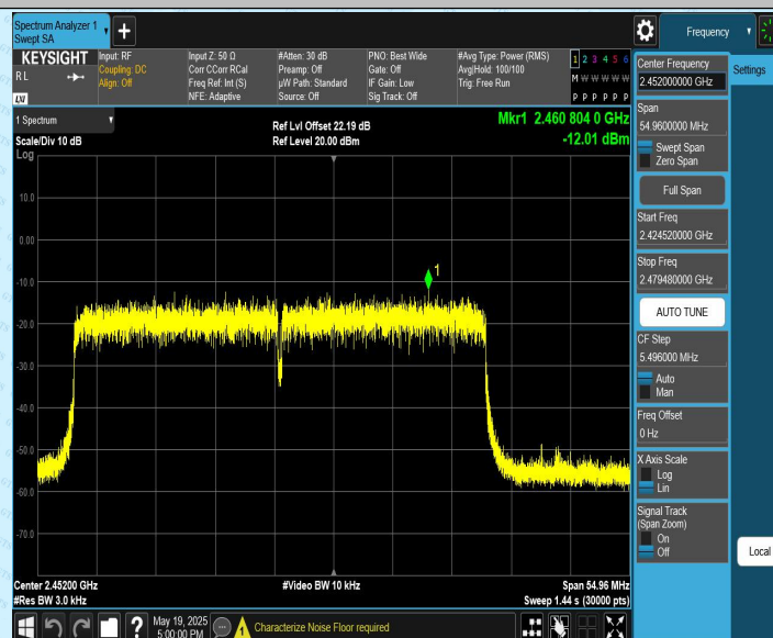
11AX40CDD_Ant2_2452
