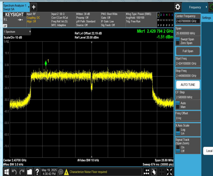
11AX20CDD_Ant2_2437
