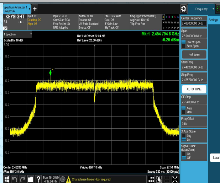
11AX20CDD_Ant2_2462
