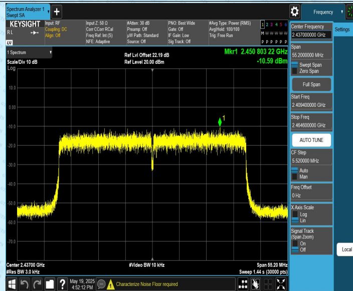
11AX40CDD_Ant2_2437
