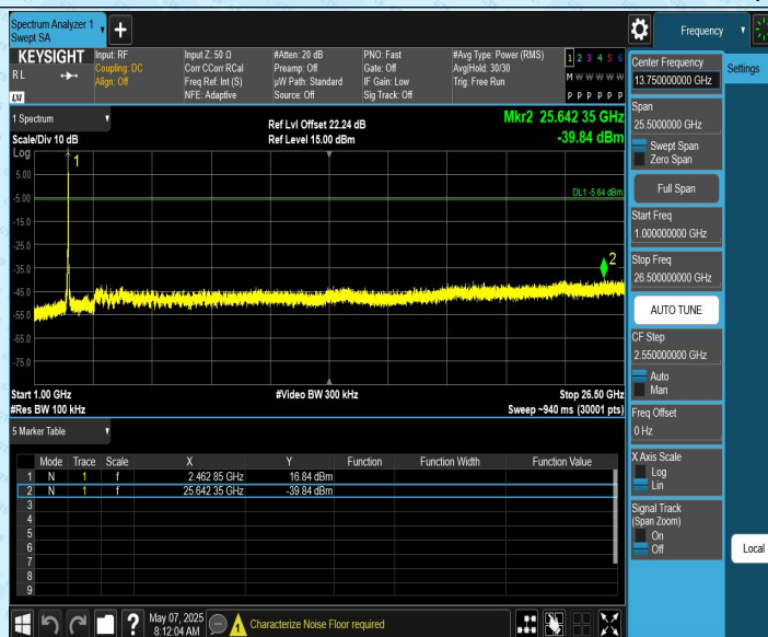
11B-CDD_Ant2_2462_0~Reference
