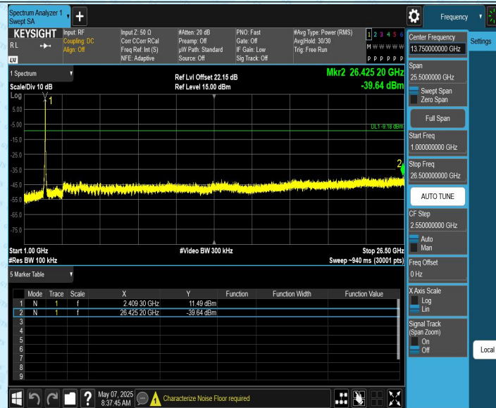
11G-CDD_Ant1_2437_0~Reference
