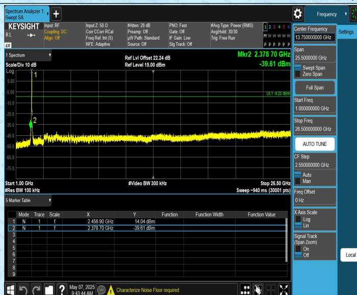
11N20CDD_Ant2_2462_0~Reference
