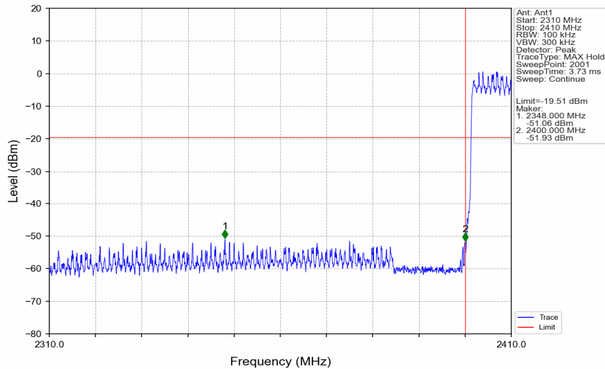
Pi/4DQPSK_2DH5_HOPP_Ant1_NTNV
