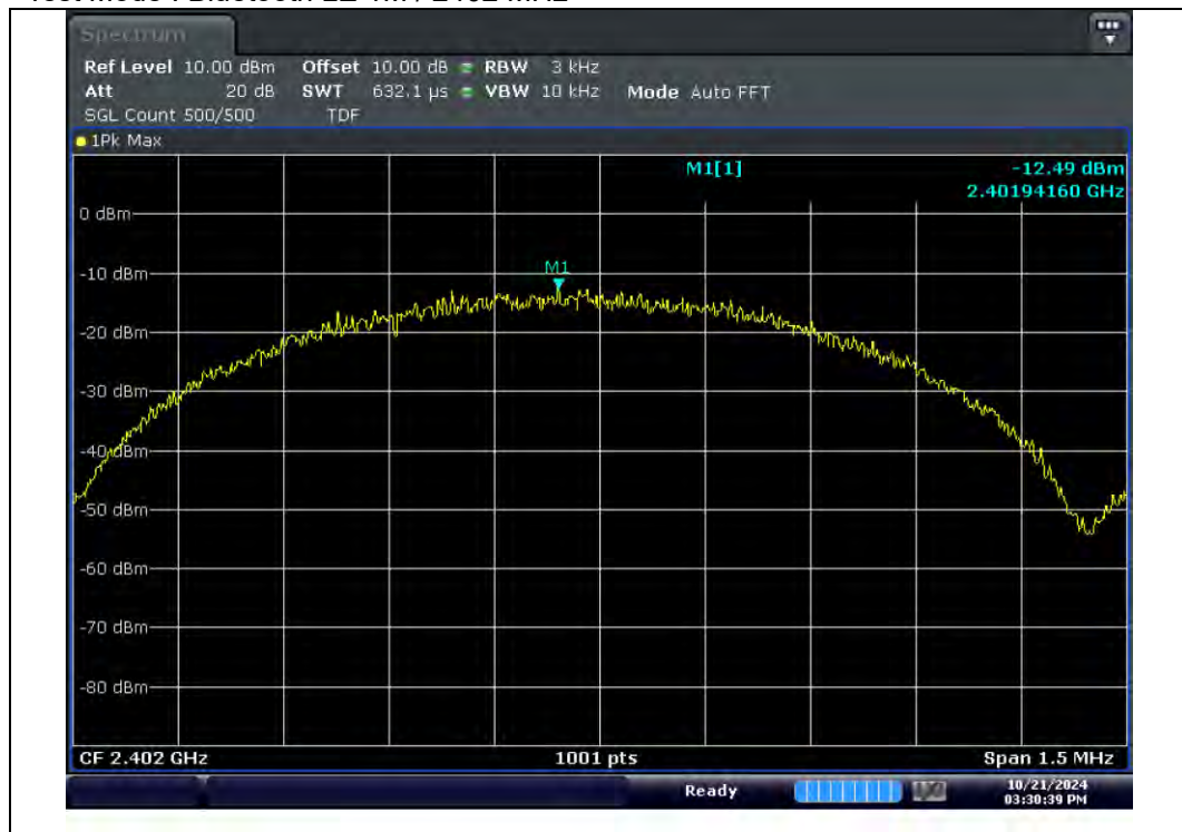
Test Mode : Bluetooth LE 1M / 2402 MHz
