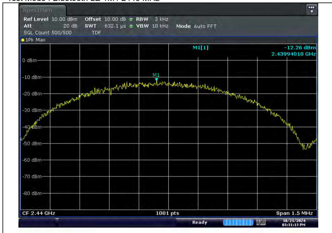
Test Mode : Bluetooth LE 1M / 2440 MHz
