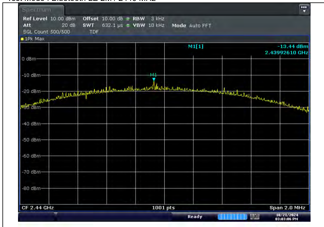
Test Mode : Bluetooth LE 2M / 2440 MHz
