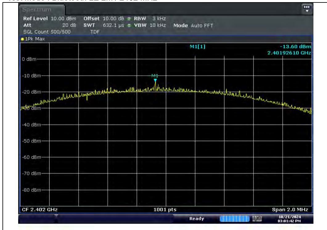
Test Mode : Bluetooth LE 2M / 2402 MHz
