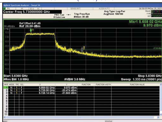
802.11n(HT20)-5700
