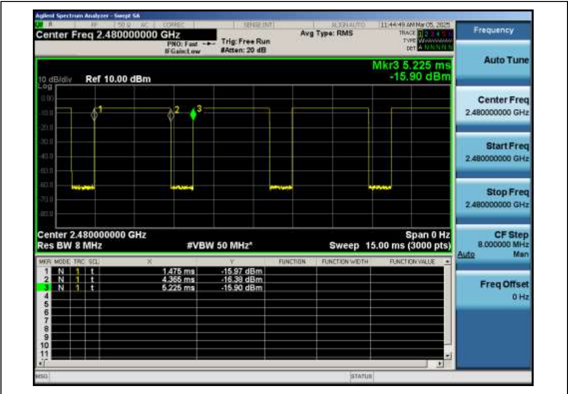
BR-GFSK-Ant1-2480
