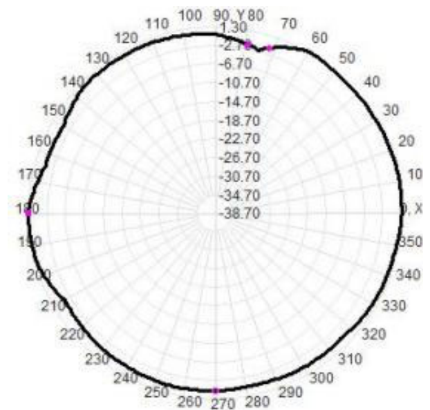
Total(H-xy)
