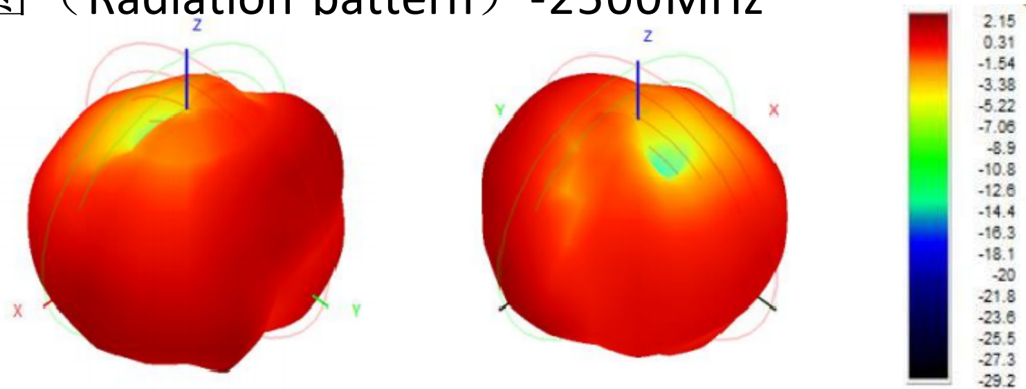
Total(E2-yz)
