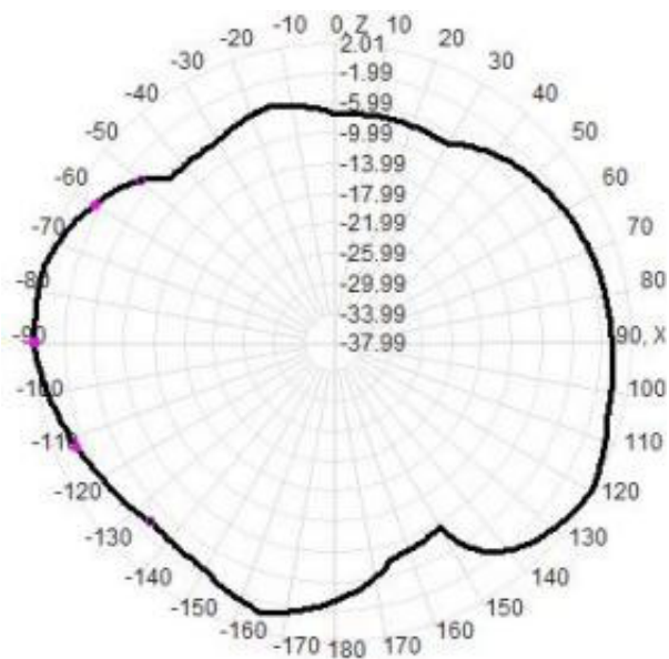
Total(E1-xz)
