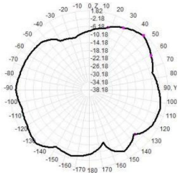
Total(E2-yz)
