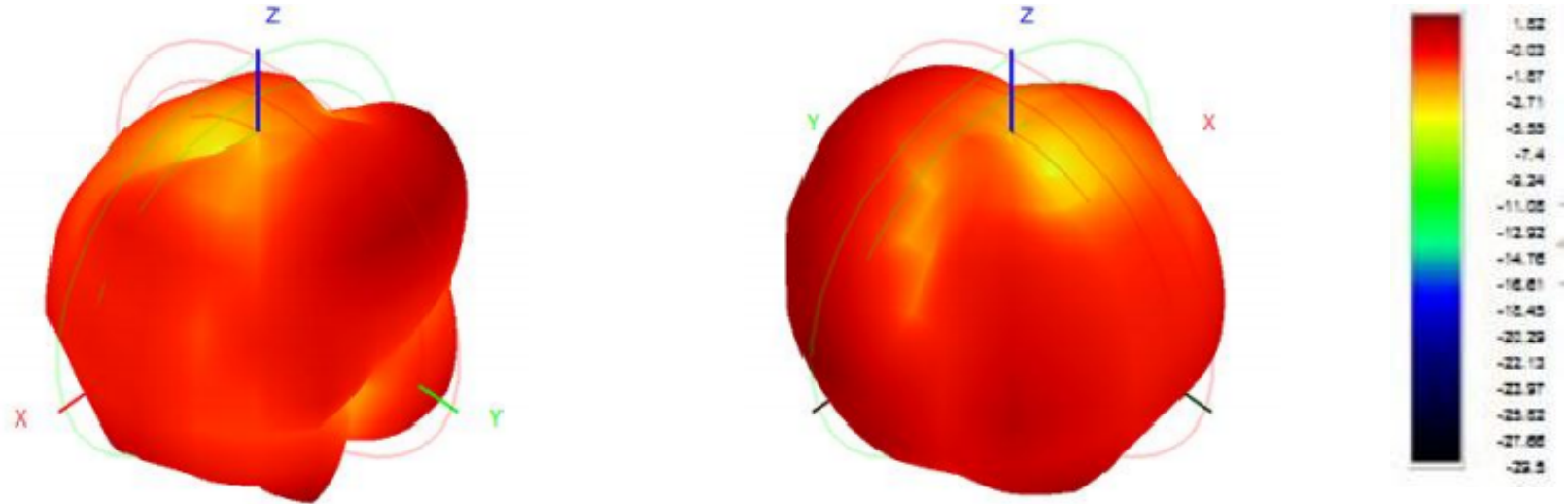
Total(E1-xz)
