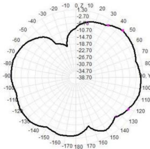
Total(E2-yz)
