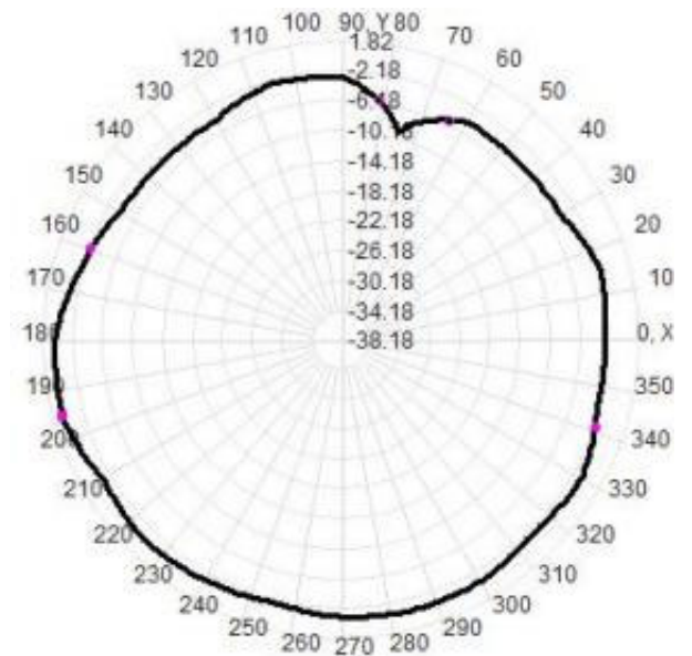
Total(H-xy)
