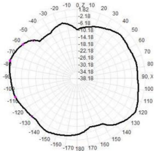
Total(E1-xz)
