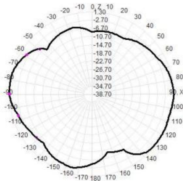
Total(E1-xz)
