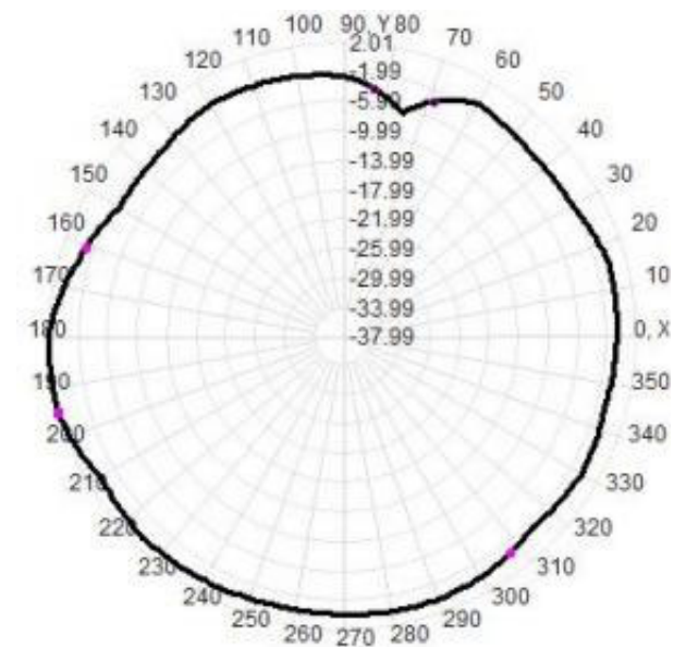
Total(H-xy)
