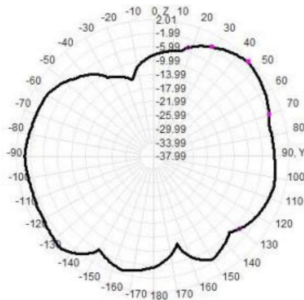
Total(E2-yz)
