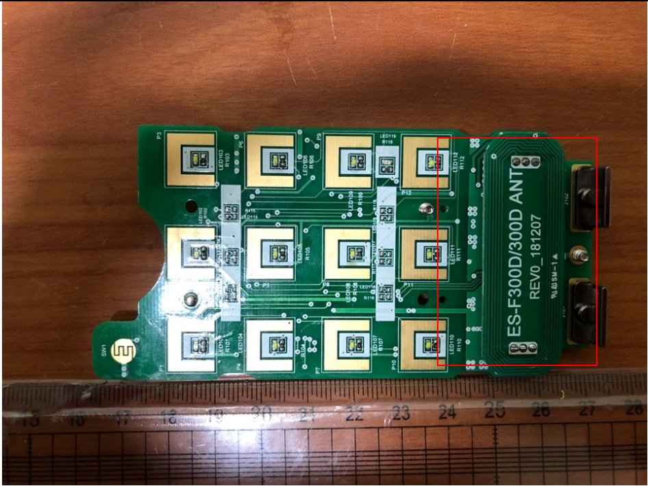
ANTENNA
