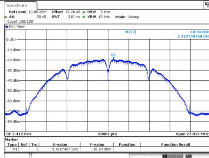
11B_Ant1_2412
